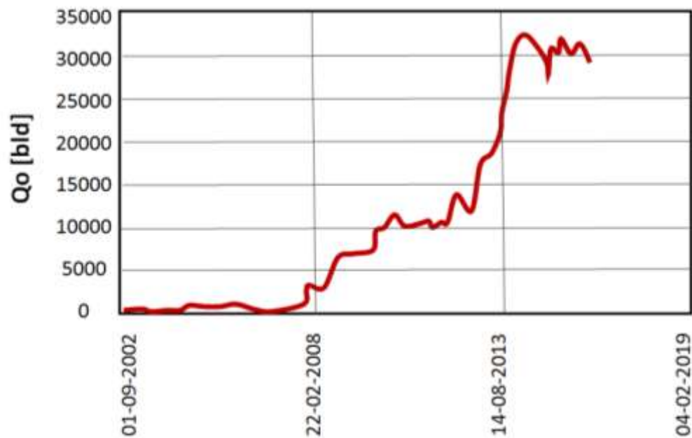
Figura 2.5 Histórico de producción. SAMARIA (Modificado de Flores, 2016)
