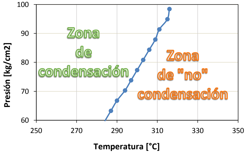
Figura 5.5 Mapa de selección de condiciones ideales de operación (caso base)
