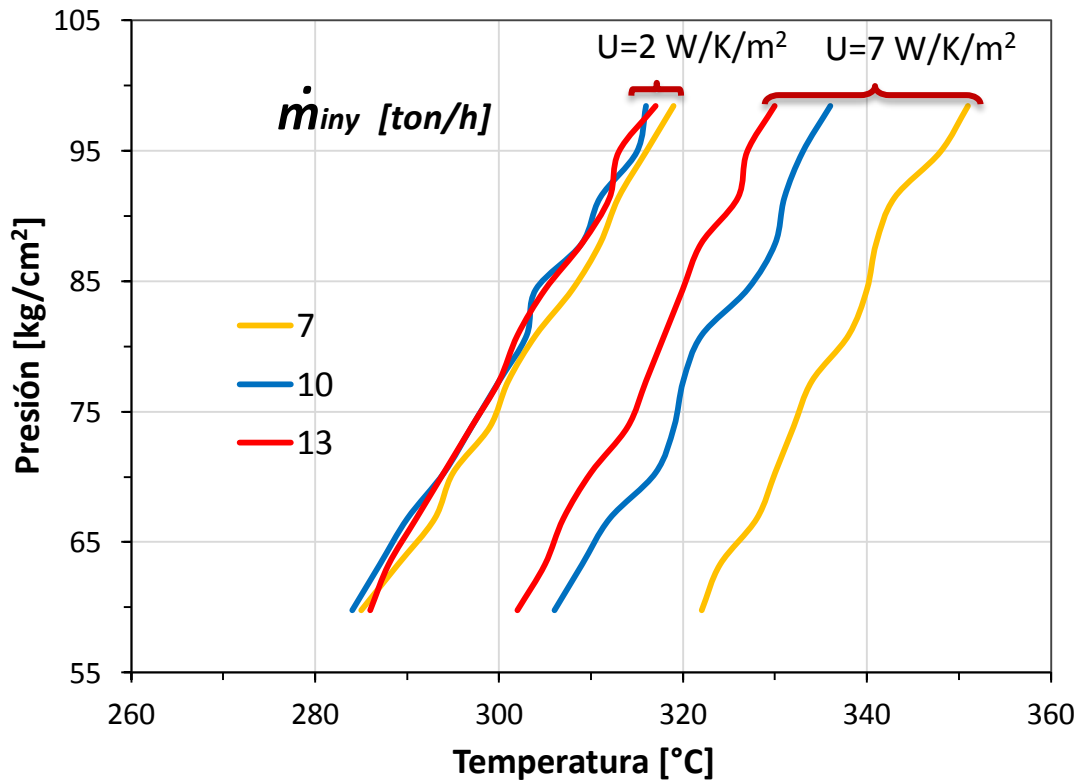
Figura 5.8 Comparación de las fronteras del mapa de selección de condiciones de operación calculadas con diferentes valores del gasto másico de inyección.
