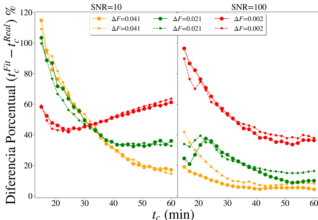
Figura 4.4: Las líneas sólidas representan la diferencia porcentual entre t_c^{Fit} y t_c^{Real} después de aplicar el modelo del trapecoide a los datos filtrados utilizando promedio móvil. Las líneas punteadas representan la misma cantidad, pero obtenida aplicando el modelo del trapecoide a las curvas simuladas sin filtrar. El color representa diferentes valores de \Delta F , se utilizaron 4%, 2% y 0.2% representados en amarillo, verde y rojo respectivamente. Estos resultados se obtuvieron a partir de curvas simuladas a las que se les insertó un ruido con una SNR = 10 .
