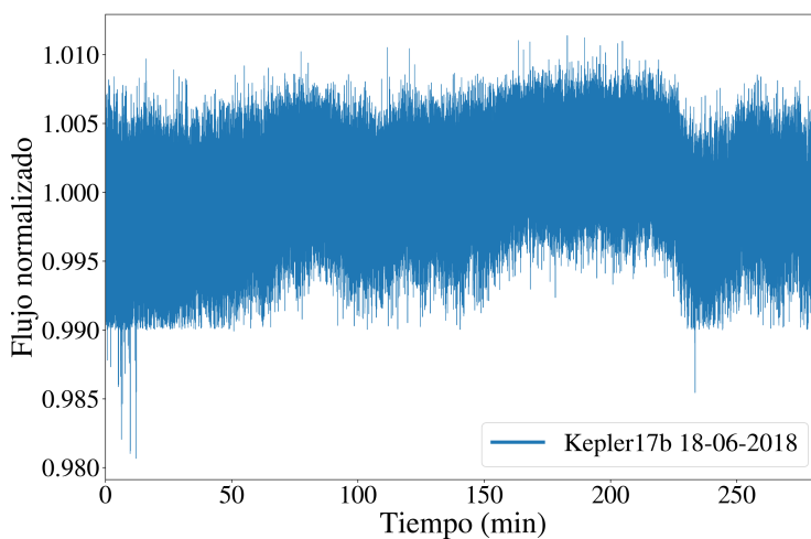
Figura 2.8: Curva de luz de alta cadencia de Kepler-17b obtenida mediante fotometría de apertura. La observación de Kepler-17b se realizó en el sitio 2 de TAOS II, utilizando una cámara Zyla de Andor. Esta curva de luz se obtuvo utilizando APPHi véase (sección III.4.1).
