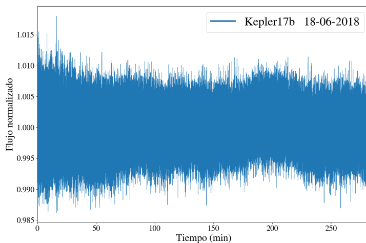
Figura 2.9: Curva de luz de alta cadencia de Kepler-17b obtenida mediante fotometría diferencial. La observación de Kepler-17b se realizó en el sitio 2 de TAOS II, utilizando una cámara Zyla de Andor. Esta curva de luz se obtuvo utilizando APPHi véase (sección III.4.1).
