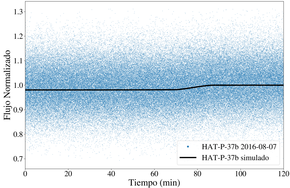
Figura 4.7: Curva de luz de HAT-P-37b tomada a 20 fps, durante la segunda mitad del tránsito. La curva de luz se obtuvo mediante fotometría de apertura con una SNR = 11.73 . La línea negra representa el modelo teórico, utilizando los parámetros presentados en (Bakos et al., 2012).
