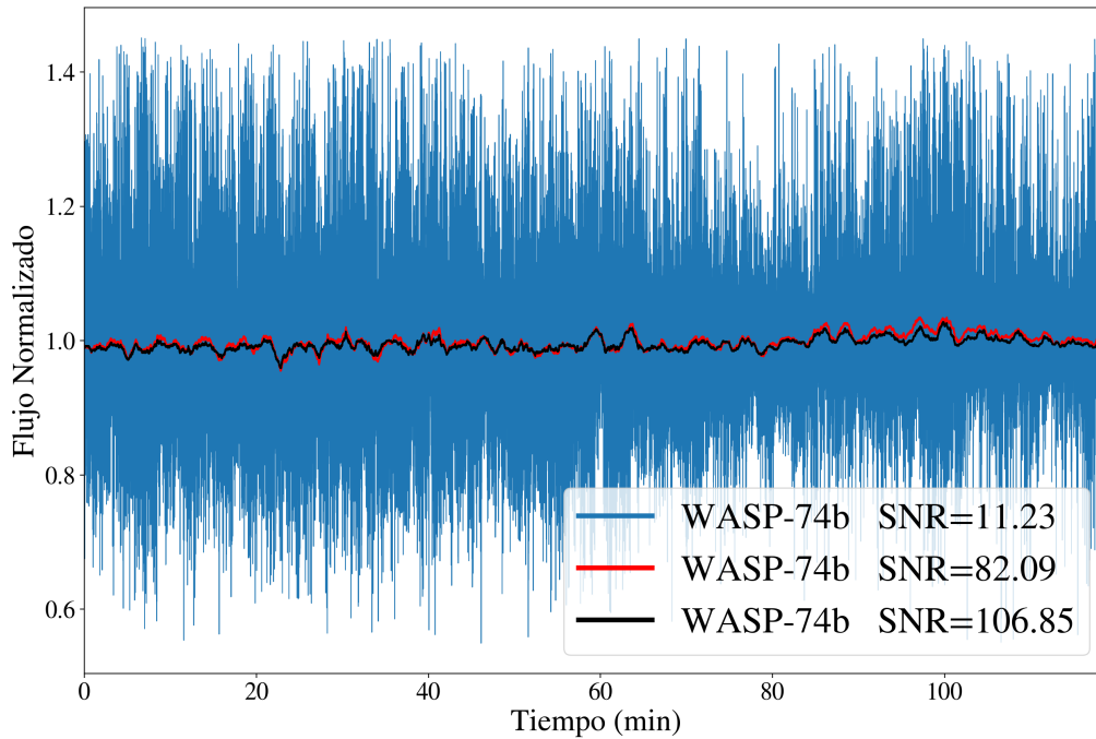
Figura 3.12: Curva de luz de WASP-74 tomada el día 28 de mayo del 2017. En azul se muestra la curva de luz original obtenida mediante fotometría de apertura. En rojo la curva resultado del promedio móvil, y en negro la curva resultado de tomar la mediana en lugar del promedio. En el recuadro se muestra la SNR calculada para cada curva de utilizando (2.11).
