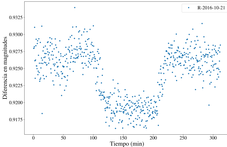
Figura 2.5: Curva de luz de XO-3, tomada con el filtro R de Johnson en el telescopio de 84 cm en el Observatorio Astronómico Nacional (OAN-SPM) el 21 de octubre del 2016.
