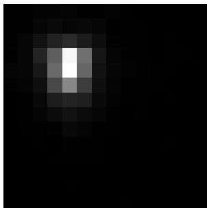
Figura 2.6: Ejemplo de la imagen de una estrella estudiada en este trabajo, obtenida con una cámara rápida IXON en el telescopio de 84 cm en el OAN-SPM.
