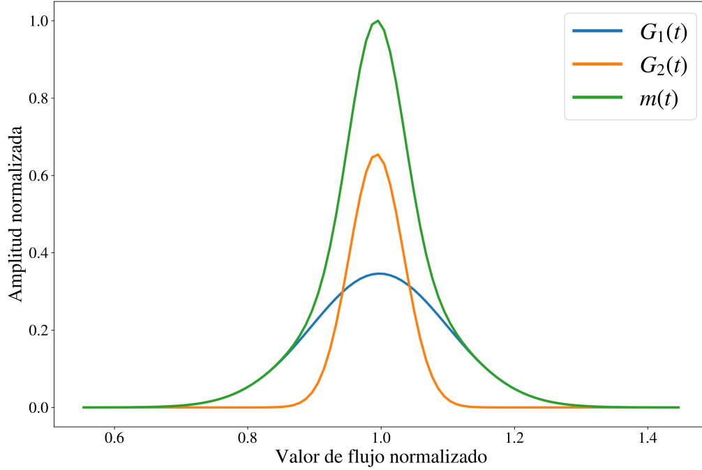
Figura 3.7: Se muestra la contribución de las componentes G_1 y G_2 y la suma m(t) .
