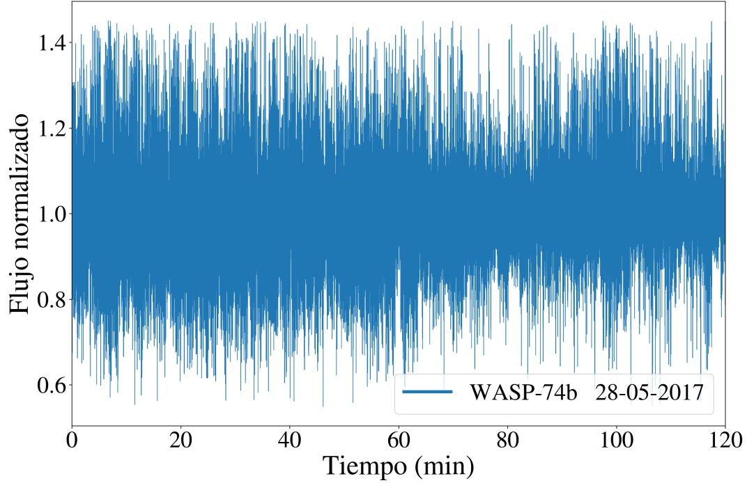
Figura 3.5: Curva de luz de WASP-74b, calculada mediante fotometría diferencial usando APPhI.
