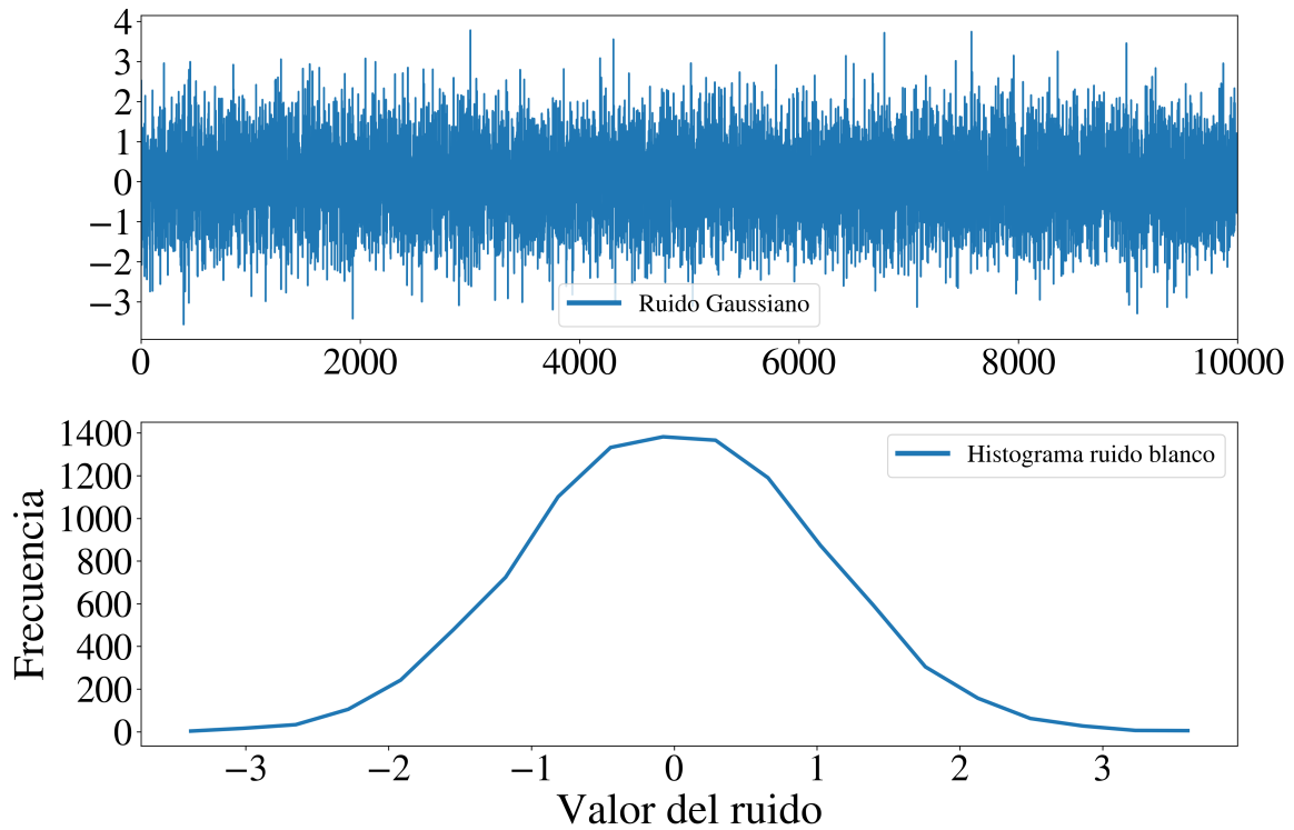
Figura 3.4: Arriba: Ejemplo de ruido blanco (gaussiano). Abajo: Histograma del ruido generado.
