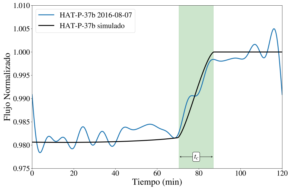
Figura 4.8: Azul: curva de luz de HAT-P-37b después del filtrado de altas frecuencias. La señal a ruido resultante fue de SNR = 124.75 . La línea negra representa el modelo teórico, utilizando los parámetros presentados en (Bakos et al., 2012). El coeficiente de correlación entre la curva y el modelo es C = 0.982 . La región sombreada representa el egreso del planeta del disco solar, la duración de este evento es t_c .
