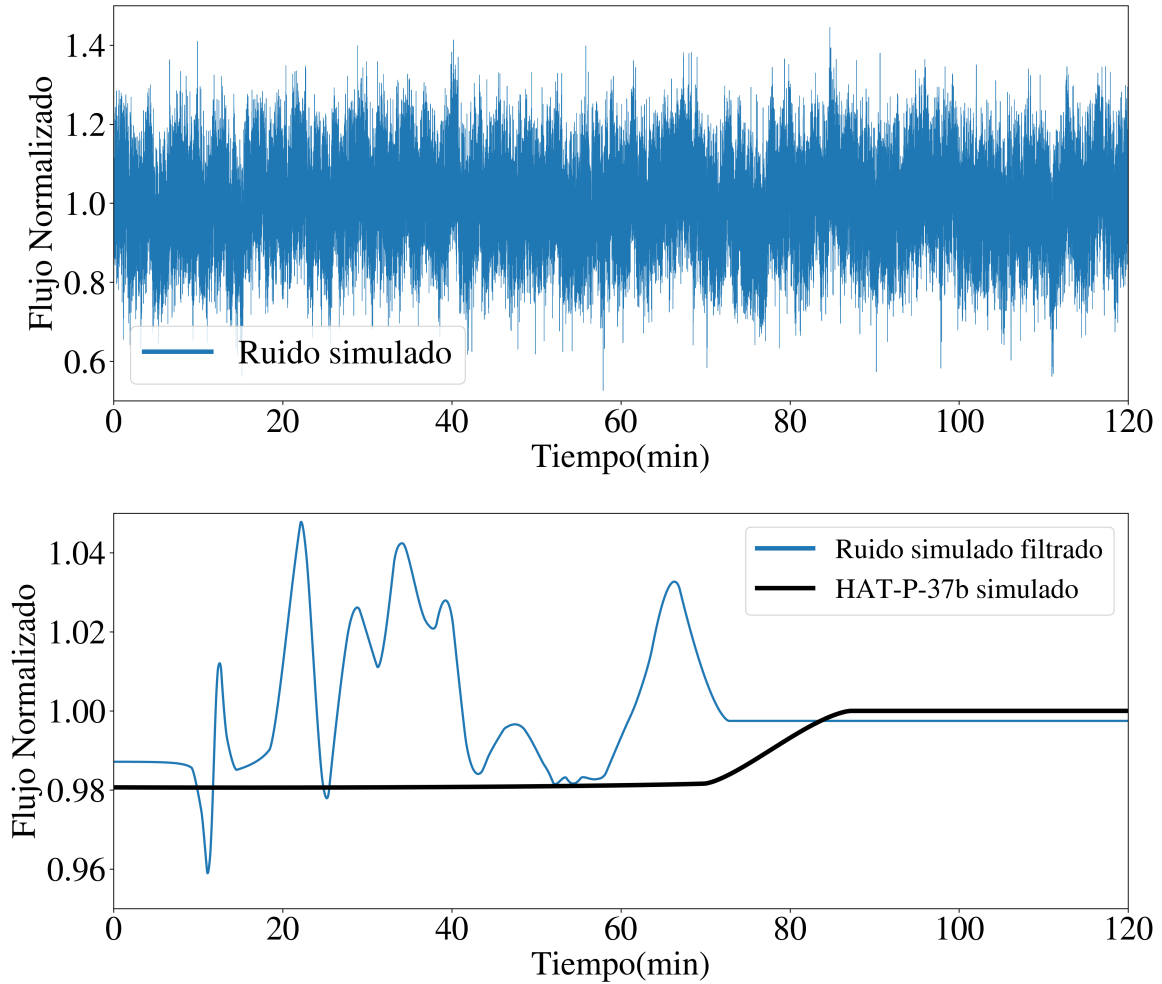
Figura 4.11: Arriba: Ruido simulado con componentes de baja frecuencia en su espectro. Abajo: en azul se muestra el resultado de PCA a una curva sin tránsito inmerso. La línea negra representa el modelo teórico de HAT-P-37b, utilizando los parámetros presentados en (Bakos et al., 2012).
