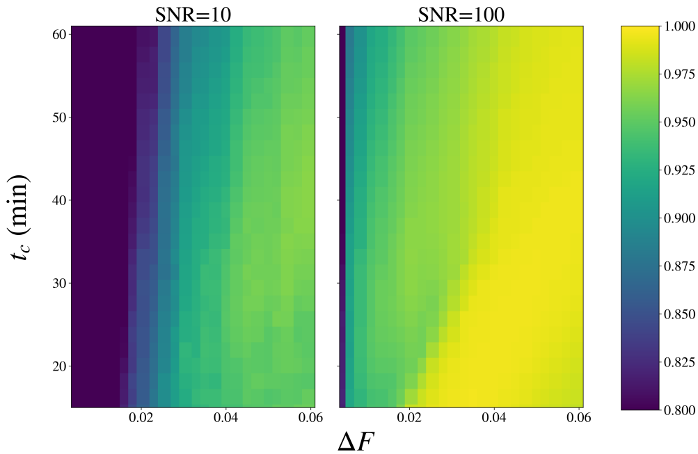
Figura 4.3: Matriz de correlaciones de los parámetros \Delta F y t_c entre las simulaciones y los calculados después de aplicar el modelo del trapecoide a los datos filtrados utilizando promedio móvil. Estos resultados se obtuvieron a partir de curvas con una SNR = 10 y SNR = 100 .
