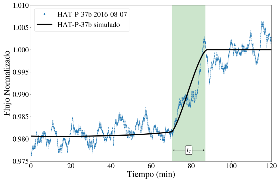
Figura 4.9: Azul: curva de luz de HAT-P-37b después del promedio móvil. La señal a ruido resultante fue de SNR = 116.64 . La línea negra representa el modelo teórico, utilizando los parámetros presentados en (Bakos et al., 2012). El coeficiente de correlación entre la curva y el modelo es C = 0.962 . La región sombreada representa el egreso del planeta del disco solar, la duración de este evento es t_c .
