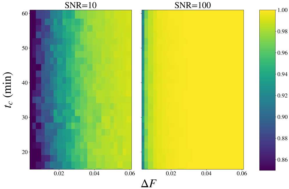
Figura 4.1: Matriz de correlaciones de los parámetros \Delta F y t_c entre las simulaciones y los calculados después de aplicar el modelo del trapecioide a los datos filtrados utilizando Fourier. Estos resultados se obtuvieron a partir de curvas simuladas con una SNR = 10 y SNR = 100 .
