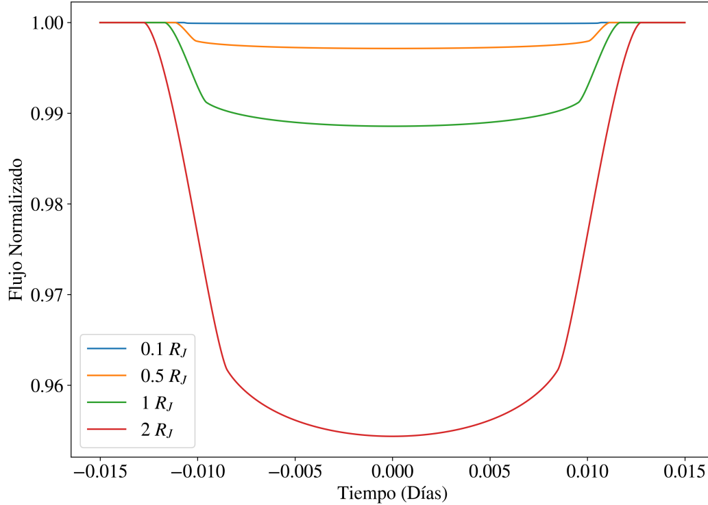
Figura 3.11: Curvas de luz de tránsitos de exoplanetas con P = 1 día, i = 90^\circ , a = 15R_* , \epsilon = 0 , \bar{\omega} = 90 y un modelo de oscurecimiento lineal. Las distintas curvas representan la diferencia en el cambio del flujo \Delta F para diferentes valores de R_p .
