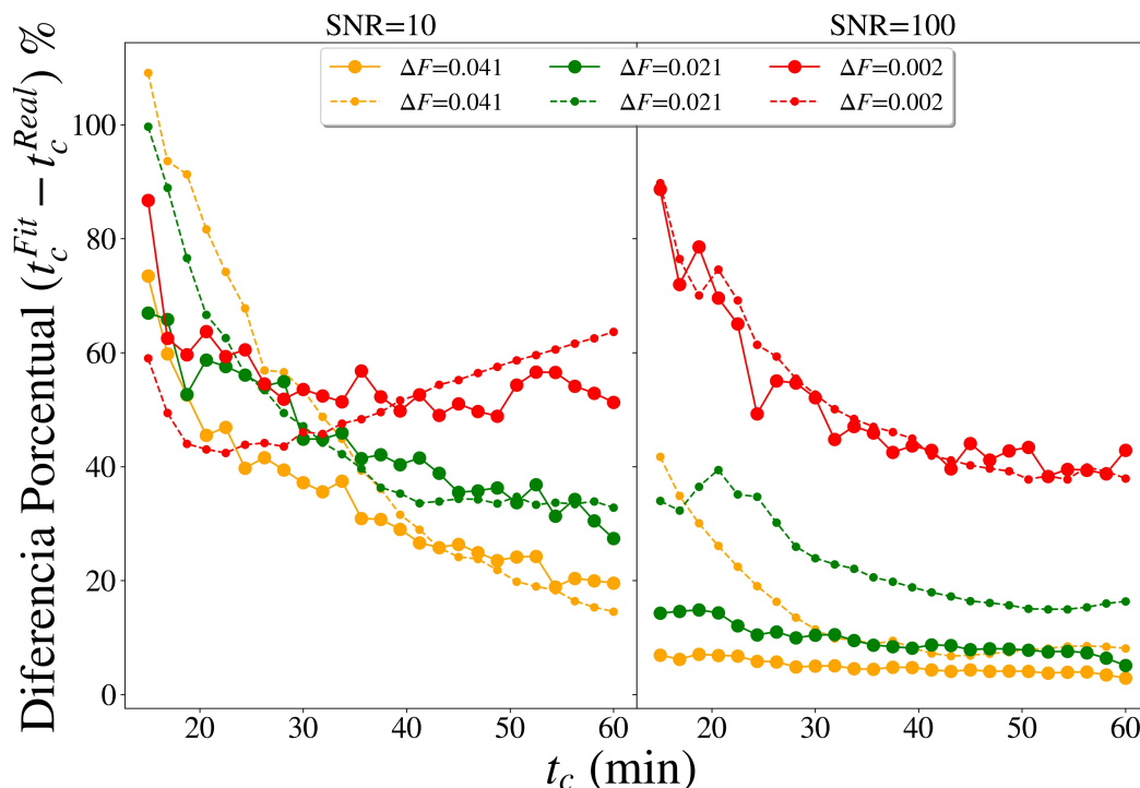
Figura 4.2: Las líneas sólidas representan la diferencia porcentual entre t_c^{Fit} y t_c^{Real} después de aplicar el modelo del trapezoide a los datos filtrados utilizando el filtro pasa bajas. Las líneas punteadas representan la misma cantidad, pero obtenida aplicando el modelo del trapezoide a las curvas simuladas sin filtrar. El color representa diferentes valores de \Delta F , se utilizaron 4%, 2% y 0.2% representados en amarillo, verde y rojo respectivamente. Estos resultados se obtuvieron a partir de curvas simuladas a las que se les insertó un ruido con una SNR = 10 (izquierda) y SNR = 100 (derecha).
