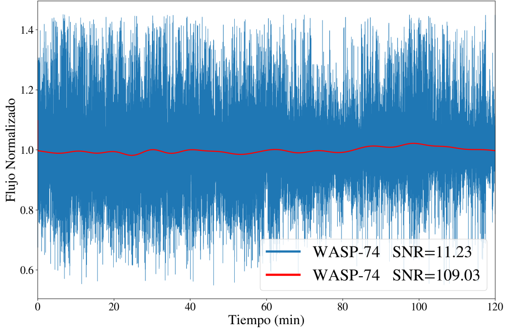
Figura 3.14: Curva de luz de WASP-74 tomada el día 28 de mayo del 2017. En azul se muestra la curva de luz original obtenida mediante fotometría de apertura. En rojo la curva resultado del filtrado de Fourier, utilizando una frecuencia de corte FC = 2 \times 10^{-3} .
