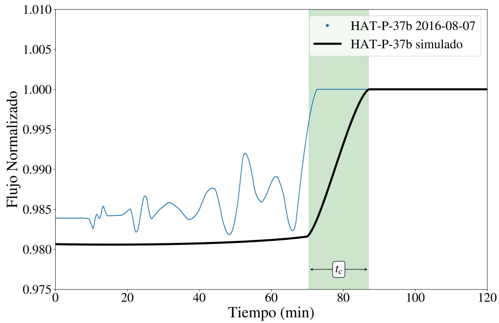
Figura 4.10: Azul: curva de luz de HAT-P-37b después del filtrado con PCA. La señal a ruido resultante fue de SNR = 135.51 . La línea negra representa el modelo teórico, utilizando los parámetros presentados en (Bakos et al., 2012). El coeficiente de correlación entre la curva y el modelo es C = 0.889 . La región sombreada representa el egreso del planeta del disco solar, la duración de este evento es t_c .
