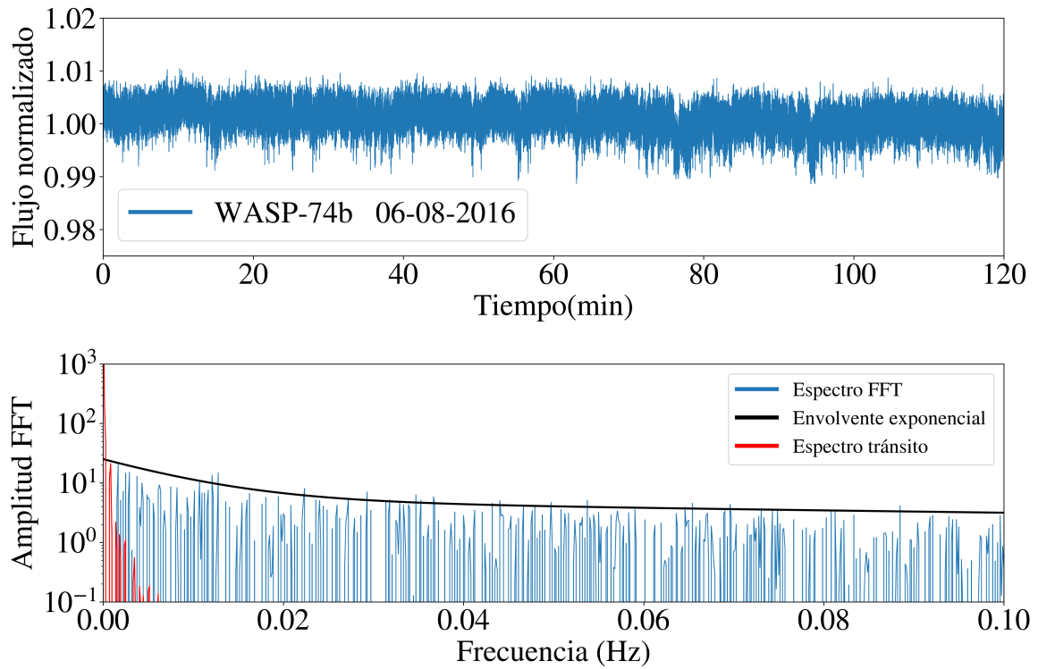
Figura 3.9: Arriba: se muestra una curva de luz de WASP-74b. Abajo: la zona de bajas frecuencias del espectro de la curva de luz, la línea negra es el ajuste de la envolvente exponencial E(f) del espectro. La línea roja indica el espectro del tránsito inmerso en la curva de luz.
