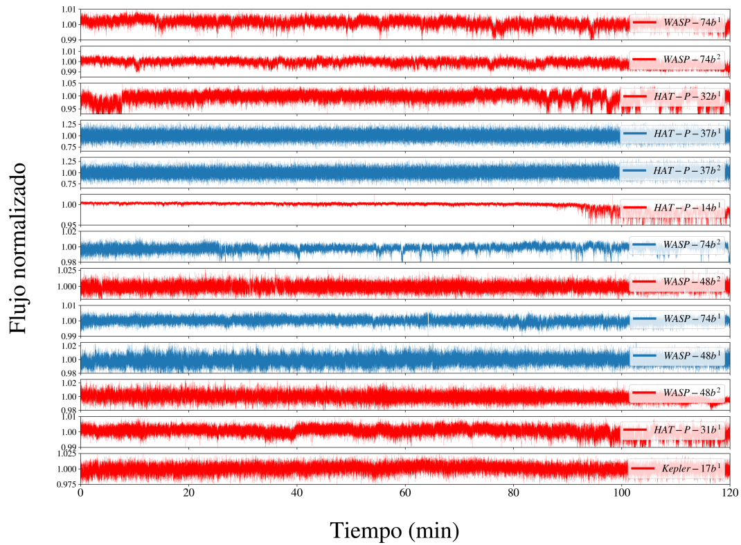
Figura 6.1: Se muestran todas las 13 curvas de luz, a partir de las cuales se encontraron los resultados presentados en la sección IV.2. Las curvas en rojo, son las curvas de luz para las cuales no pudimos detectar el tránsito inmerso en el ruido. Las curvas azules son las observaciones donde si se detectó un tránsito, esto de acuerdo a la tabla 4.1.
