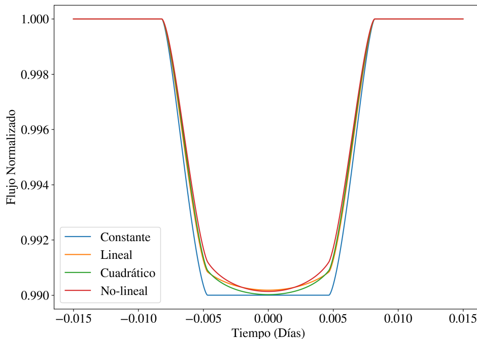
Figura 2.3: Efecto del oscurecimiento del limbo (LD) en curvas de luz de tránsitos simulados. Se muestran 4 modelos distintos, en azul tenemos LD constante, en naranja un modelo lineal, en verde un modelo cuadrático y en rojo un modelo no-lineal.
