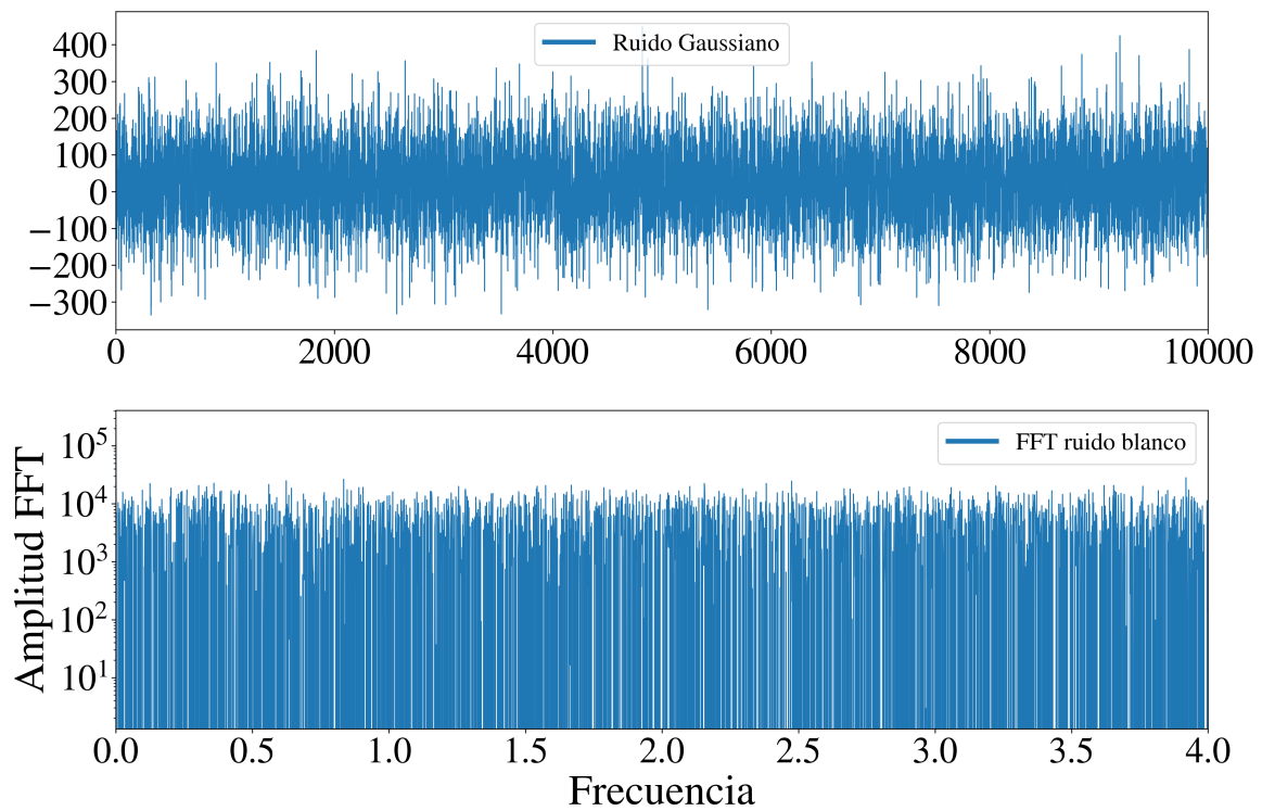
Figura 3.8: Arriba: se muestra una curva de ruido blanco con dos componentes G_1 y G_2 . Abajo: el espectro de frecuencias de la curva de luz, el cual permanece plano sin importar el número de componentes gaussianas.
