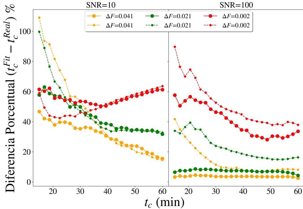
Figura 4.6: Las líneas sólidas representan la diferencia porcentual entre t_c^{Fit} y t_c^{Real} después de aplicar el modelo del trapecoide a los datos filtrados utilizando PCA. Las líneas punteadas representan la misma cantidad, pero obtenida aplicando el modelo del trapecoide a las curvas simuladas sin filtrar. El color representa diferentes valores de \Delta F , se utilizaron 4%, 2% y 0.2% representados en amarillo, verde y rojo respectivamente. Estos resultados se obtuvieron a partir de curvas simuladas a las que se les insertó un ruido con una SNR = 10 (izquierda) y SNR = 100 (derecha).
