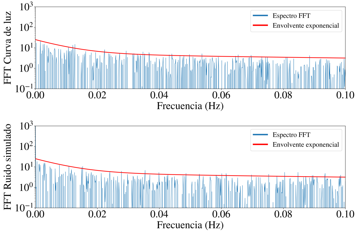
Figura 3.10: Arriba: se muestra la FFT de la curva de luz de WASP-74b. Abajo: el espectro de frecuencias de la serie de tiempo R(t) generada utilizando la metodología planteada en esta sección. Ambas gráficas son un acercamiento a la zona de bajas frecuencias para mejorar la visualización. La línea roja es la misma envolvente exponencial E(f) para ambos espectros.
