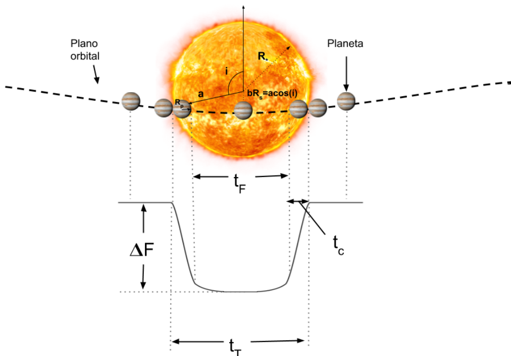
Figura 2.2: Proceso que ocurre durante un tránsito planetario. La curva en la parte inferior representa el flujo de la estrella medido por el observador, i representa la inclinación de la órbita, R_* es el radio de la estrella, R_p el radio del planeta, \Delta F es el cambio en el flujo visto por el observador, t_T es la duración total del tránsito y b el parámetro de impacto.
