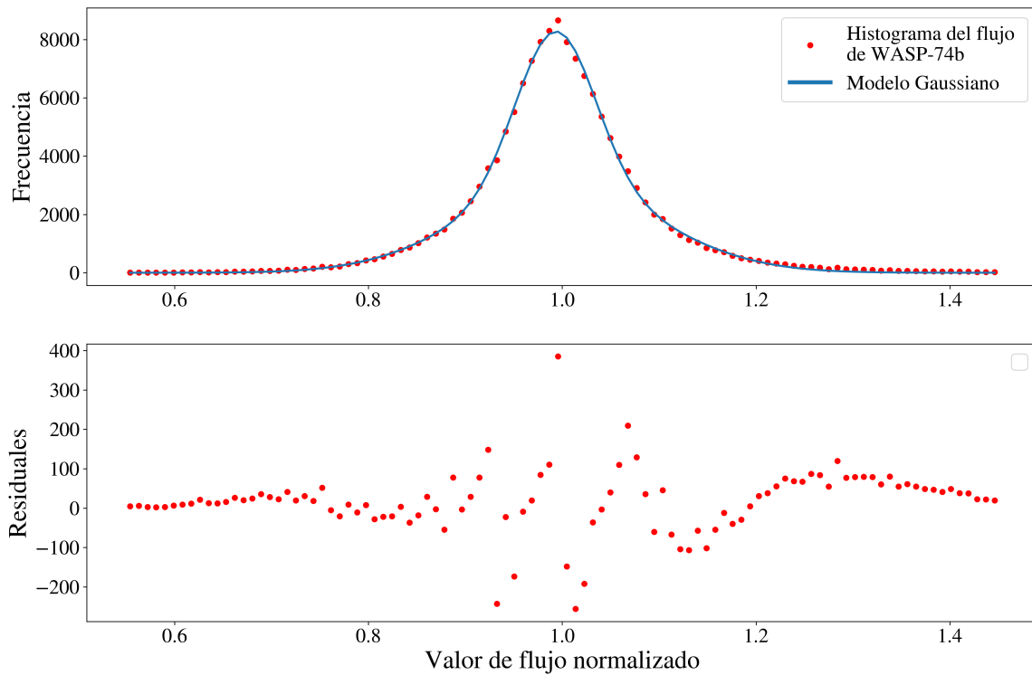
Figura 3.6: Arriba: Los puntos rojos son la distribución temporal de la curva de luz de WASP-74b. La línea azul sólida, es m(t) resultado de un ajuste no lineal utilizando el algoritmo de Levenberg-Marquardt. Abajo: se aprecia los residuales de la diferencia entre la distribución y el modelo.
