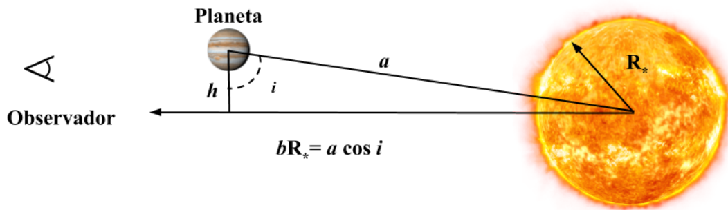
Figura 2.1: Esquema de un tránsito de exoplaneta observable. i representa la inclinación de la órbita y R_* es el radio de la estrella. b es el parámetro de impacto, esta cantidad adimensional es utilizada para resumir la información de la inclinación de la órbita y el semi eje de la órbita a .
