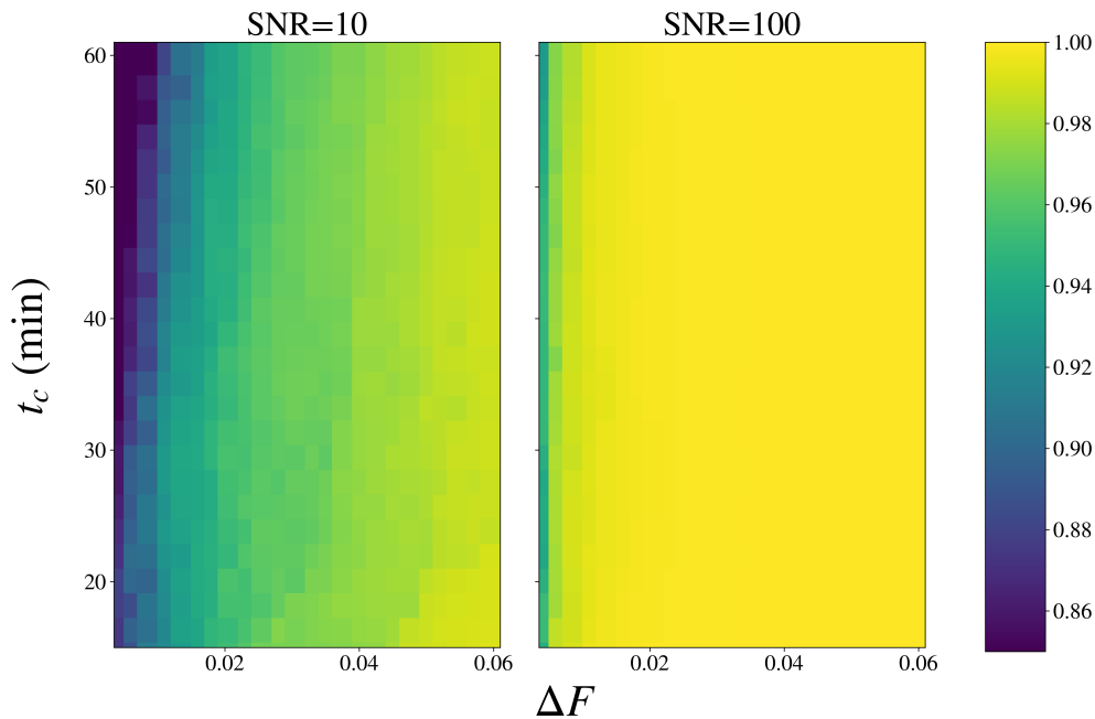
Figura 4.5: Matriz de correlaciones de los parámetros \Delta F y t_c entre las simulaciones y los calculados después de aplicar el modelo del trapecioide a los datos filtrados utilizando PCA. Estos resultados se obtuvieron a partir de curvas con una SNR = 10 y SNR = 100 .
