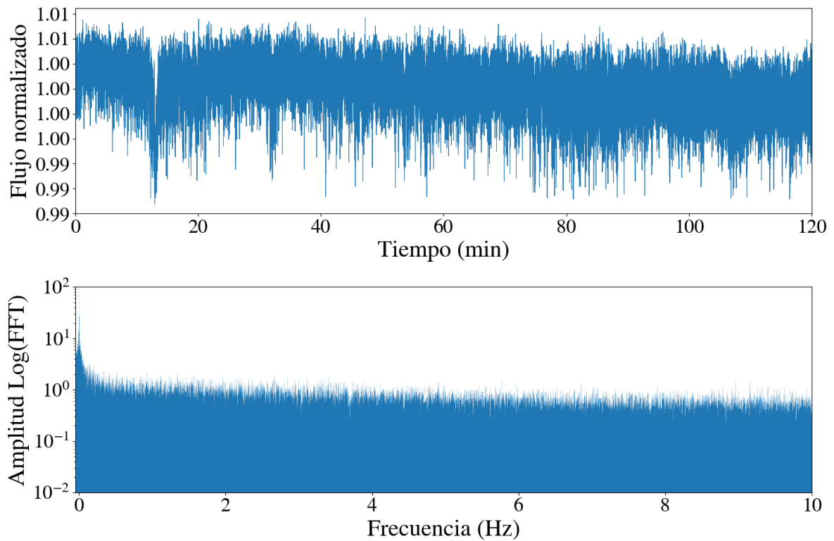
Figura 2.10: Arriba: Curva de luz de alta cadencia de HAT-p-14b, tomada a 20Hz, con el telescopio de 84cm del OAN. Abajo: mostramos su espectro de frecuencias (FFT), con la amplitud en escala logarítmica para mejorar la visualización.
