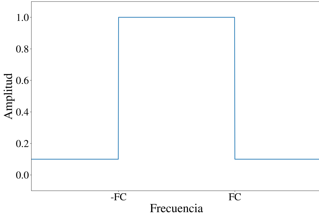
Figura 3.13: Filtro pasa-bajas \mathcal{H}(f) utilizado para remover altas frecuencias. FC representa la frecuencia de corte la cual puede variar dependiendo la curva de luz.
