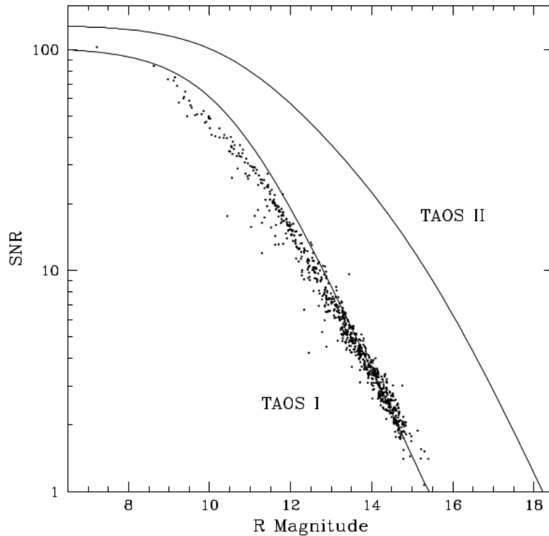
Figura 3.2: SNR en función de la magnitud en el filtro R. Los puntos representan la SNR medida utilizando curvas de luz obtenidas en TAOS I. Las líneas sólidas representan la predicción de SNR utilizando ruido con distribución de Poisson, ruido del cielo y ruido de lectura. Gráfica tomada de (Lehner et al., 2016).
