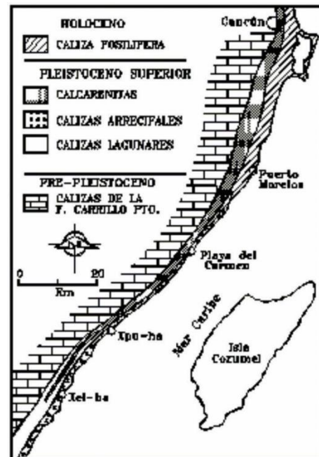
Fig.: 5.1 Mapa geológico general de la costa este de la Península de Yucatán. (Modificado por W. C. Ward y J. Brady 1979)
