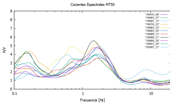
Figura D.3. Cocientes espectrales de los acelerogramas de la estación MT50 de 1995 a 2000.
