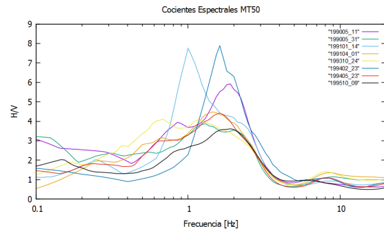
Figura D.2. Cocientes espectrales de los acelerogramas de la estación MT50 de 1990 a 1995.
