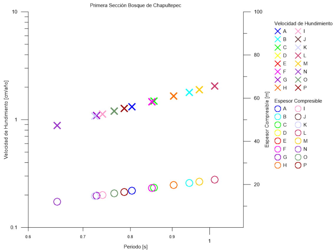
Figura 3.17. Correlación entre el periodo de vibración del suelo, velocidad de hundimiento y espesor de la capa compresible de las mediciones realizadas en la Primera Sección del Bosque de Chapultepec
