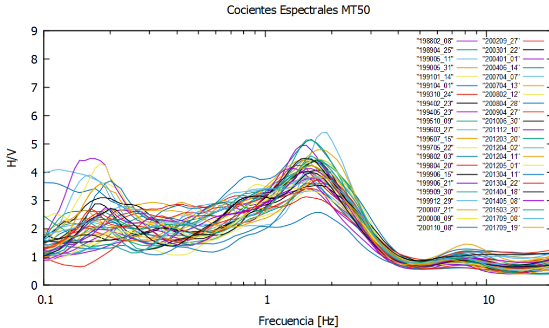
Figura 3.4. Cocientes espectrales de los sismos registrados en la estación MT50 de 1988 a 2017, considerando la señal completa de los acelerogramas analizados.
