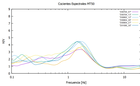
Figura C.5. Cocientes espectrales de los acelerogramas de la estación MT50 de 2005 a 2010.
