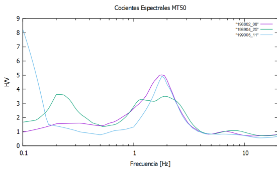
Figura E.1. Cocientes espectrales de los acelerogramas de la estación MT50 de 1988 a 1990.
