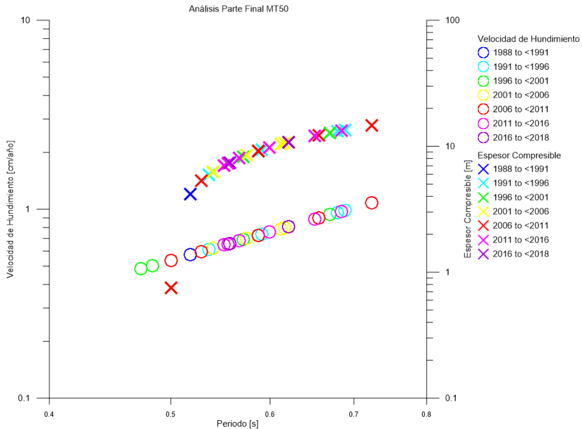
Figura 3.14. Correlación entre el periodo de vibración del suelo, velocidad de hundimiento y espesor de la capa compresible, considerando la parte final de los sismos registrados en la estación MT50.
