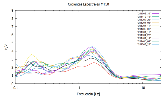
Figura C.6. Cocientes espectrales de los acelerogramas de la estación MT50 de 2010 a 2015.
