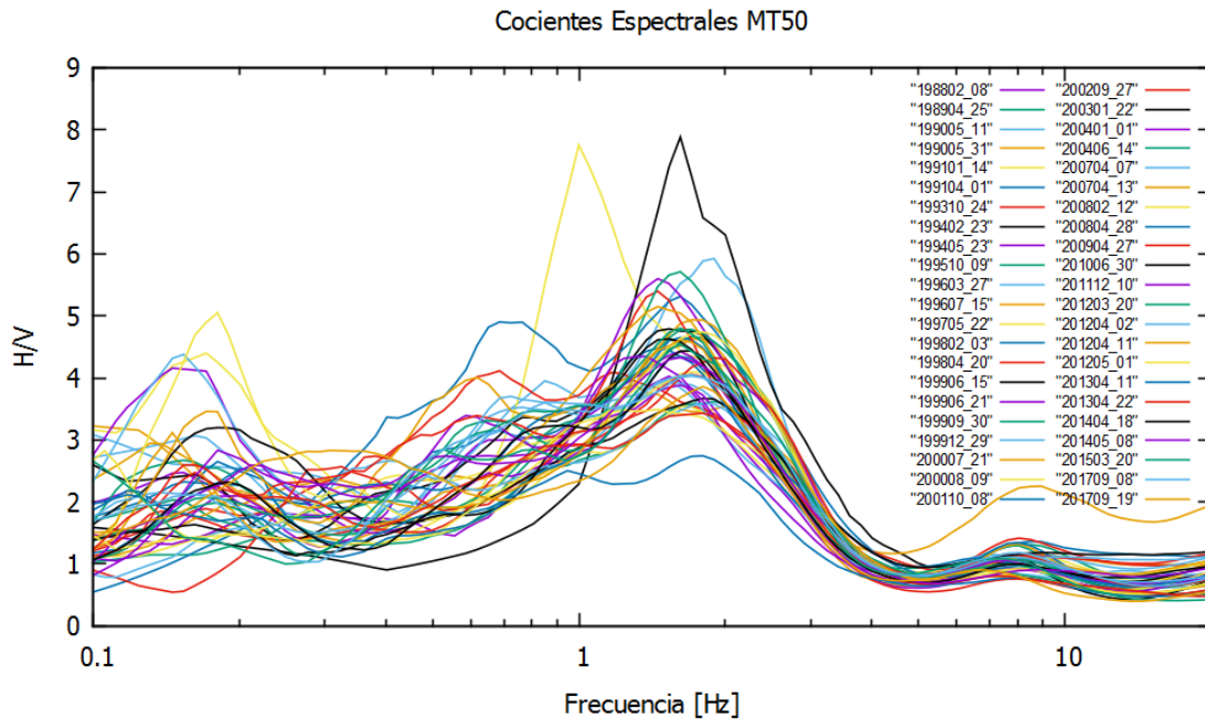
Figura 3.7. Cocientes espectrales de los sismos registrados en la estación MT50 de 1988 a 2017, considerando la parte intensa de la señal.
