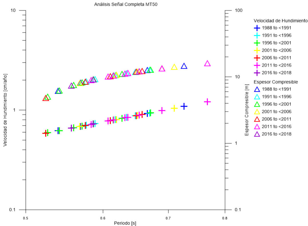
Figura 3.12. Correlación entre el periodo de vibración del suelo, velocidad de hundimiento y espesor de la capa compresible, considerando la señal completa de los sismos registrados en la estación MT50.
