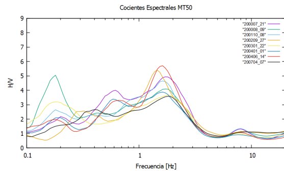
Figura D.4. Cocientes espectrales de los acelerogramas de la estación MT50 de 2000 a 2005.
