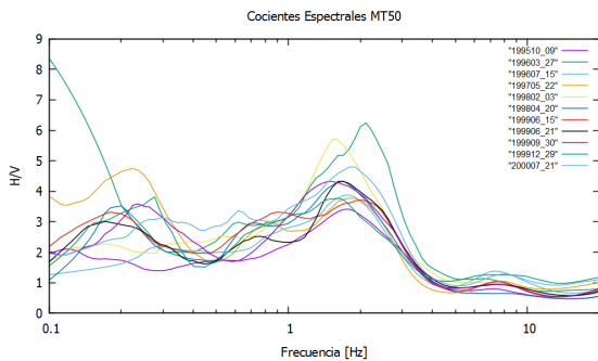
Figura E.3. Cocientes espectrales de los acelerogramas de la estación MT50 de 1995 a 2000.
