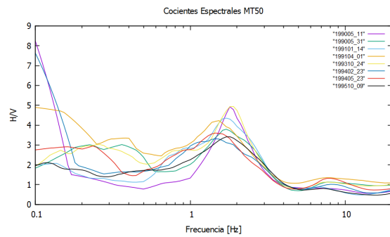
Figura E.2. Cocientes espectrales de los acelerogramas de la estación MT50 de 1990 a 1995.
