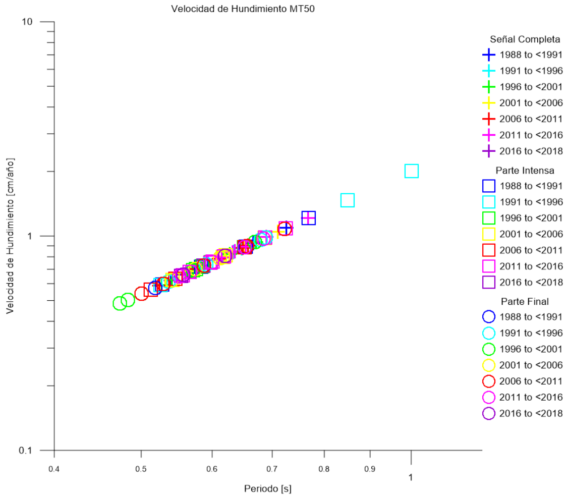
Figura F.1. Velocidad de Hundimiento en la estación MT50, considerando el procesamiento de la señal completa, parte intensa y final de los acelerogramas registrados
