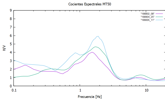
Figura D.1. Cocientes espectrales de los acelerogramas de la estación MT50 de 1988 a 1990.
