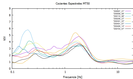
Figura E.4. Cocientes espectrales de los acelerogramas de la estación MT50 de 2000 a 2005.
