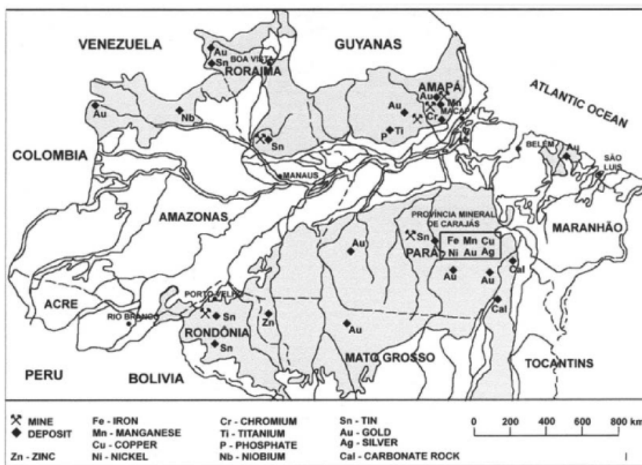
Figura 4 – Pré-cambriano na Amazônia: principais depósitos minerais
