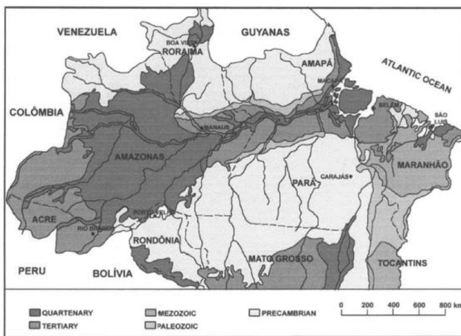
Figura 3 – Amazônia: mapa geológico simplificado
