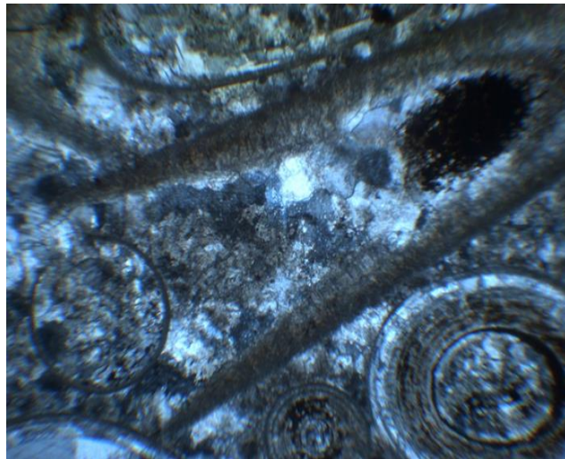
Figura 16. Microfotografía (X7) Ejemplar USONDG-147. Superficie pulida que muestra la sección transversal de dos ejemplares de Salterella conulata , Clark, 1924. El interior de las cámaras está parcialmente reemplazado por sílice y presenta algunas disoluciones. La muestra corresponde con un packstone de bioclastos.
