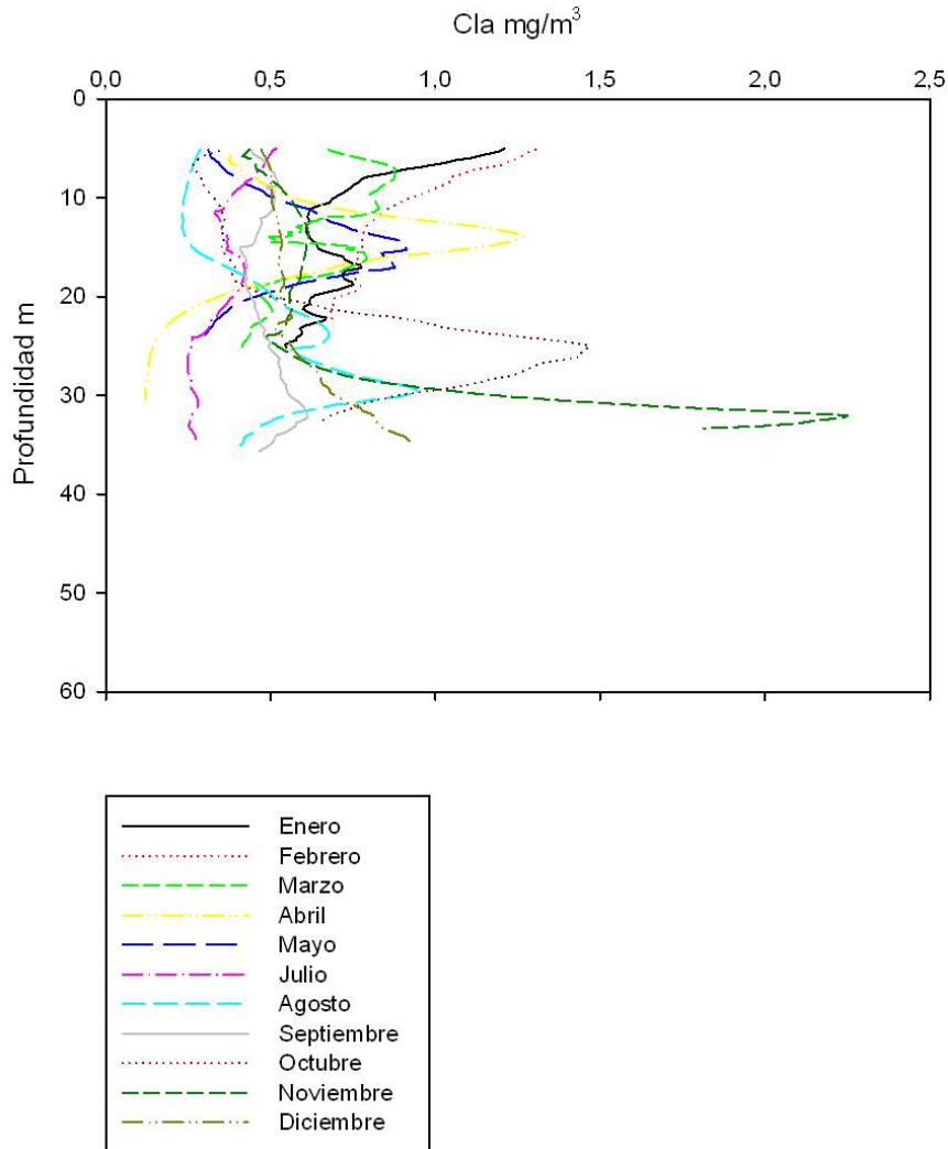
Imagen 7. Perfiles de la concentración de clorofila a (Clor-a) en el lago Alchichica durante el año 2007
