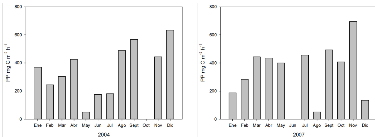
Imagen 12. Producción primaria (PP) integrada por unidad de área para 2004 (a) y para 2007
