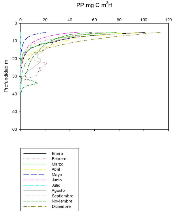
Imagen 9. Perfiles verticales de productividad primaria (PP) en el lago Alchichica durante el año 2004.
