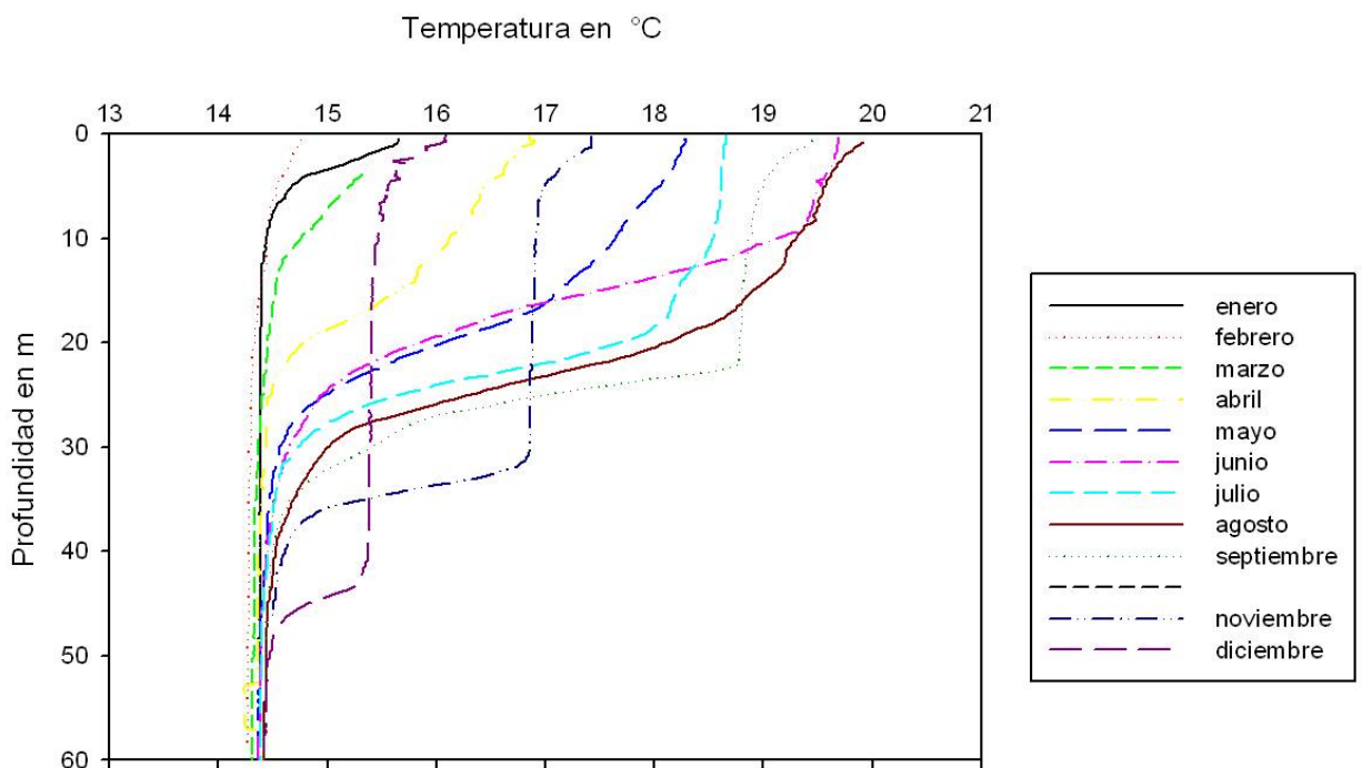
Imagen 3. Perfiles de temperatura en el Lago de Alchichica a lo largo del 2004
