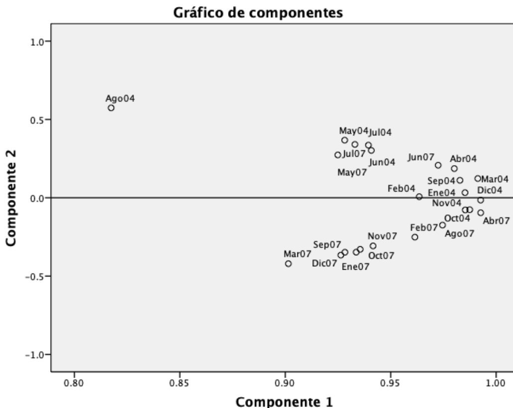
Imagen 11. Gráfico del análisis de componente principales con base en las variables ambientales, concentración de Clor-a y PP
