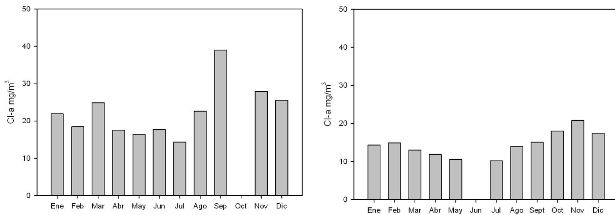
Imagen 8. Concentración de clorofila a (Clor-a) integrada por unidad de área en el lago Alchichica durante el año 2007.
