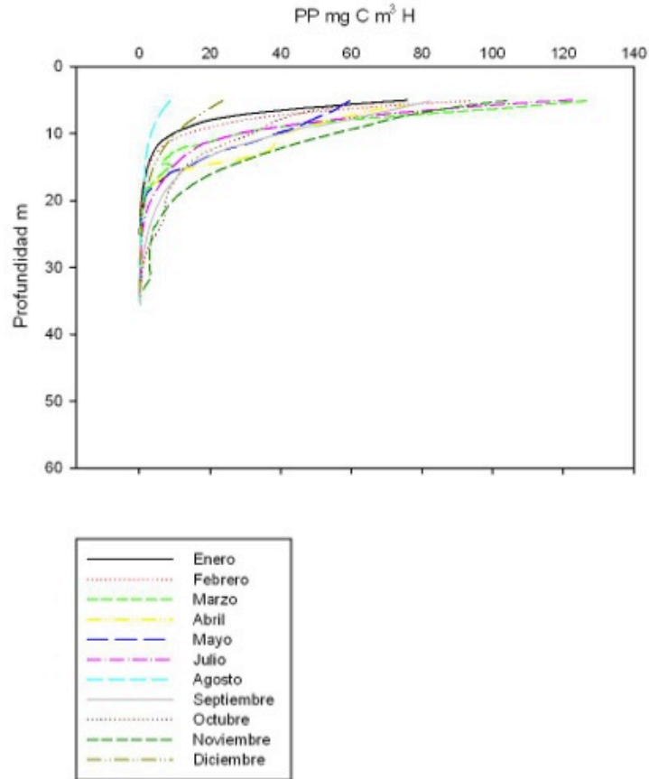
Imagen 10. Perfiles verticales de productividad primaria (PP) en el lago Alchichica durante el año 2007.
