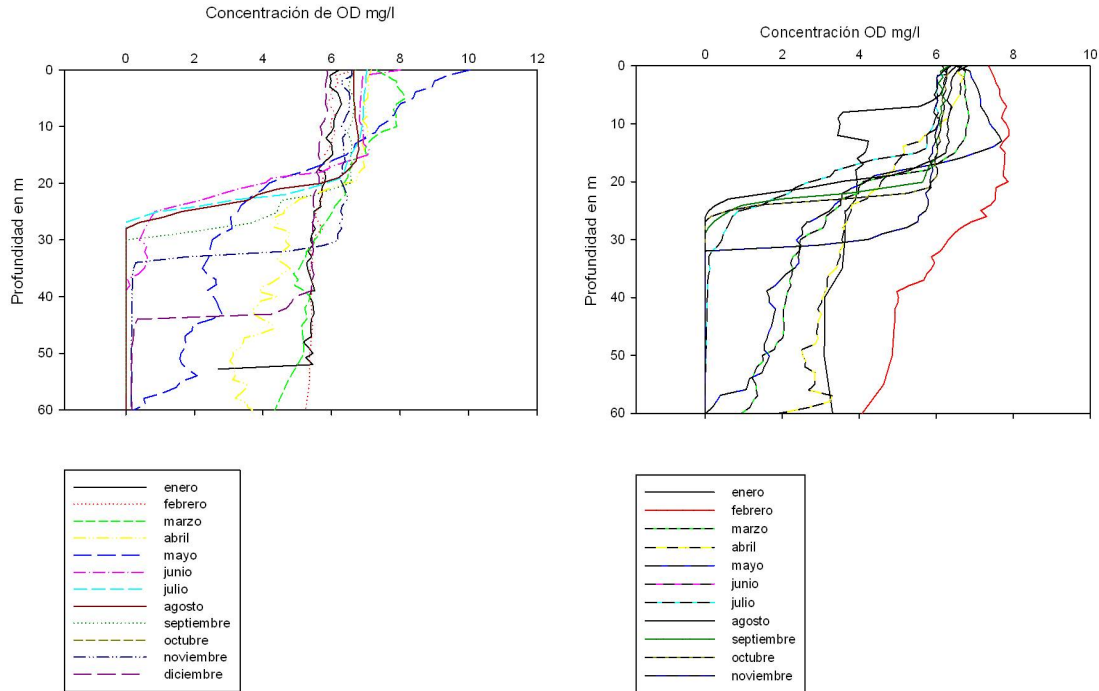
Imagen 5. Perfiles de la concentración de oxígeno disuelto (OD) en el lago Alchichica: a) 2004 y b) 2007
