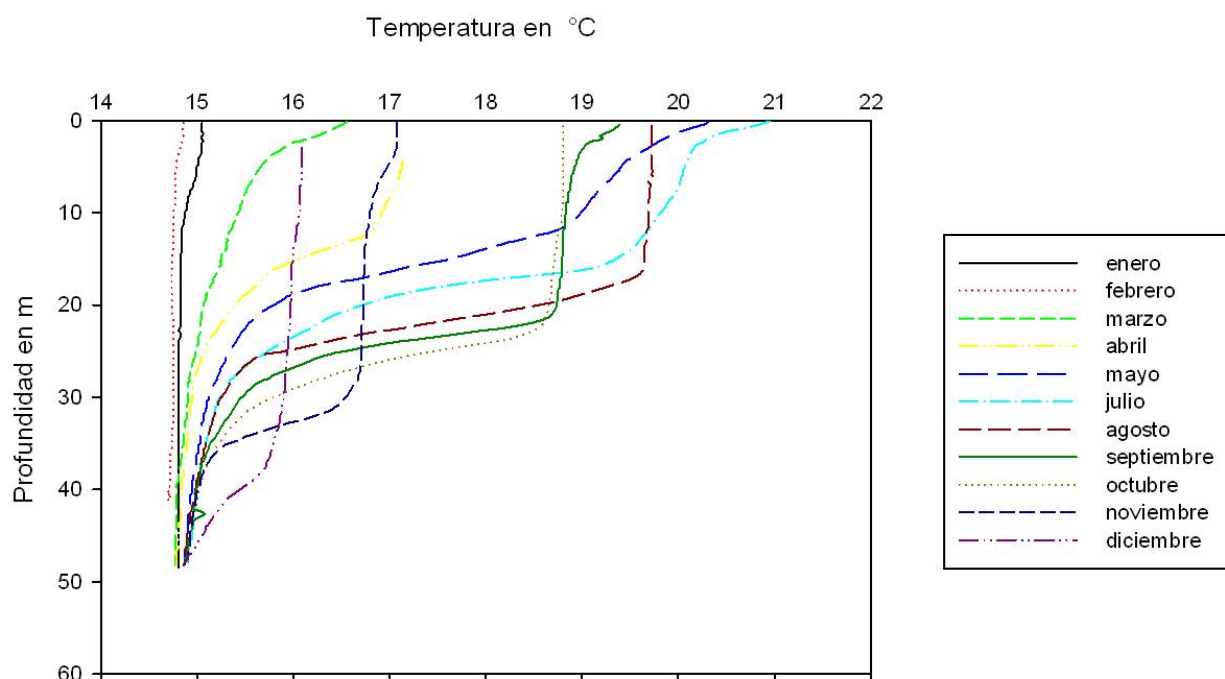
Imagen 4. Perfiles de temperatura en el Lago de Alchichica a lo largo de 2007.
