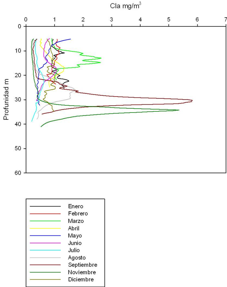
Imagen 6. Perfiles de la concentración de clorofila a (Clor-a) en el lago Alchichica durante el 2004
