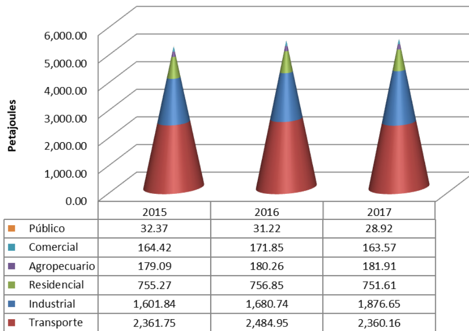
Gráfica 1.2 Consumo energético total en Petajoules. Elaboración propia.
