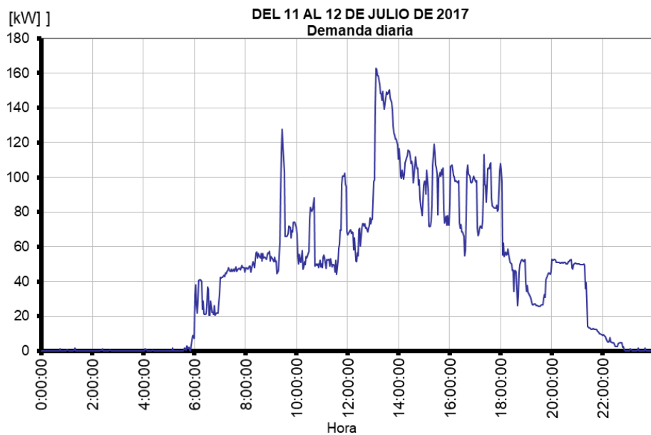
Gráfica 1.10 Demanda diaria en la empresa
