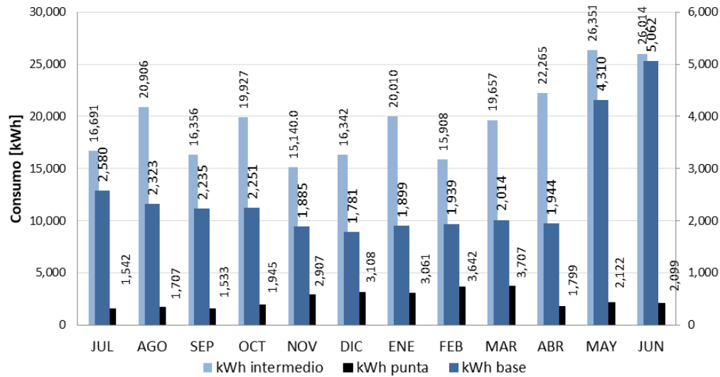
Gráfica 1.6 Consumo mensual 2016-2017
