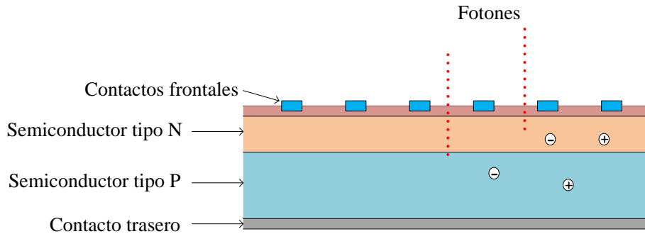
Figura 3.1 Esquema de una celda solar de silicio
