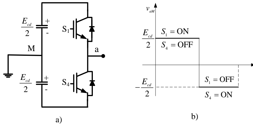
Figura 3.7 a) Representación esquemática del convertidor VSC de medio puente b) Voltaje de salida de CA
