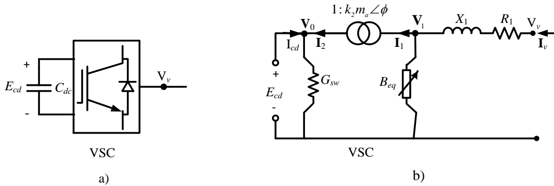
Figura 3.10 a) Representación esquemática del VSC b) Circuito equivalente en estado estable del VSC
