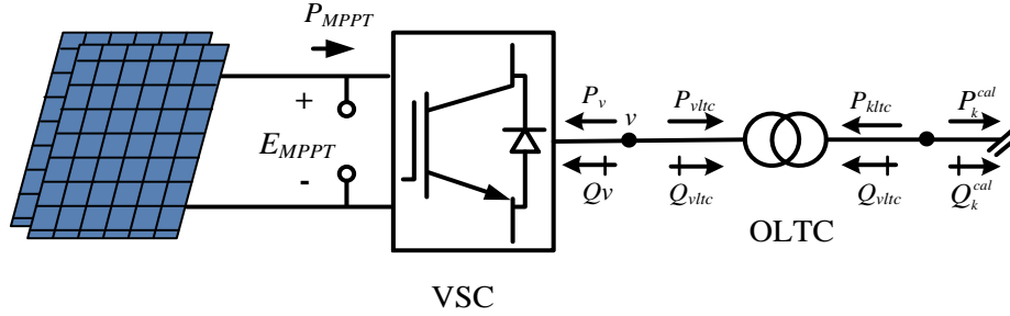
Figura 3.12 Diagrama esquemático del SFV para estado estacionario
