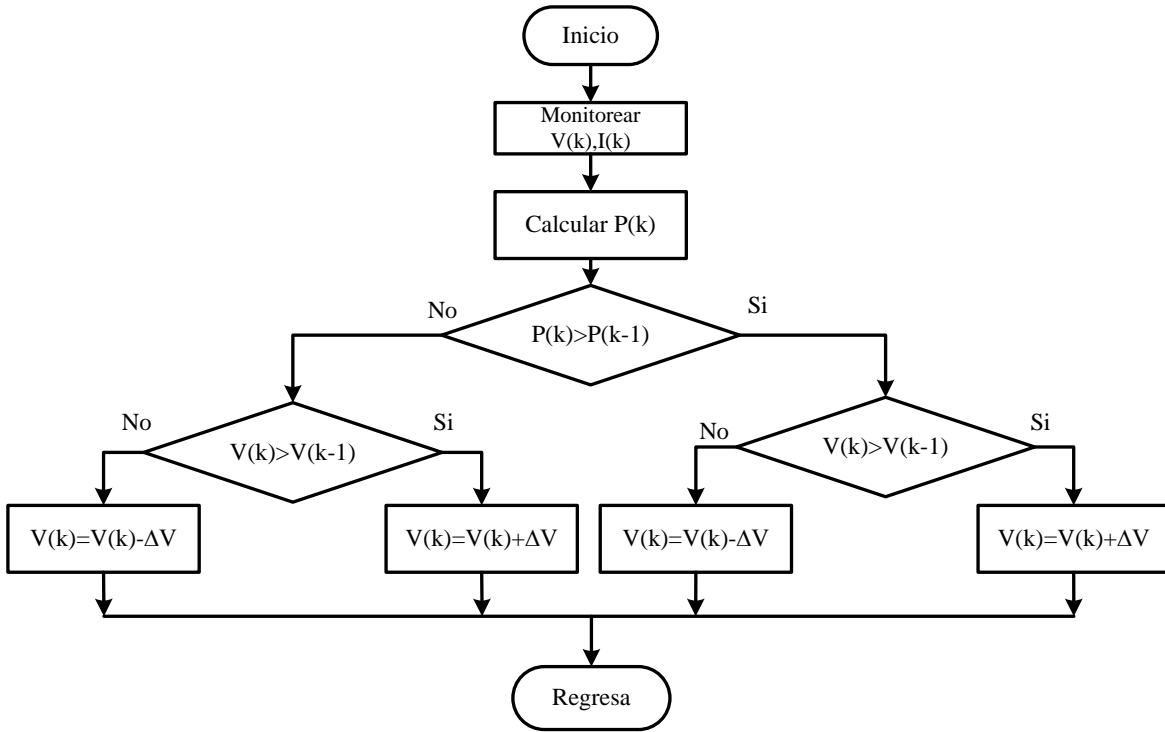
Figura 3.6 Diagrama de flujo del algoritmo P&O.
