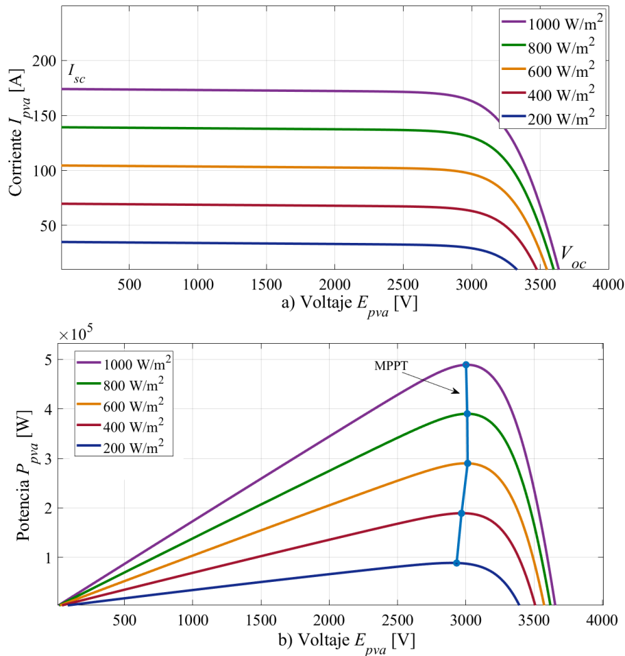
Figura 3.4 Gráficas características de un arreglo fotovoltaico a 25°C; a) Voltaje contra corriente b) Voltaje contra potencia
