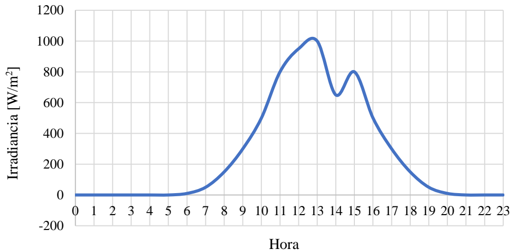
Figura 4.4 Curva de irradiancia típica en un día considerando nubosidad
