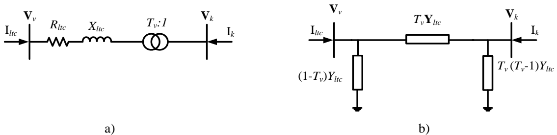
Figura 3.11 Representación del transformador OLTC para flujos de potencia a) Derivación en posición nominal b) Derivación fuera de posición nominal
