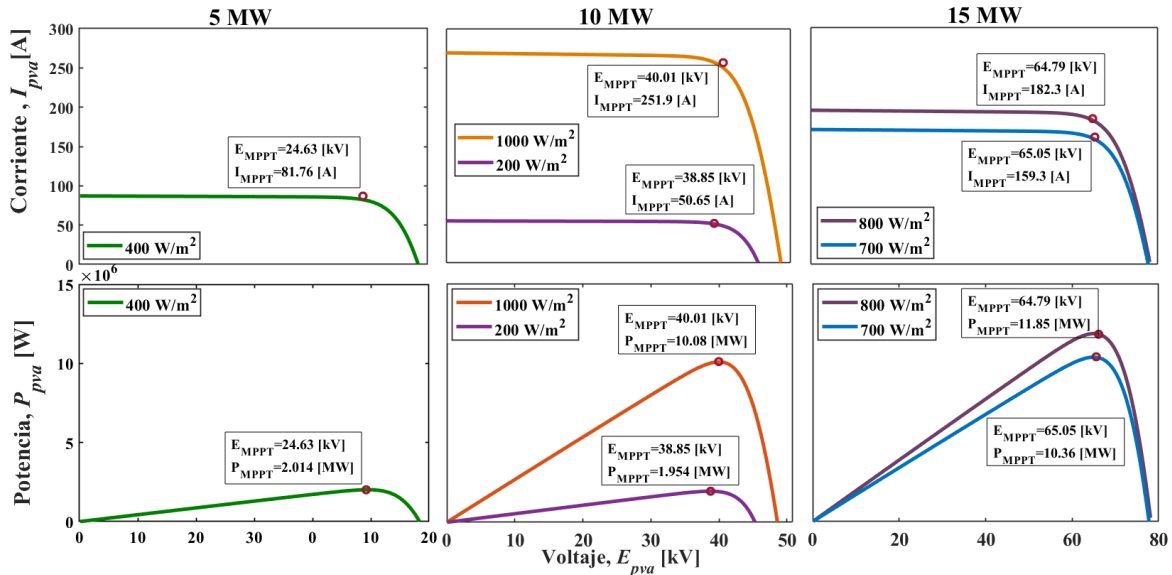
Figura 4.7 Curvas características obtenidas de Simulink, módulos FV del NREL
