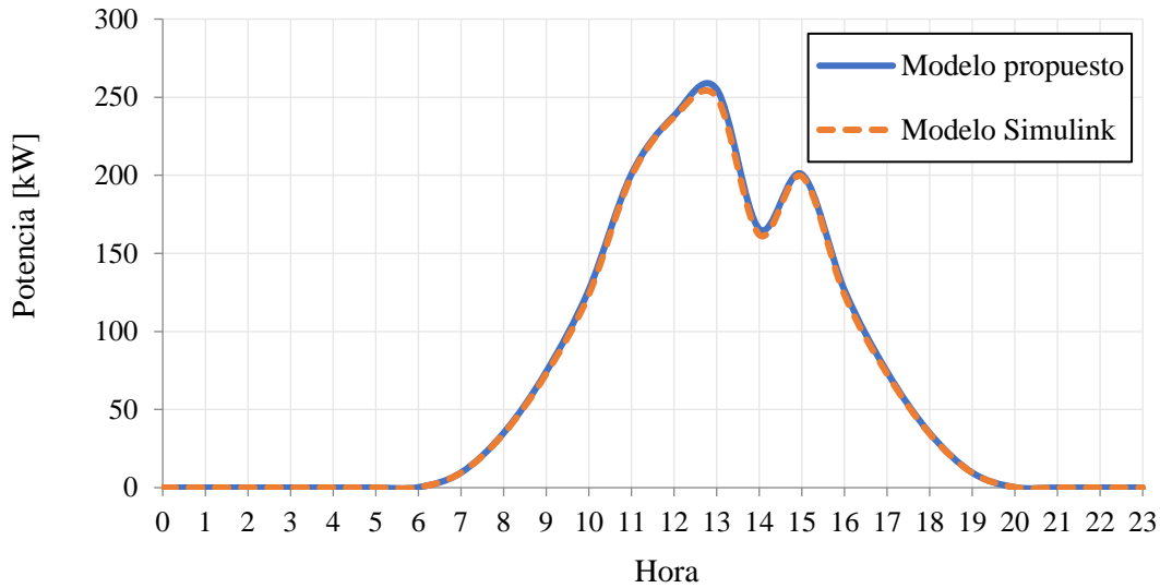
Figura 4.5 Potencias generadas por el SFV cada hora
