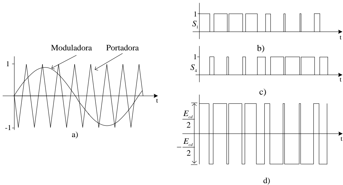
Figura 3.9 Modulación PWM a) Comparación de onda sinusoidal a la frecuencia fundamental con onda triangular de alta frecuencia b) Señal de control de S1 c) Señal de control de S4 d) Señal entre las terminales A y M
