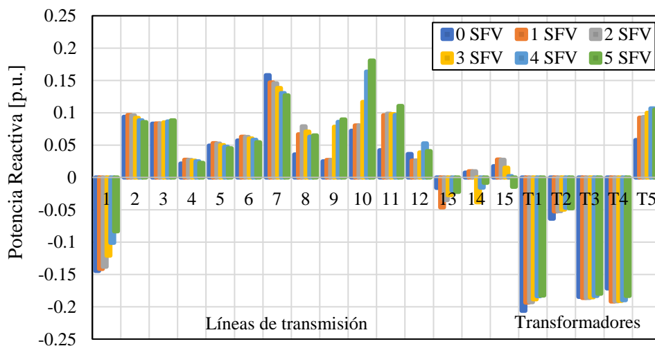
Figura 4.10 Flujos de potencia reactiva en el SEP
