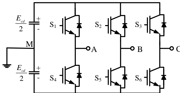
Figura 3.8 Representación esquemática del convertidor VSC trifásico, de 2 niveles
