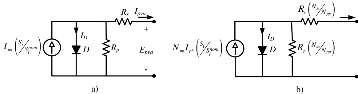
Figura 3.3 a) Circuito equivalente de una celda fotovoltaica b) circuito equivalente de un arreglo fotovoltaico
