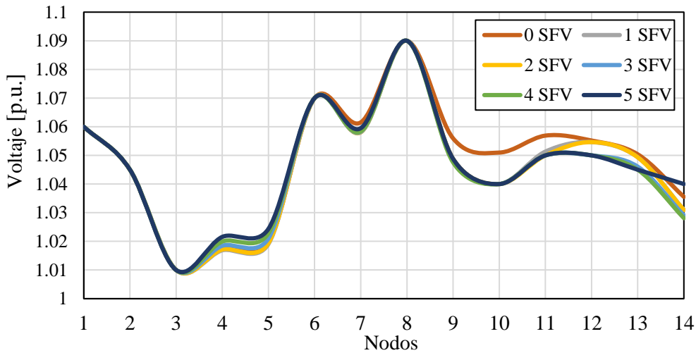
Figura 4.8 Perfil de voltajes nodales en el SEP, considerando de 0 a 5 SFV
