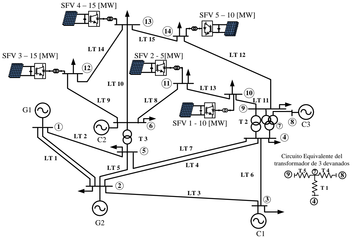
Figura 4.6 Red de prueba de 14 nodos del IEEE con 5 sistemas FV distribuidos
