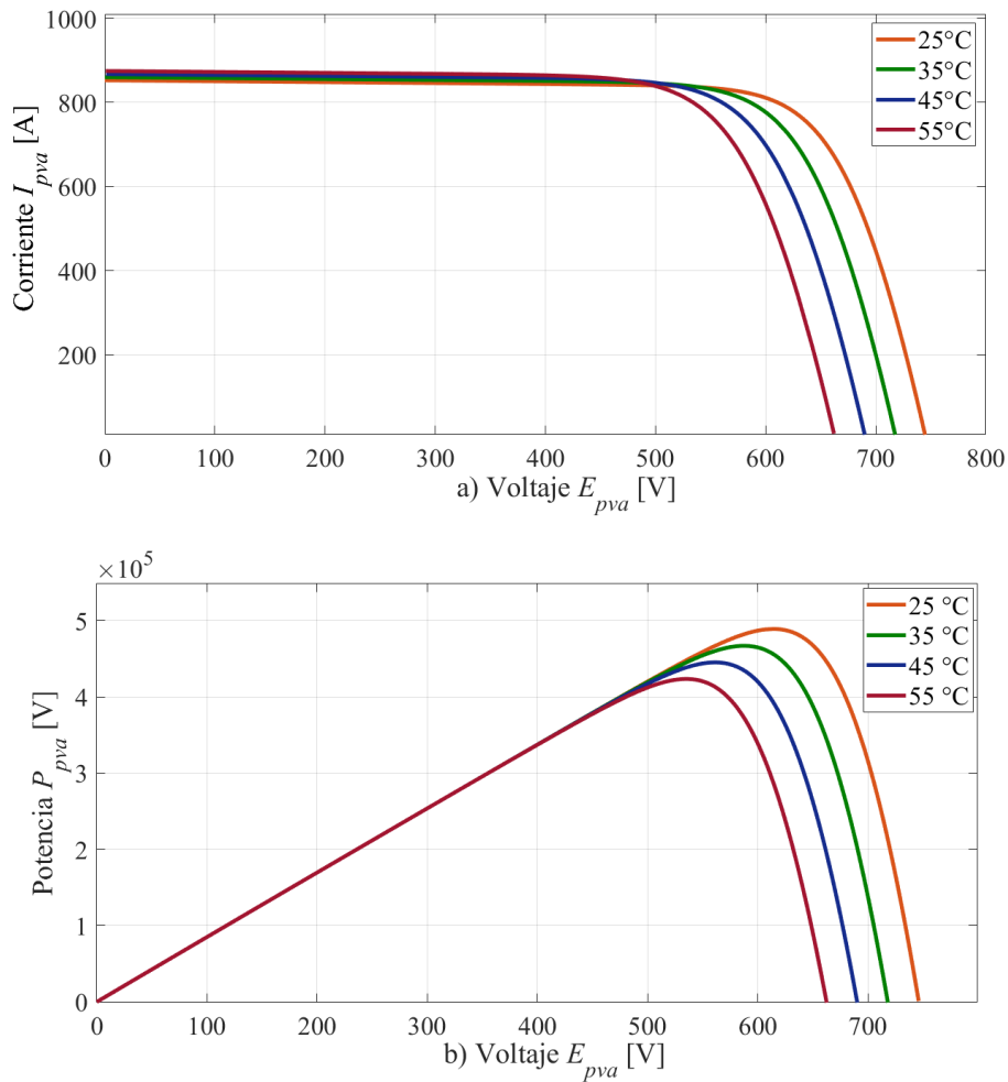
Figura 3.5 Gráficas características de un arreglo fotovoltaico con 1000W/m 2 ; a) Curvas de corriente vs voltaje; b) Curvas de potencia vs voltaje
