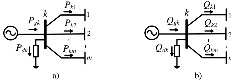
Figura 2.3 Balance de potencia en el nodo k con carga y generación; a) Potencia activa b) Potencia reactiva
