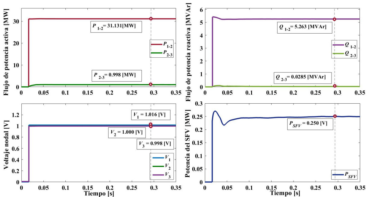
Figura 4.2 Resultados de la simulación dinámica con Simulink
