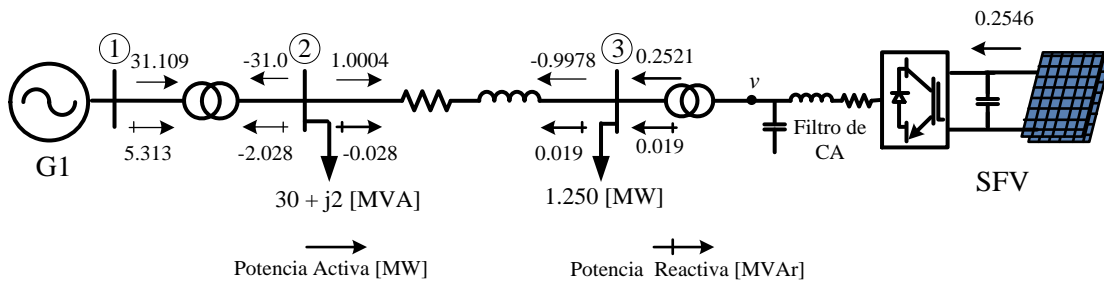
Figura 4.3 Solución final de flujos de potencia
