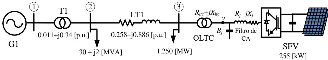
Figura 4.1 Sistema empleado para validar el modelo del SFV
