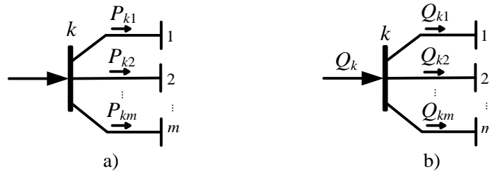
Figura 2.2 Potencias en el nodo k a) Potencia activa b) Potencia reactiva
