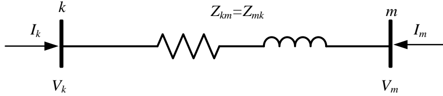
Figura 2.1 Red de dos nodos
