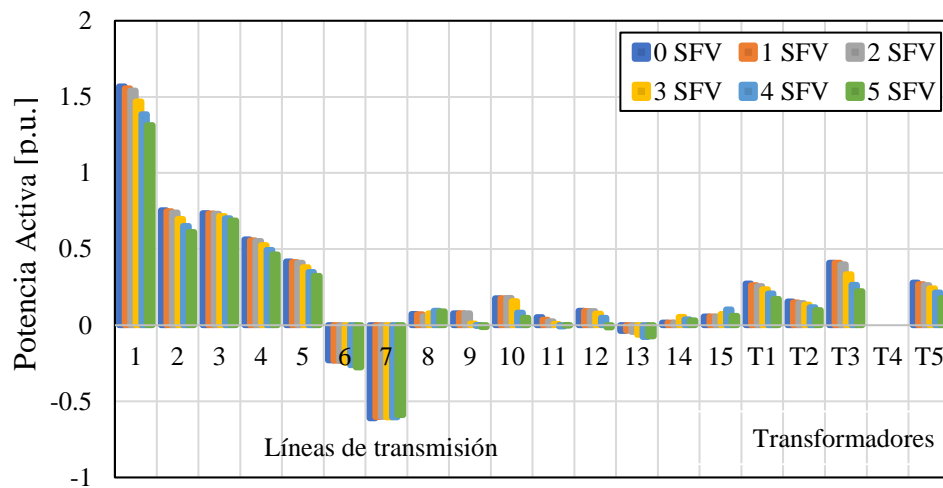
Figura 4.9 Flujos de potencia activa en el SEP
