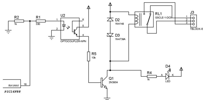
Figura 3-15 Circuito de protección para el PIC16F88.
