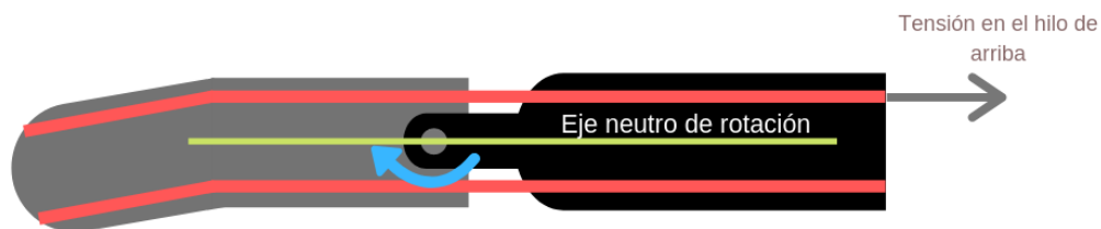
Figura 3.12. Muestra como al jalar el hilo de arriba, se genera un momento flector que la falange distal gire hacia arriba, permitiendo que la mano se abra.
