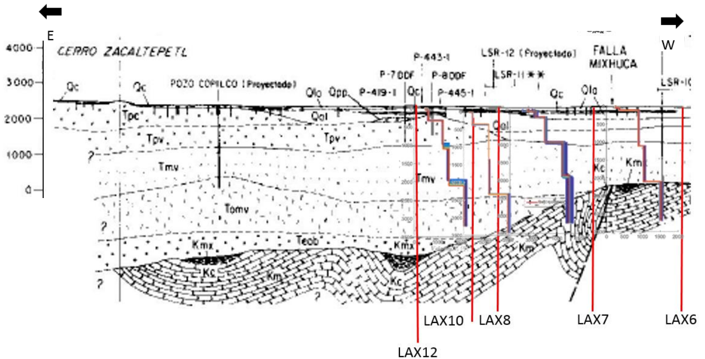
Figura 28 Sección geológica C de la Ciudad de México con las proyecciones de línea de sensores con el perfil de velocidad de onda de corte. El perfil fue tomado y modificado de Vázquez-Sánchez & Jaimes-Palomera (1989).
