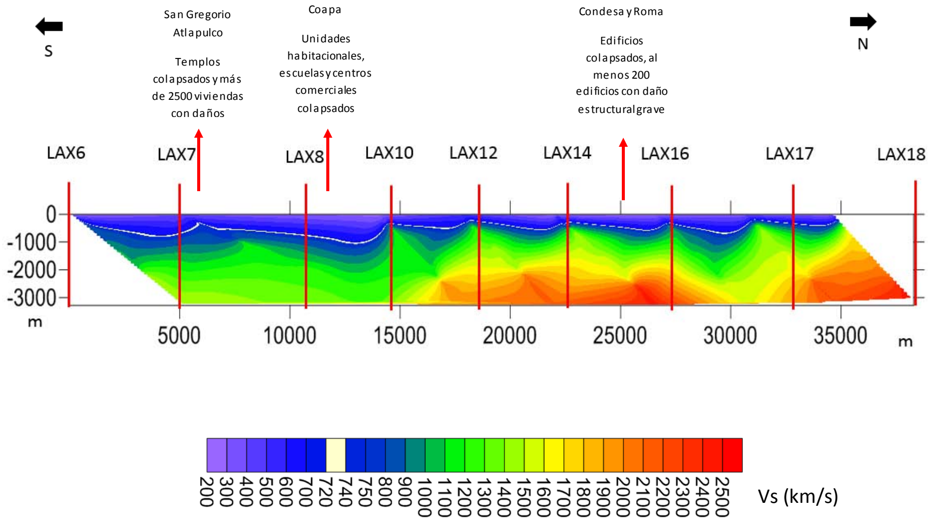
Figura 29 Modelo interpolado de la cuenca del Valle de México. Las barras de color rojo indican la ubicación de los sensores. La línea blanca representa el basamento ingenieril.
