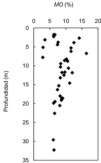
Figura 4.3. Perfil de contenido de materia orgánica del suelo del ex Lago de Texcoco.
