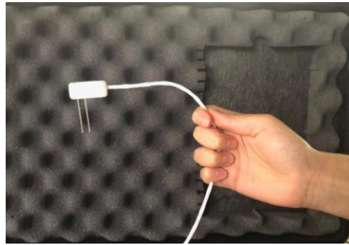
Figura 3.11. Sensor de aguja doble SH-1.
