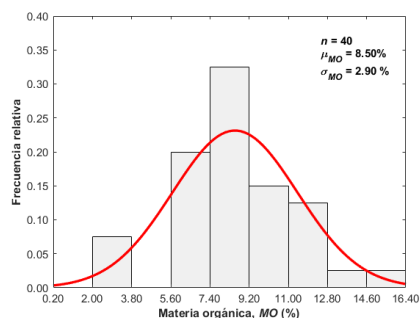
Figura 4.4. Histograma y curva de distribución normal del contenido de materia orgánica del suelo del ex Lago de Texcoco.
