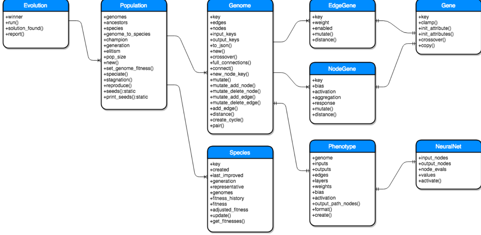
Fig 5A. Diagrama de relación de entidades con propiedades y métodos de cada clase
