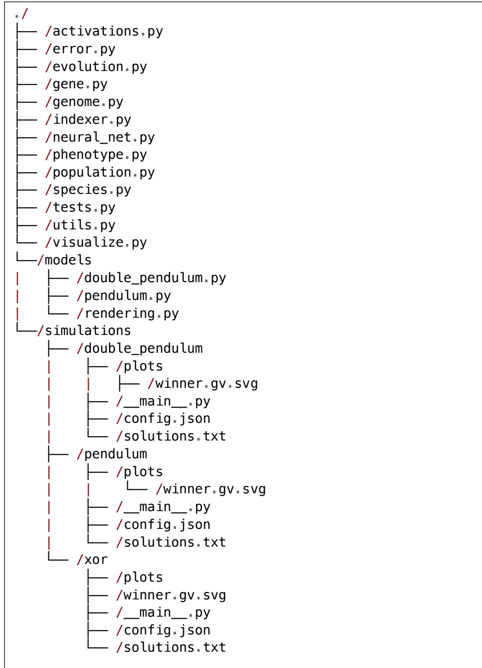
Fig 5B. Árbol de módulos y archivos del sistema.
