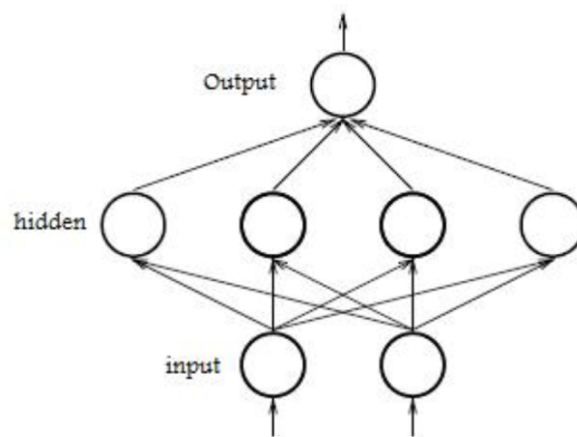
Fig 2E. Ejemplo de una red neuronal simple con 2 entradas, 1 salida y 1 capa oculta.
