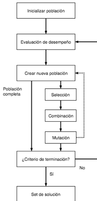
Fig 2B. Diagrama de flujo de un algoritmo genético básico.
