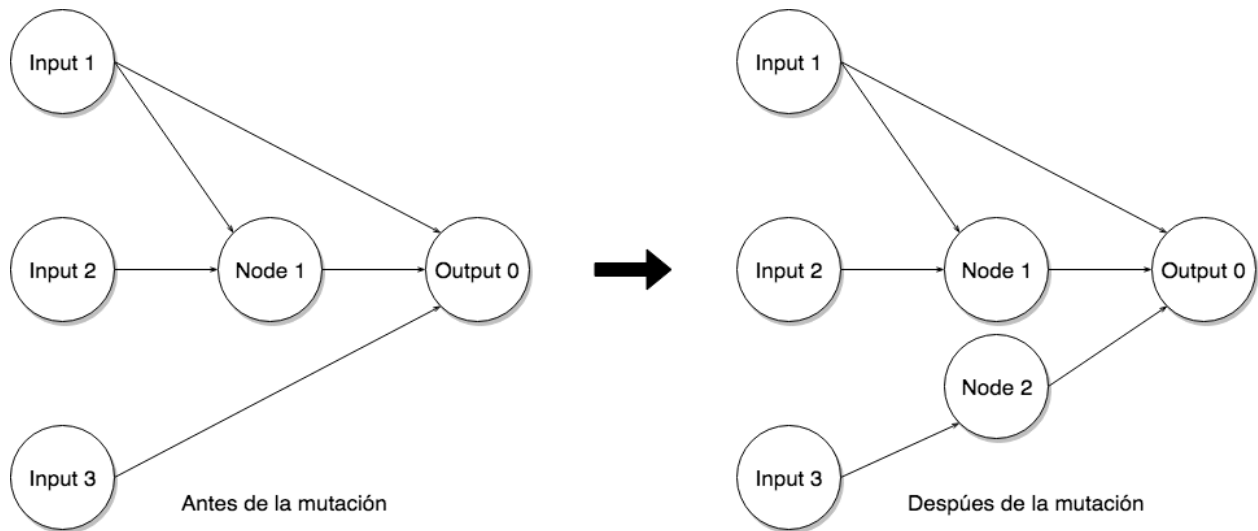
Fig 3E. Ejemplo de mutación estructural de genoma
