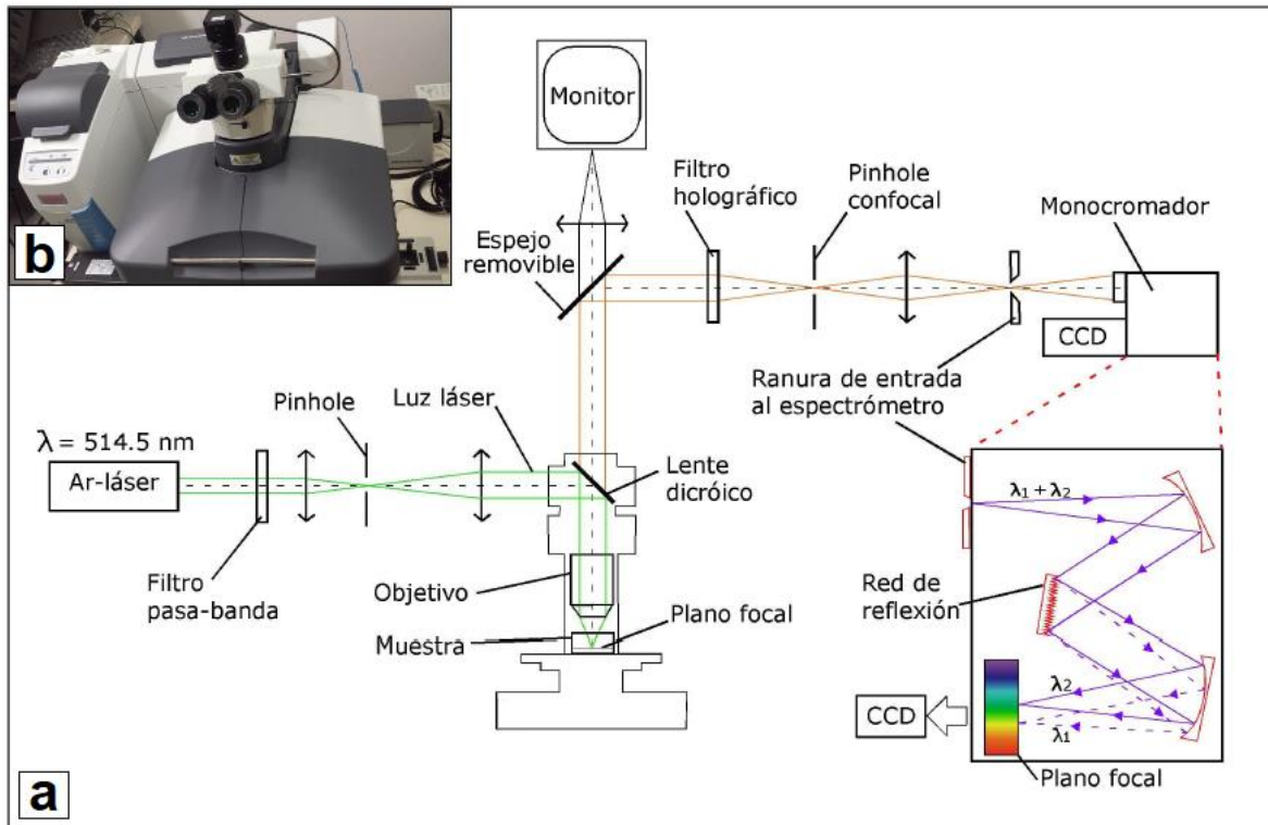
Fig. 3.10. a) Esquema del enfoque del láser en la muestra y la recolección de la dispersión Raman en un detector. b) Microscopio Raman confocal de alto rendimiento ( Thermo Scientific™ DXR™ 2 ).
