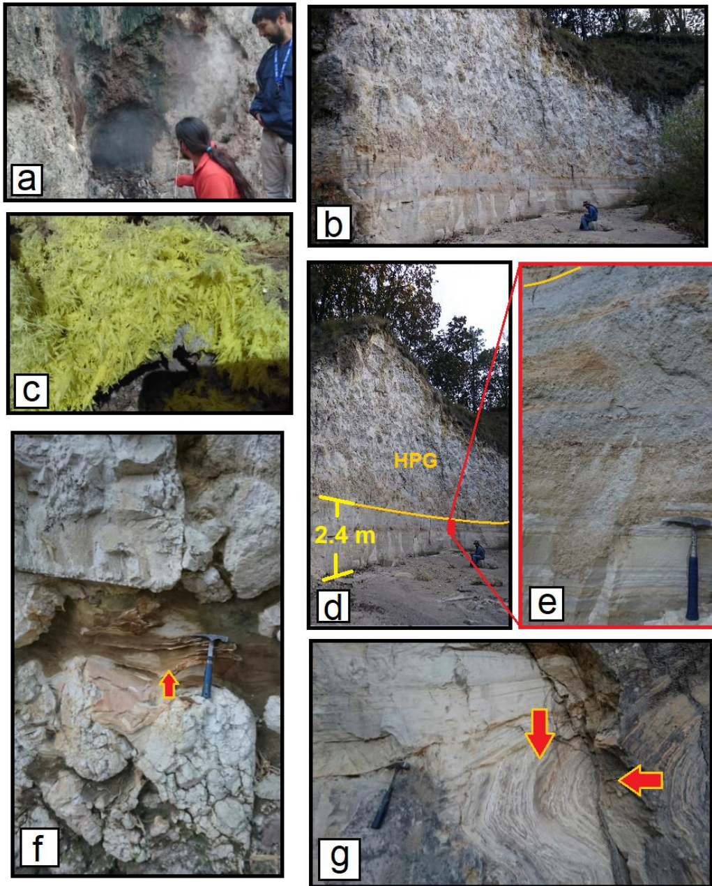
Fig. 4.8. a) Fumarola emergente de la Toba Tala. b) Afloramiento VM-04 donde se observa el límite inferior del HPG, c) Cristales de azufre en fumarolas. d y e) Vista panorámica del corte (VM-04) con el espesor de paquetes que hay por debajo del HPG. f) Depósitos lacustres y cenizas deformadas y siguiendo el contorno de los clastos de pómez gigantes. g) Depósitos lacustres deformados por debajo del HPG. HPG: Horizonte de Pómez Gigante.
