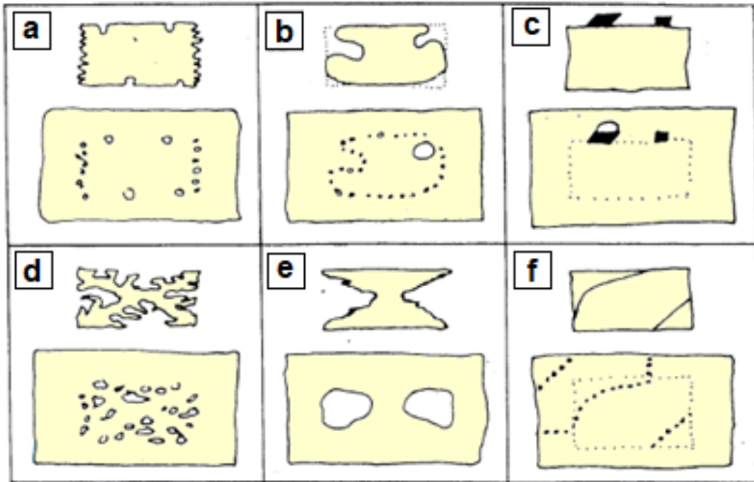
Fig. 3.4. Los seis mecanismos más comunes para el atrapamiento de inclusiones de fundido silicatado. a) Crecimiento repentino. b) Disolución parcial. c) Por inclusiones sólidas. d) Crecimiento dendrítico o esquelético. e) Crecimiento rápido en un hábito tabular. f) Por fracturamiento (Roedder, 1979)
