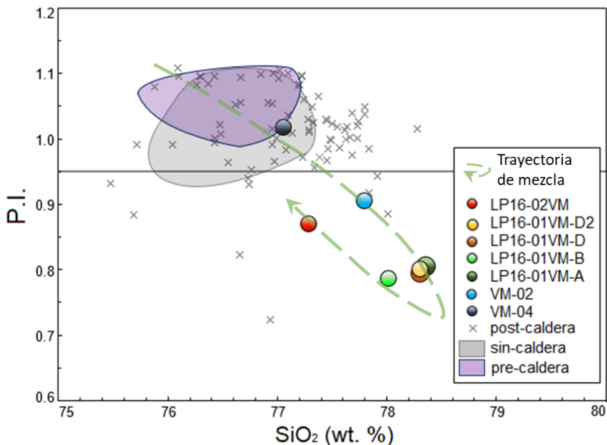
Fig. 5.2. Diagramas para pómez de índice de peralcalinidad P.I. ( [(NaO_2+K_2O)/Al_2O_3] molar) vs. Sílice, con la trayectoria de evolución composicional (flecha verde). La muestras que se grafican por arriba de la línea son peralcalinas (tomada desde 0.95 por los posibles errores analíticos). Los datos se comparan con la geoquímica publicada de La Primavera.
