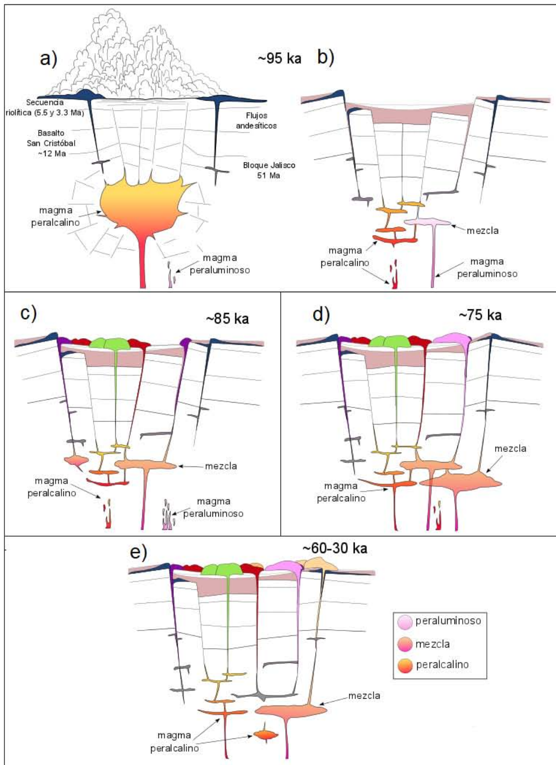
Fig. 5.6. Modelo esquemático del sistema de bombeo de La Primavera, no está a escala. A) La erupción de Toba Tala. B) Condiciones pre-eruptivas del HPG, domos centrales y domos anulares antiguos. C) Condiciones pre-eruptivas domos anulares jóvenes. D) Levantamiento topográfico hacia el sur. E) Formación Arco de lavas Sur y domo El Colli.
