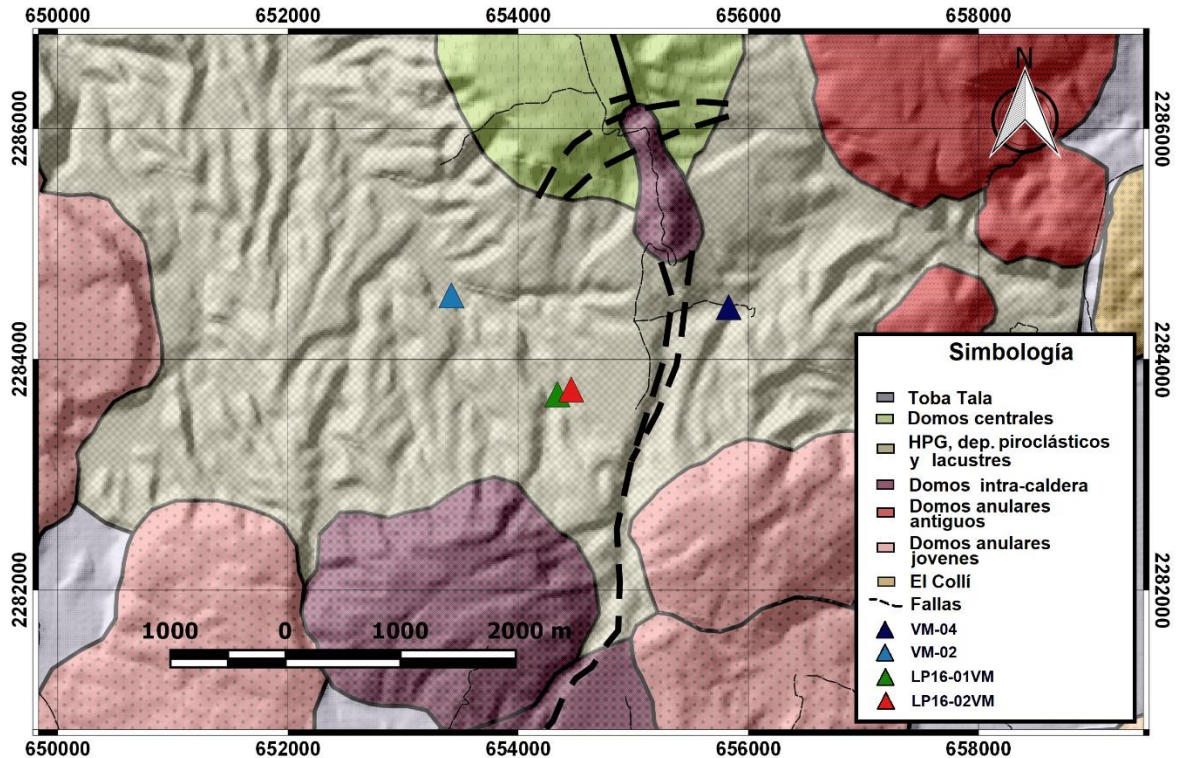
Fig. 4.7. Mapa geológico de la caldera de La Primavera. Se muestra la localización de los afloramientos donde se tomaron las muestras (Triángulos de colores). En las localidades VM-04 y VM-02 se observó el HPG. Por otra parte LP16-01VM y LP16-02VM están estratigráficamente por encima del HPG, siendo LP16-02VM la cima de la columna estratigráfica descrita en este estudio.
