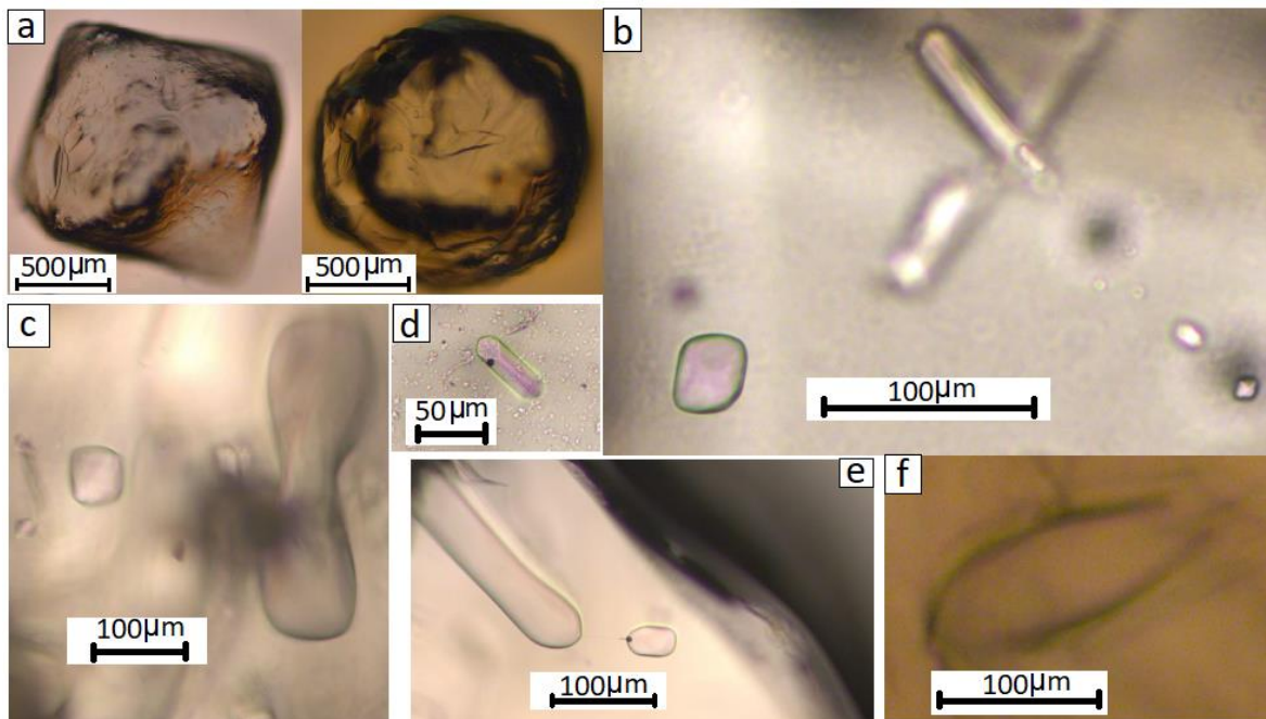
Fig. 4.20. Fotomicrografías tomadas con microscopio petrográfico de los cristales e inclusiones de fundido (IFu) del horizonte de caídas de pómez (LP16-02VM). a) Cristales huésped de cuarzo. b) Grupo de IFu en cuarzo "J1", se pueden ver distintas formas de inclusiones en un mismo cristal. c) IFu monofásica de diferentes formas y tamaños, alojadas en "J2". d) IFu bifásica en "J2". e) Una gran IFu alargada y monofásica con una más pequeña y bifásica, alojadas en "K5". f) IFu ovalada a irregular en "J3".
