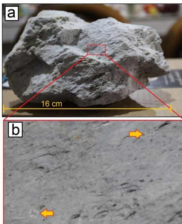
Fig. 4.17. a) Bloque de pómez del HPG en el afloramiento VM-02, se puede apreciar vesicularidad alineada y un color gris claro. b) Detalle de la fotografía donde las flechas señalan dos finos cristales.
