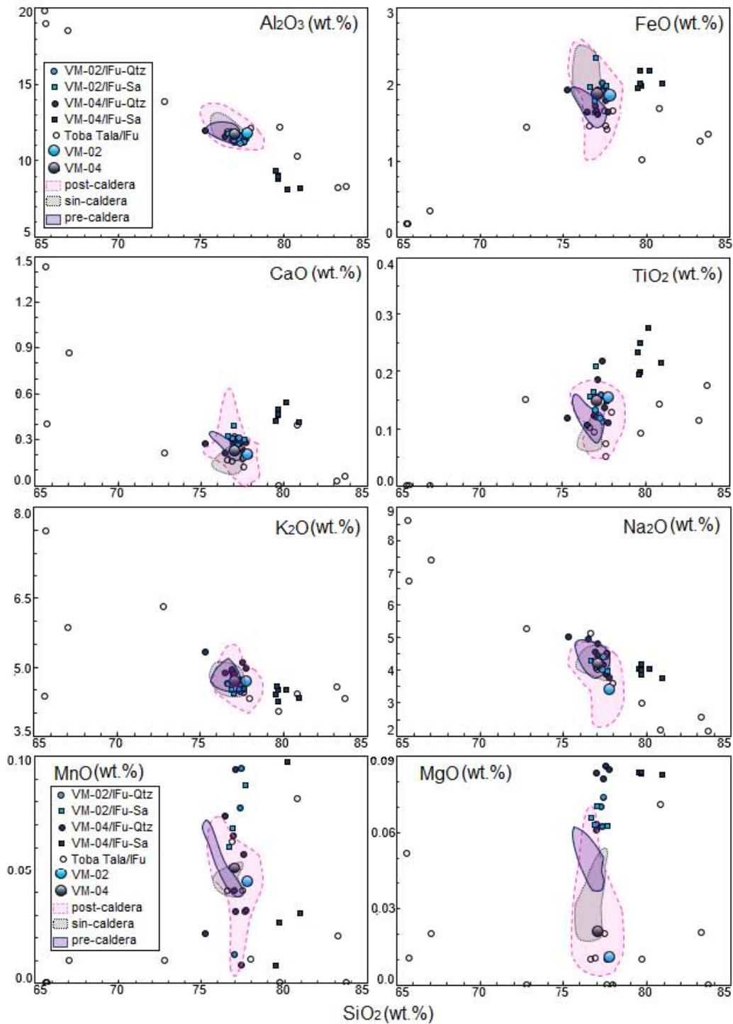
Fig. 4.33. Diagramas Harker para VM-04 y VM-02 (Pómez gigante). Se comparan las inclusiones de fundido (círculos y cuadrados pequeños con relleno) y pómez (círculos grandes con relleno) analizadas en esta tesis, con la geoquímica publicada de La Primavera (áreas de color)(Mahood 1977, 1981a y 1981b; Cruz-Lara, 2015; Gómez-Álvarez, 2015; Miguel-Cruz, 2016; Tinoco-Murrillo, 2017; Ávila-Ortiz, 2018; Sourisseau, en proceso), y con la geoquímica de las IFu de Toba Tala (círculos pequeños sin relleno) (Miguel-Cruz, 2016).
