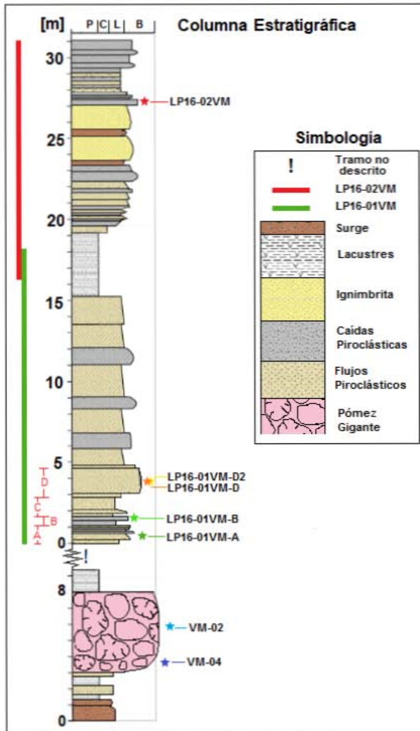
Fig. 4.12. Columna estratigráfica simplificada, y ubicación de las muestras colectadas en La Primavera. Las estrellas muestran la posición estratigráfica de las muestras colectadas en campo. Las líneas verde y roja del lado izquierdo limitan las dos secciones descritas. Las letras: A, B, C y D representan los límites de los paquetes en los que se dividió la primera sección (LP16-01VM). En la base se muestra la última etapa de Toba Tala (sin-caldera).
