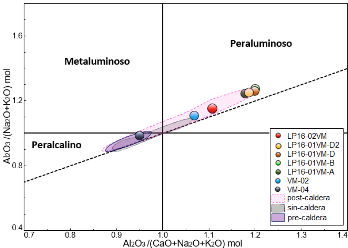
Fig. 4.22. Diagrama Al_2O_3/(Na_2O+K_2O+CaO) vs. Al_2O_3/(Na_2O+K_2O) (Shand, 1943). Los círculos de colores corresponden a las muestras de pómez colectadas para este trabajo.
