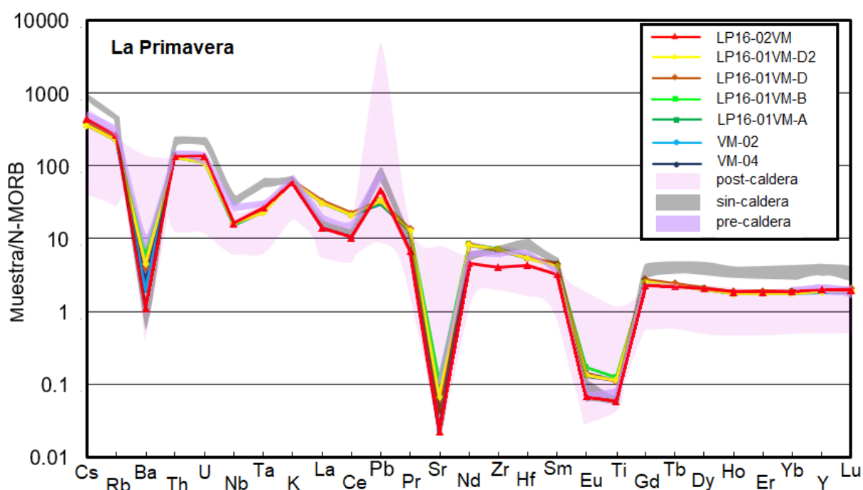
Fig. 4.27. Diagrama spider, normalizado con respecto a NMORB (Sun & McDonough, 1989). Las líneas de colores representan la composición de las muestras de pómez analizadas en esta tesis. Áreas de colores: datos de Mahood (1977, 1981a y 1981b); Cruz-Lara (2015); Gómez-Álvarez (2015); Miguel-Cruz (2016); Tinoco-Murrillo (2017); Ávila-Ortiz (2018); Sourisseau (en proceso). Se pueden observar anomalías negativas en Ba, Sr, Eu y Ti.
