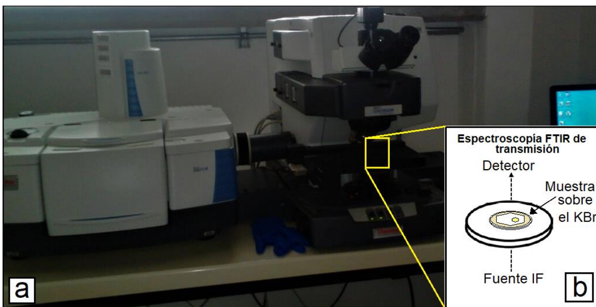
Fig. 4.37. a) Equipo utilizado para el análisis de volátiles en inclusiones de fundido: microscopio y espectrómetro FTIR. b) Esquema de espectroscopía FTIR de transmisión. Modificado de Chen et al. (2015).
