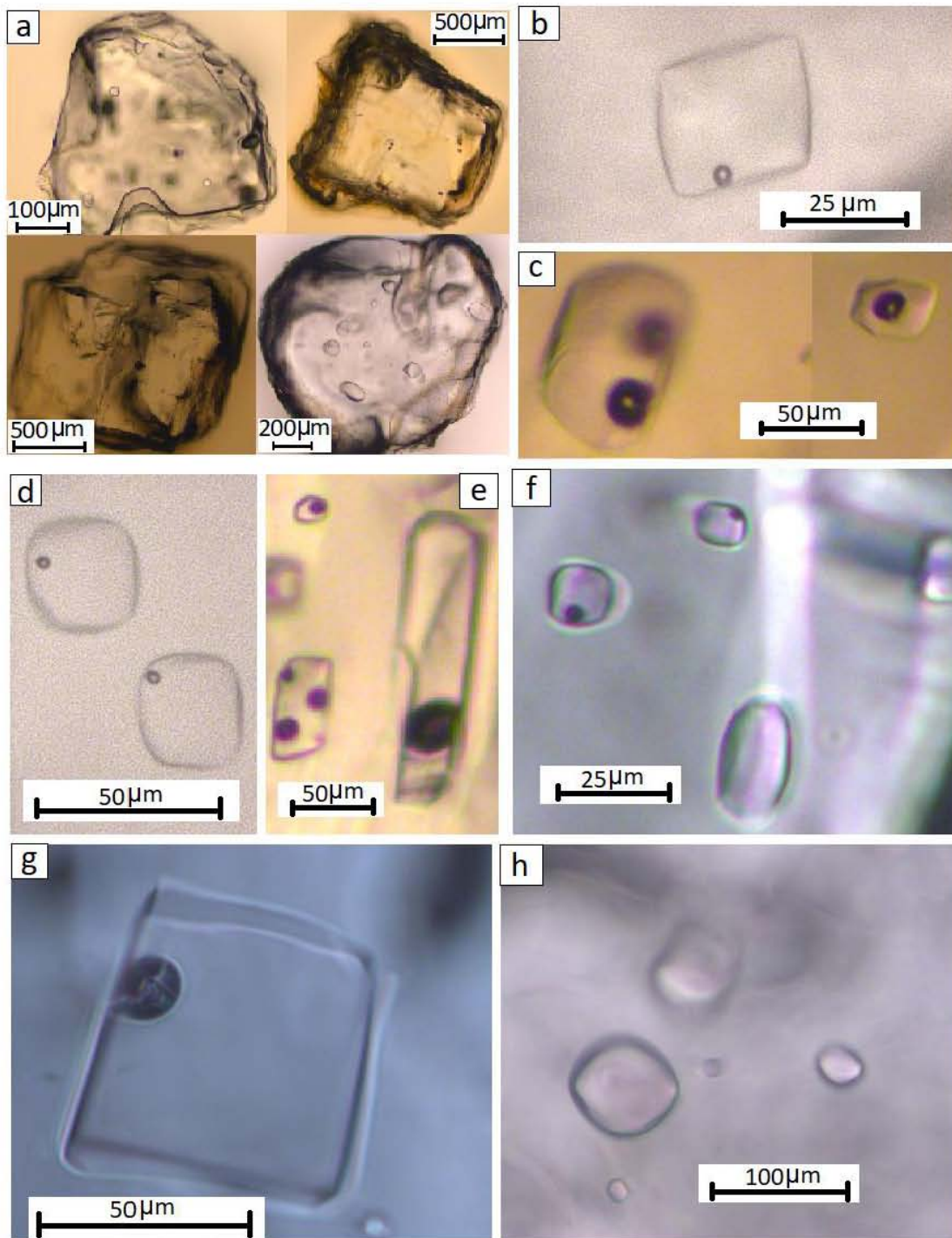
Fig. 4.18. Fotomicrografías de cristales huésped e inclusiones de fundido (IFu) del Horizonte de Pómez Gigante (VM-2 y VM-4). a) Cristales de cuarzo y sanidino. b) Inclusión de fundido con forma de cristal negativo en cuarzo "O1". c) IFu en sanidino "N4" con distintos tamaños, y diferente número de burbujas. d) IFu bifásicas en cuarzo "O2", donde G > V . e) IFu de diferentes formas y tamaños, y número de fases presentes en sanidino "N2". f) Grupo de IFu bifásicas y monofásicas en cuarzo "O2". g) IFu con forma de cristal negativo en sanidino "L3". h) Grupo de IFu monofásicas en cuarzo "M2". Todas las muestras fueron tomadas con luz transmitida y condensador.
