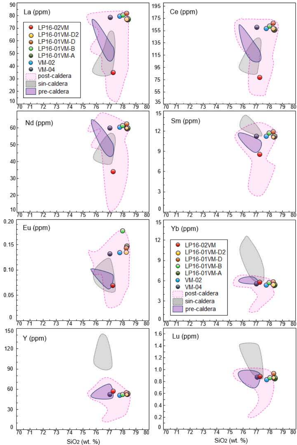
Fig. 4.26. Diagramas de variación de elementos traza vs sílice para LREE (La, Ce, Nd, Sm y Eu) y HREE (Yb, Y y Lu). Los círculos de colores corresponden a las muestras de pómez colectadas para este trabajo, y los datos con los que se construyeron las áreas (pre-caldera, sin-caldera y post-caldera) son de Mahood (1977, 1981a y 1981b), Cruz-Lara (2015), Gómez-Álvarez (2015), Miguel-Cruz (2016), Tinoco-Murrillo (2017), Ávila-Ortiz (2018) y Sourisseau (en proceso).
