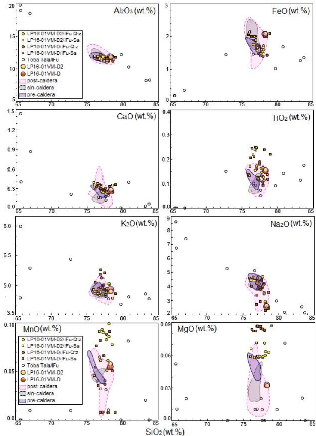
Fig. 4.35. Diagramas Harker para muestras de la sección LP16-01VM, horizontes D y D2. Se comparan las inclusiones de fundido (círculos y cuadrados pequeños con relleno) y pómez (círculos grandes con relleno) analizadas en esta tesis, con la geoquímica publicada de La Primavera (áreas de color)(Mahood 1977, 1981a y 1981b; Cruz-Lara, 2015; Gómez-Álvarez, 2015; Miguel-Cruz, 2016; Tinoco-Murrillo, 2017; Ávila-Ortiz, 2018; Sourisseau, en proceso), y con la geoquímica de las IFu de Toba Tala (círculos pequeños sin relleno) (Miguel-Cruz, 2016).
