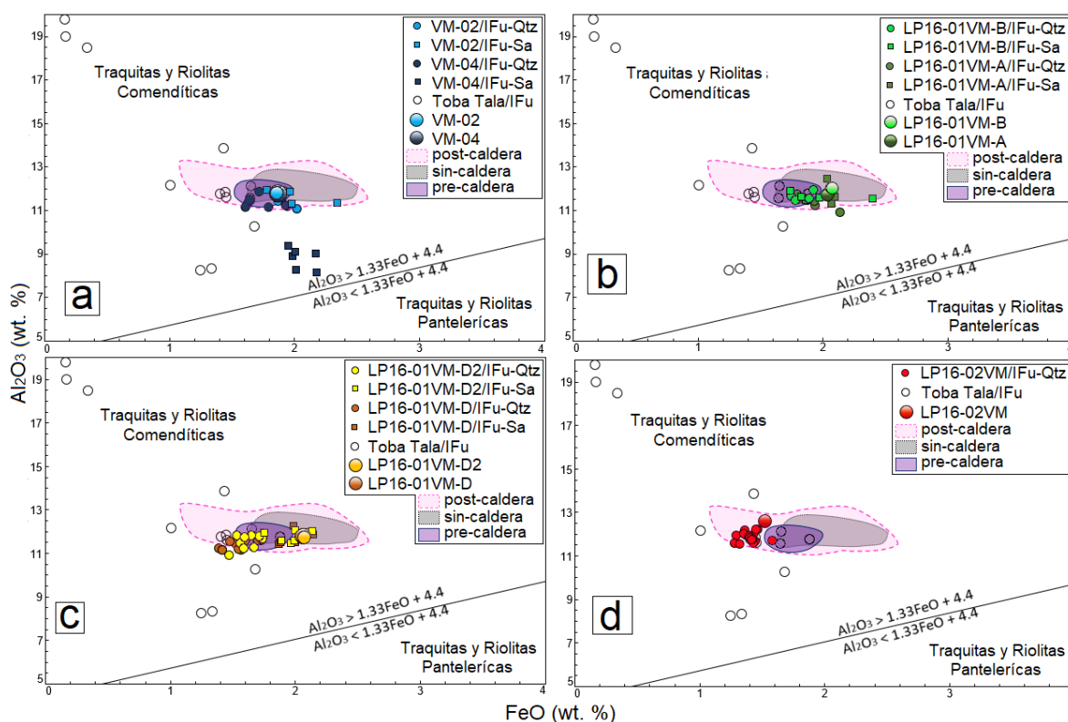
Fig. 4.32. Diagramas para clasificación de traquitas y riolitas en rocas comendíticas y pantelleríticas (Macdonald, 1974). a) Pómez Gigante. b) Sección LP16-01VM (horizontes A y B). c) Sección LP16-01VM (horizontes D y D2). d) Sección LP16-02VM. El hierro total se calculó con la expresión: FeO^* = FeO + Fe_2O_3(0.8998) . Se comparan las inclusiones de fundido (círculos y cuadrados pequeños con relleno) y pómez (círculos grandes con relleno) analizadas en esta tesis, con la geoquímica publicada de La Primavera (áreas de color)(Mahood 1977, 1981a y 1981b; Cruz-Lara, 2015; Gómez-Álvarez, 2015; Miguel-Cruz, 2016; Tinoco-Murrillo, 2017; Ávila-Ortiz, 2018; Sourisseau, en proceso), y con la geoquímica de las IFu de Toba Tala (círculos pequeños sin relleno) (Miguel-Cruz, 2016).
