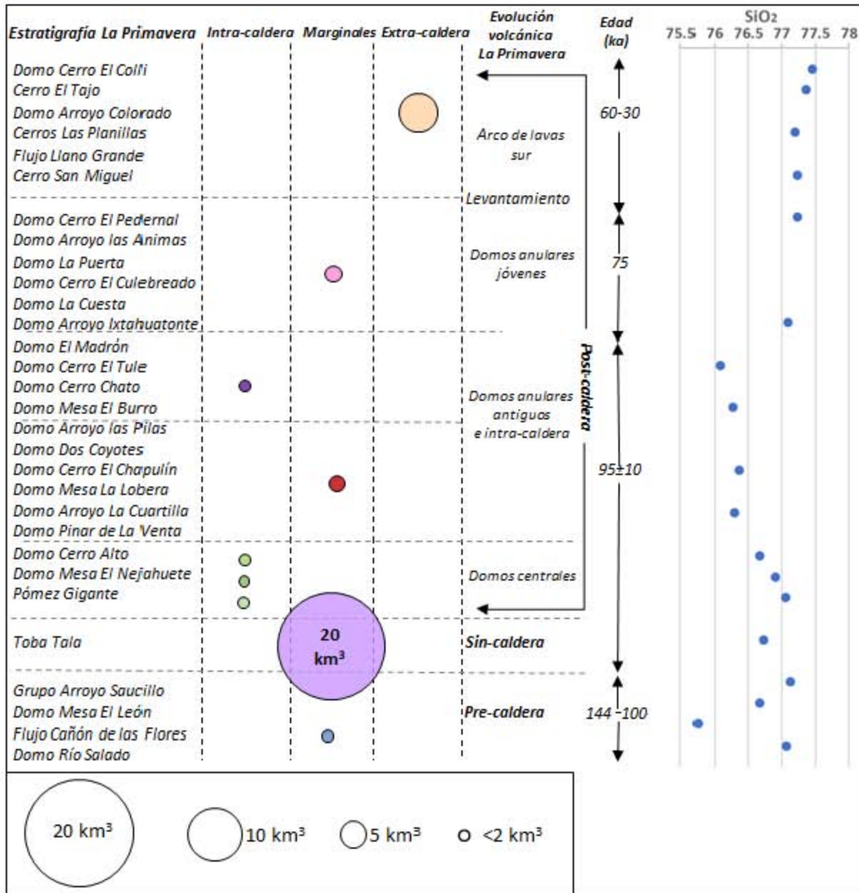
Fig. 4.1. Estratigrafía de La Primavera y la relación con su edad, volumen de magma y contenido en sílice, datos tomados de Mahood (1981).
