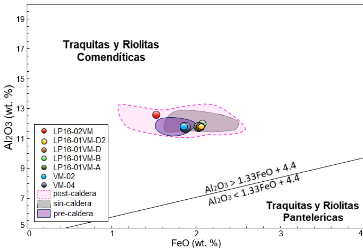
Fig. 4.23. Diagrama para clasificación de traquitas y riolitas en rocas comendíticas y pantelericas (Macdonald, 1974). Los símbolos circulares indican la composición de pómez estudiadas en esta tesis. El óxido de hierro total se calculó con la expresión: FeO^* = FeO + Fe_2O_3(0.8998) .
