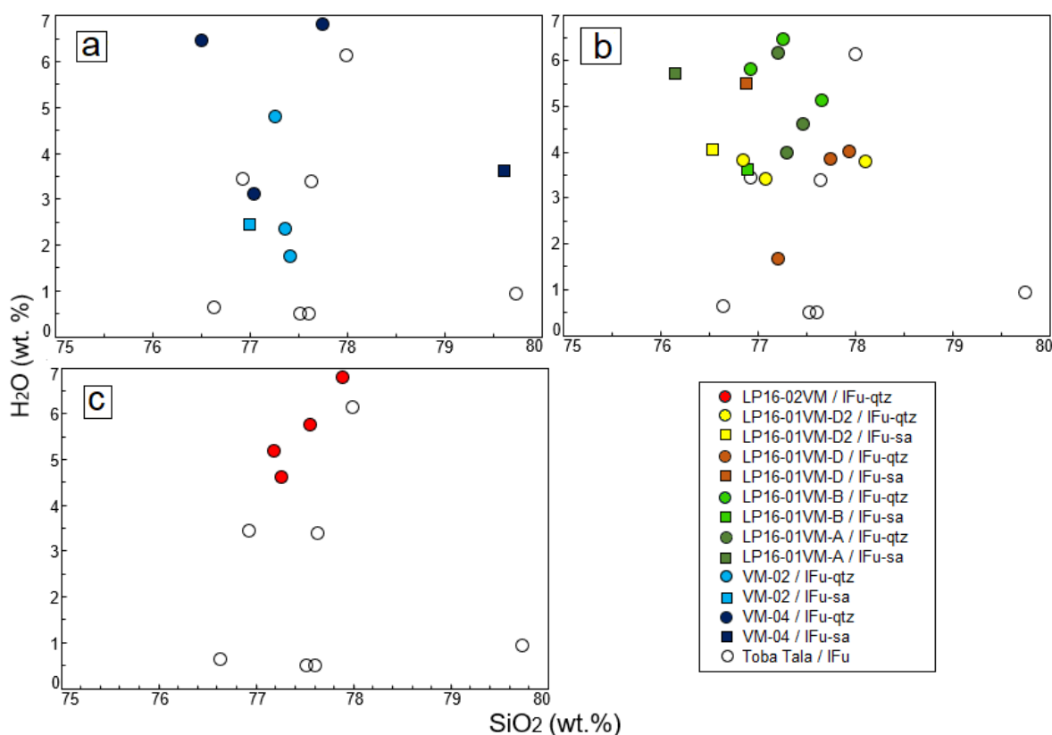
Fig. 4.39. Diagramas binarios de H 2 O vs SiO 2 . a) IFu de la Pómez Gigante. b) IFu de la sección LP16-01VM. c) IFu de la sección LP16-02VM. Círculos sin relleno: IFu en Toba Tala (Miguel-Cruz, 2016).
