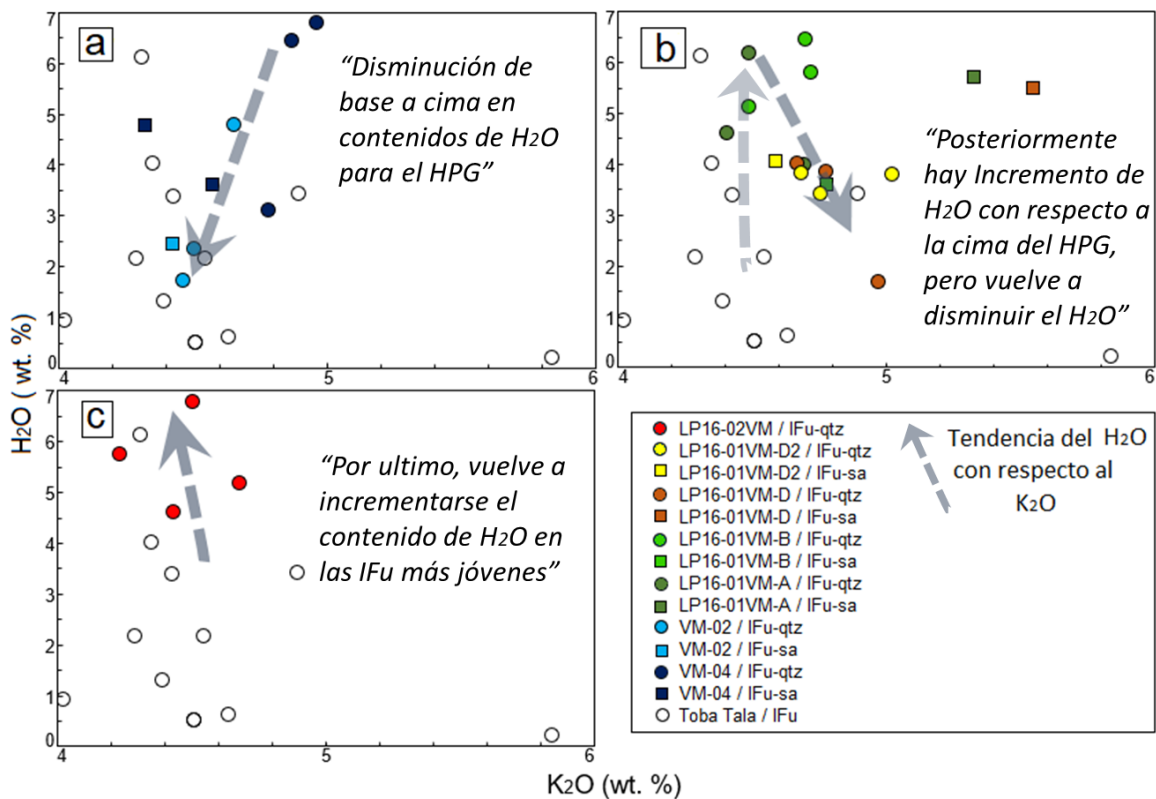
Fig. 5.5. Diagramas binarios de agua vs potasio. a) IFu de la Pómez Gigantes. b) IFu de la sección LP16-01VM. c) IFu de la sección LP16-02VM. Círculos sin relleno: IFu en Toba Tala (Miguel-Cruz, 2016). Se muestra la tendencia evolutiva de los eventos post-caldera.
