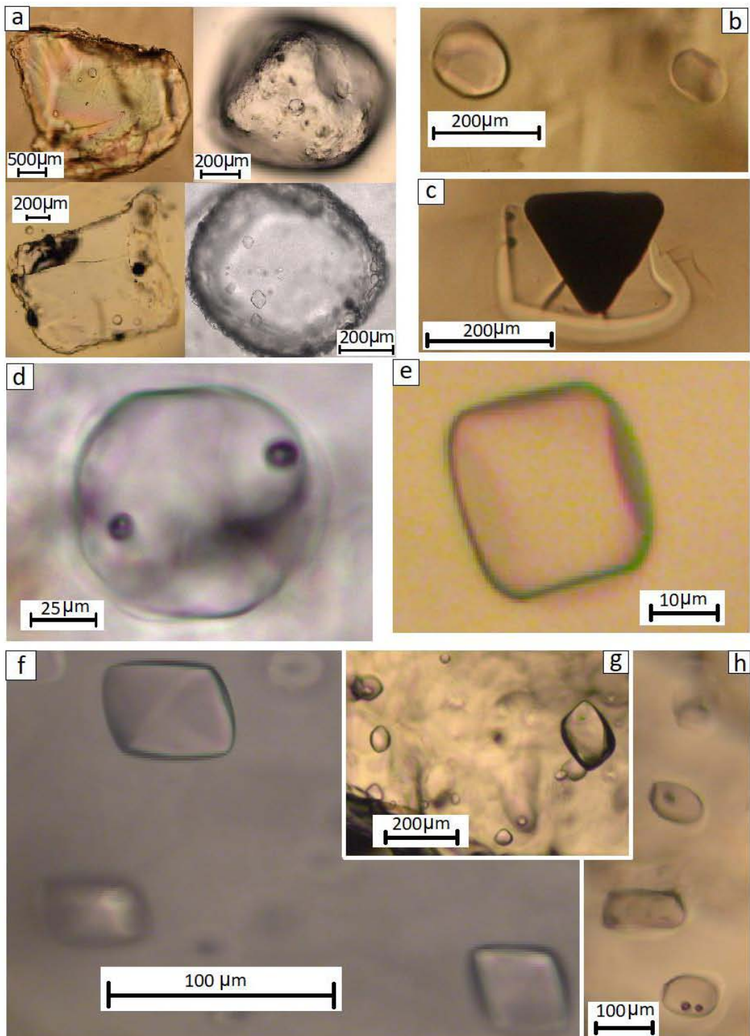
Fig. 4.19. Fotomicrografías con microscopio petrográfico de los cristales e inclusiones de fundido (IFu) de los flujos de pómez (LP16-01VM). a) Cristales huéspedes de cuarzo y sanidino. b) IFu monofásicas y redondeadas en "A1". c) IFu en feldespato "A2", bifásica y fracturada, que parece haber nucleado en una inclusión sólida de ilmenita(?). d) IFu bifásica con dos burbujas en cuarzo "B3". e) Pequeña IFu con forma de cristal negativo en feldespato "F2". f) IFu en cuarzo "H3" con forma de cristal negativo. g) Conjunto de IFu monofásicas dispuestas aleatoriamente en el cuarzo "G3". h) IFu alineadas con distintas formas y tamaños en "H2".
