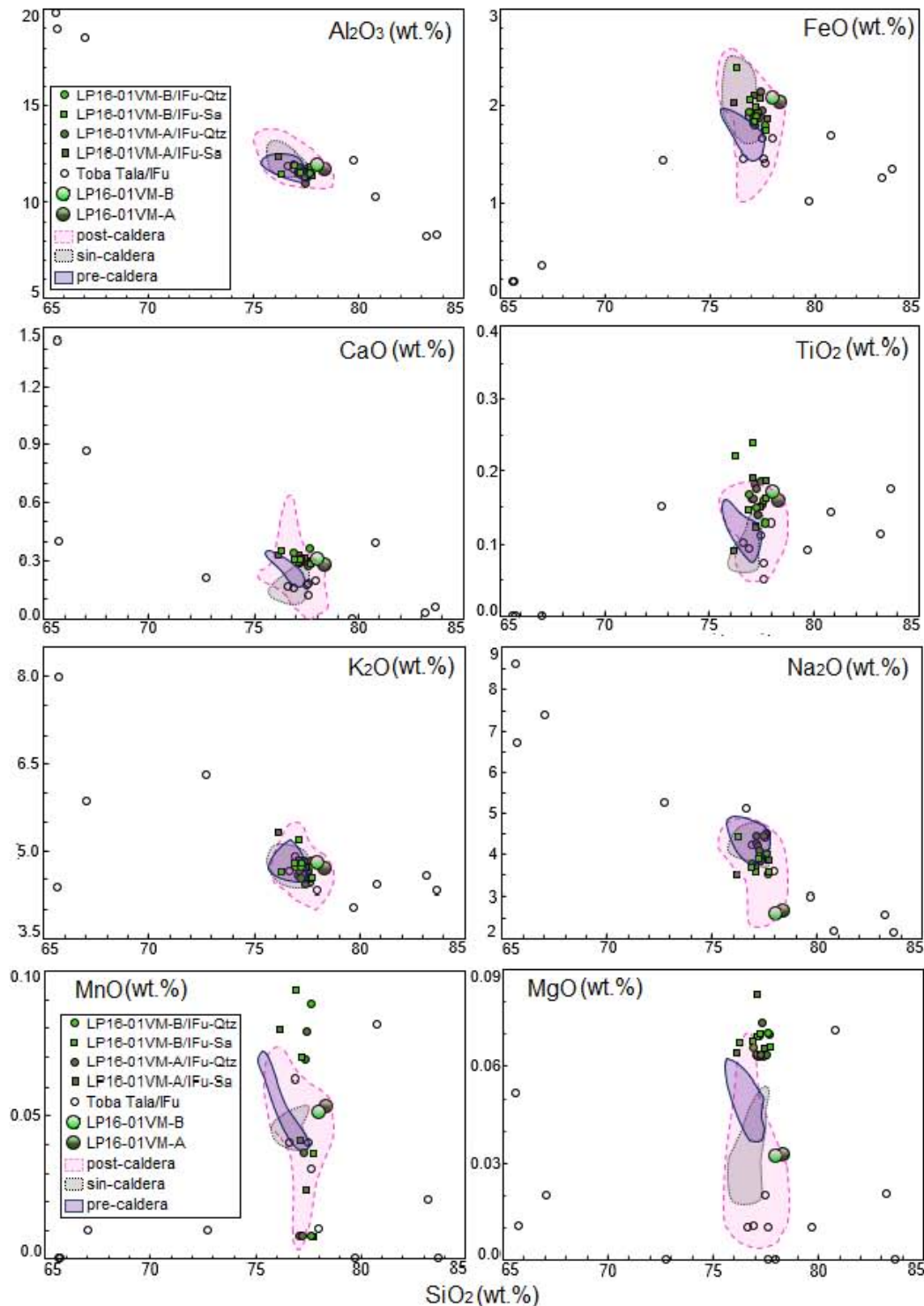
Fig. 4.34. Diagramas Harker para la sección LP16-01VM, horizontes A y B. Se comparan las inclusiones de fundido (círculos y cuadrados pequeños con relleno) y pómez (círculos grandes con relleno) analizadas en esta tesis, con la geoquímica publicada de La Primavera (áreas de color)(Mahood 1977, 1981a y 1981b; Cruz-Lara, 2015; Gómez-Álvarez, 2015; Miguel-Cruz, 2016; Tinoco-Murrillo, 2017; Ávila-Ortiz, 2018; Sourisseau, en proceso), y con la geoquímica de las IFu de Toba Tala (círculos pequeños sin relleno) (Miguel-Cruz, 2016).
