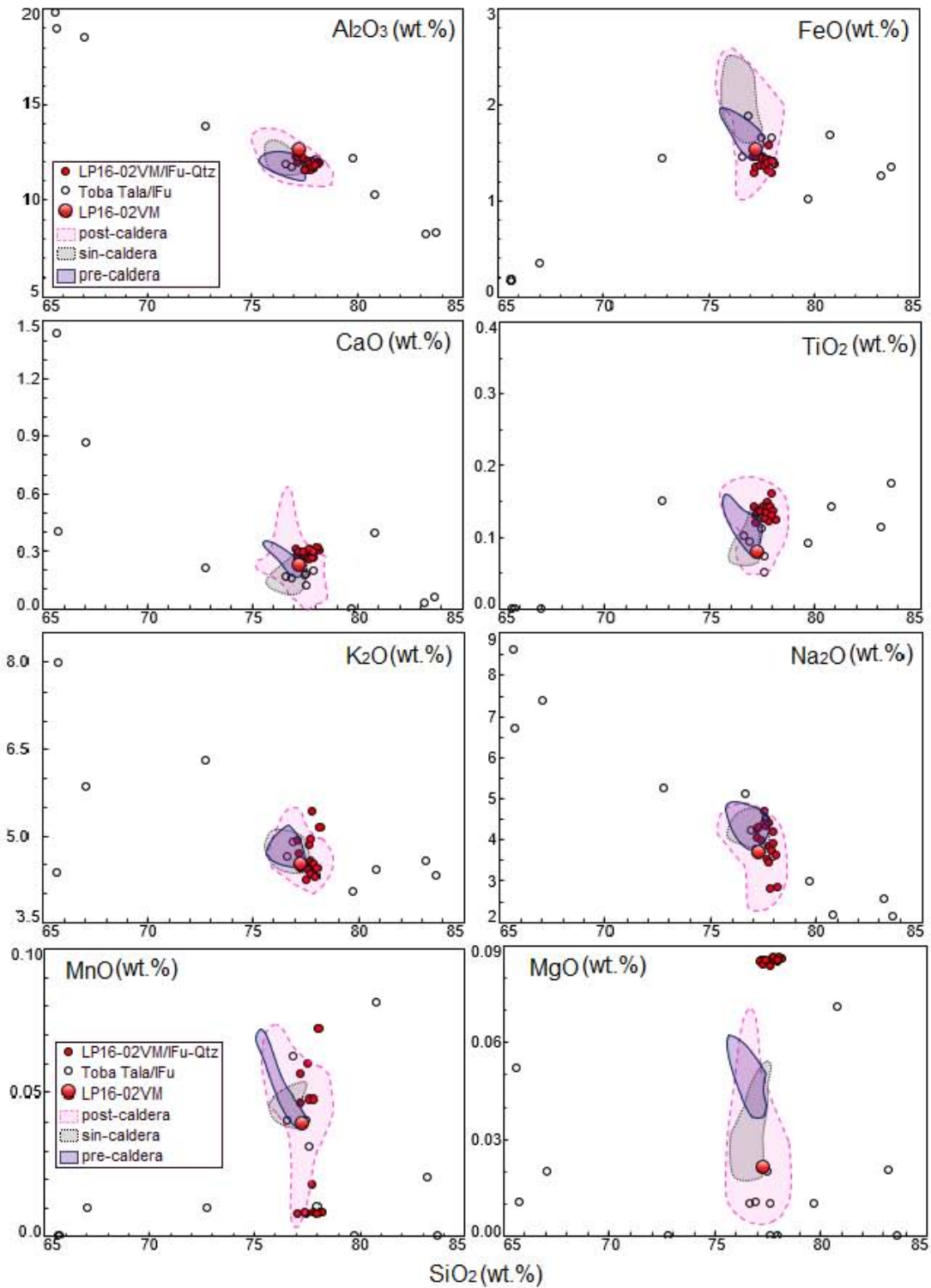
Fig. 4.36. Diagramas Harker para LP16-02VM (horizonte de caídas piroclásticas). Se comparan las inclusiones de fundido (círculos y cuadrados pequeños con relleno) y pómez (círculos grandes con relleno) analizadas en esta tesis, con la geoquímica publicada de La Primavera (áreas de color)(Mahood 1977, 1981a y 1981b; Cruz-Lara, 2015; Gómez-Álvarez, 2015; Miguel-Cruz, 2016; Tinoco-Murrillo, 2017; Ávila-Ortiz, 2018; Sourisseau, en proceso), y con la geoquímica de las IFu de Toba Tala (círculos pequeños sin relleno) (Miguel-Cruz, 2016).
