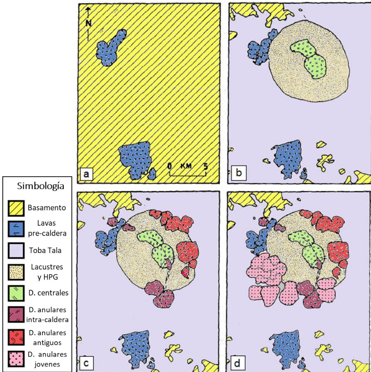
Fig. 4.3. Paleografía de la Caldera de La Primavera. (a) hace 100 ka, después de la erupción de las lavas pre-caldera. (b) hace 95 ka, después de la erupción de la Toba Tala, el colapso de la caldera y la erupción de los domos centrales a través del centro del lago. (c) hace 90 ka, después de la erupción de los antiguos domos anulares. Estos domos anulares hicieron erupción a lo largo de dos arcos paralelos: uno a lo largo de la fractura de anillo en el margen noreste del lago, y el otro a través del medio del lago. La falla intra-caldera y la intrusión del magma parecen haber sido contemporáneas. (d) hace 65 ka, después de la erupción de los domos anulares más jóvenes, a lo largo de la fractura de anillo en el margen sur del lago. Rocas volcánicas pre-Primavera: en amarillo; Lavas pre-caldera: en azul; Toba Tala: en morado claro (sin marcas); Sedimentos del lago: en café con punteado; Domos centrales y domos anulares más antiguas: en verde, violeta y rojo; Domos anulares más jóvenes: en rosa; Fallas: líneas discontinuas. (Mahood, 1980).
