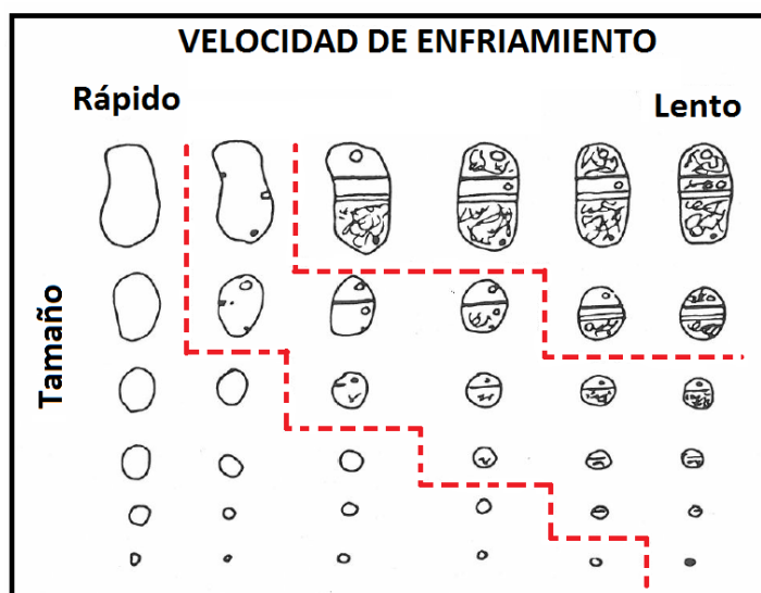
Fig. 3.5. Diagrama que muestra los efectos de la velocidad de enfriamiento y tamaño sobre la nucleación y crecimiento de fases dentro de inclusiones de fundido en olivino. Tomada de Roedder (1979).
