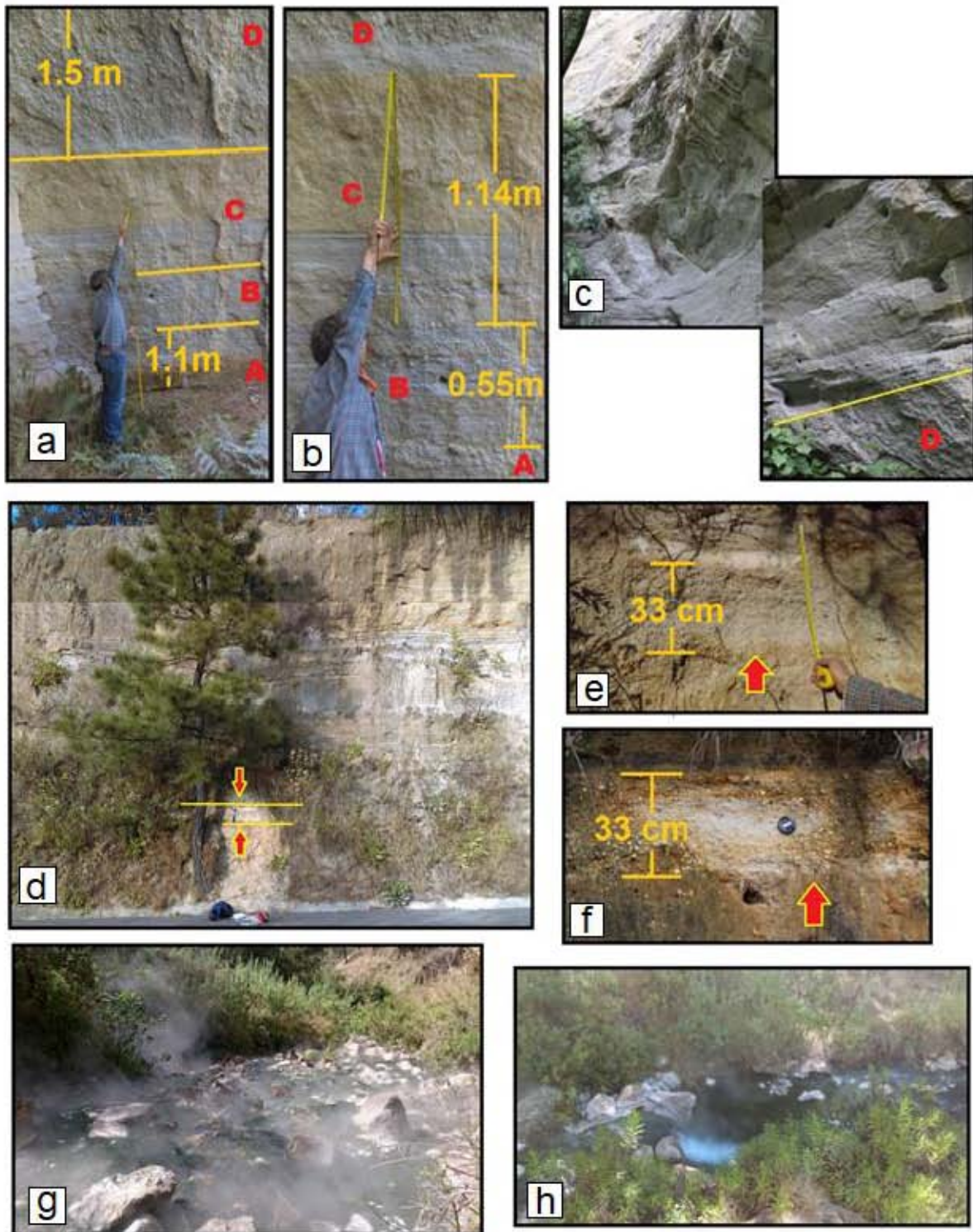
Fig. 4.11. a-c) Fotografías de la sección LP16-01VM, se muestra el espesor de las partes en las que se dividió la sección. d) Sección LP16-02VM. e) y f) Detalle mostrando y señalando el espesor donde se tomó LP16-02VM, fotografías tomadas en distintas salidas de campo. g) y h) Rio Caliente al noroeste de la caldera, la temperatura del agua se encuentra aproximadamente a 70°C.
