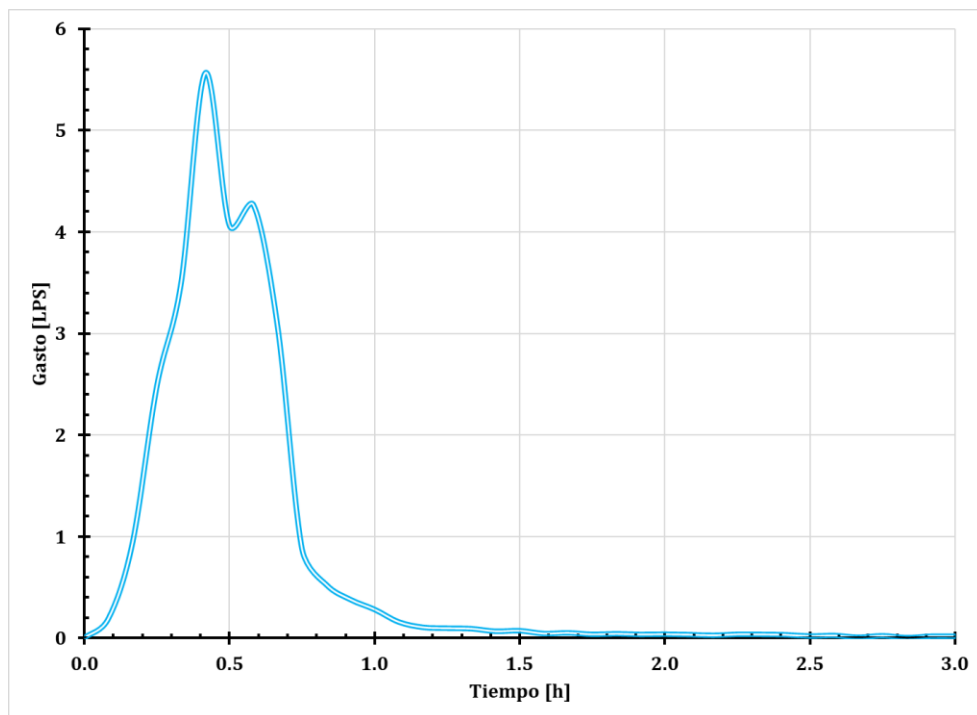
Figura 72. Hidrograma nodo 76.
