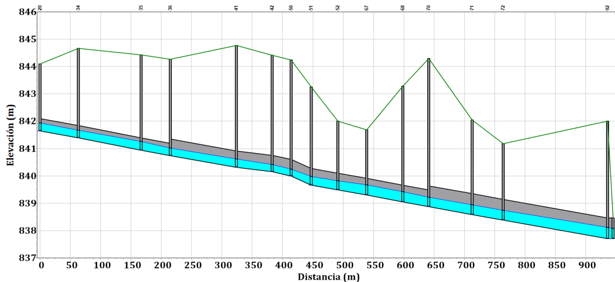
Figura 26. Perfil del colector más desfavorable (fórmula racional).
