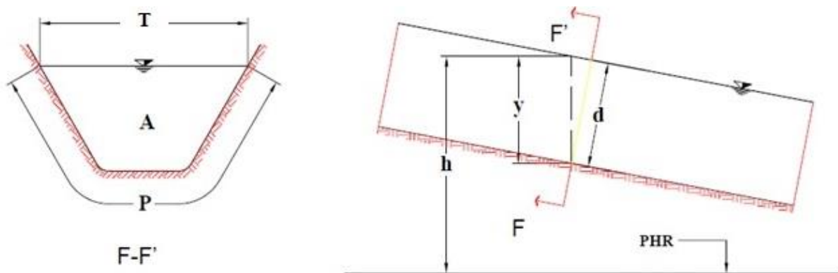
Figura 6. Parámetros hidráulicos en una sección a superficie libre.
