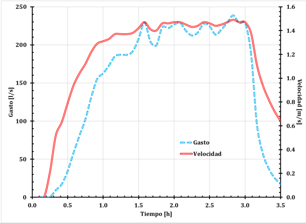
Figura 54. Gráfica del tubo 128 (tramo 92-91).
