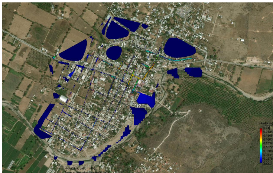
Figura 47. Modelo de IBER.
