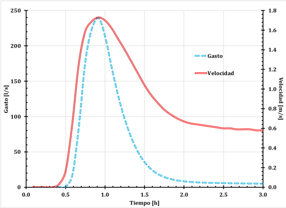
Figura 42. Gráfica del tubo 63 (tramo 42-50).
