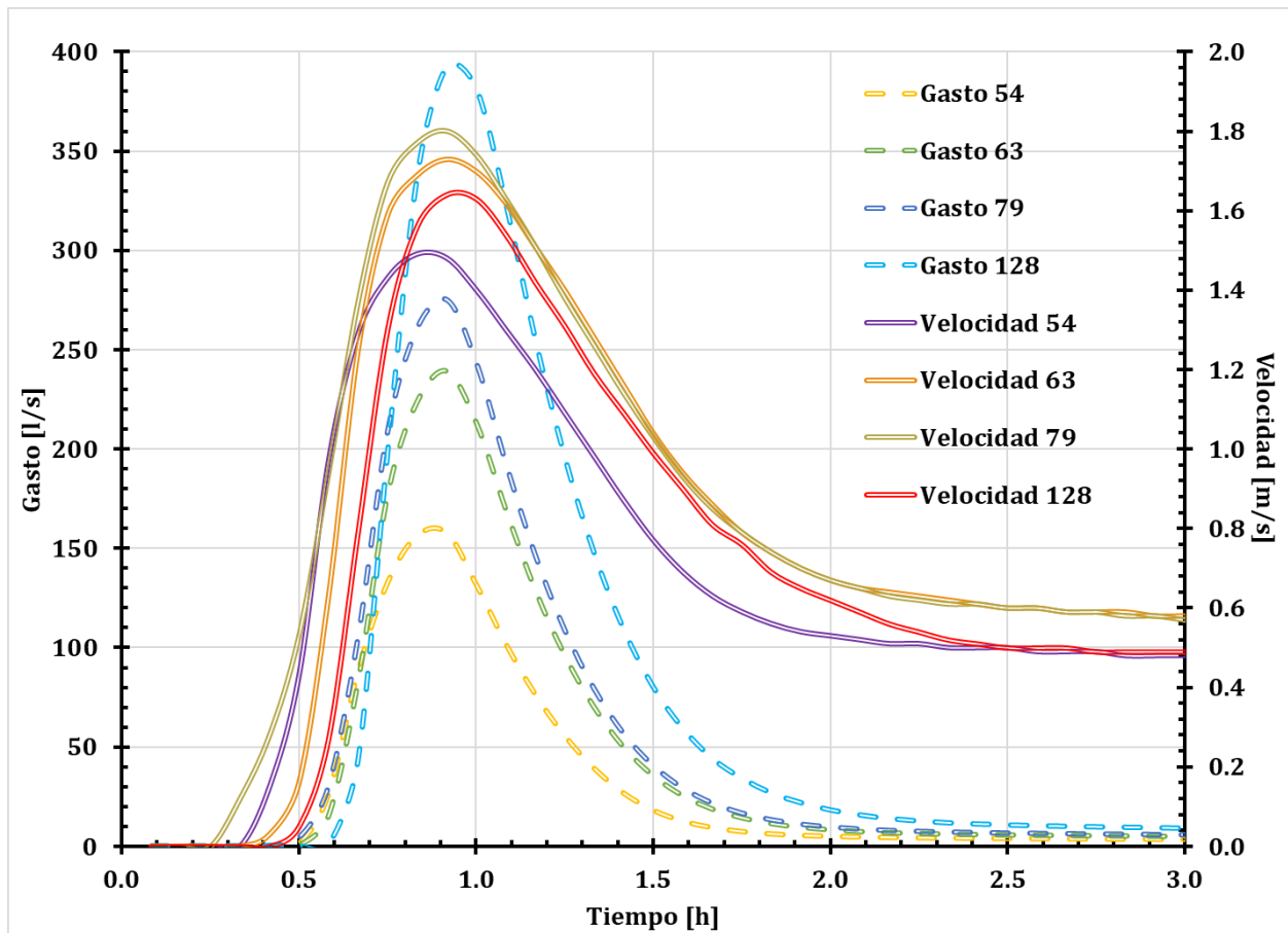
Figura 45. Resumen de gasto y velocidad del colector más desfavorable.
