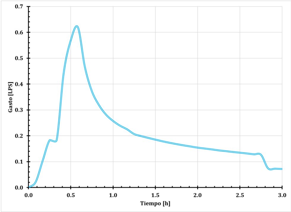
Figura 66. Hidrograma nodo 31.
