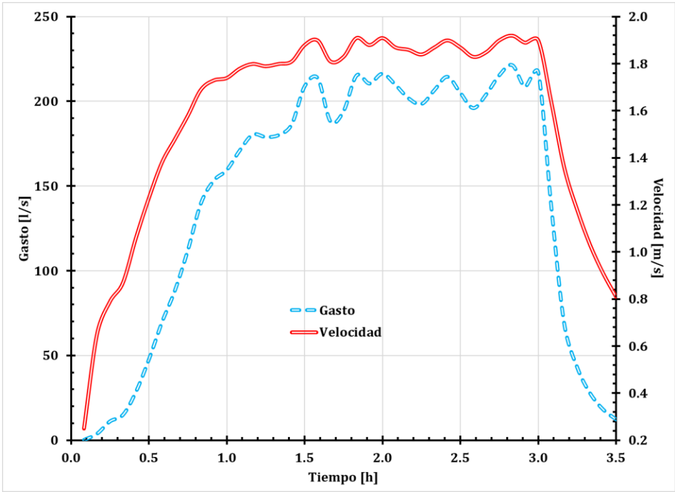
Figura 53. Gráfica del tubo 125 (tramo 70-71).
