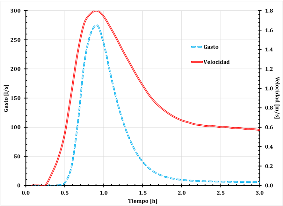
Figura 43. Gráfica del tubo 79 (tramo 50-51).
