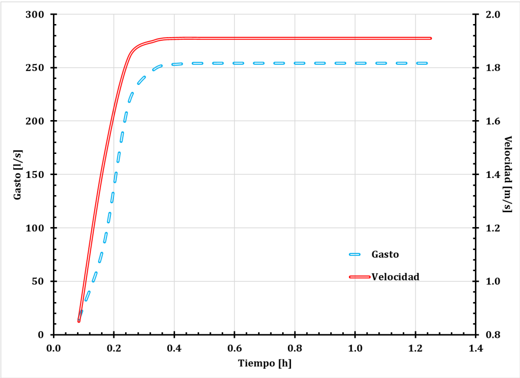
Figura 31. Gráfica del tubo 79 (tramo 50-51).
