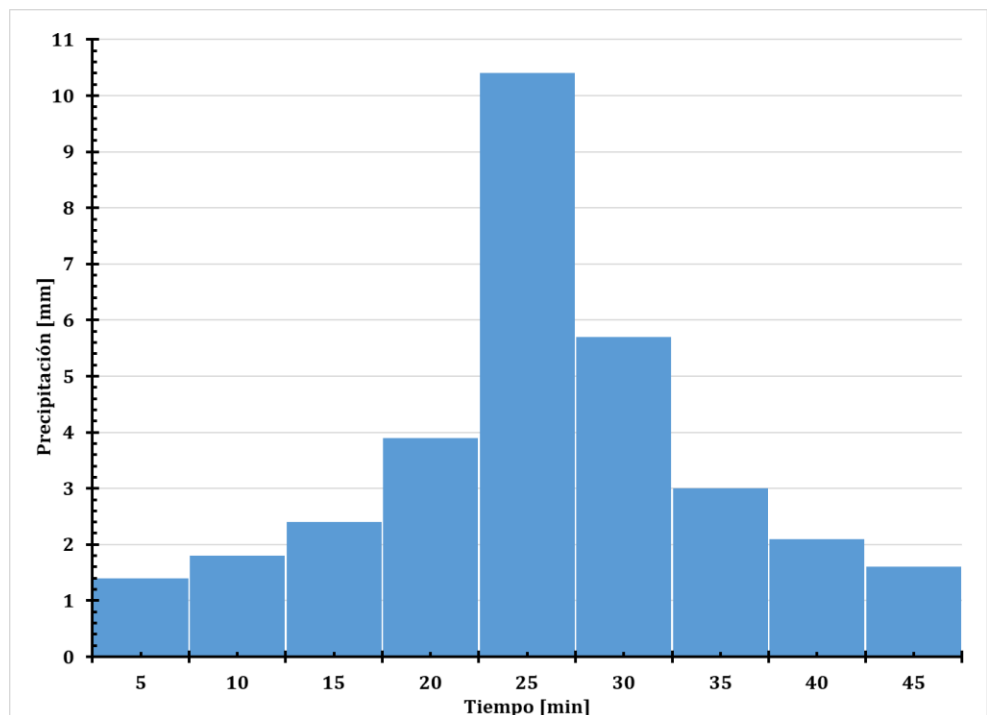
Figura 35. Hietograma de precipitación total.
