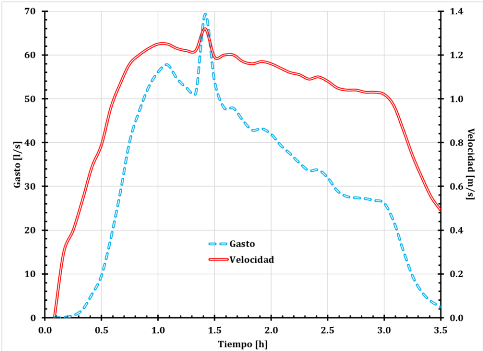
Figura 49. Gráfica del tubo 54 (tramo 20-34).
