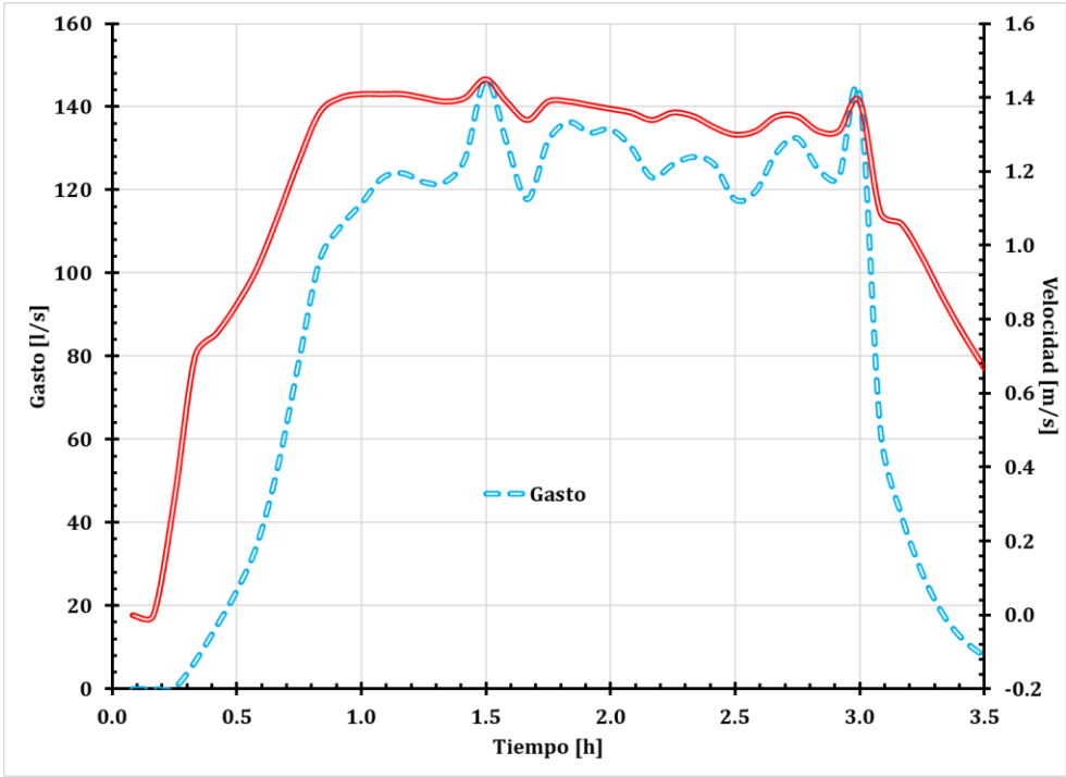
Figura 52. Gráfica del tubo 81 (tramo 52-67).
