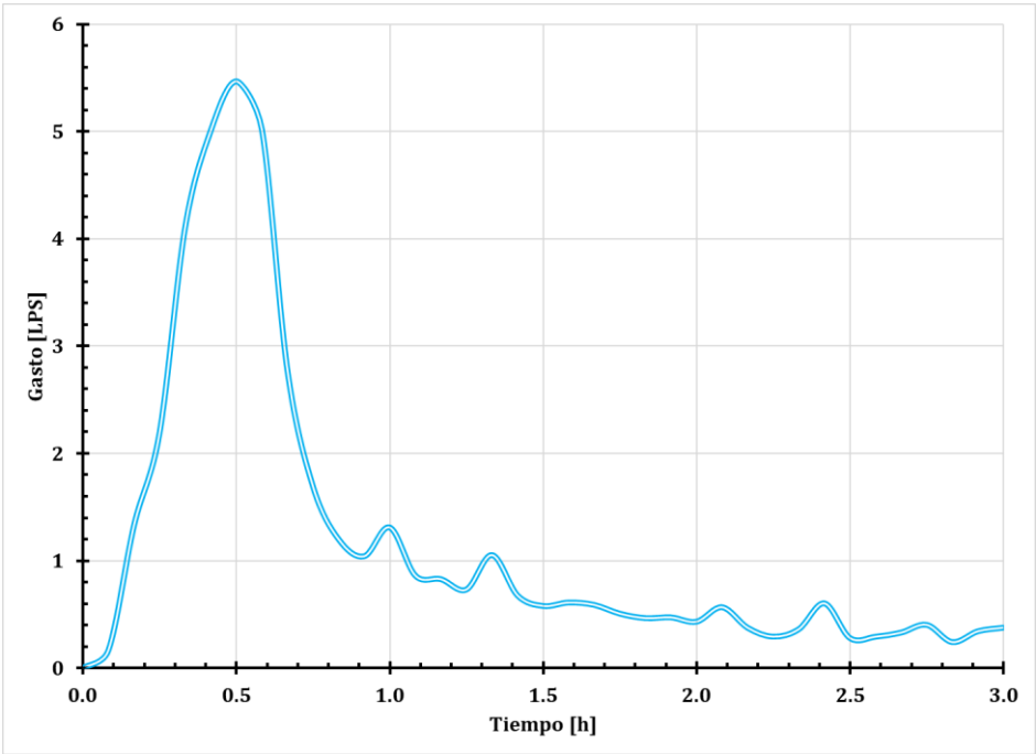
Figura 64. Hidrograma nodo 38.
