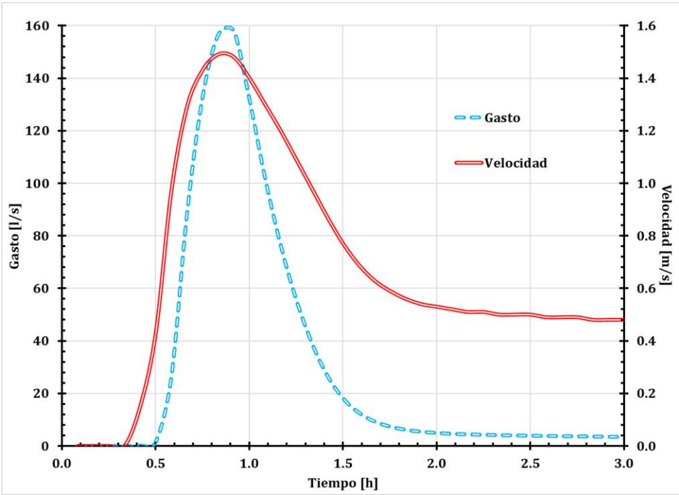
Figura 41. Gráfica del tubo 54 (tramo 20-34).
