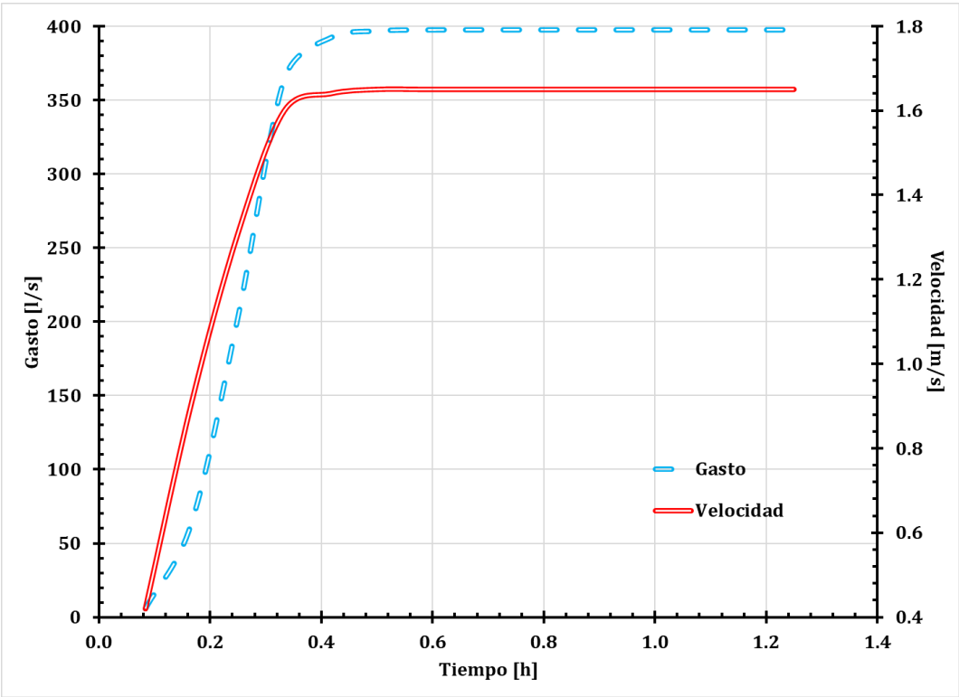
Figura 33. Gráfica del tubo 128 (tramo 92-91).
