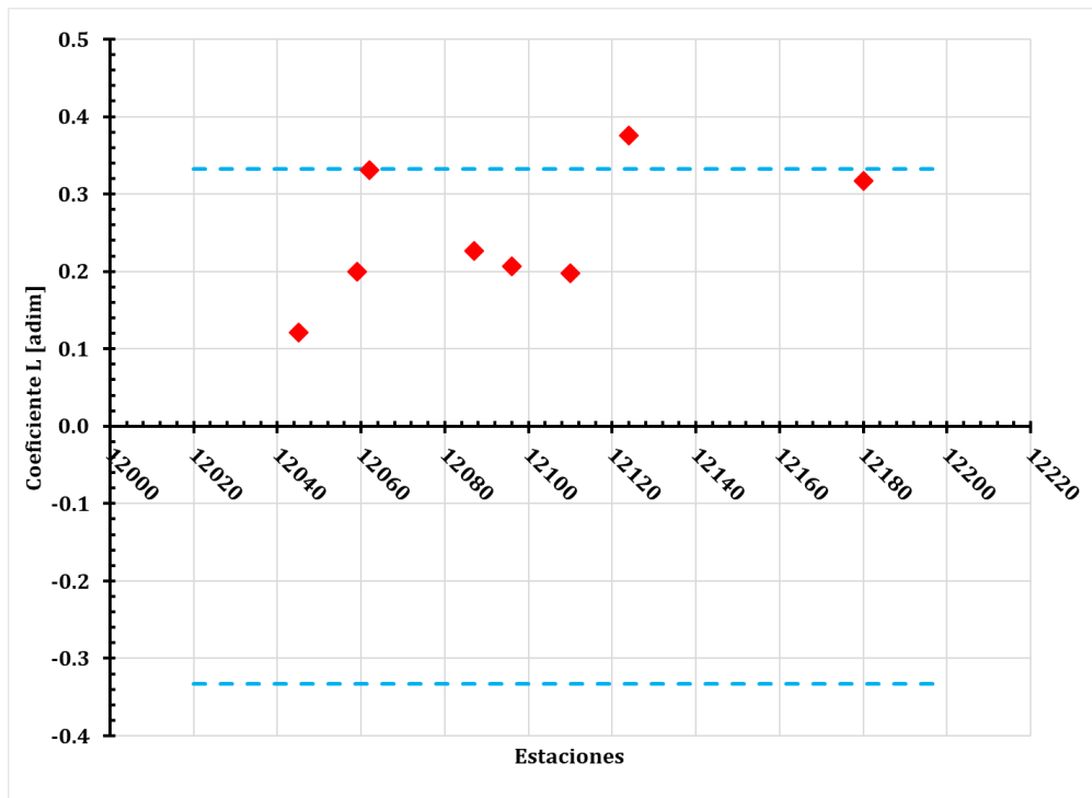
Figura 19. Gráfica Coeficiente de variación L.
