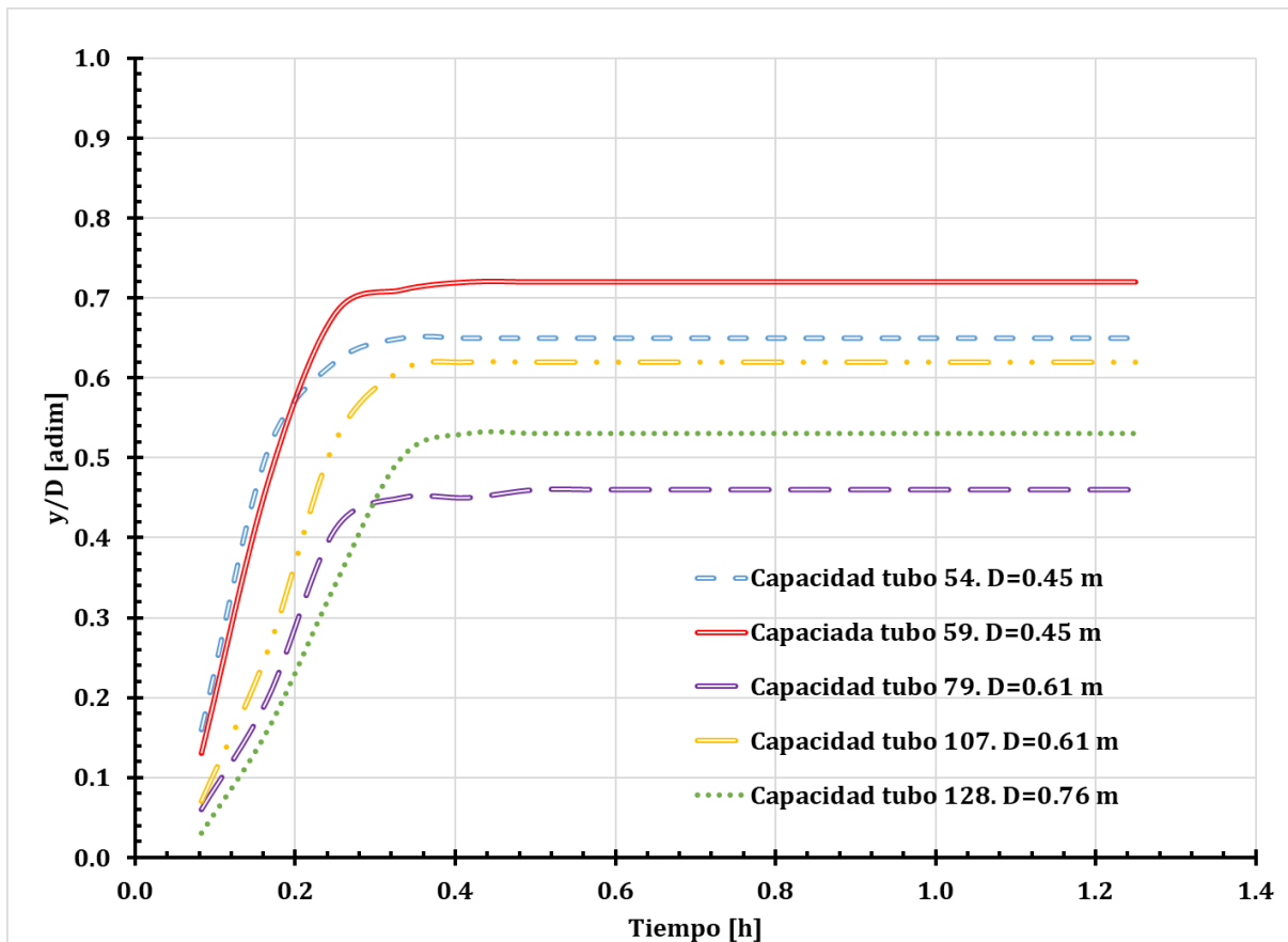
Figura 28. Capacidad del colector más desfavorable.
