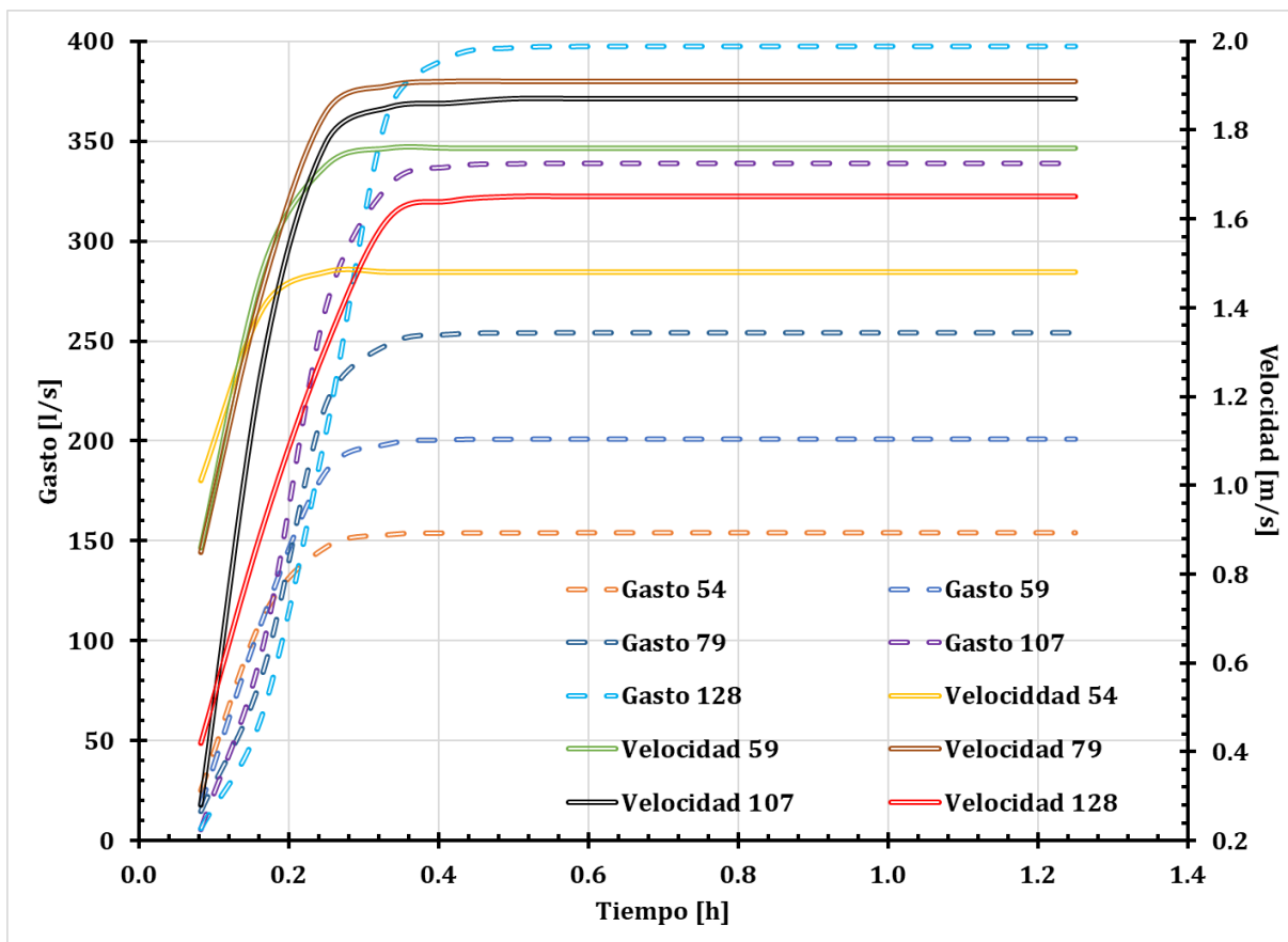
Figura 34. Resumen de gasto y velocidad del colector.
