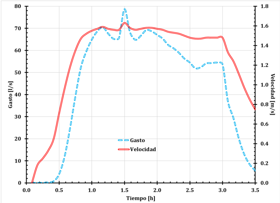
Figura 50. Gráfica del tubo 62 (tramo 41-42).
