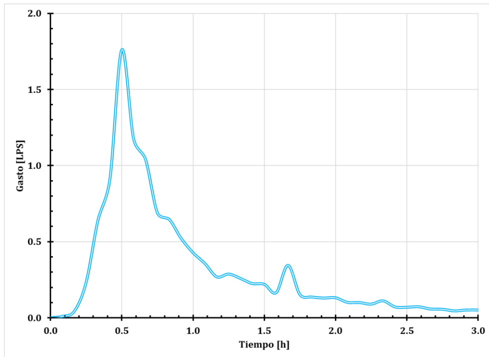
Figura 71. Hidrograma nodo 6.
