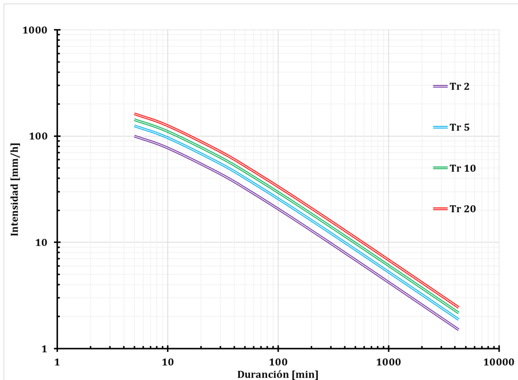
Figura 22. Curvas IDT.
