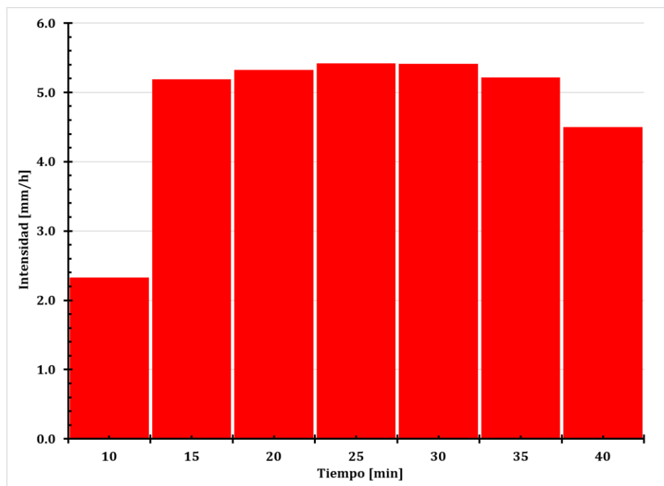
Figura 24. Hietograma de intensidad efectiva.
