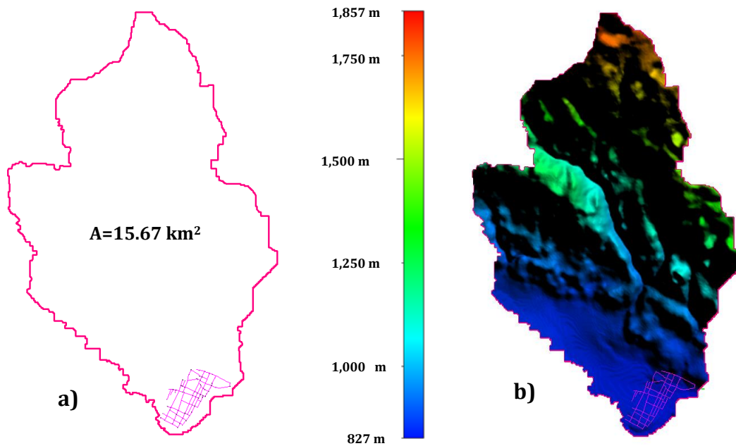
Figura 12. Parteaguas (a) y modelo digital de terreno (b) de la cuenca de estudio.
