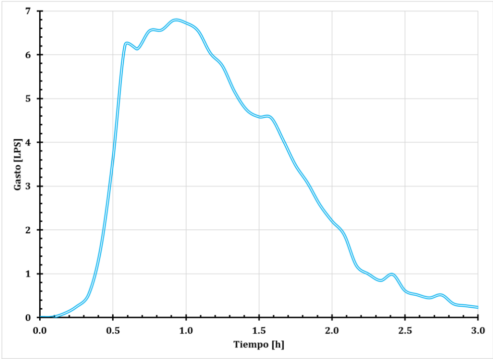
Figura 68. Hidrograma nodo 13.
