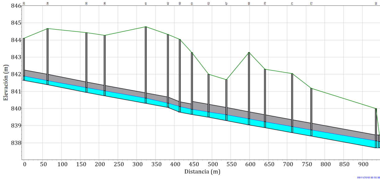
Figura 37. Perfil del colector más desfavorable (EPA SWMM).
