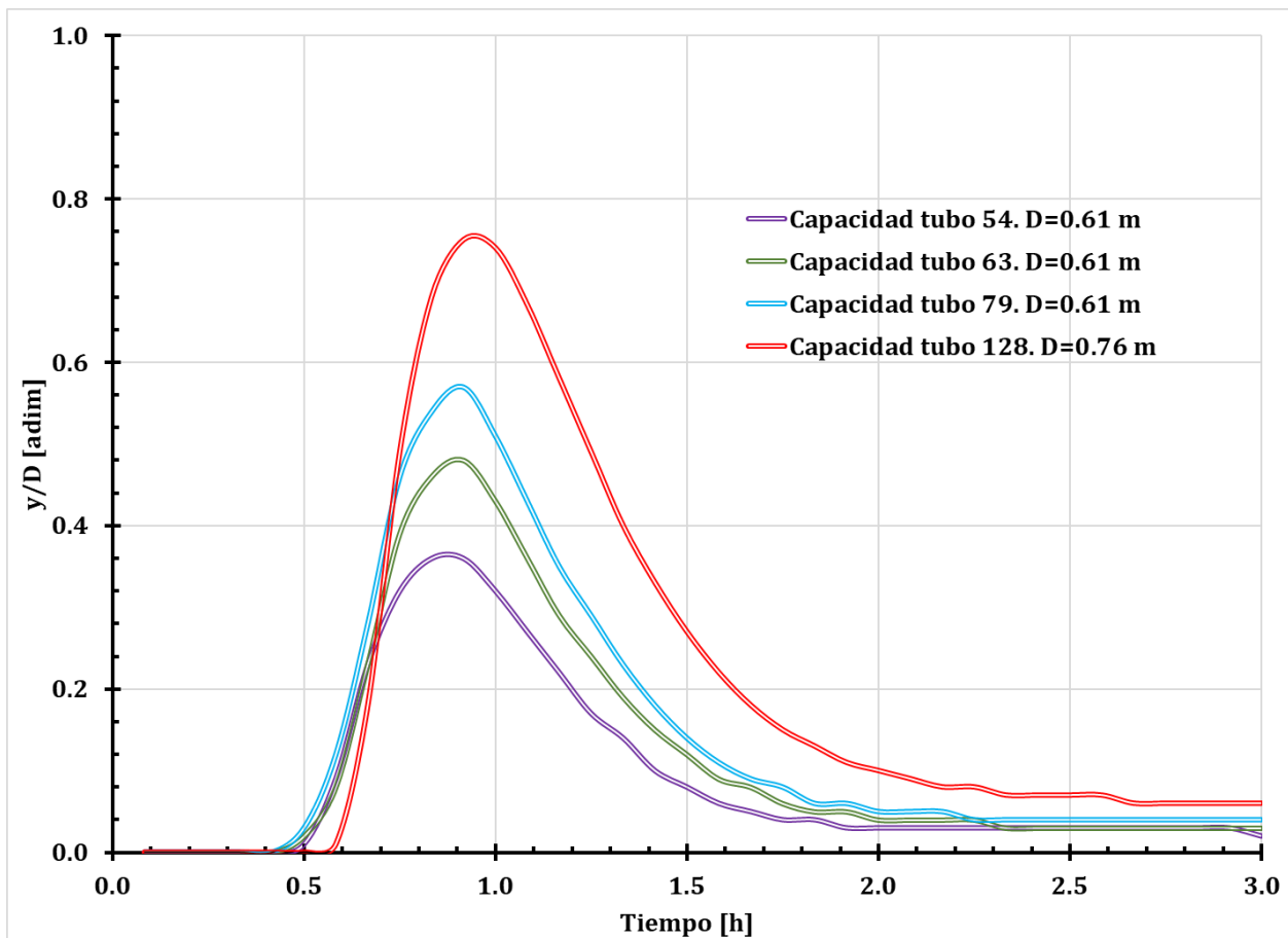
Figura 40. Capacidad de los tubos del colector más desfavorable.
