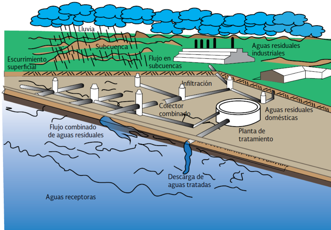
Figura 1. Sistema de drenaje combinado (adaptado de Kibler, 1982, MAPAS 2012).
