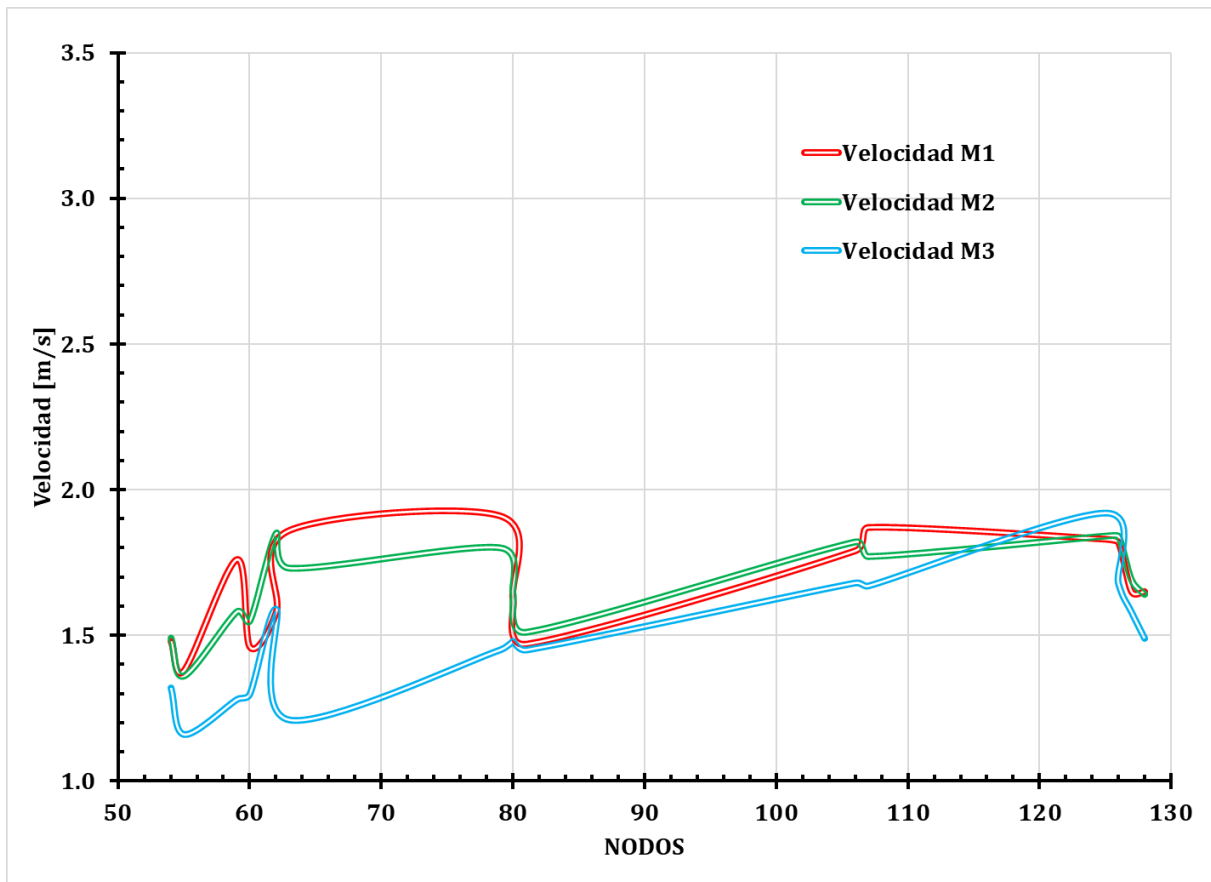
Figura 60. Variación de velocidad en el colector.
