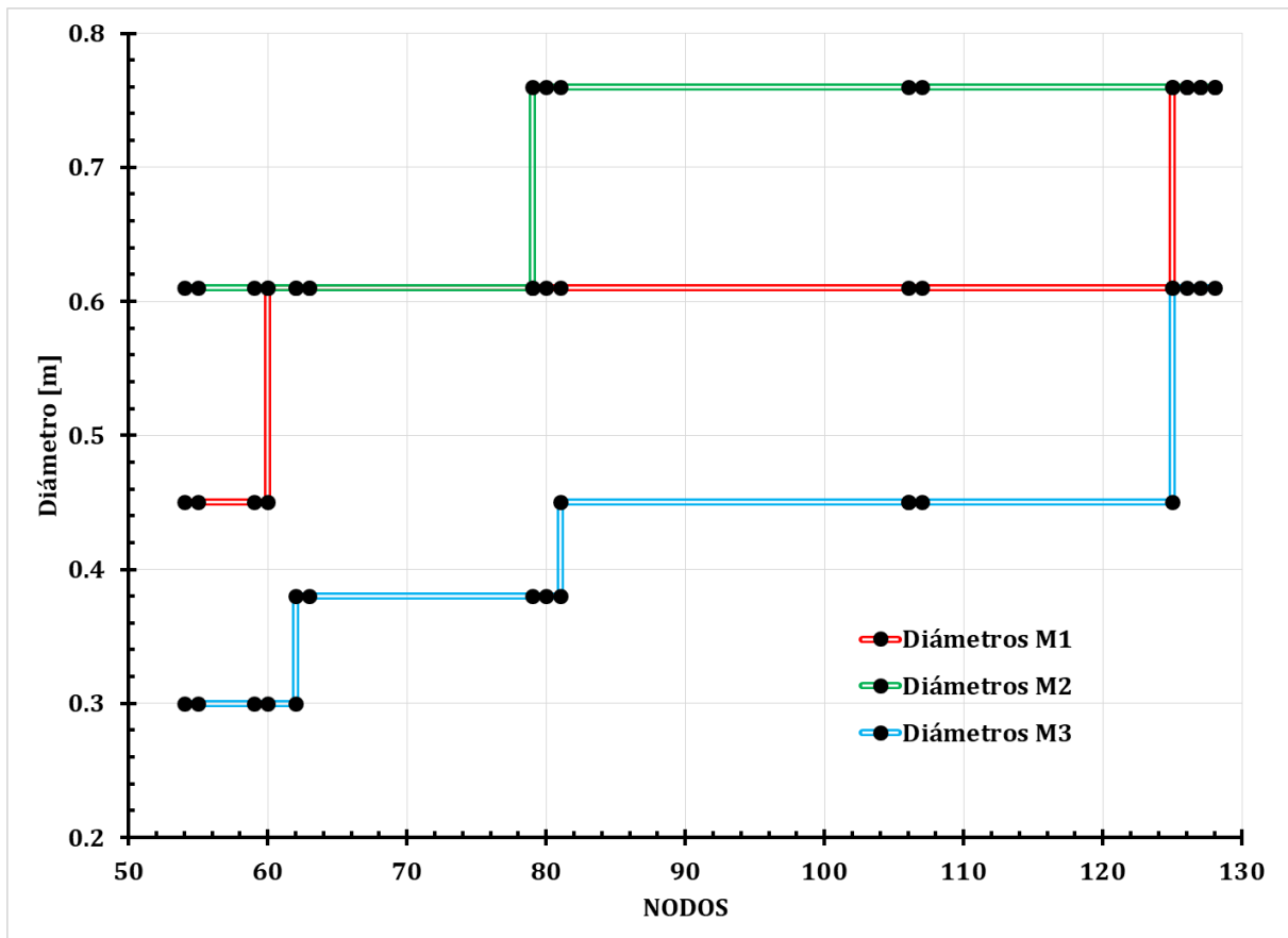
Figura 59. Variación de diámetros.
