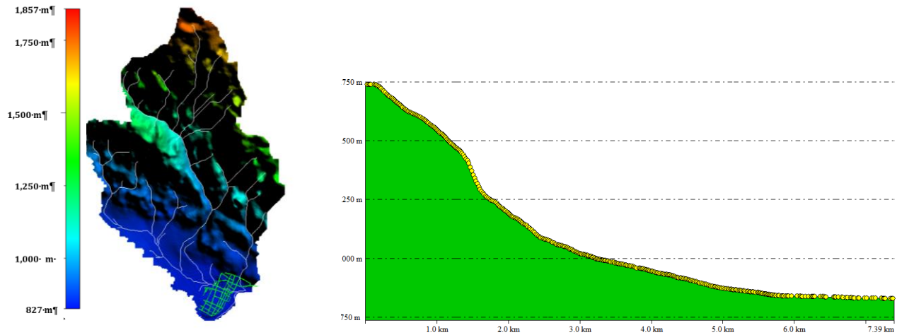
Figura 17. Red de drenaje natural y perfil del cauce principal.
