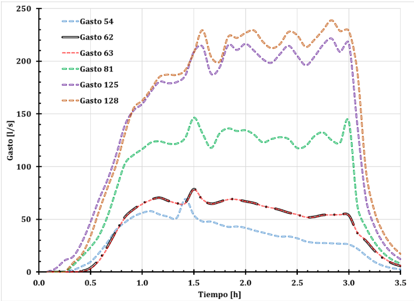
Figura 55. Resumen de gastos del colector.
