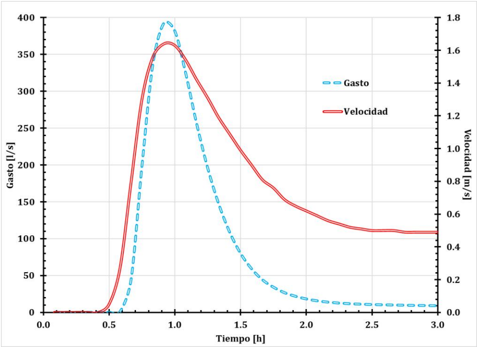
Figura 44. Gráfica del tubo 128 (tramo 92-91).
