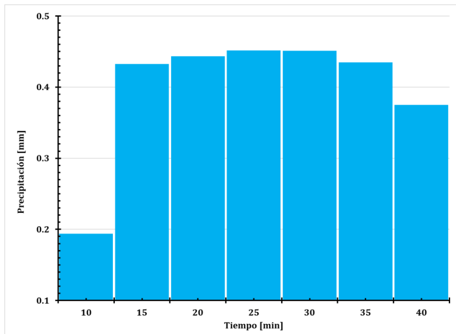
Figura 23. Hietograma de precipitación efectiva.
