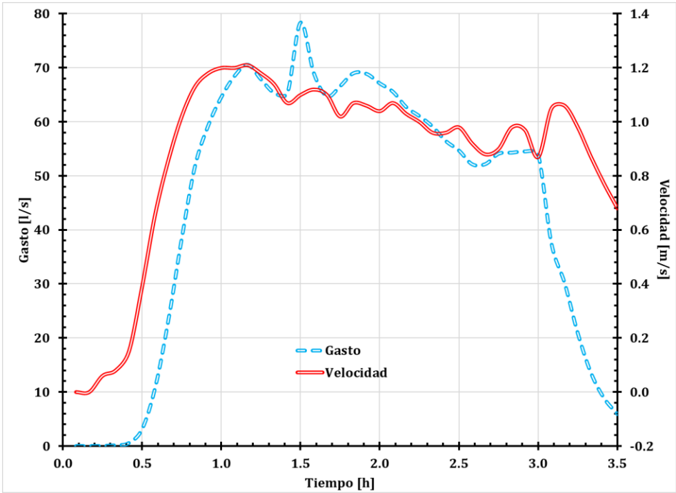
Figura 51. Gráfica del tubo 63 (tramo 42-50).
