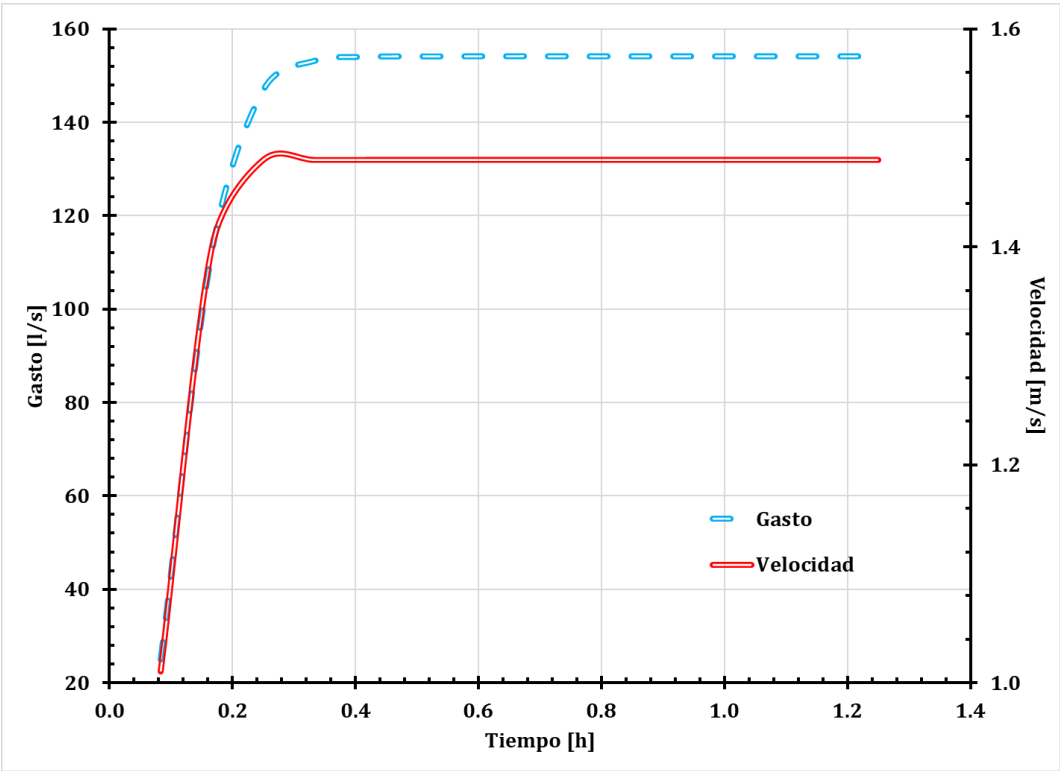
Figura 29. Gráfica del tubo 54 (tramo 20-34).
