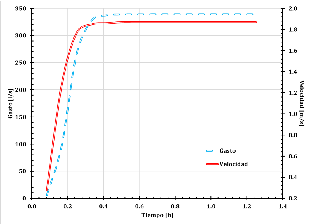
Figura 32. Gráfica del tubo 107 (tramo 68-70).
