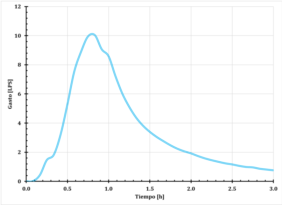
Figura 69. Hidrograma nodo 12.
