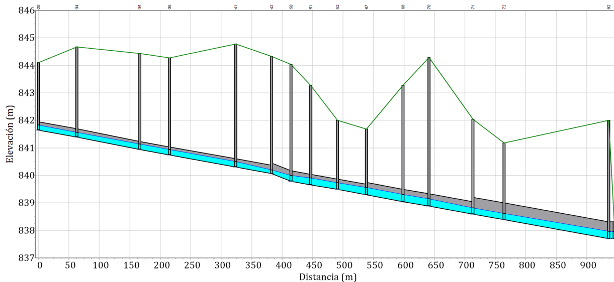
Figura 48. Perfil del colector más desfavorable (IBER).
