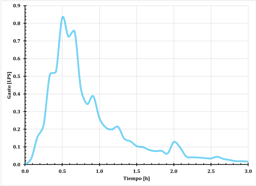
Figura 70. Hidrograma nodo 10.
