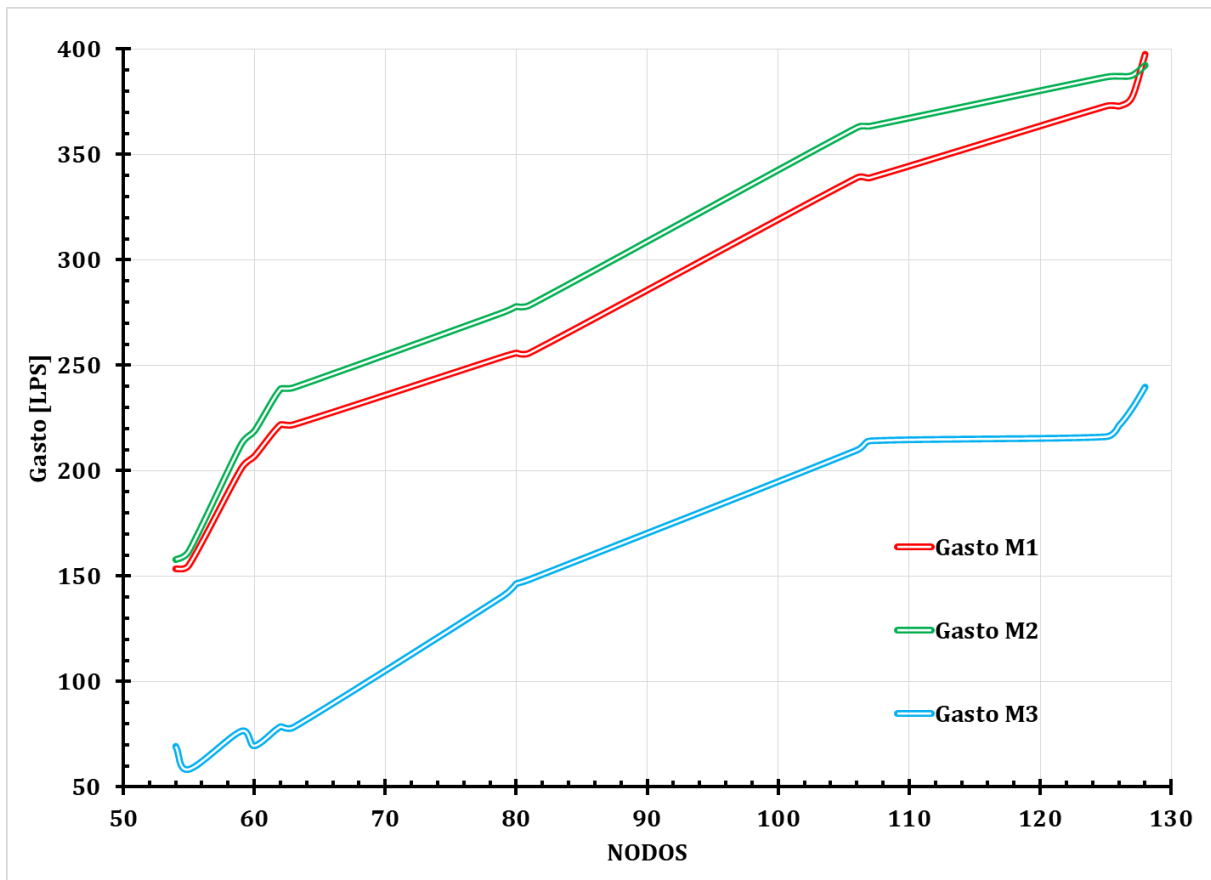
Figura 61. Variación de gastos.
