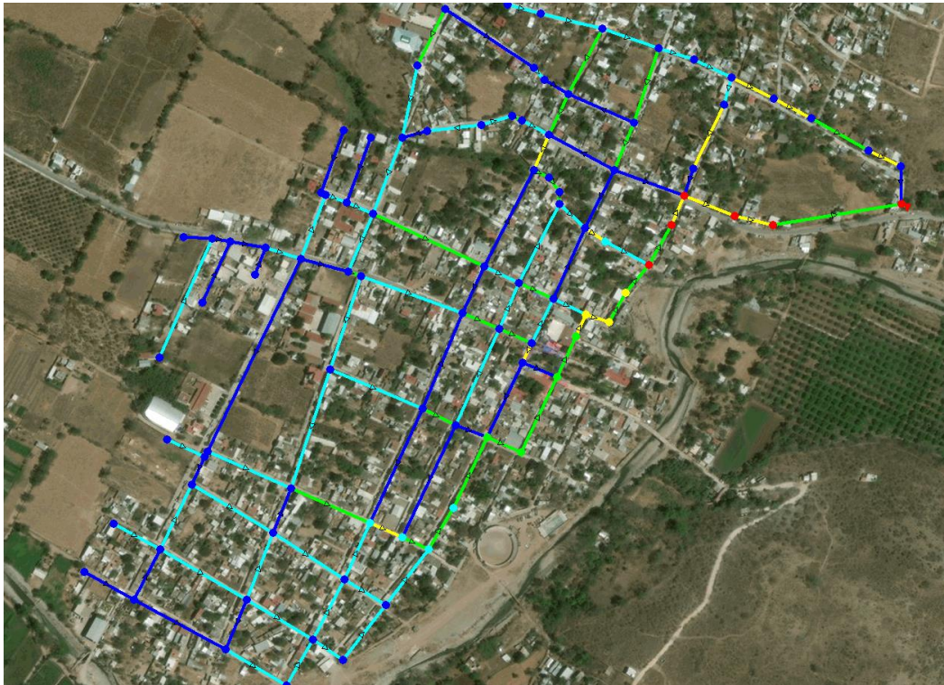
Figura 27. Red de drenaje pluvial diseñada con la fórmula racional.
