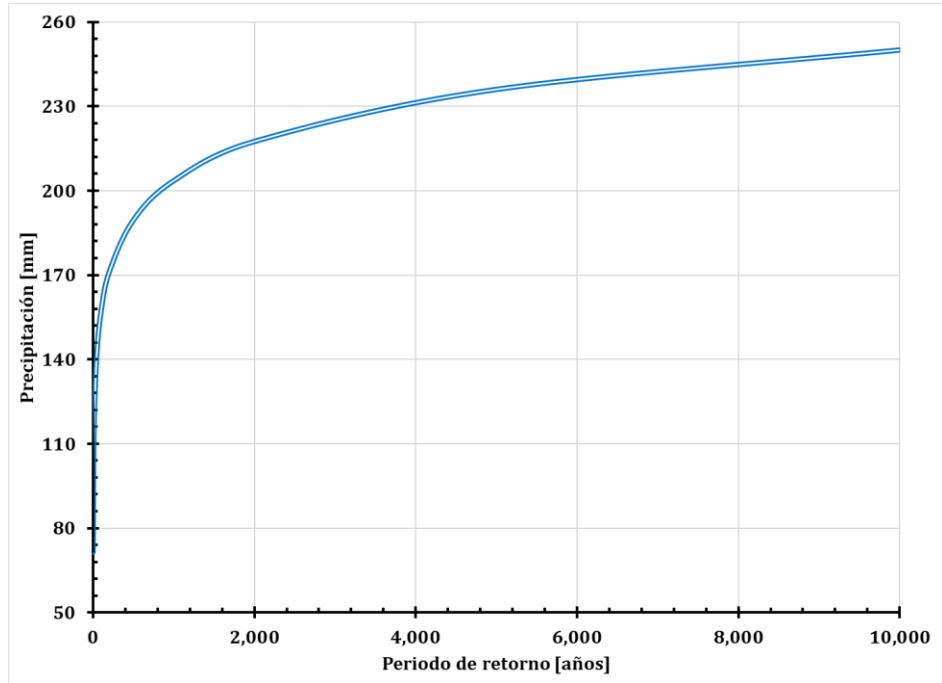
Figura 20. Gráfica de la función Gumbel de dos parámetros
