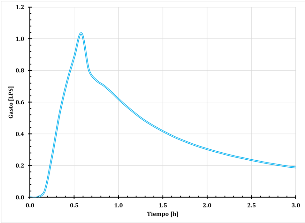
Figura 65. Hidrograma nodo 34.
