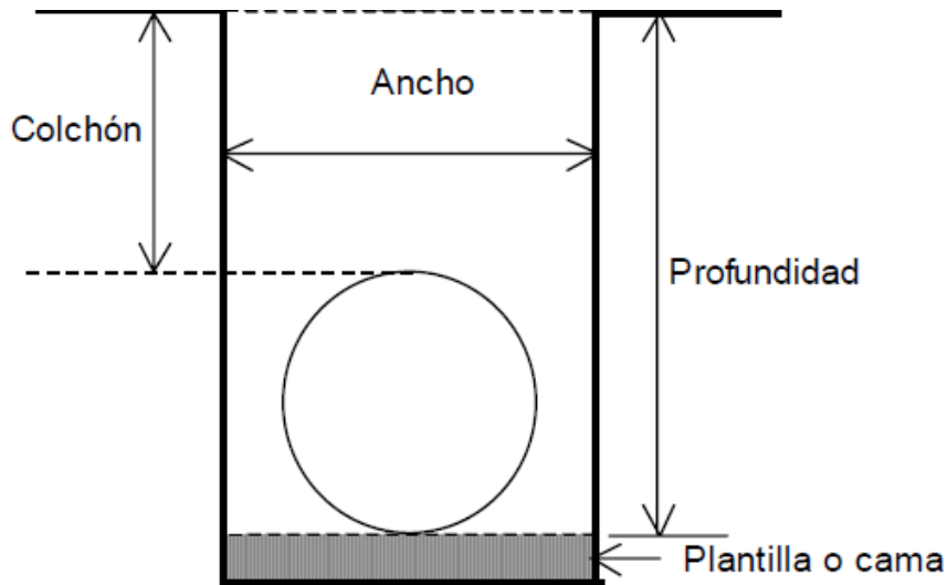
Figura 9. Características de una zanja
