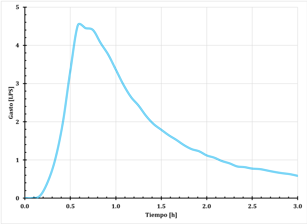
Figura 67. Hidrograma nodo 20.
