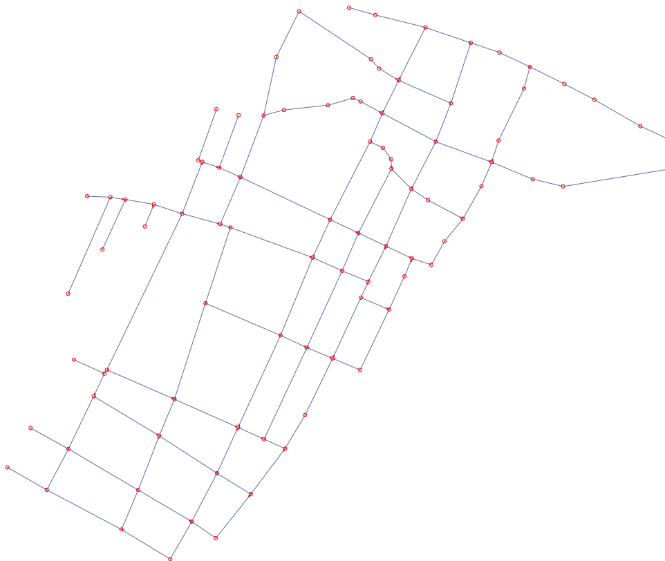
Figura 25. Ubicación de pozos de visita y red de drenaje.
