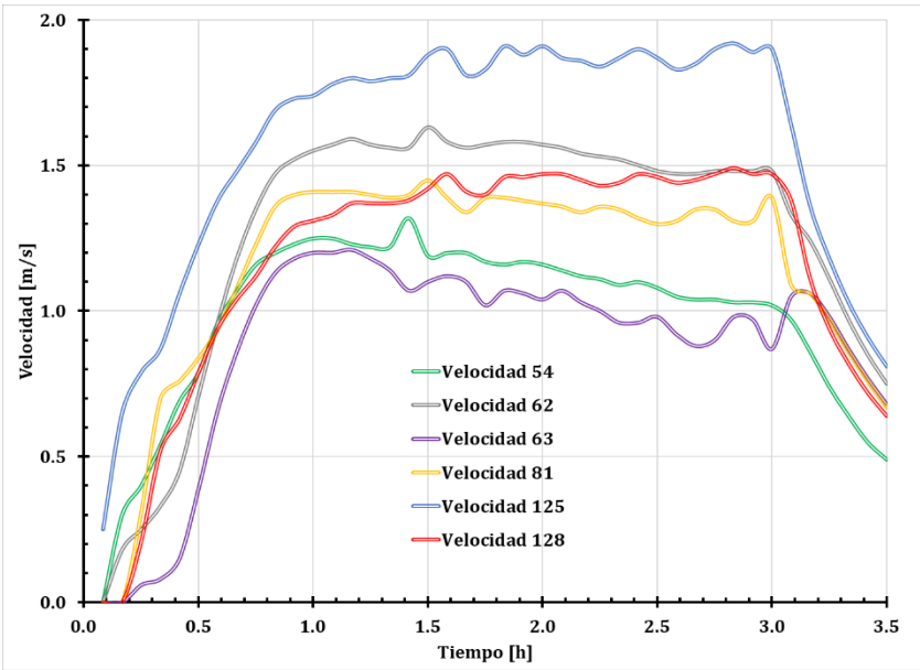
Figura 56. Resumen de velocidades del colector.
