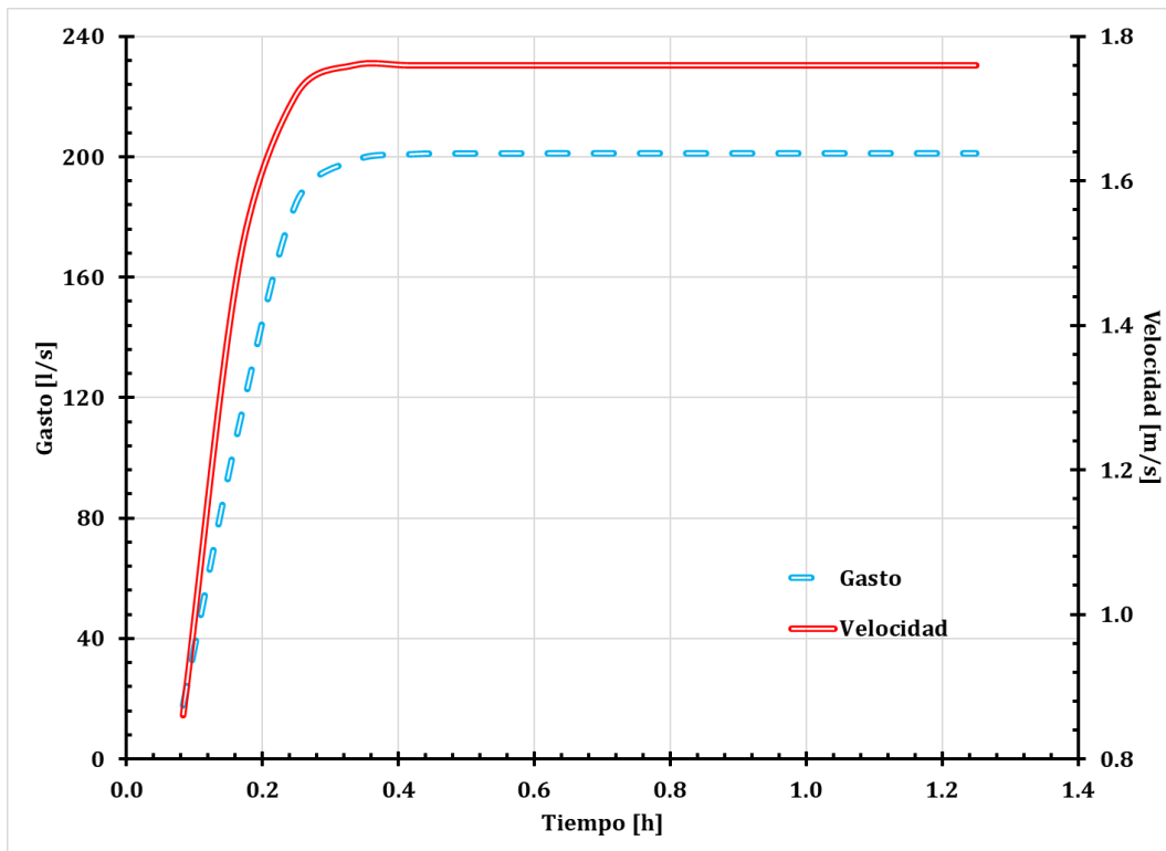
Figura 30. Gráfica del tubo 59 (tramo 35-36).
