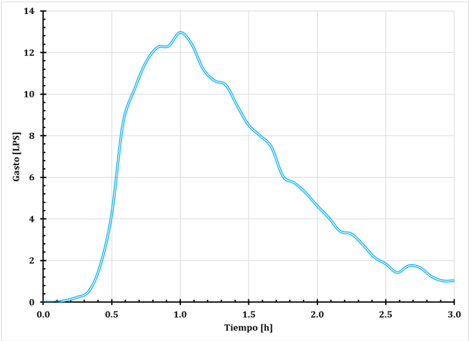
Figura 63. Hidrograma nodo 43.
