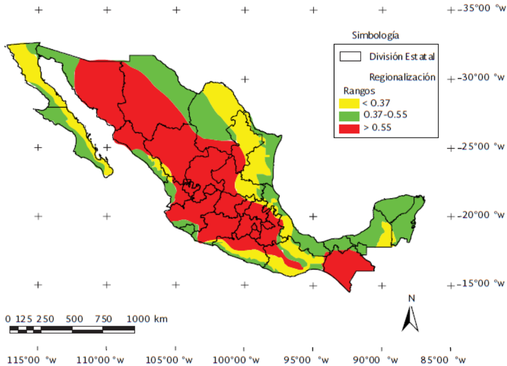
Figura 21. Factor “R” por región (adaptado de Baeza, 2007).
