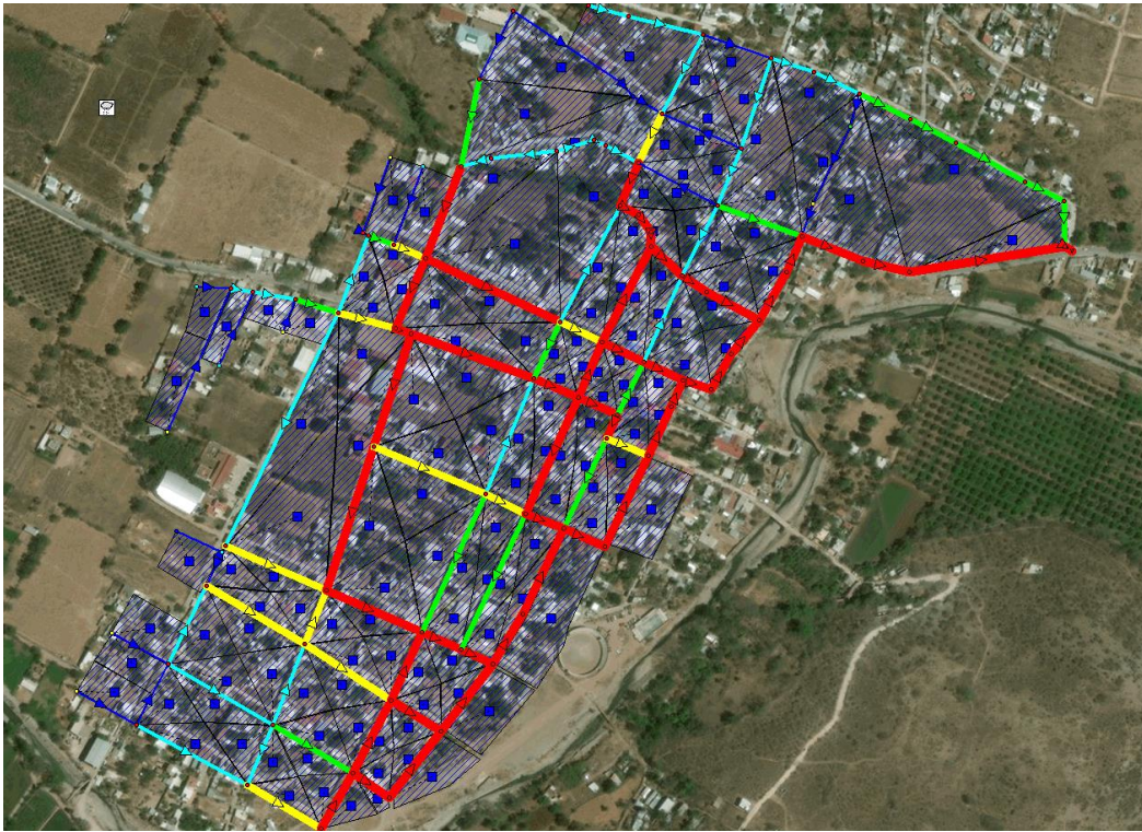
Figura 36. Red de drenaje pluvial diseñada con EPA SWMM.
