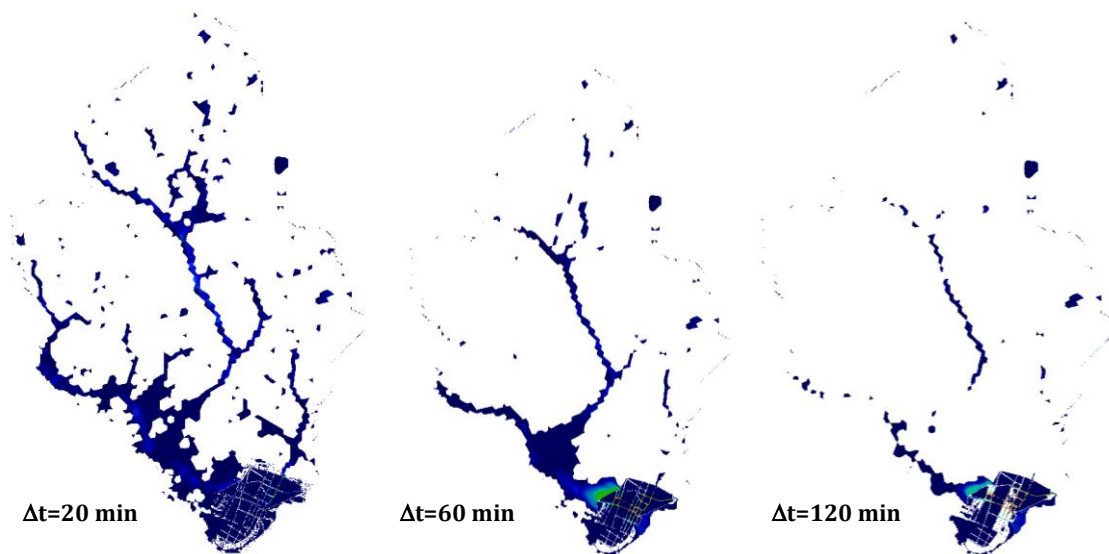
Figura 58. Tirantes en la zona de estudio (escala 0.001 [m]).
