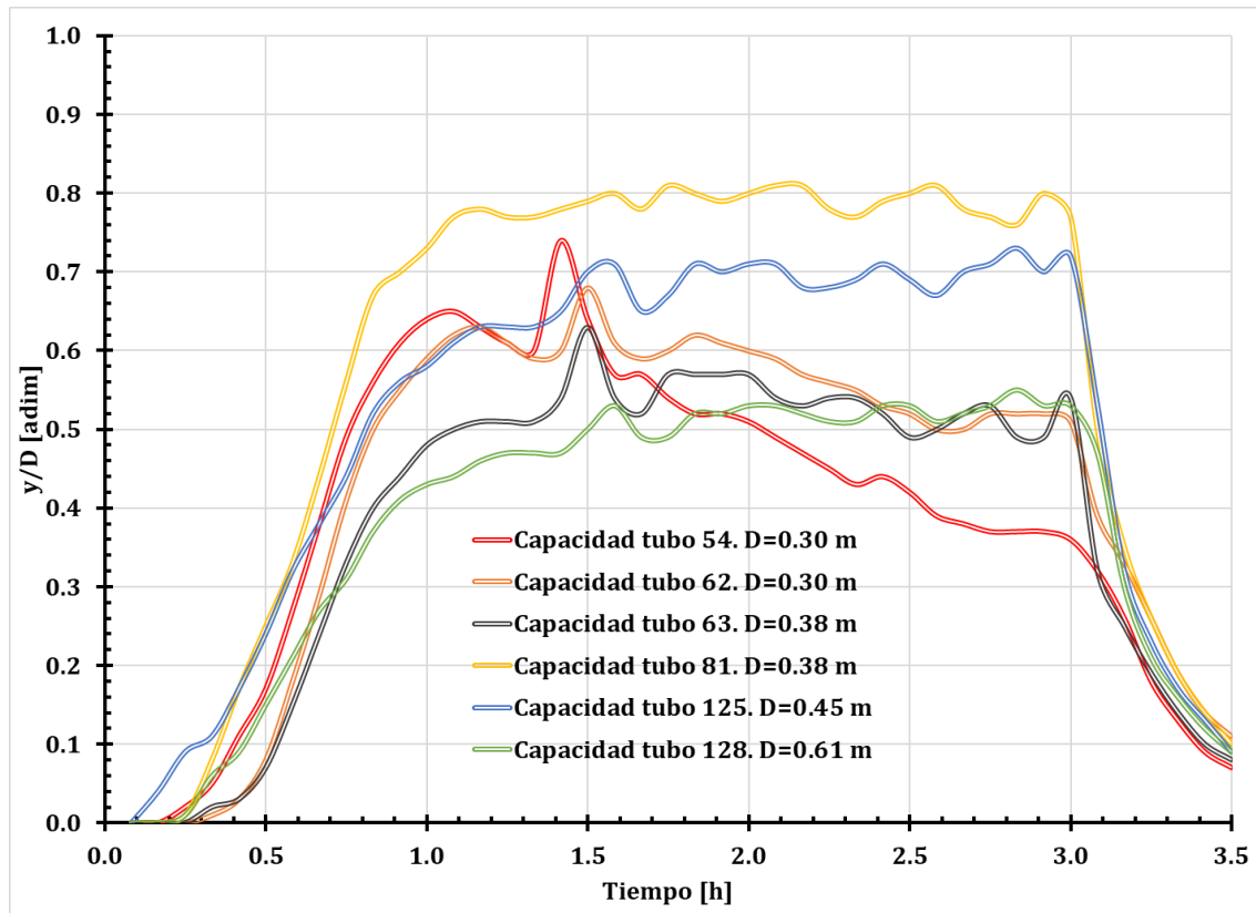
Figura 57. Capacidad del colector más desfavorable.
