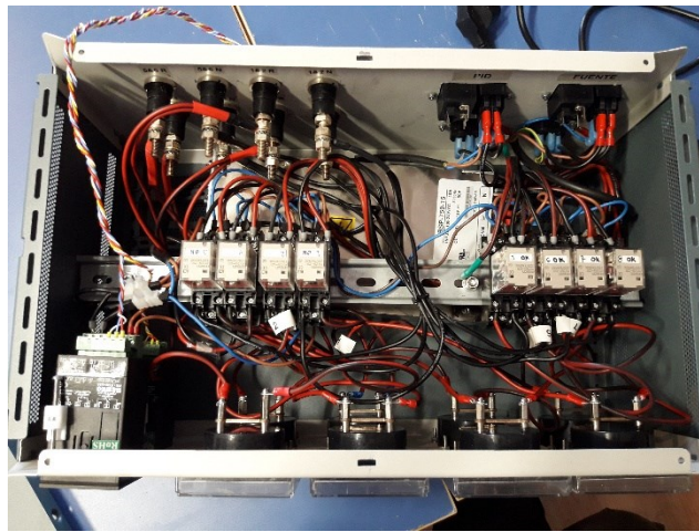
Figura 1.4 Contenido interno del antiguo sistema de alimentación.
