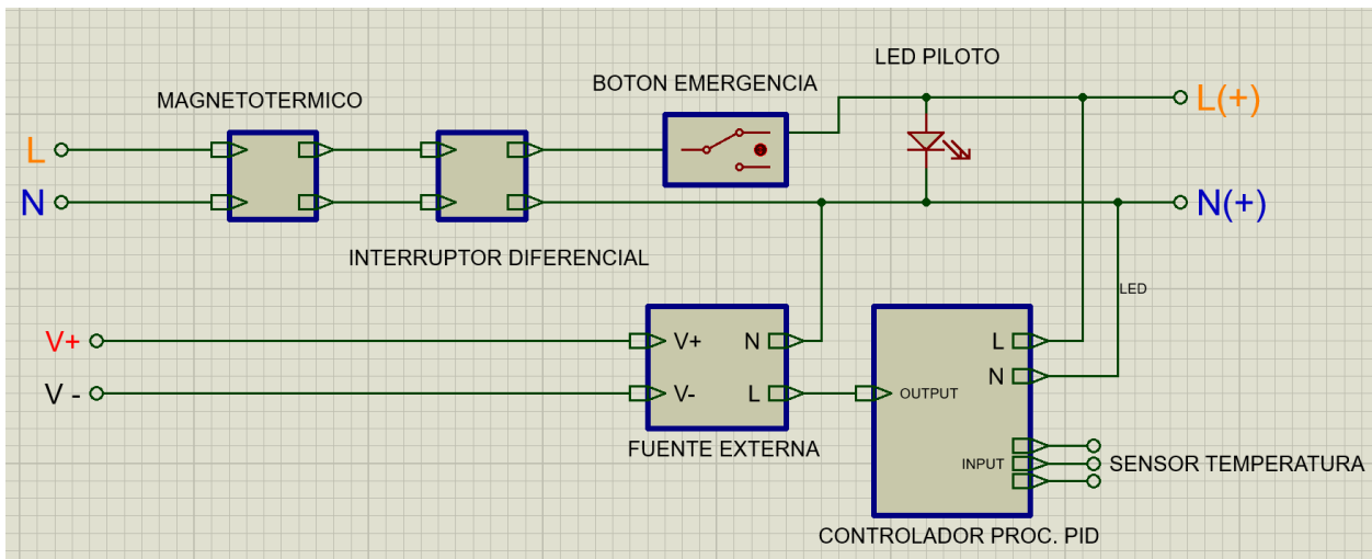
Figura 3.17 Elementos eléctricos que interactúan con corriente alterna.
