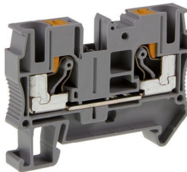
Figura 3.14 Borne de paso de carril DIN. [46]
