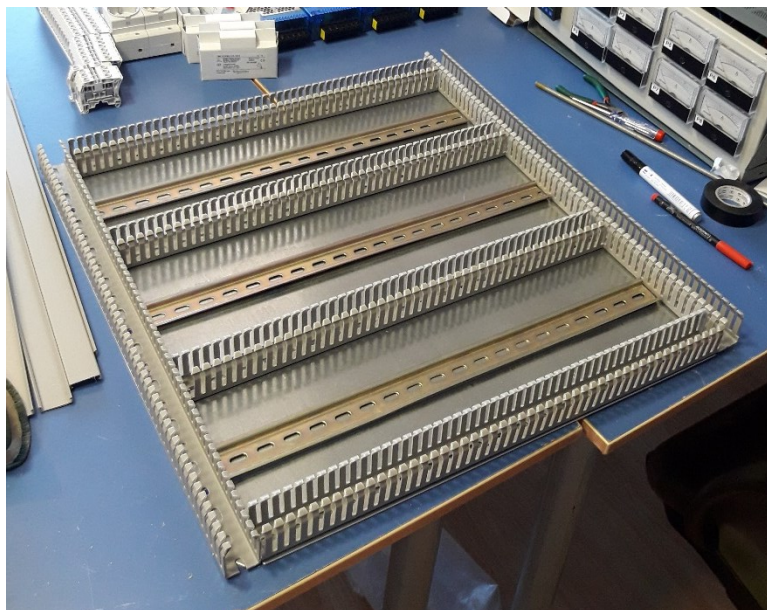
Figura 3.26 Colocación de carriles DIN sobre la plancha.
