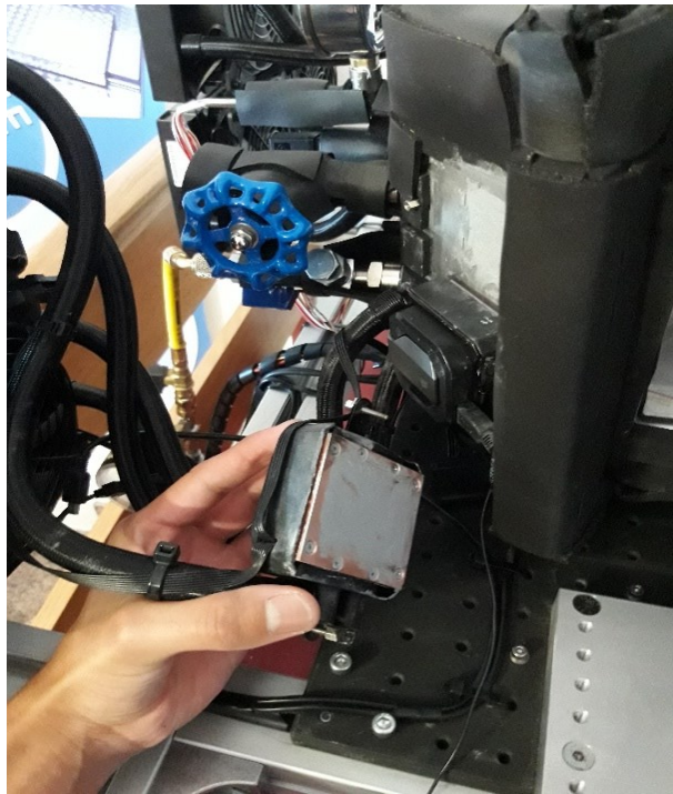
Figura 3.39 Desmontaje de la bomba para cambiar las células Peltier.
