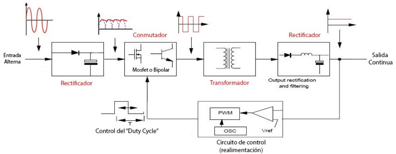
Figura 2.3 Esquema de una fuente de alimentación conmutada. [12]
