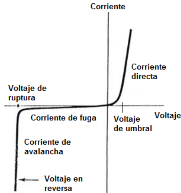
Figura 2.12 Curva característica del diodo real. [20]
