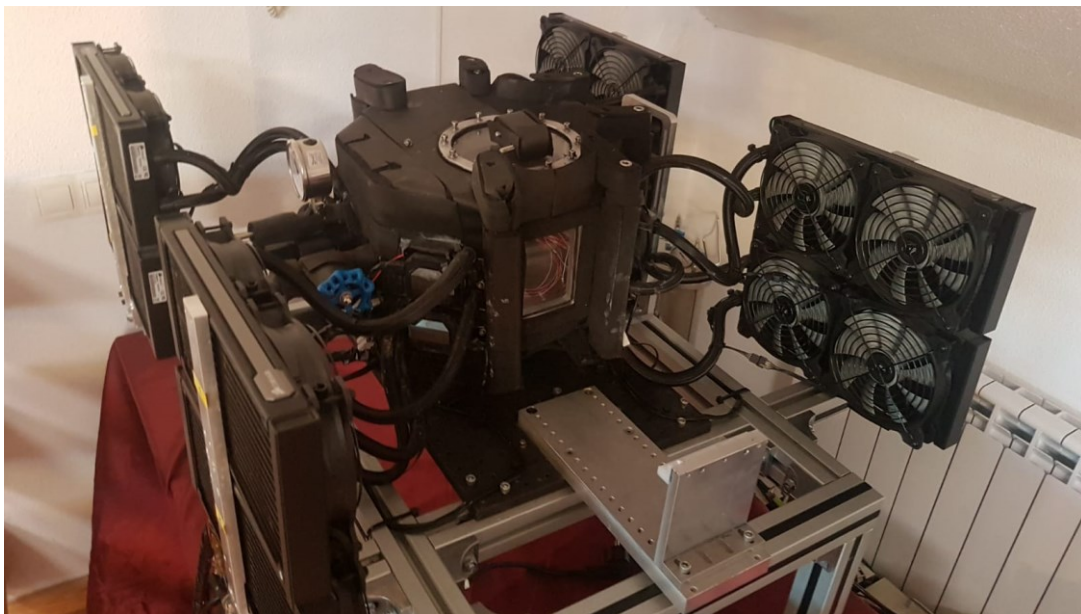
Figura 4.6 Vista 1 de la cámara climática ordenada.
