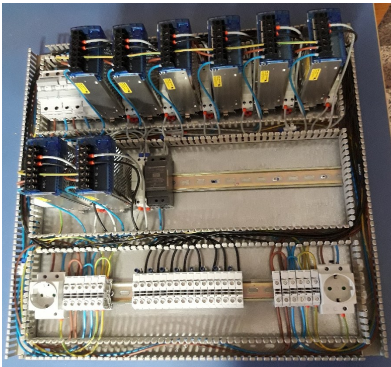
Figura 3.33 Conexión de todas las señales en la plancha.
