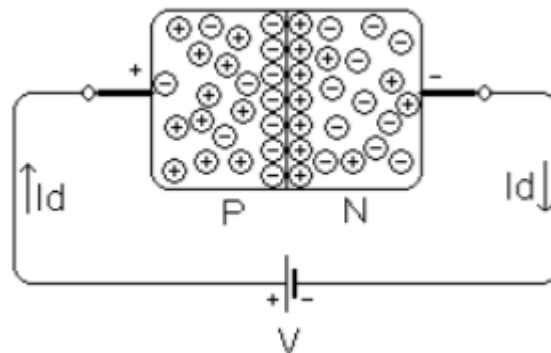
Figura 2.11 Polarización directa. [18]
