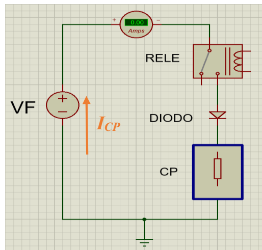
Figura 3.3 Circuito principal.
