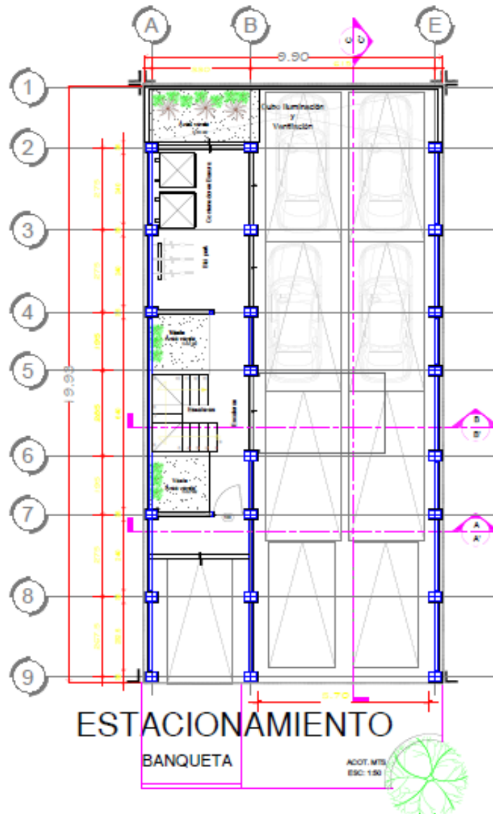
Figura 5. 2. Dibujo arquitectónico de planta del inmueble.
