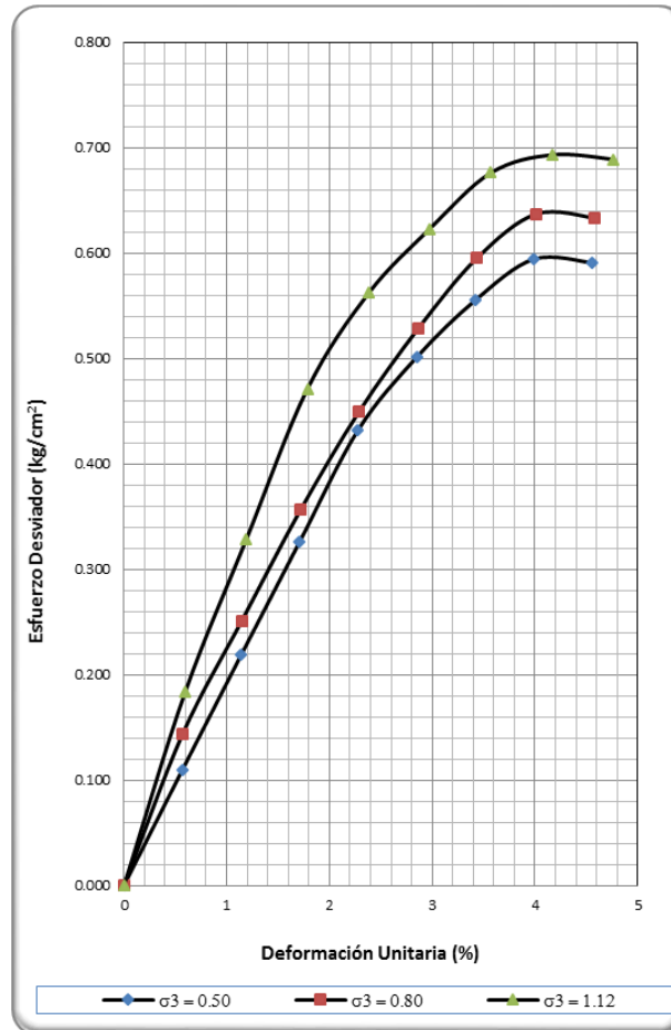
Grafica 3.4. Curvas Esfuerzo-deformación
