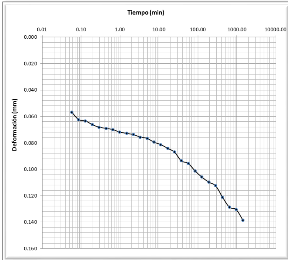
Grafica 3.3. Curva de consolidación.
