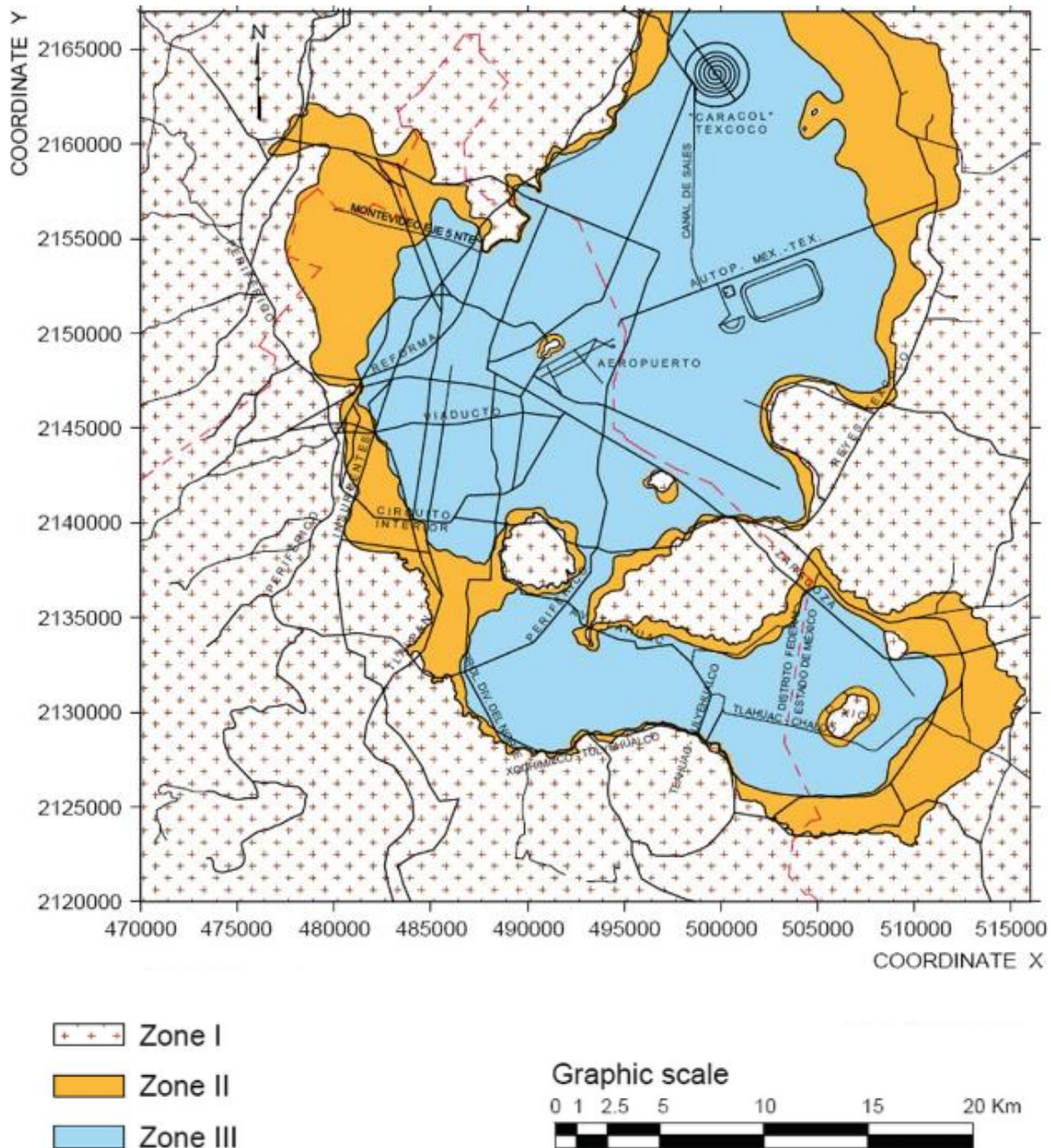
Figura 2.3 Zonificación Geotécnica de la Ciudad de México (Auvinet, G., et al, 2016).
