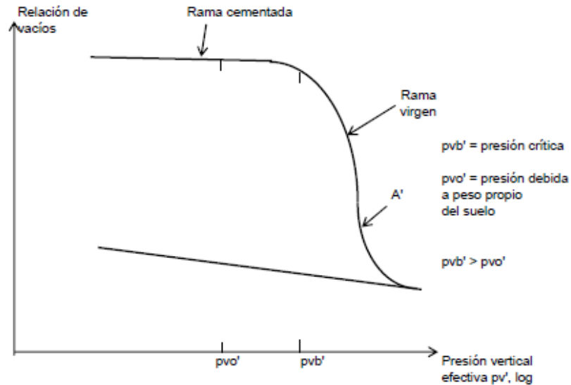
Gráfica 4.2. Ejemplo ilustrativo de Curva de compresibilidad de una arcilla sensitiva.
