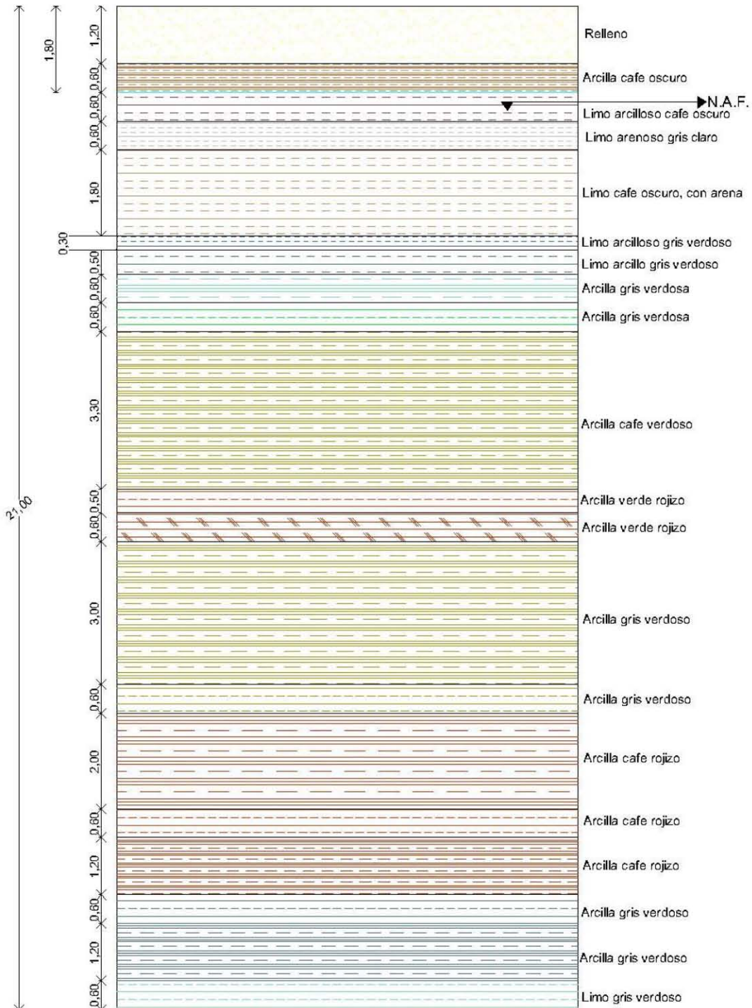
Figura 3.1 Estratigrafía de la zona de análisis.
