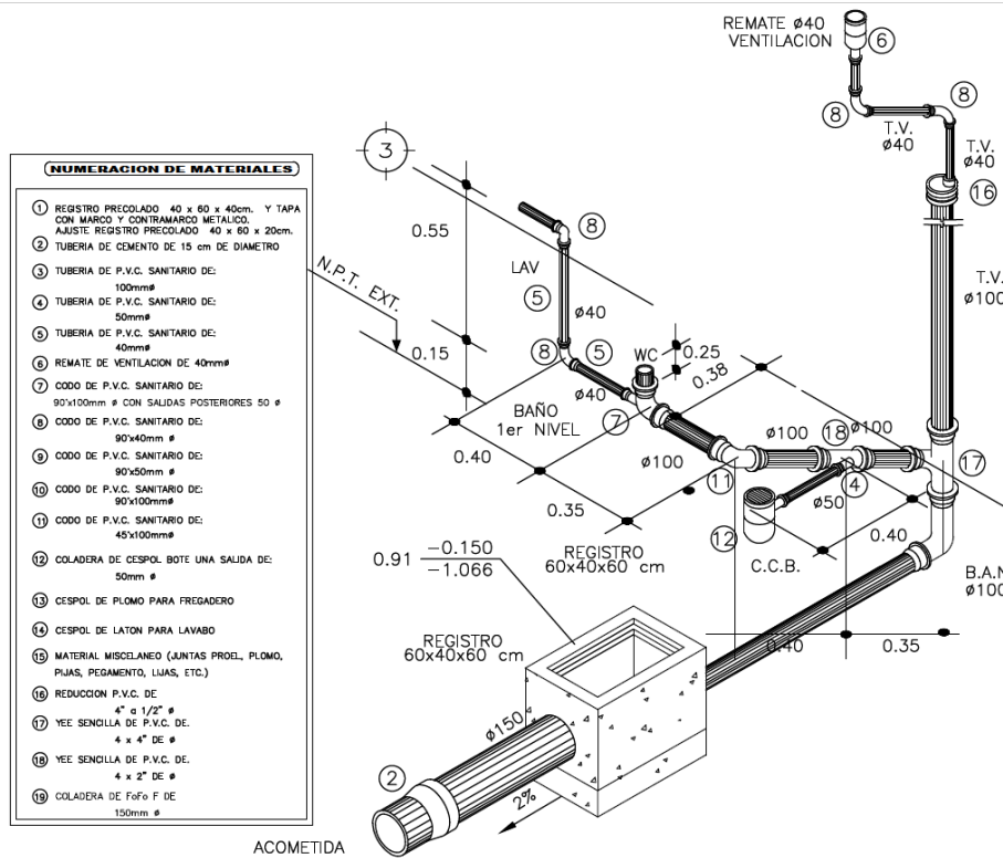
Detalle 2, Isométrico instalación sanitaria y despiece. Fuente: propia
