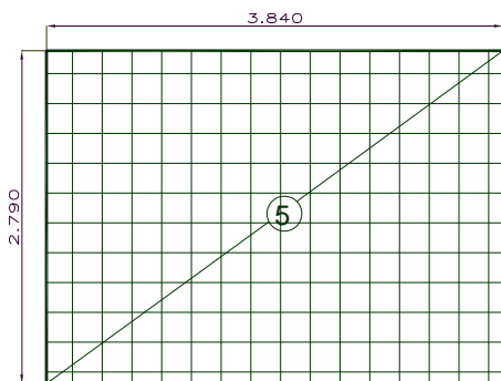
MALLAS DE ACERO 6 x 6 - 8/8 DE 3.840 x 2.790 M
