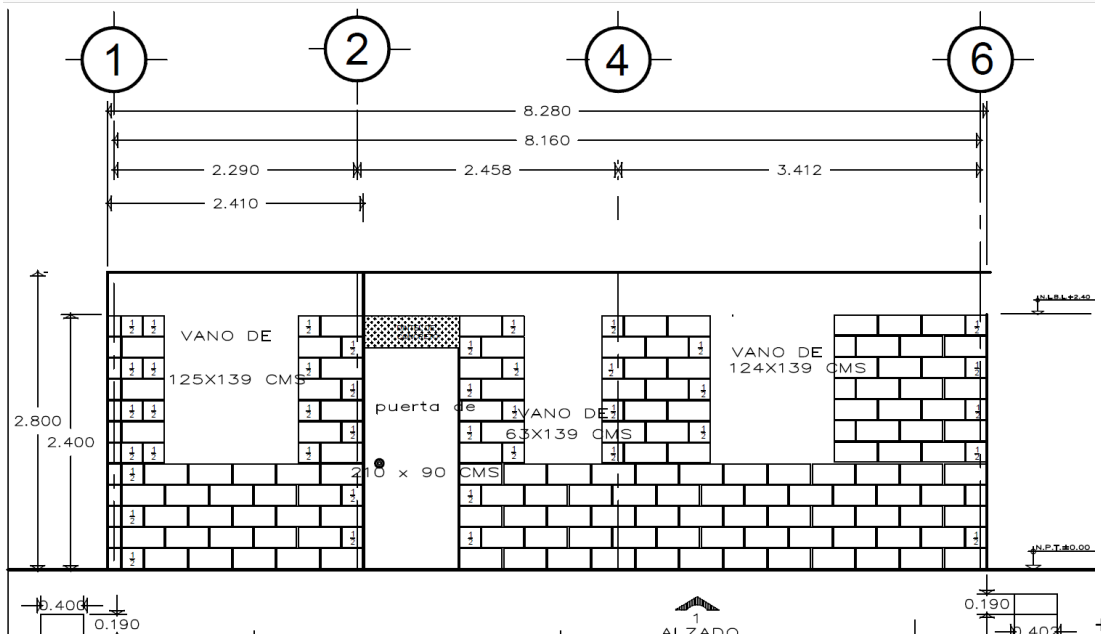
Detalle 1, Despiece de muros de block. Fuente: propia
