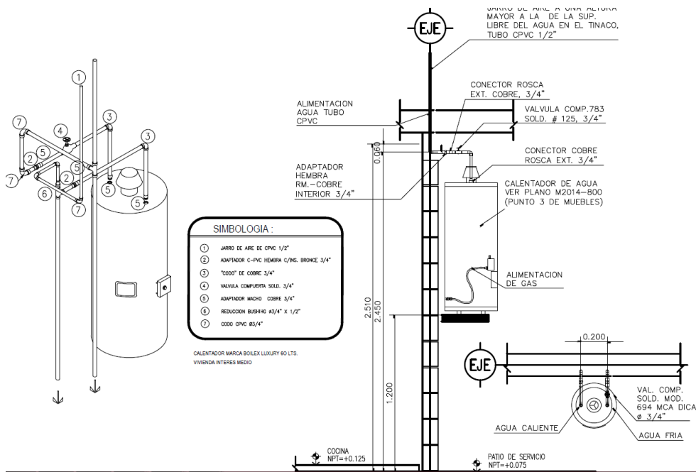
Detalle 5, Isométrico detalle hidráulico. Fuente: propia
