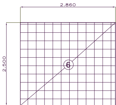
MALLAS DE ACERO 6 x 6 - 8/8 DE 2.860 x 2.500 M
