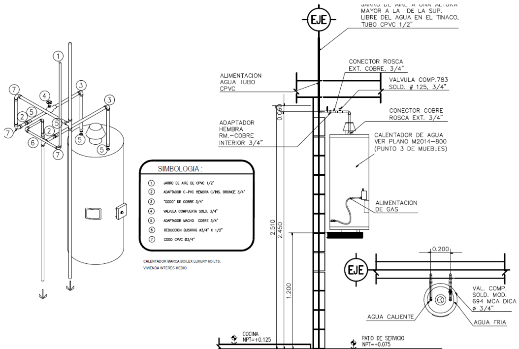
Detalle 3, Isométrico, alzado y planta de detalle hidráulico. Fuente: propia
