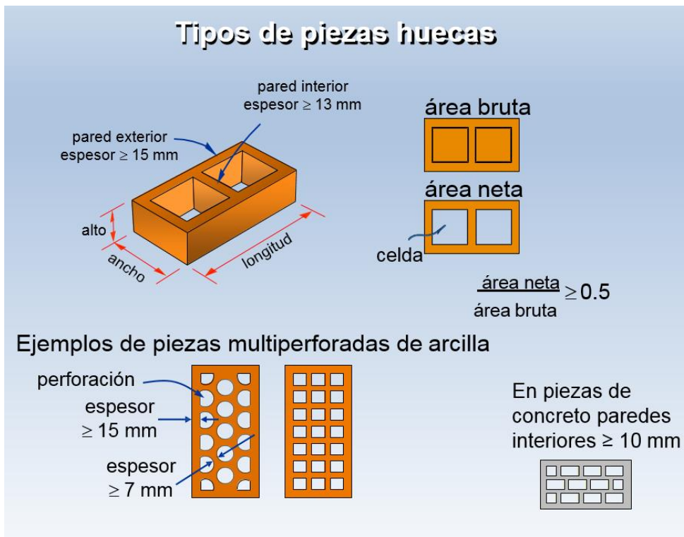
Figura 3, Propiedades de los materiales para mampostería. Álvaro Pérez Gómez, Leonardo Flores Corona Fuente: SMIE, Sociedad Mexicana de Ingeniería Estructural, A.C
