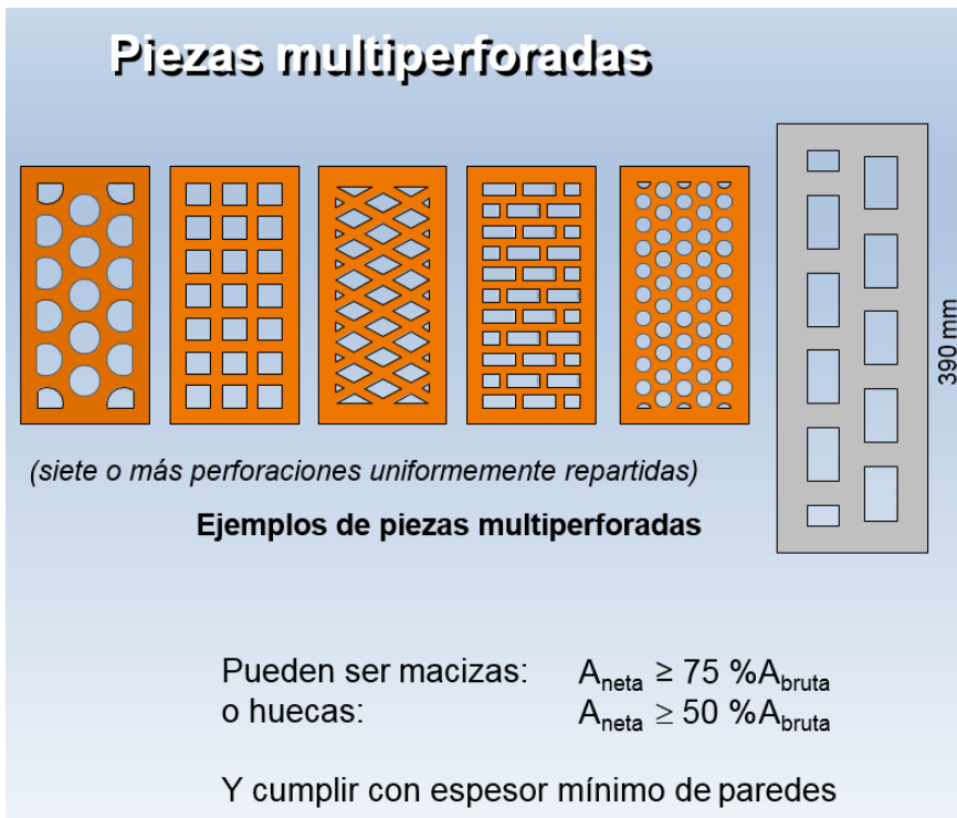
Figura 2, Propiedades de los materiales para mampostería. Álvaro Pérez Gómez, Leonardo Flores Corona Fuente: SMIE, Sociedad Mexicana de Ingeniería Estructural, A.C
