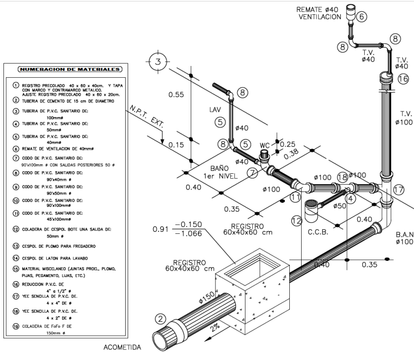
Detalle 4, Isométrico instalación sanitaria y despiece. Fuente: propia
