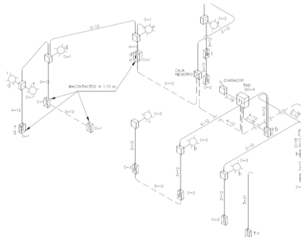
Detalle 4, Isométrico, detalle eléctrico para cuantificación de generador. Fuente: propia
