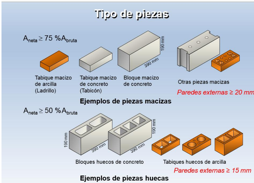
Figura 1, Propiedades de los materiales para mampostería. Álvaro Pérez Gómez, Leonardo Flores Corona Fuente: SMIE, Sociedad Mexicana de Ingeniería Estructural, A.C
