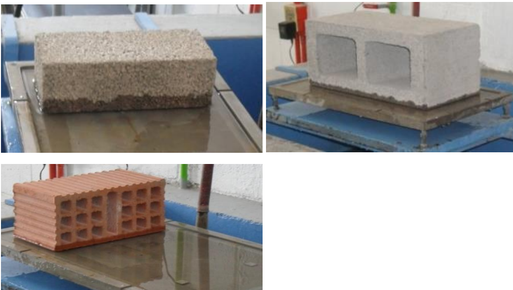
Foto 6: Pruebas de absorción, Fuente: Industrial Bloquera Mexicana, 2018
