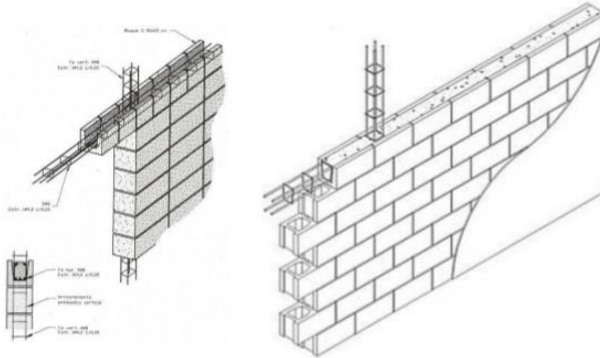
Figura 4, Propiedades de los materiales para mampostería. Álvaro Pérez Gómez, Leonardo Flores Corona Fuente: SMIE, Sociedad Mexicana de Ingeniería Estructural, A.C
