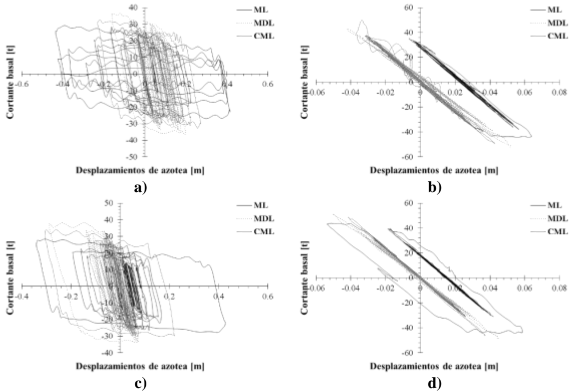
Figura C.24. Comportamiento sísmico de marcos de concreto reforzado de 5 niveles empleando el registro LI33SIM-02 en la dirección EW diseñadas con: a) RCDF-1977 y b) RCDF-2004 (DDF, 1977a y GDF, 2004a) y en la dirección NS diseñadas con: c) RCDF-1977 y d) RCDF-2004 (DDF, 1977a y GDF, 2004a)
