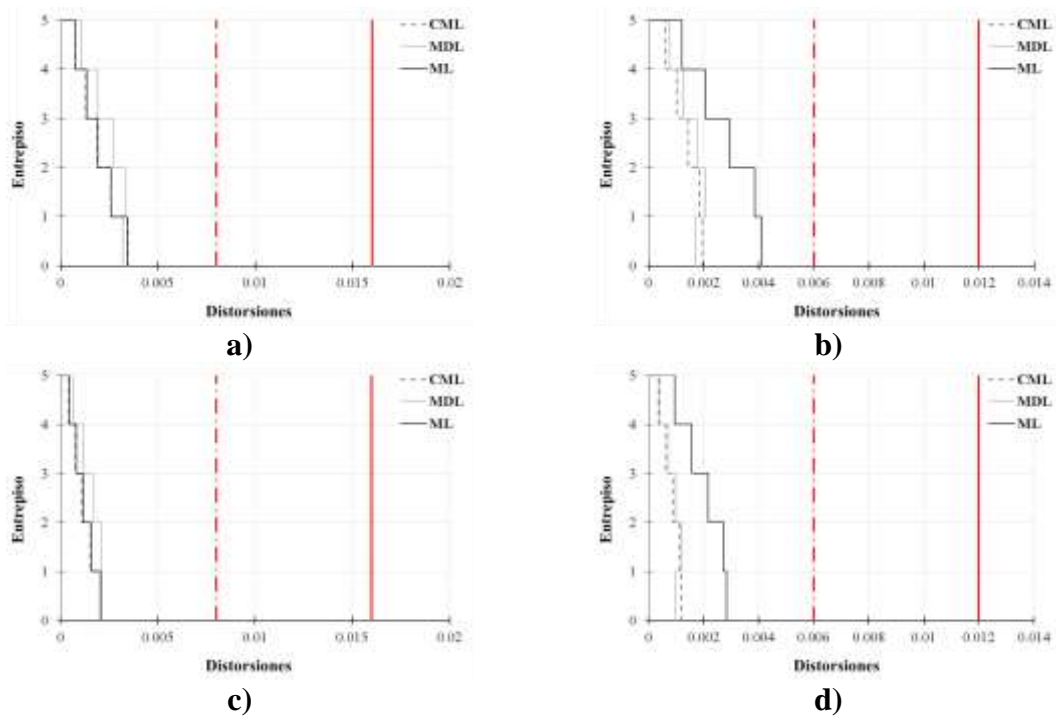
Figura D.21. Distorsiones de entrepiso para MCR de 5 niveles para la estación SXVI para el sismo de 1985 en la dirección EW: a) RCDF-1977 (DDF, 1977) y b) RCDF-2004 (GDF, 2004) y en la dirección NS: c) RCDF-1977 (DDF, 1977) y d) RCDF-2004 (GDF, 2004).
