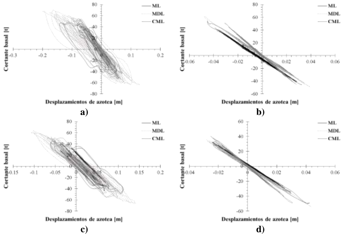
Figura C.33. Comportamiento sísmico de marcos de concreto reforzado de 7 niveles empleando el registro IB22SIM-01 en la dirección EW diseñadas con: a) RCDF-1977 y b) RCDF-2004 (DDF, 1977a y GDF, 2004a) y en la dirección NS diseñadas con: c) RCDF-1977 y d) RCDF-2004 (DDF, 1977a y GDF, 2004a)
