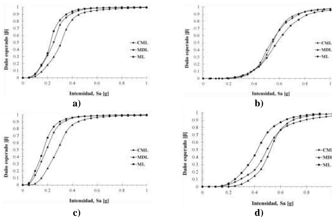
Figura 40. Curvas de vulnerabilidad para marcos de concreto reforzado de 5 niveles diseñados con: a) RCDF-1977 y b) RCDF-2004 (DDF, 1977a y GDF, 2004a) y marcos de concreto reforzado de 7 niveles diseñados con: c) RCDF-1977 y d) RCDF-2004 (DDF, 1977a y GDF, 2004a)
