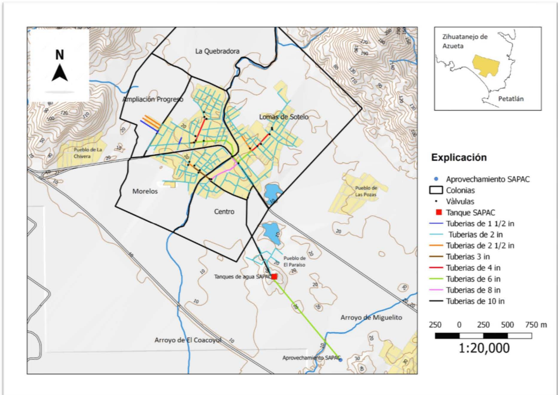
Figura 3.10. Infraestructura del SAPAC.
