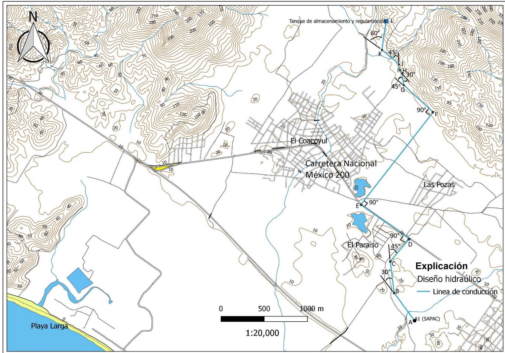
Figura 5.25. Trazo planimétrico de la línea de conducción.
