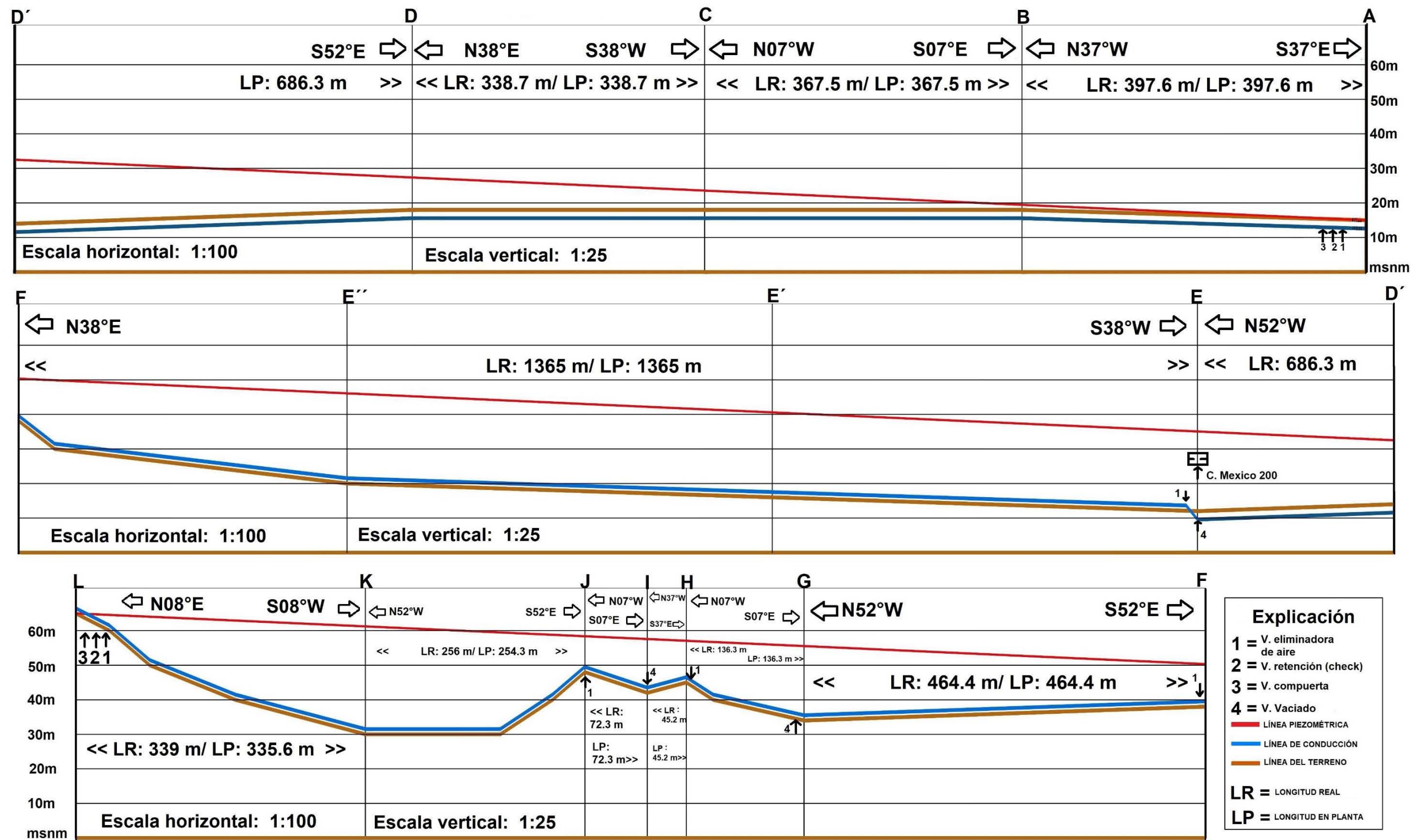
Figura 5.26. Trazo altimétrico de la línea de conducción.
