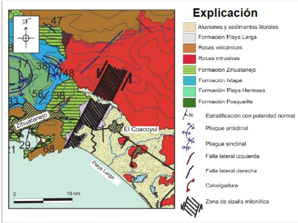
Figura 4.2. Mapa geológico del área de estudio según Martini.
