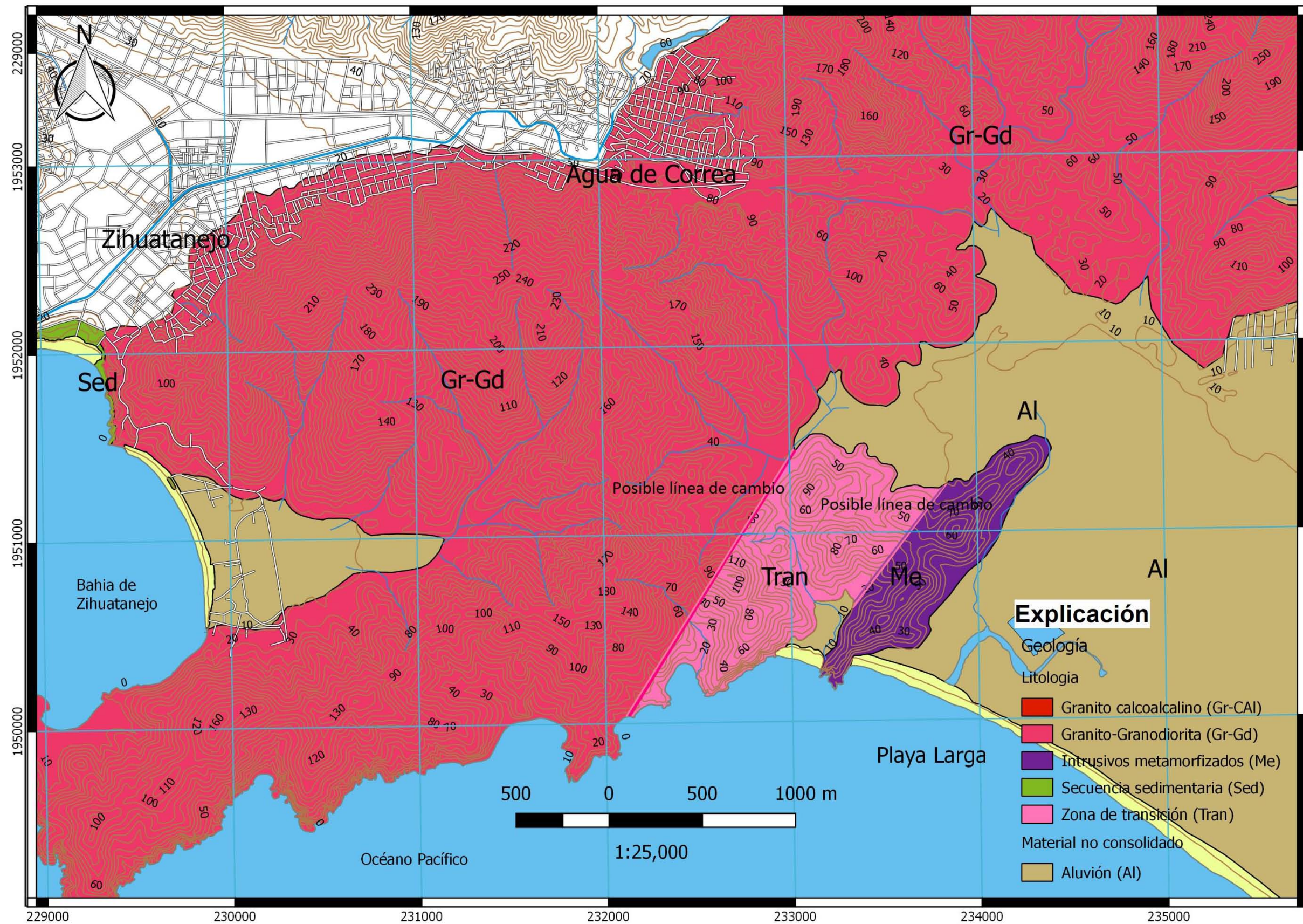
Figura 5.17. Mapa geológico de la zona oeste del área de estudio.
