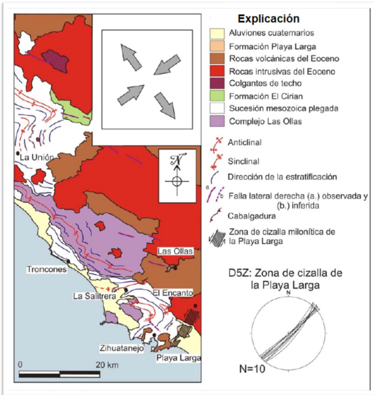
Figura 4.3. Zona de cizalla milonítica de Playa Larga, según Martini.
