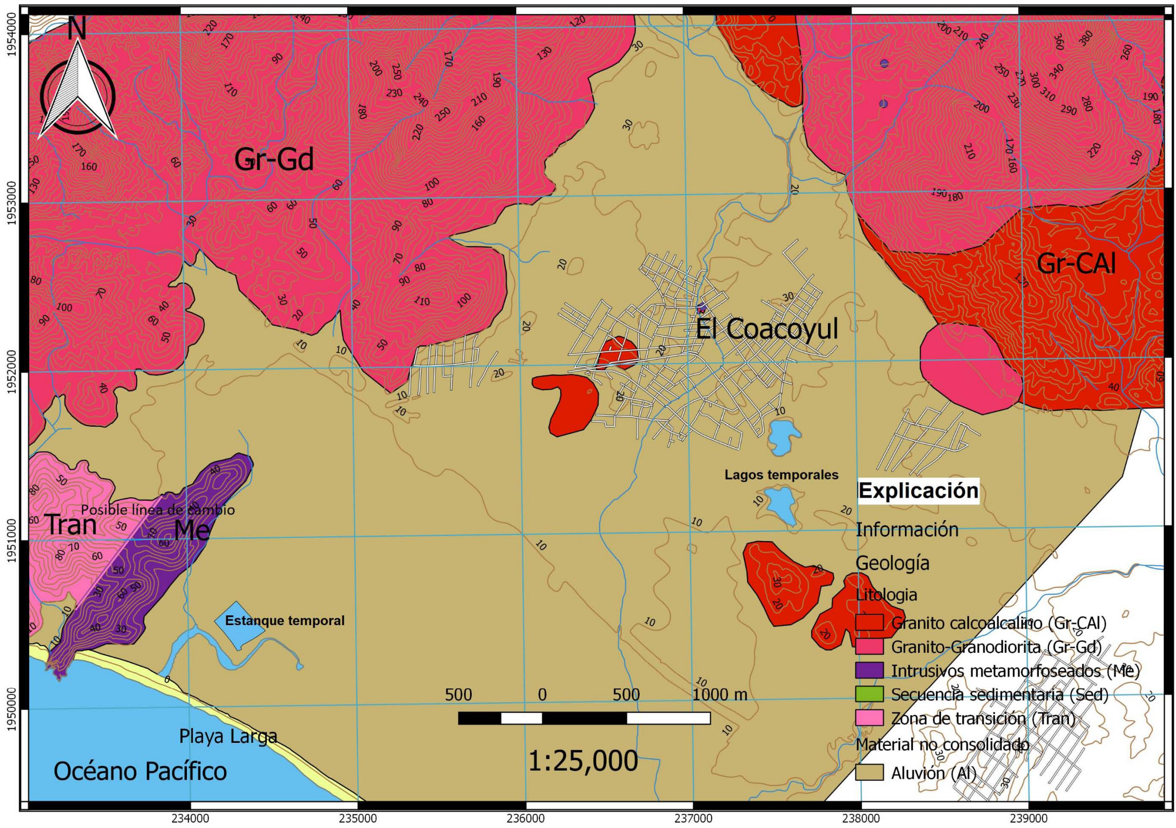
Figura 5.18. Mapa geológico de la zona este del área de estudio.
