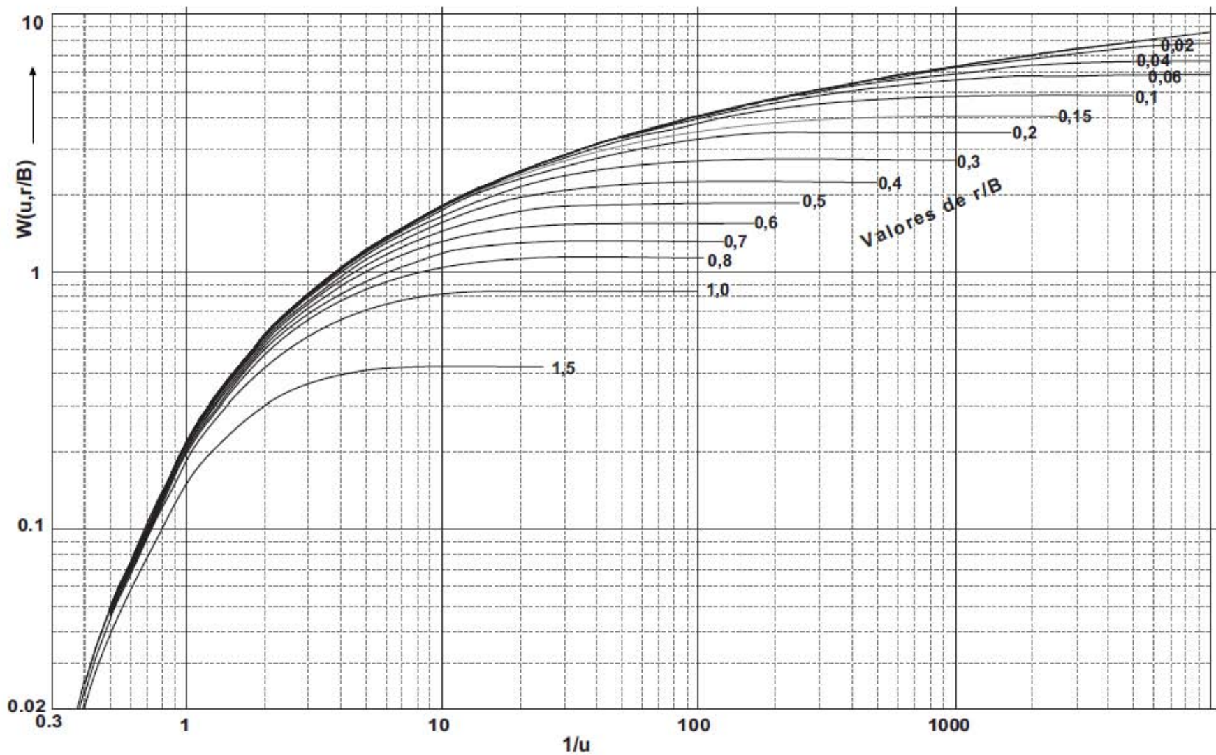
Anexo 4. Gráfico patrón de Walton utilizado en la interpretación de la curva generada por la prueba de bombeo.
