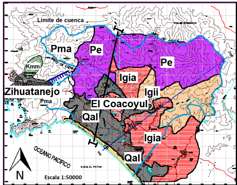
Figura 4.1. Mapa geológico de área de estudio según CONAGUA.
