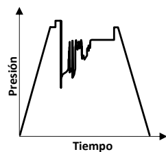
Estrangulador obstruido
