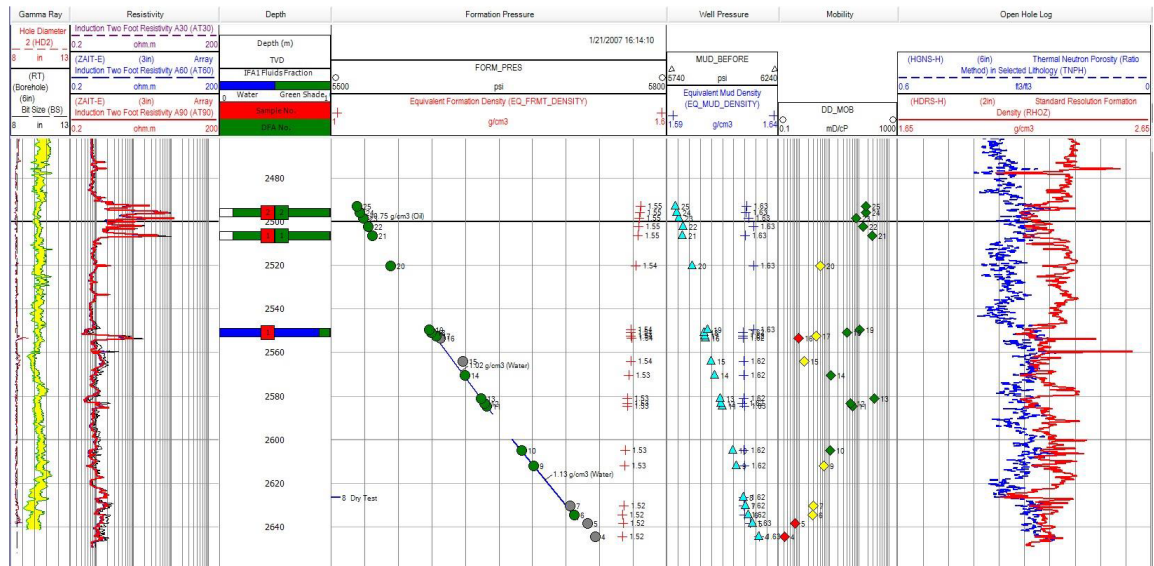
Figura 5.14: Resultados MDT H-4DEL etapa 8.5”. Copyright Schlumberger.
