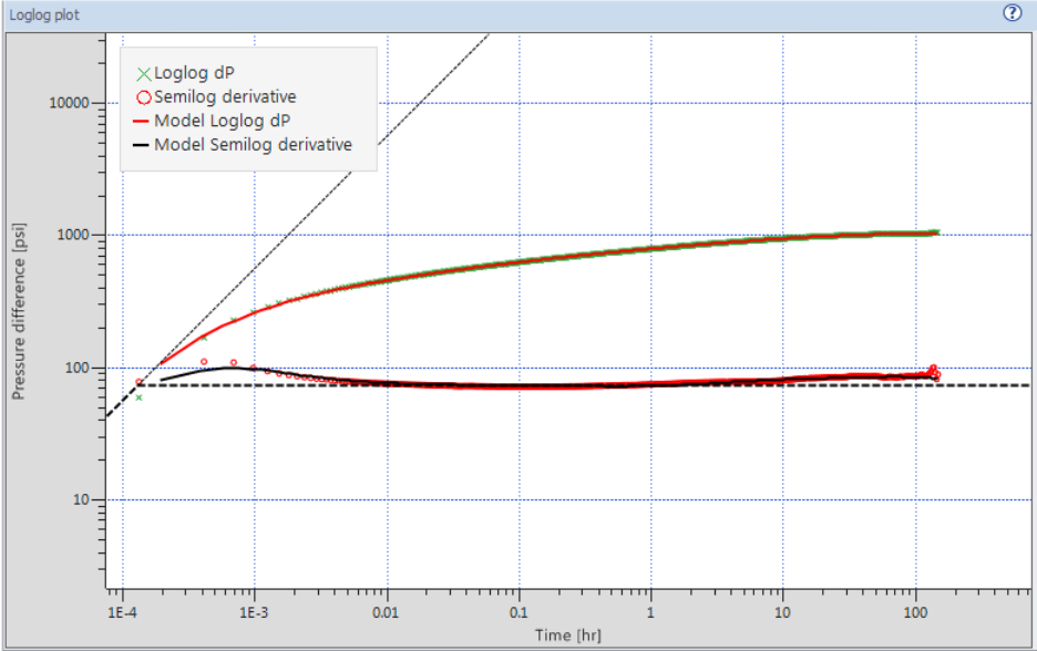
Figura 5.11: Gráfico log-log. La curva negra muestra la derivada del delta P generada a partir del modelo numérico, teniendo en cuenta el efecto del acuñamiento hacia el noreste.
