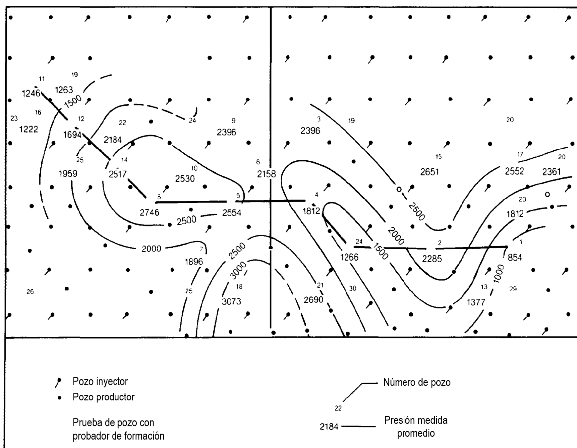
Figura 4.2: Mapa de curvas de contorno en una zona de inyección. Copyright: Western Atlas International, 1987.
