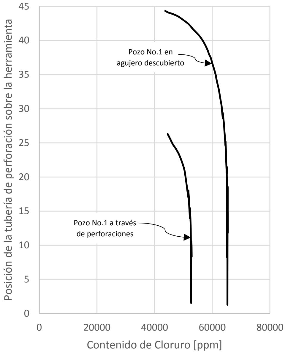
Figura 3.4: Ejemplo de falla de la prueba de formación detrás del revestimiento. Copyright: Black (1956).
