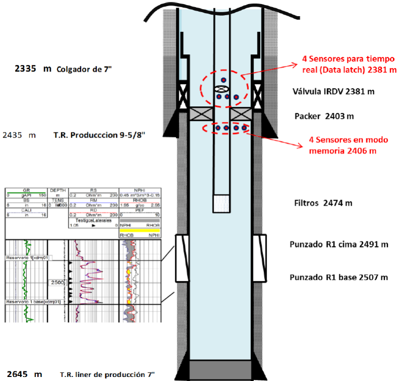
Figura 5.5: Esquema con ubicación de componentes principales del BHA para DST y registros geofísicos del yacimiento punzado.
