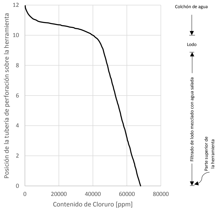
Figura 3.3: Ejemplo del efecto de una inadecuada producción para recuperar agua. Copyright: Black (1956).
