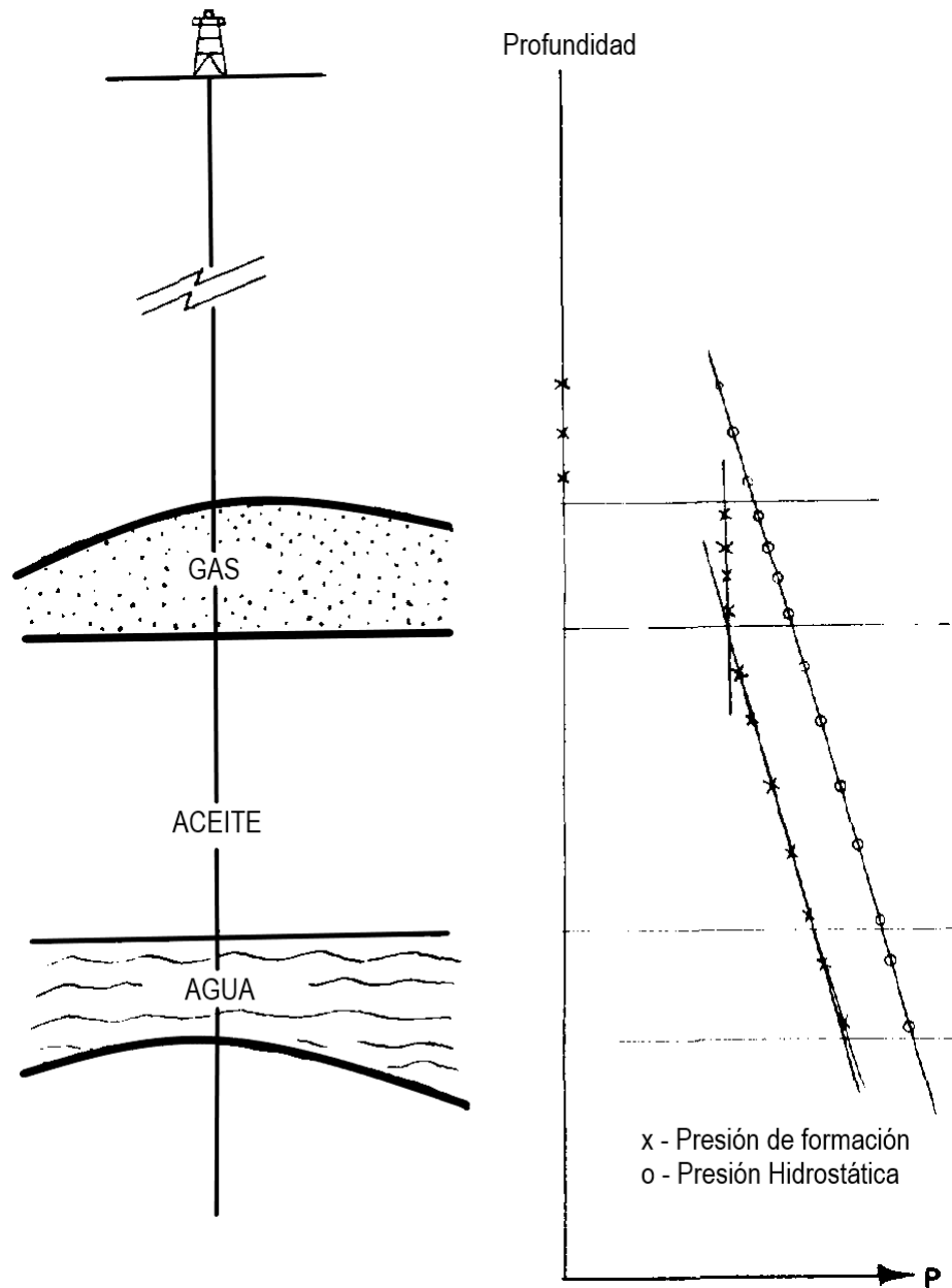
Figura 4.1: Presiones medidas con la herramienta WFT a través del yacimiento. Copyright: Schlumberger Well Services, 1981.
