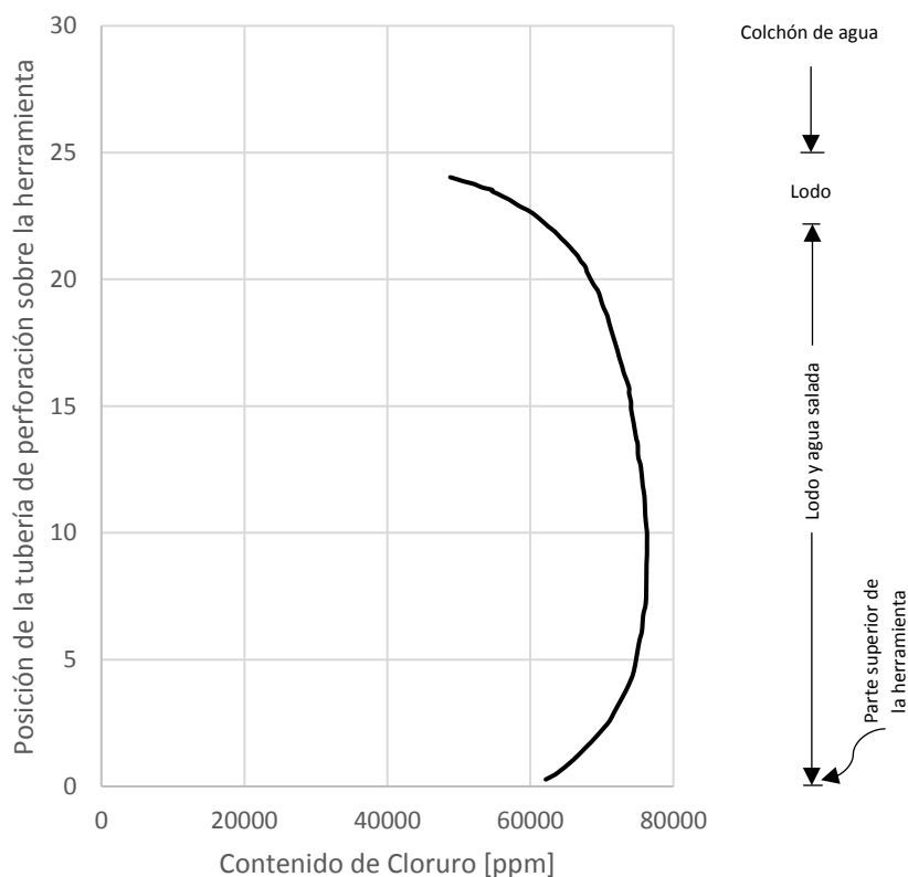
Figura 3.2: Ejemplo del efecto de filtración del empacador en una variación de salinidad contra la profundidad de la columna de agua. Copyright: Black (1956) .
