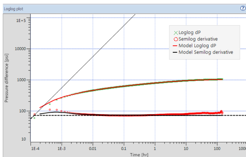
Figura 5.9: Gráfico de diagnóstico con las curvas dp y derivada. En negro y rojo continuo se observan los resultados del modelado analítico (radial infinito).
