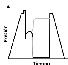
Ancla obstruida
