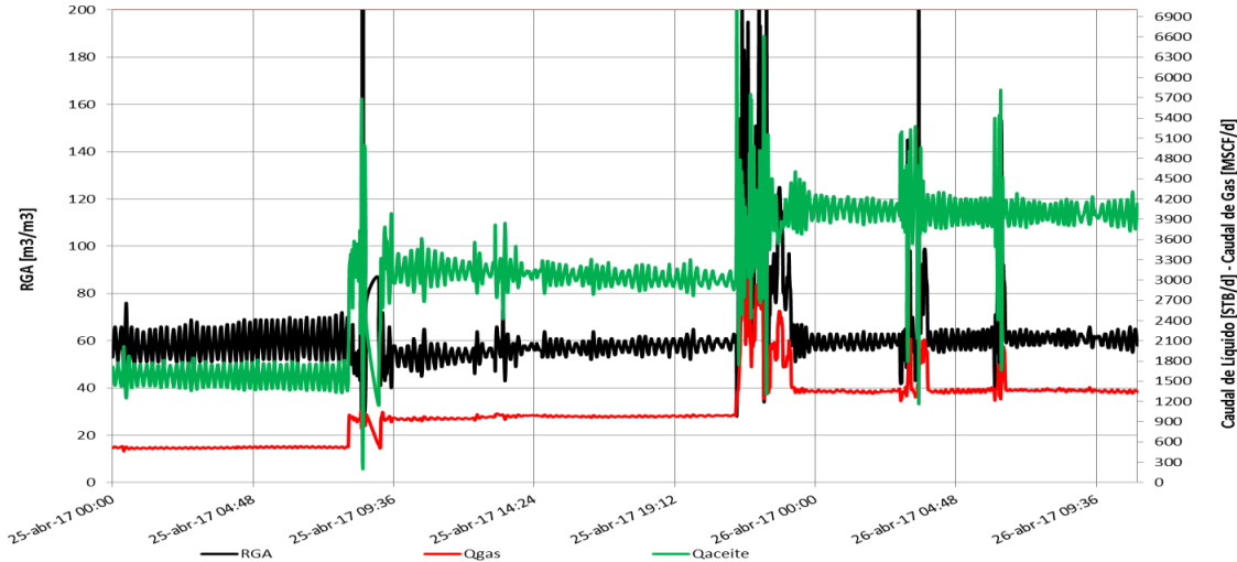
Figura 5.6: Caudales instantáneos durante la etapa de fluencia. Copyright Schlumberger.
