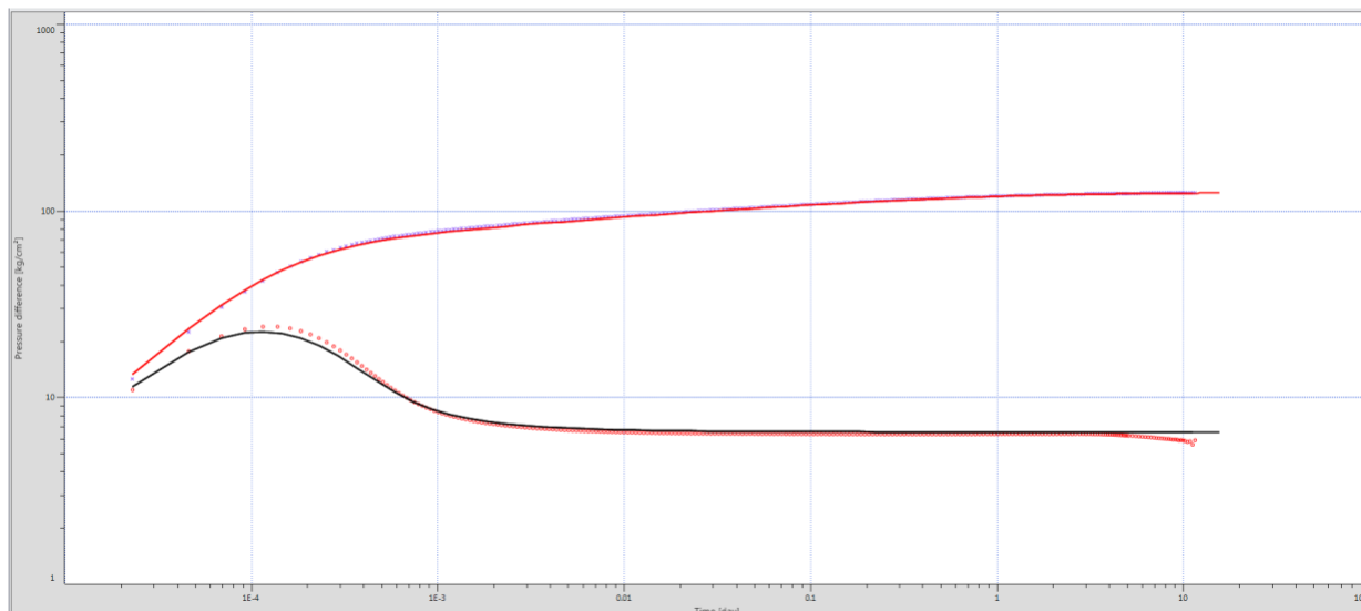
Figura 5.4: Resultado de la extracción del Delta P y su derivada. La curva de puntos rojos es el resultado del modelo y la curva negra es el resultado como si no existiera el acunamiento (flujo radial infinito).
