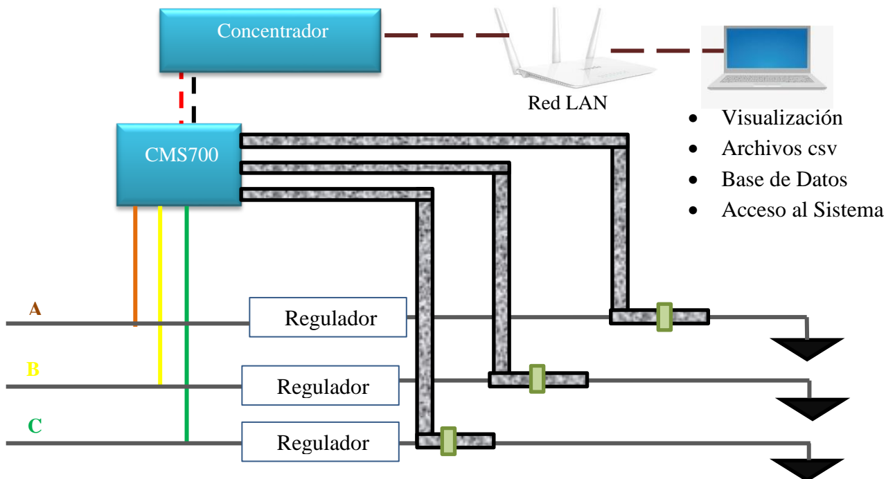
Figura 3.17 Diagrama de implementación del sistema de monitoreo de cargas en circuito de prueba
