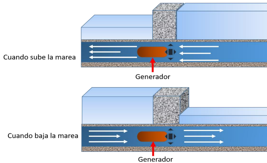
Figura 2.8 Generación mareomotriz.
