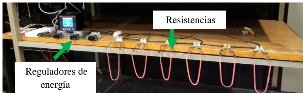
Figura 3.15 Sistema de pruebas
