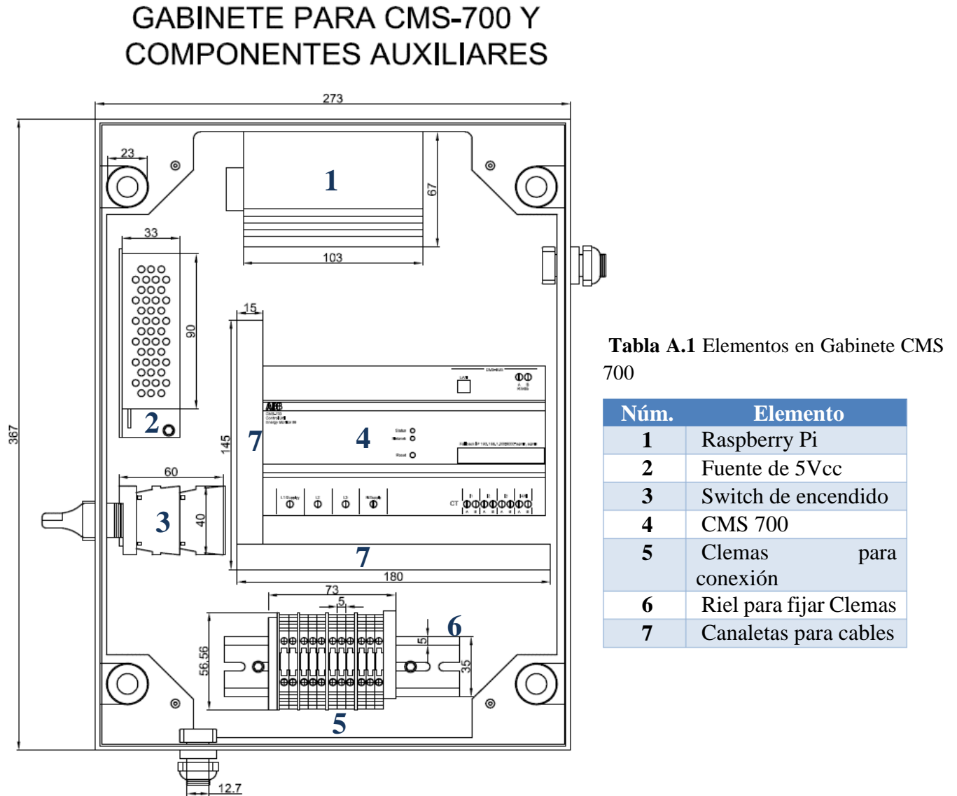
Figura A.1 Configuración de los elementos en el gabinete del concentrador para el CMS700
