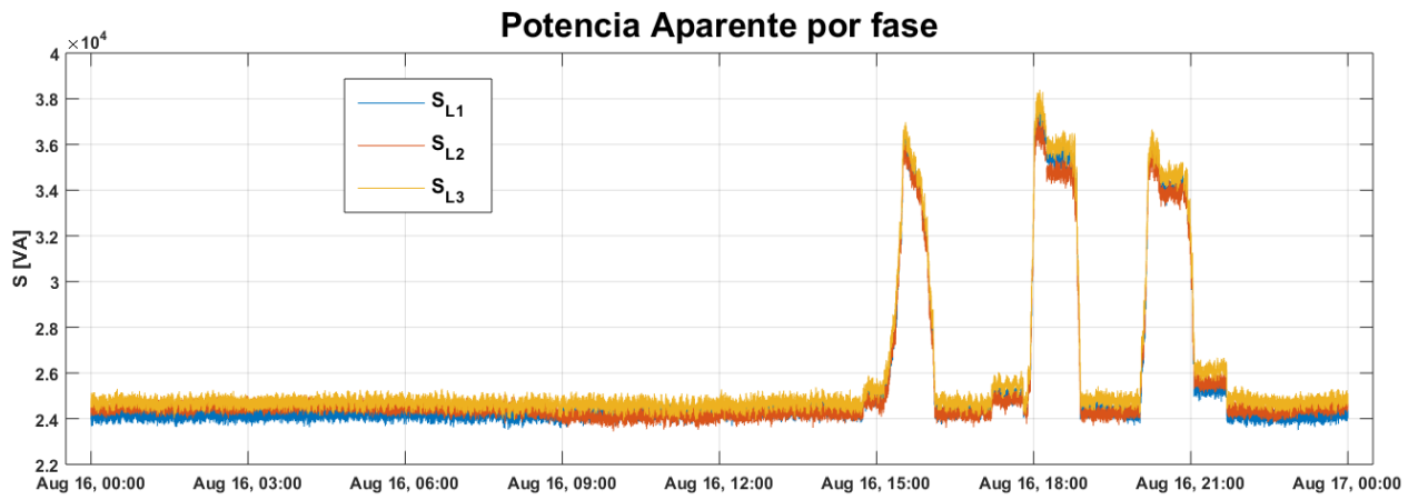
Figura D.3 Gráfica Potencia Aparente
