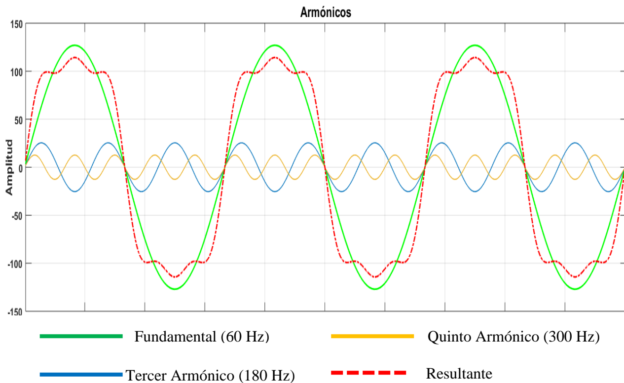
Figura 2.3 Ejemplo de señal con armónicos
