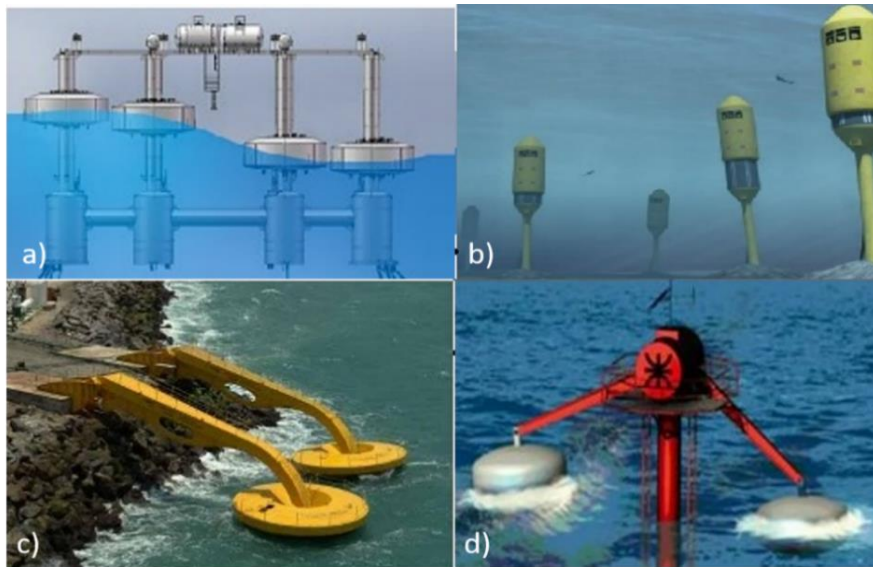
Figura 2.7 a) Captador Energía de olas, b) Sistema con boyas, c) sistema anclado a litoral marino con brazos flotantes, d) Sistema anclado al fondo marino con brazos flotantes
