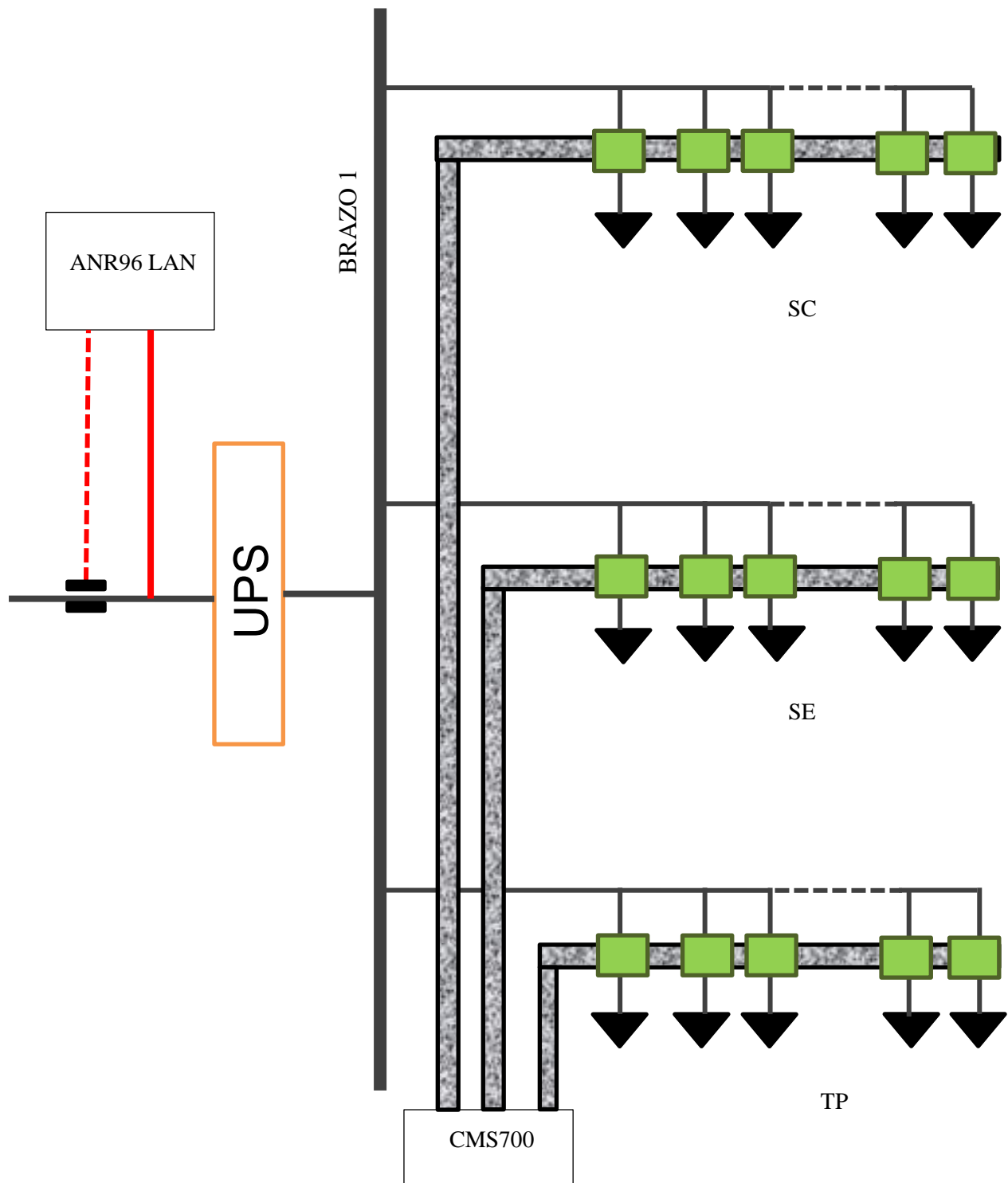
Figura 4.1 Diagrama unifilar del centro de cómputo de DGTC.
