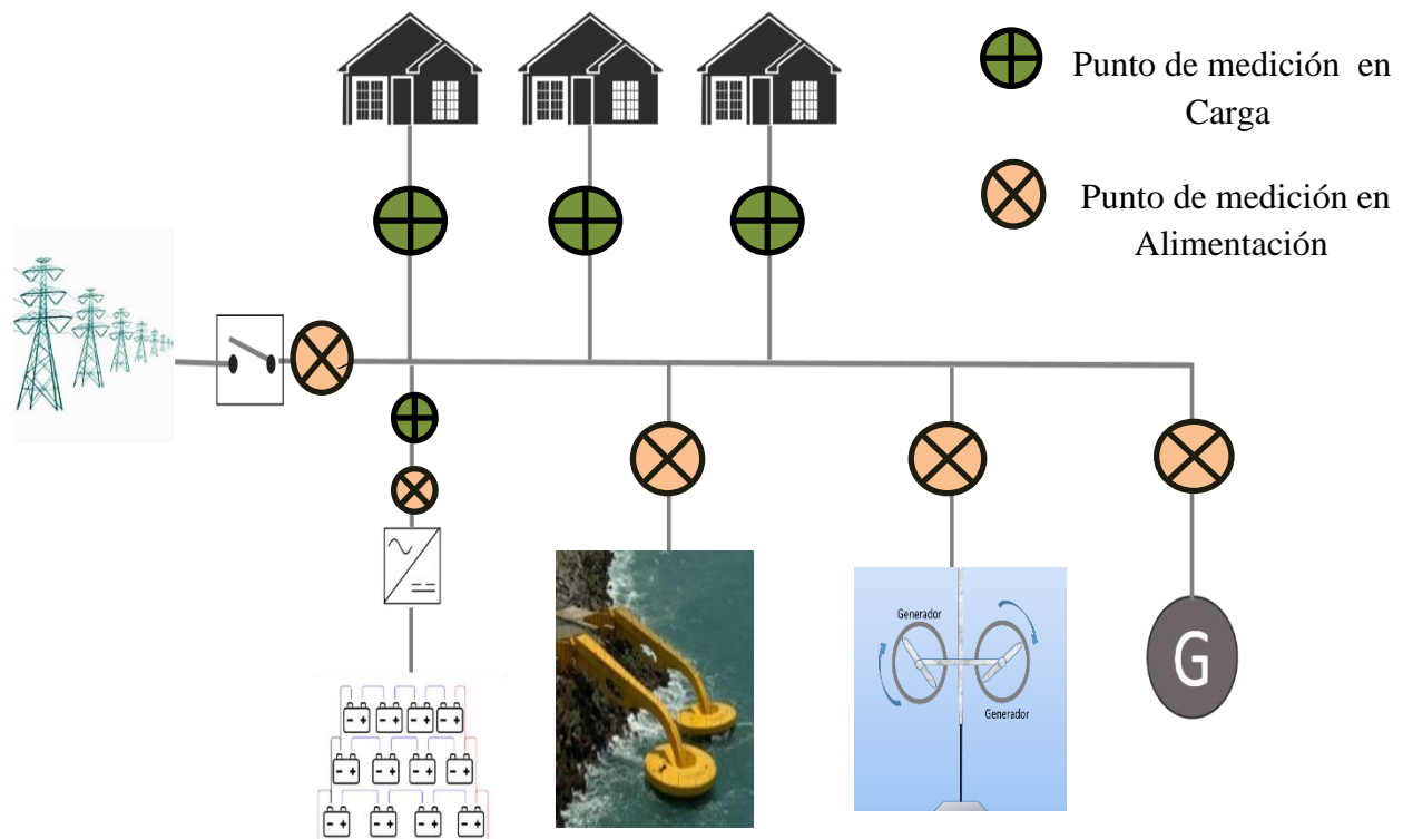
Figura 3.1 Sistema de Monitoreo implementado en una microrred
