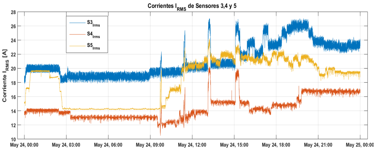
Figura 4.9 Gráfica de corrientes rms de sensores 3, 4 y 5 tomadas el 24 de Mayo de 2018
