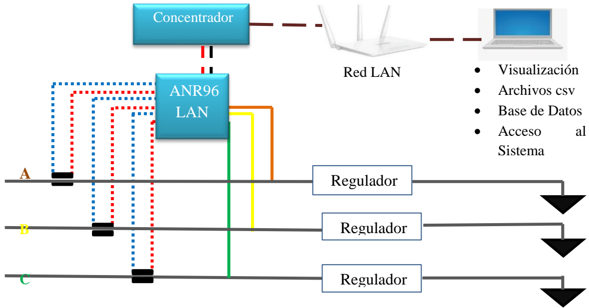
Figura 3.16 Diagrama de implementación del sistema de monitoreo de alimentación en el circuito de prueba
