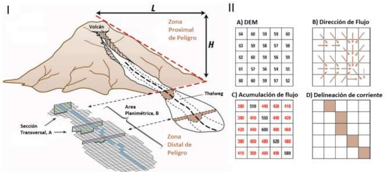
Figura 3.1) Imágenes decriptivas del funcionamiento de Laharz . I) Muestra los elementos que ocupa Laharz para el funcionamiento del software. II) Muestra un ejemplo de los archivos Raster que genera Laharz a partir del Modelo Digital de Elevación, con los cuales se efectúa simulación del lahar. Modificado de Schilling (2014).
