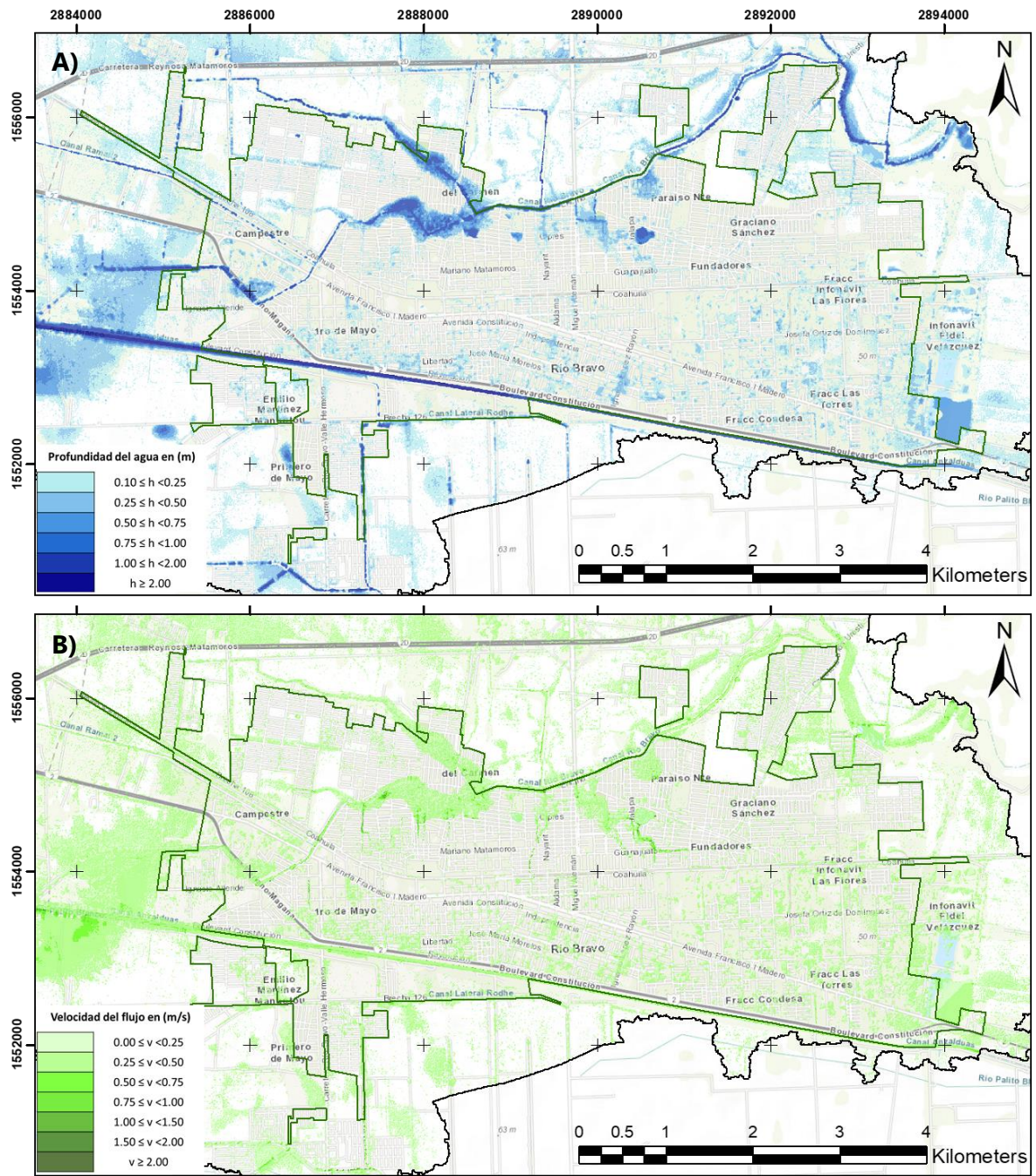
Figura 5-1. Mapa de máximos tirantes (A) y máximas velocidades (B) asociados un periodo de retorno de 2 años para la ciudad de Río Bravo, Tamaulipas.
