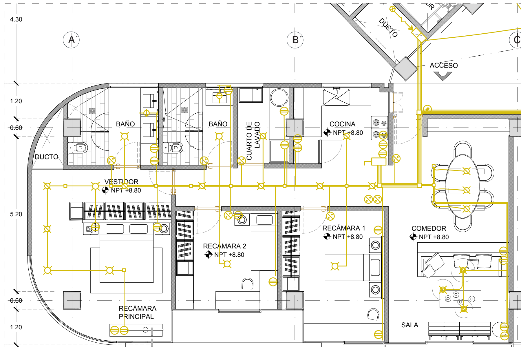
DETALLE PLANTA TIPO
