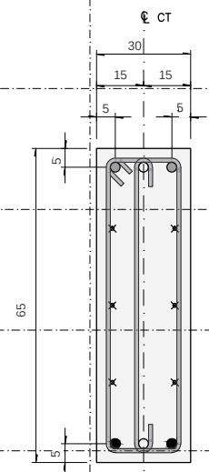
DETALLE DE CONTRABE CT-1 ESC. 1:125
