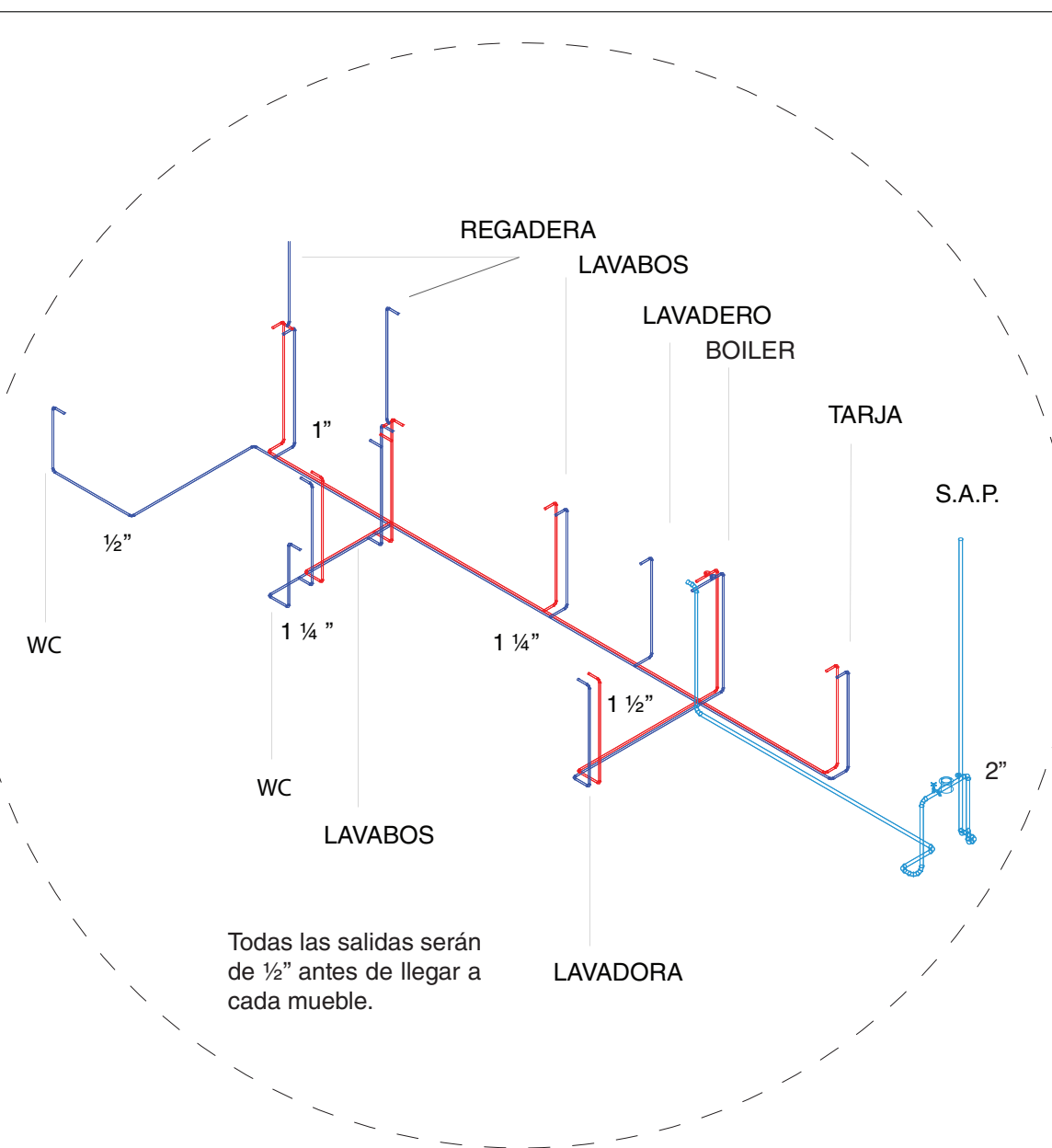
ISOMÉTRICO INSTALACIÓN HIDRÁULICA
