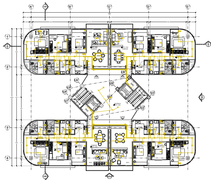
PLANTA TIPO
