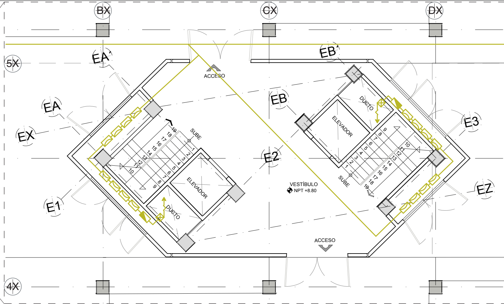
DETALLE PLANTA BAJA
