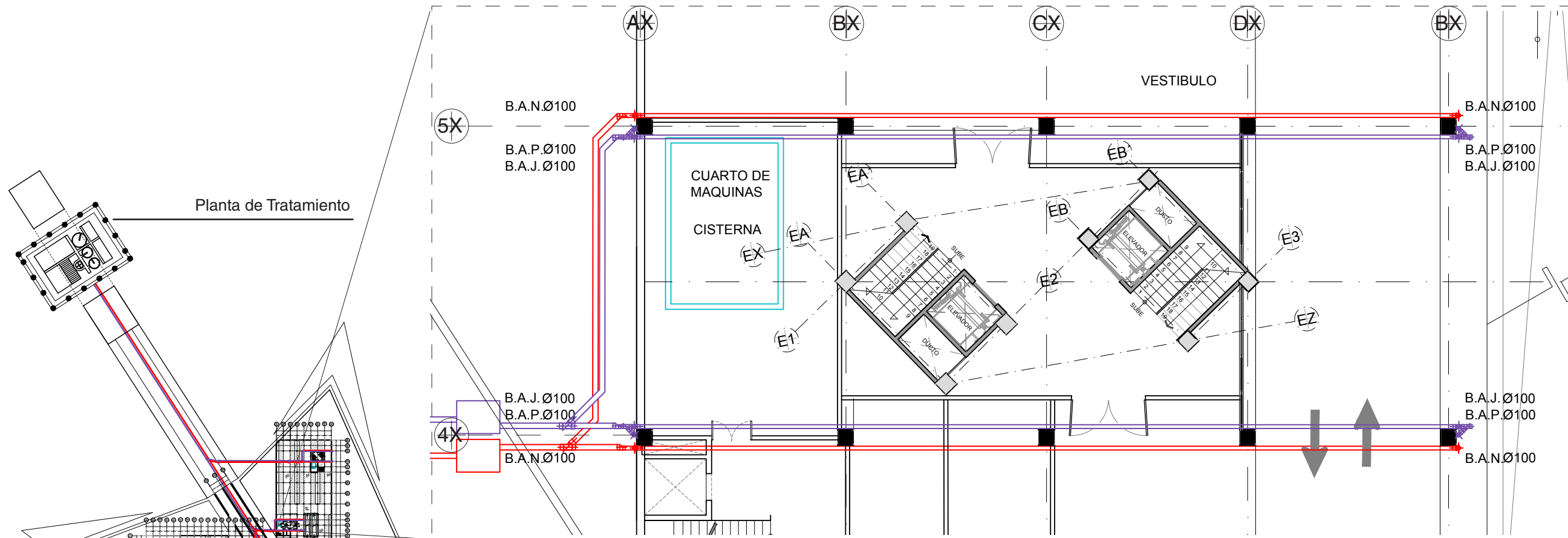
DETALLE PLANTA SÓTANO 1
