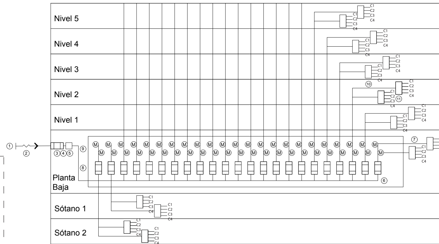
DETALLE CAJA DE CONTROL DE DISTRIBUCION ELÉCTRICA
