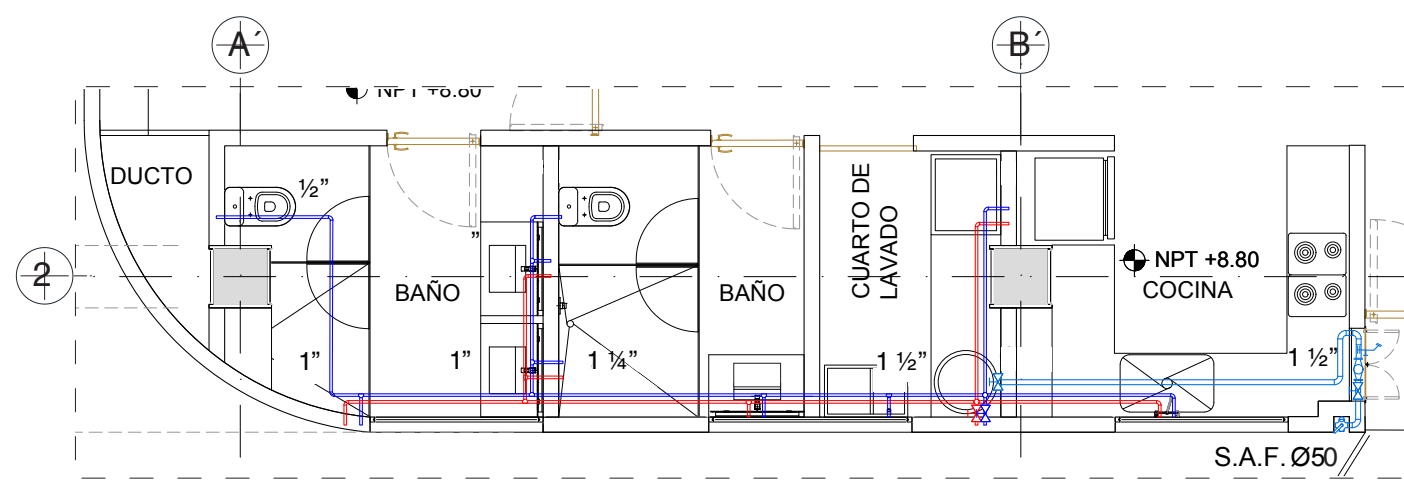
DETALLE DE PLANTA TIPO
