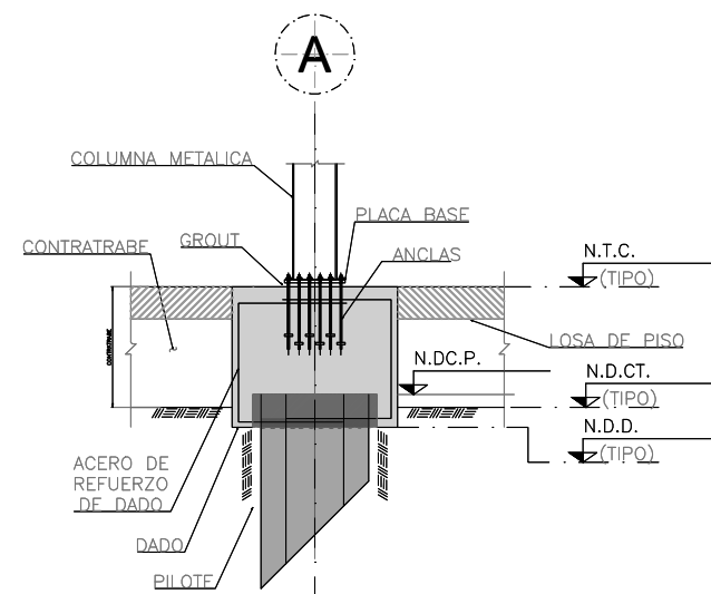
DETALLE TÍPICO UNIÓN
