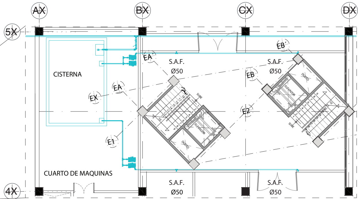
PLANTA SÓTANO 2
