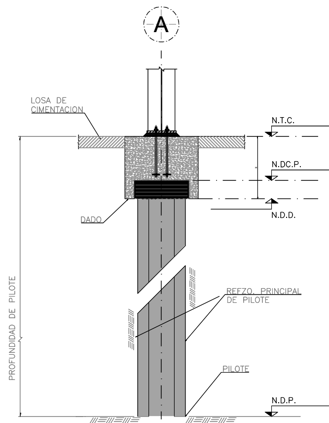
ELEVACIÓN TIPO DE PILOTE
