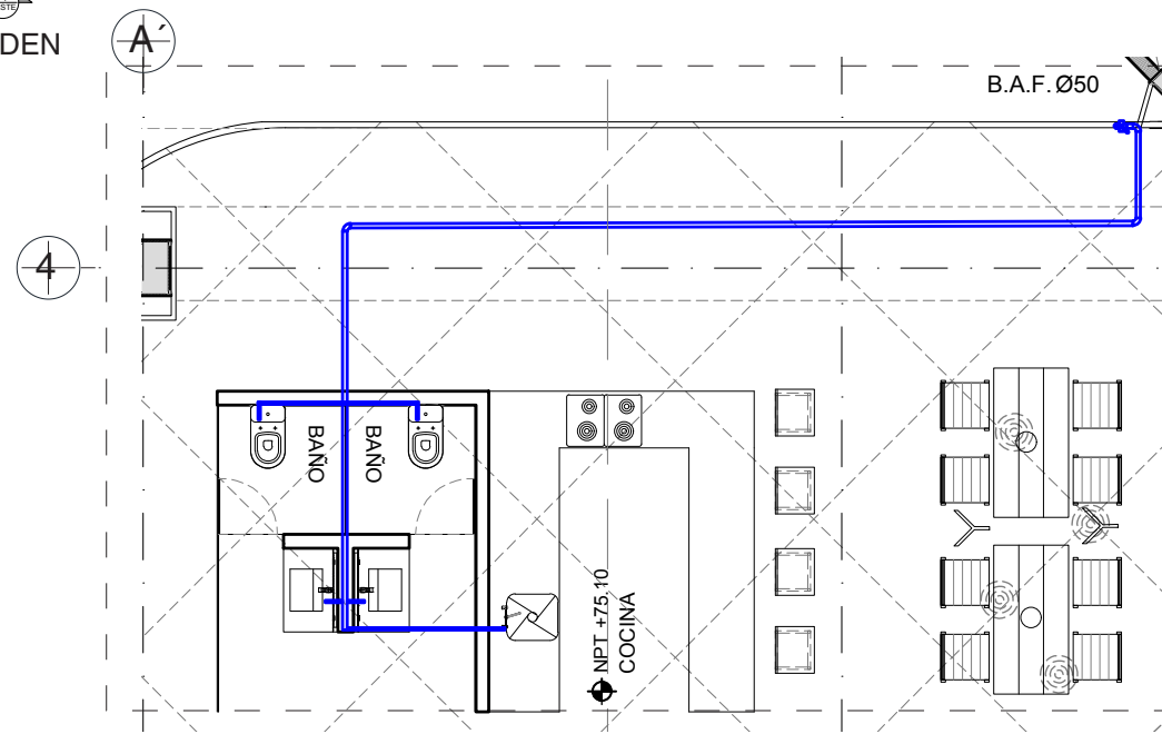
PLANTA DETALLE DE ROOF GARDEN
