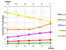
Figura 119. Utilización de procesos en Salamanca para el escenario 1
