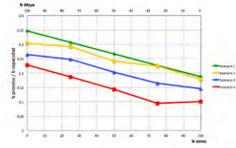
Figura 91. Utilización de coquización en Madero por escenario
