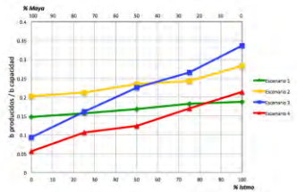
Figura 117. Rendimientos de destilados intermedios en Salamanca por escenario
