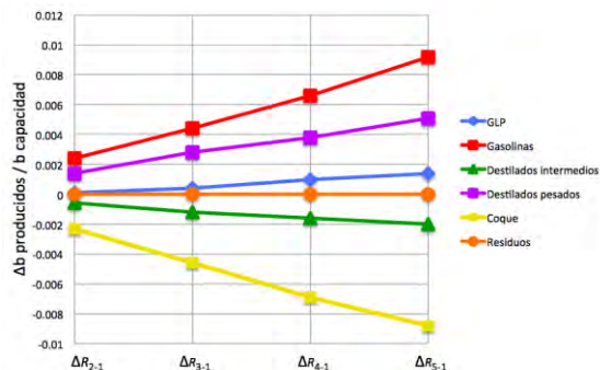
Figura 311. Diferencial de Rendimientos al sustituir crudo Maya por Árabe pesado en Nueva refinera
