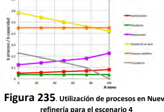
Figura 235. Utilización de procesos en Nueva refinería para el escenario 4
