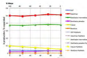
Figura 224. Rendimientos de petrolíferos en Nueva refinería para el escenario 2
