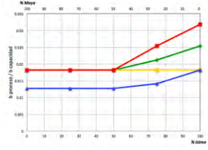
Figura 124. Utilización de Alquilación en Salamanca por escenario
