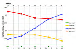
Figura 99. Rendimientos de destilados pesados en Minatitlán por escenario
