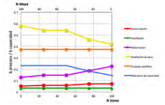
Figura 154. Utilización de procesos en Tula para el escenario 1
