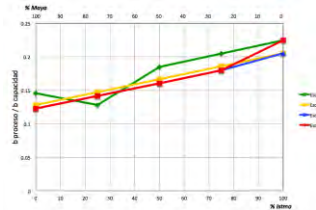
Figura 179. Utilización de Reformación en Salamanca reconfigurada por escenario
