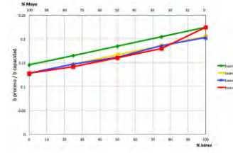
Figura 218. Utilización de Reformación en Tula reconfigurada por escenario
