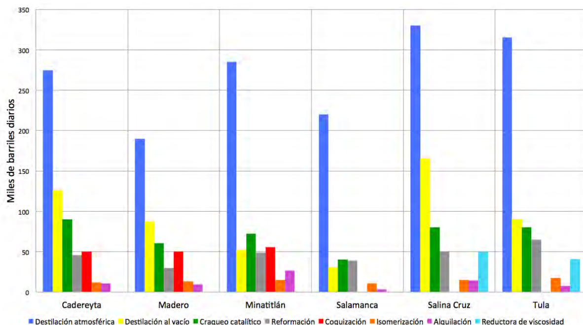
Figura 27. Capacidades nominales de procesos seleccionados en las refinéras del SNR 2017
