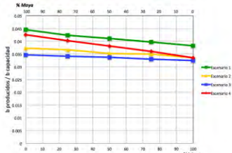
Figura 168. Rendimientos de GLP en Salamanca reconfigurada por escenario
