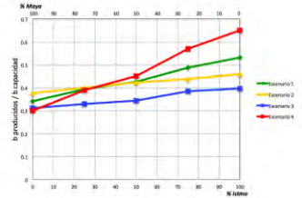
Figura 116. Rendimientos de gasolinas en Salamanca por escenario
