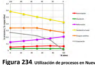
Figura 234. Utilización de procesos en Nueva refinería para el escenario 3
