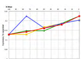
Figura 160. Utilización de Reformación en Tula por escenario
