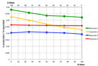
Figura 207. Rendimientos de GLP en Tula reconfigurada por escenario
