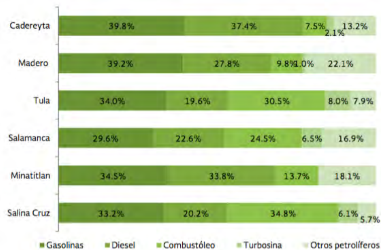
Figura 37. Rendimientos del crudo en la producción de petrolíferos 2015 (distribución porcentual)
