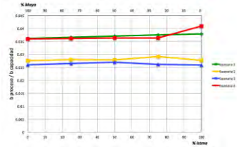
Figura 87. Utilización de Alquilación en Madero por escenario
