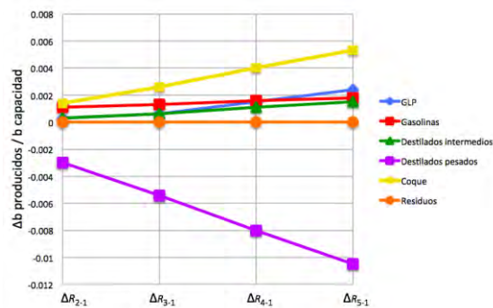
Figura 279. Diferencial de Rendimientos al sustituir crudo Istmo por WTS en Salina Cruz reconfigurada
