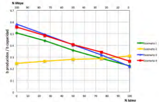
Figura 135. Rendimientos de destilados pesados en Salina Cruz por escenario
