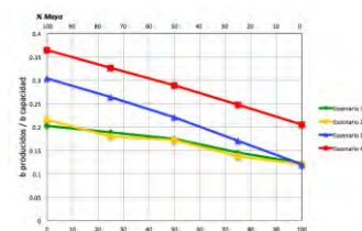
Figura 153. Rendimientos de destilados pesados en Tula por escenario
