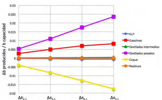
Figura 319. Diferencial de Rendimientos al sustituir crudo Maya por SGC en Salina Cruz reconfigurada
