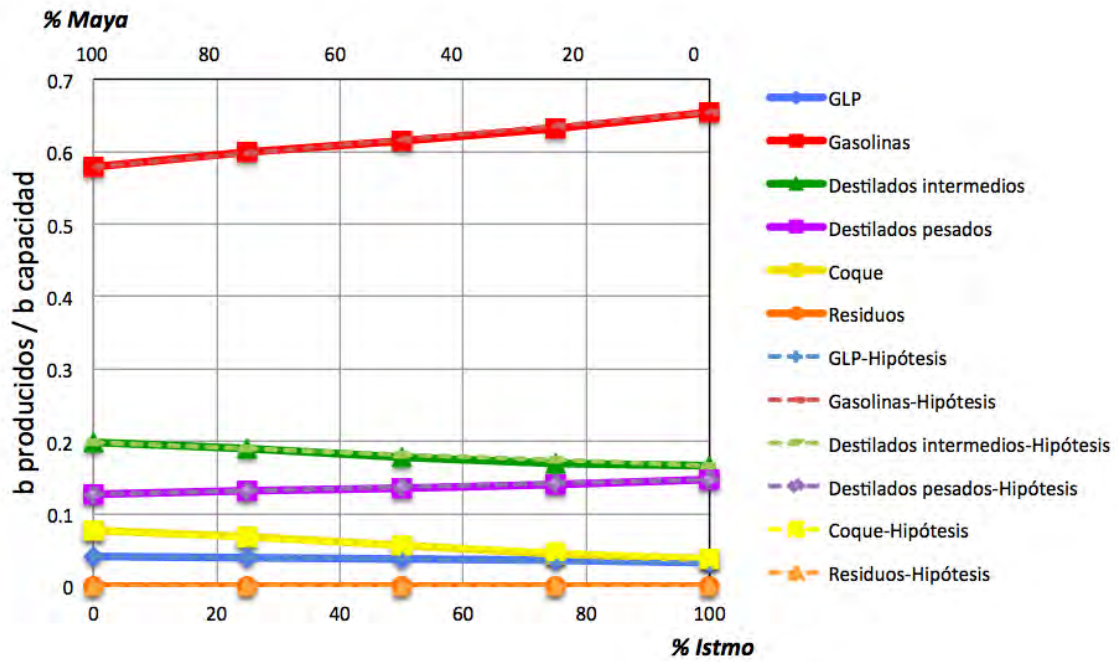
Figura 57. Rendimientos de petrolíferos en Cadereyta para el escenario 4
