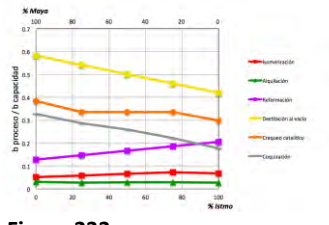
Figura 233. Utilización de procesos en Nueva refinería para el escenario 2
