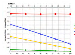
Figura 171. Rendimientos de destilados pesados en Salamanca reconfigurada por escenario
