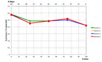
Figura 143. Utilización de Destilación al vacío en Salina Cruz por escenario
