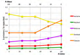
Figura 122. Utilización de procesos en Salamanca para el escenario 4
