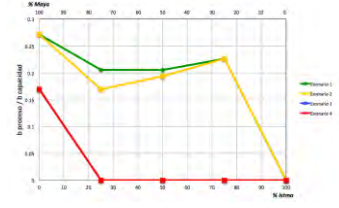
Figura 145. Utilización de Reductora de viscosidad en Salina Cruz por escenario
