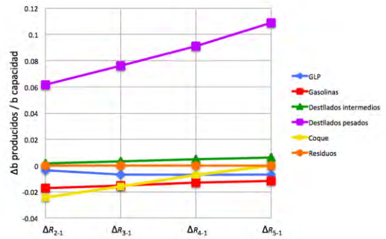
Figura 288. Diferencial de Rendimientos al sustituir crudo Maya por Tubarao en Salamanca reconfigurada
