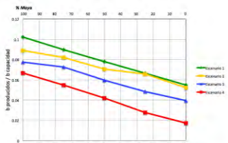
Figura 81. Rendimientos de coque en Madero por escenario
