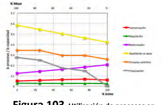
Figura 103. Utilización de procesos en Minatitlán para el escenario 3
