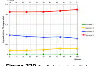
Figura 230. Rendimientos de destilados pesados en Nueva refinería por escenario
