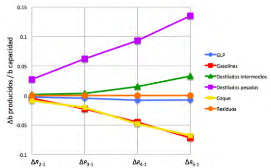
Figura 289. Diferencial de Rendimientos al sustituir crudo Maya por Tubarao en Salina Cruz reconfigurada
