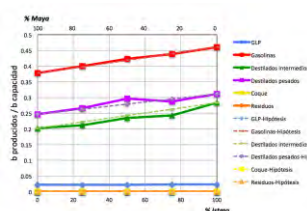
Figura 112. Rendimientos de petrolíferos en Salamanca para el escenario 2
