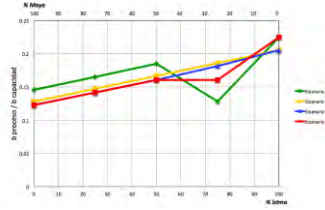
Figura 107. Utilización de Reformación en Minatitlán por escenario
