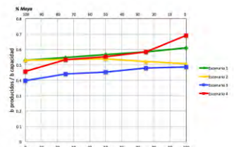
Figura 97. Rendimientos de gasolinas en Minatitlán por escenario
