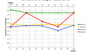
Figura 144. Utilización de Craqueo catalítico en Salina Cruz por escenario
