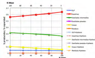
Figura 223. Rendimientos de petrolíferos en Nueva refinería para el escenario 1
