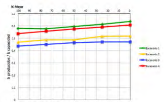
Figura 78. Rendimientos de gasolinas en Madero por escenario
