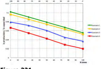
Figura 231. Rendimientos de coque en Nueva refinería por escenario
