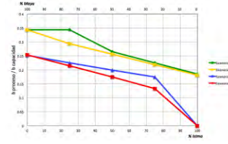
Figura 182. Utilización de Coquización en Salamanca reconfigurada por escenario
