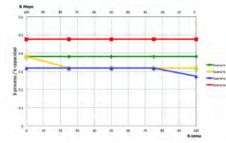
Figura 181. Utilización de Craqueo catalítico en Salamanca reconfigurada por escenario
