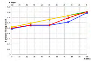
Figura 123. Utilización de Isomerización en Salamanca por escenario
