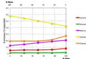
Figura 121. Utilización de procesos en Salamanca para el escenario 3
