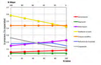
Figura 212. Utilización de procesos en Tula reconfigurada para el escenario 1
