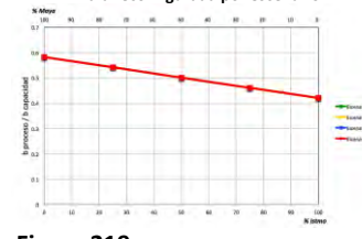
Figura 219. Utilización de Destilación al vacío en Tula reconfigurada por escenario
