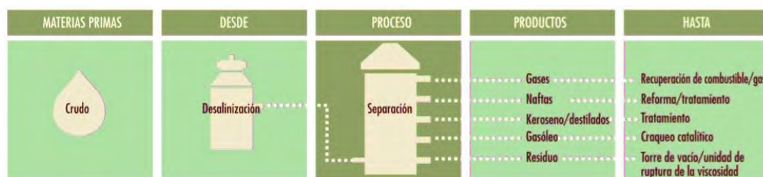
Figura 12. Representación del proceso de destilación atmosférica
