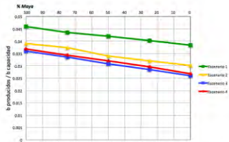
Figura 77. Rendimientos de GLP en Madero por escenario
