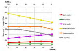
Figura 102. Utilización de procesos en Minatitlán para el escenario 2
