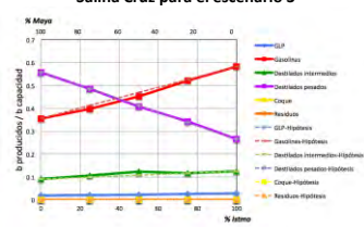
Figura 131. Rendimientos de petrolíferos en Salina Cruz para el escenario 4
