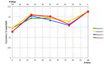
Figura 142. Utilización de Reformación en Salina Cruz por escenario
