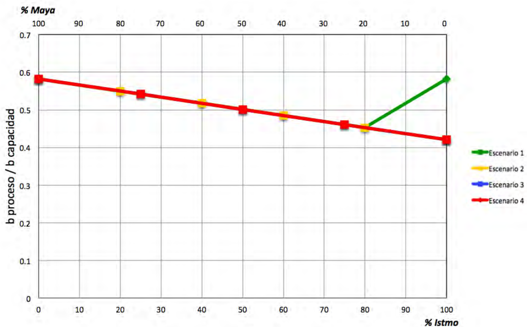
Figura 70. Utilización de Destilación al vacío en Cadereyta por escenario
