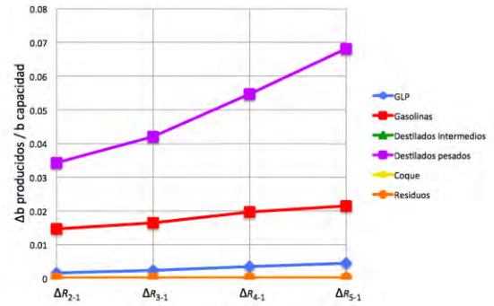
Figura 316. Diferencial de Rendimientos al sustituir crudo Maya por SGC en Salina Cruz
