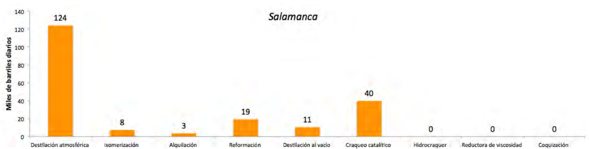
Figura 350. Utilización optimizada de procesos en Salamanca mediante la plataforma
