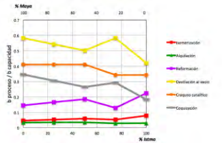
Figura 101. Utilización de procesos en Minatitlán para el escenario 1
