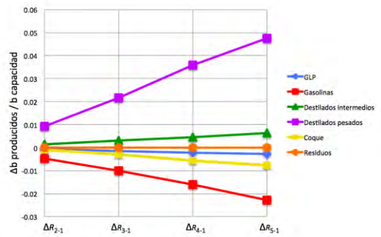
Figura 329. Diferencial de Rendimientos al sustituir crudo Maya por Bachaquero en Salina Cruz reconfigurada
