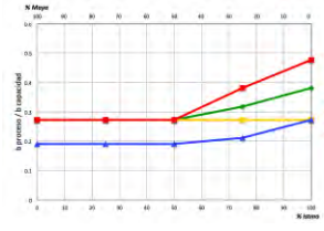
Figura 127. Utilización de Craqueo catalítico en Salamanca por escenario
