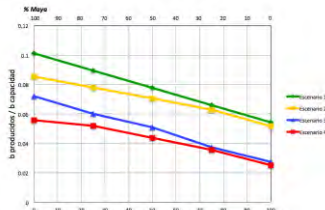
Figura 100. Rendimientos de coque en Minatitlán por escenario
