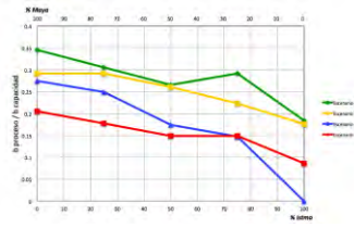
Figura 110. Utilización de coquización en Minatitlán por escenario
