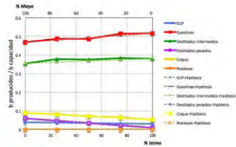
Figura 74. Rendimientos de petrolíferos en Madero para el escenario 2
