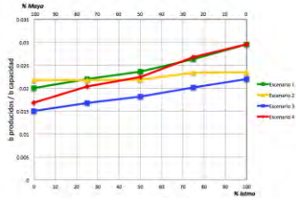
Figura 115. Rendimientos de GLP en Salamanca por escenario
