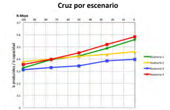
Figura 133. Rendimientos de gasolinas en Salina Cruz por escenario
