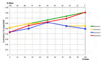
Figura 216. Utilización de Isomerización en Tula reconfigurada por escenario
