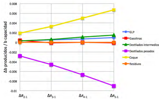
Figura 278. Diferencial de Rendimientos al sustituir crudo Istmo por WTS en Salamanca reconfigurada
