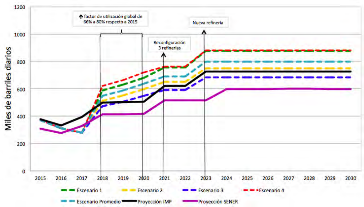
Fuente: Elaboración propia Figura 354. Producción nacional de gasolinas 2015-2030
