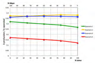
Figura 229. Rendimientos de destilados intermedios en Nueva refinería por escenario
