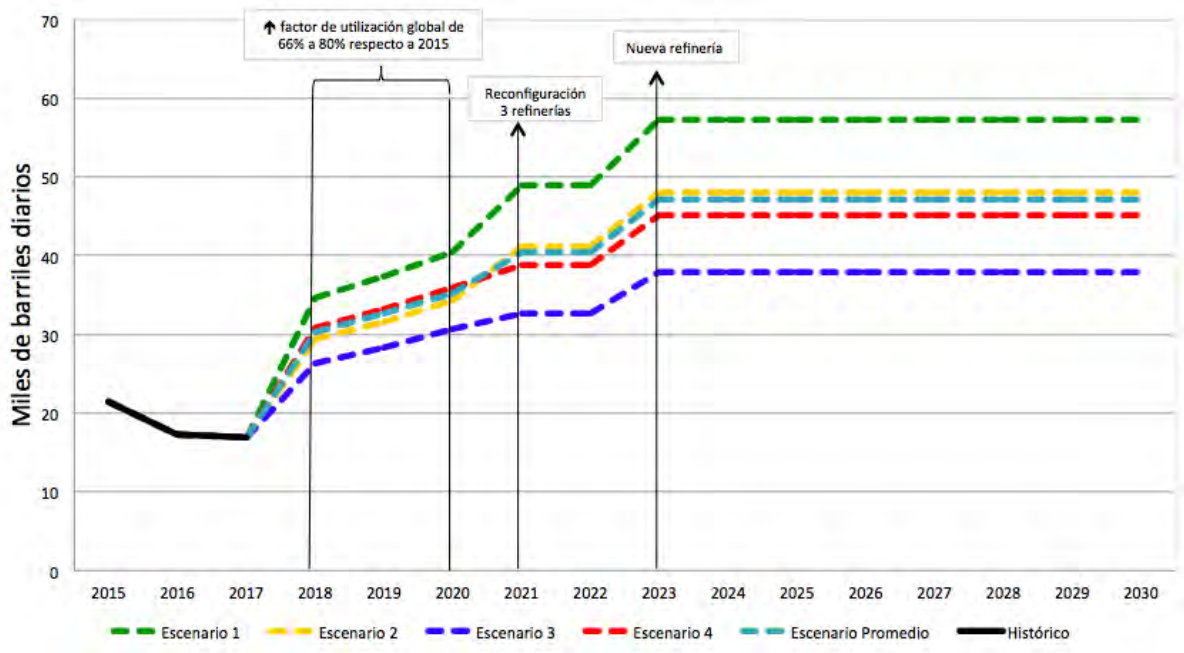
Fuente: Elaboración propia Figura 353. Producción nacional de GLP 2015-2030
