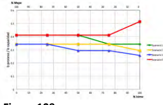
Figura 109. Utilización de Craqueo catalítico en Minatitlán por escenario
