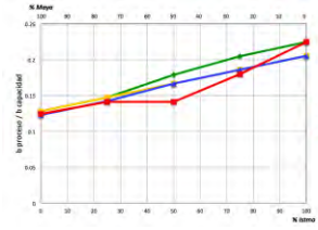
Figura 125. Utilización de Reformación en Salamanca por escenario
