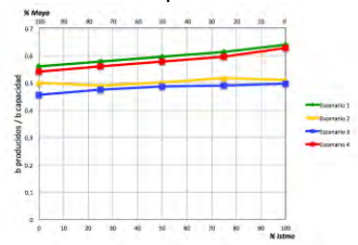
Figura 228. Rendimientos de gasolinas en Nueva refinería por escenario
