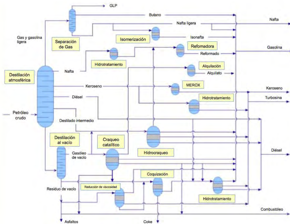
Figura 16. Diagrama de una refinera compleja
