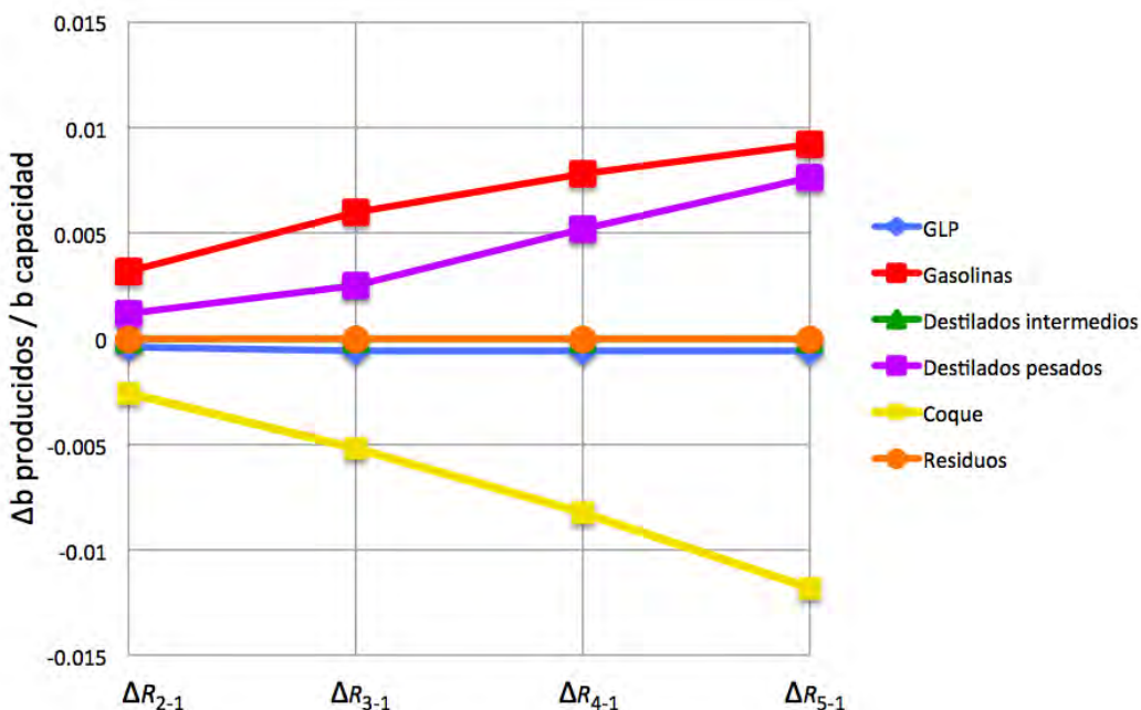
Figura 244. Diferencial de Rendimientos al sustituir crudo Istmo por WTI en Minatitlán
