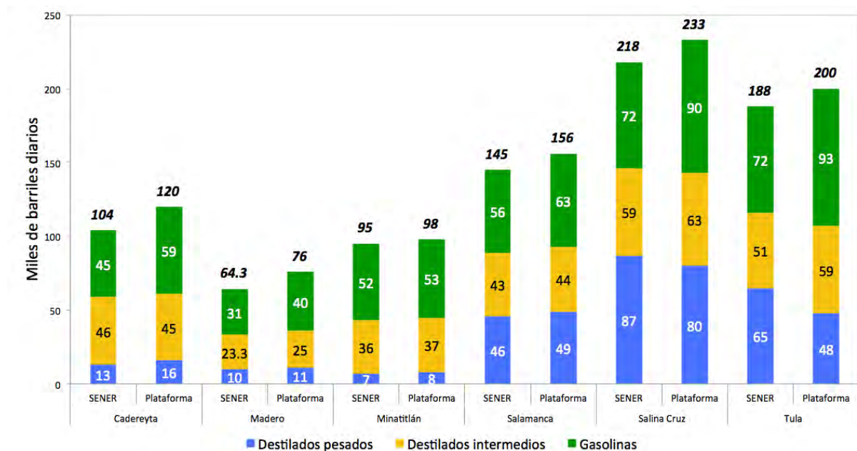
Figura 332. Comparación de producción de petrolíferos en 2016 entre la información de SENER y la plataforma de modelos
