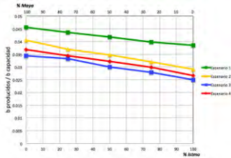
Figura 227. Rendimientos de GLP en Nueva refinería por escenario
