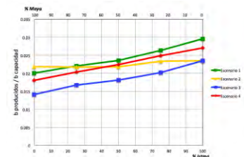
Figura 132. Rendimientos de GLP en Salina Cruz por escenario
