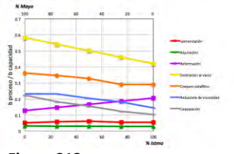
Figura 213. Utilización de procesos en Tula reconfigurada para el escenario 2
