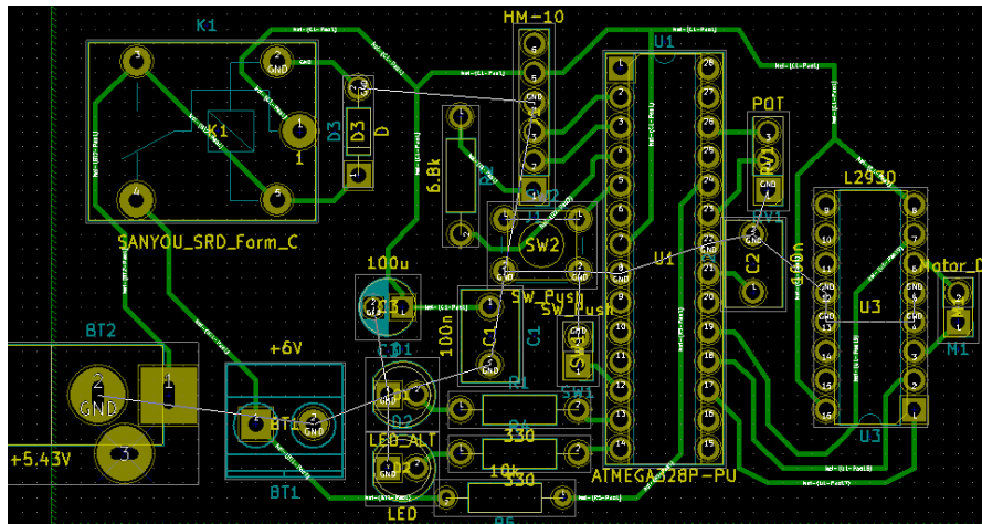
Figura 4.13 Posicionamiento y conexión de los componentes. (Fuente: Elaboración propia)
