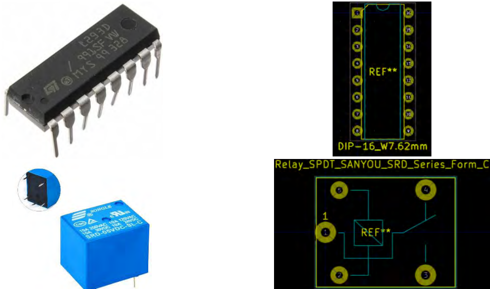
Figura 4.12 Ejemplos de huellas asociadas al driver L293D y relevador utilizados.
