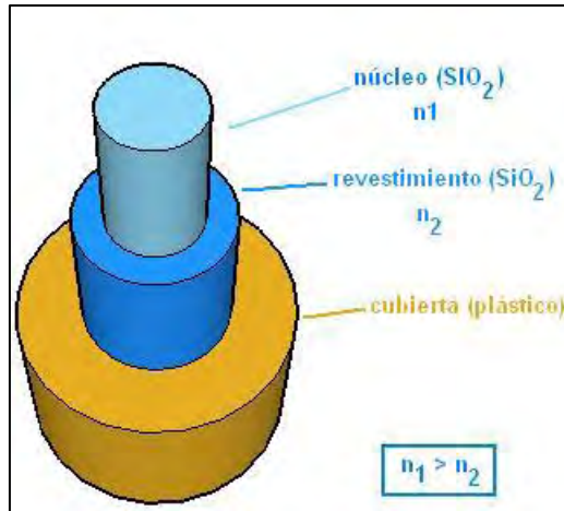
Figura 2.7 Composición interna de la fibra óptica
