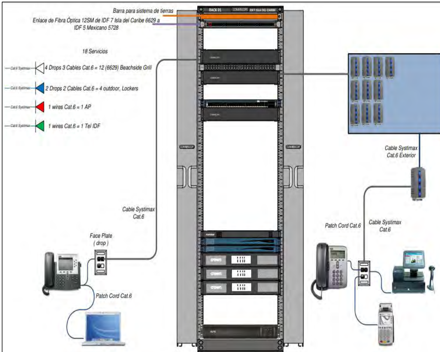
Figura 7.12 Diseño de conexión de un rack en un IDF
