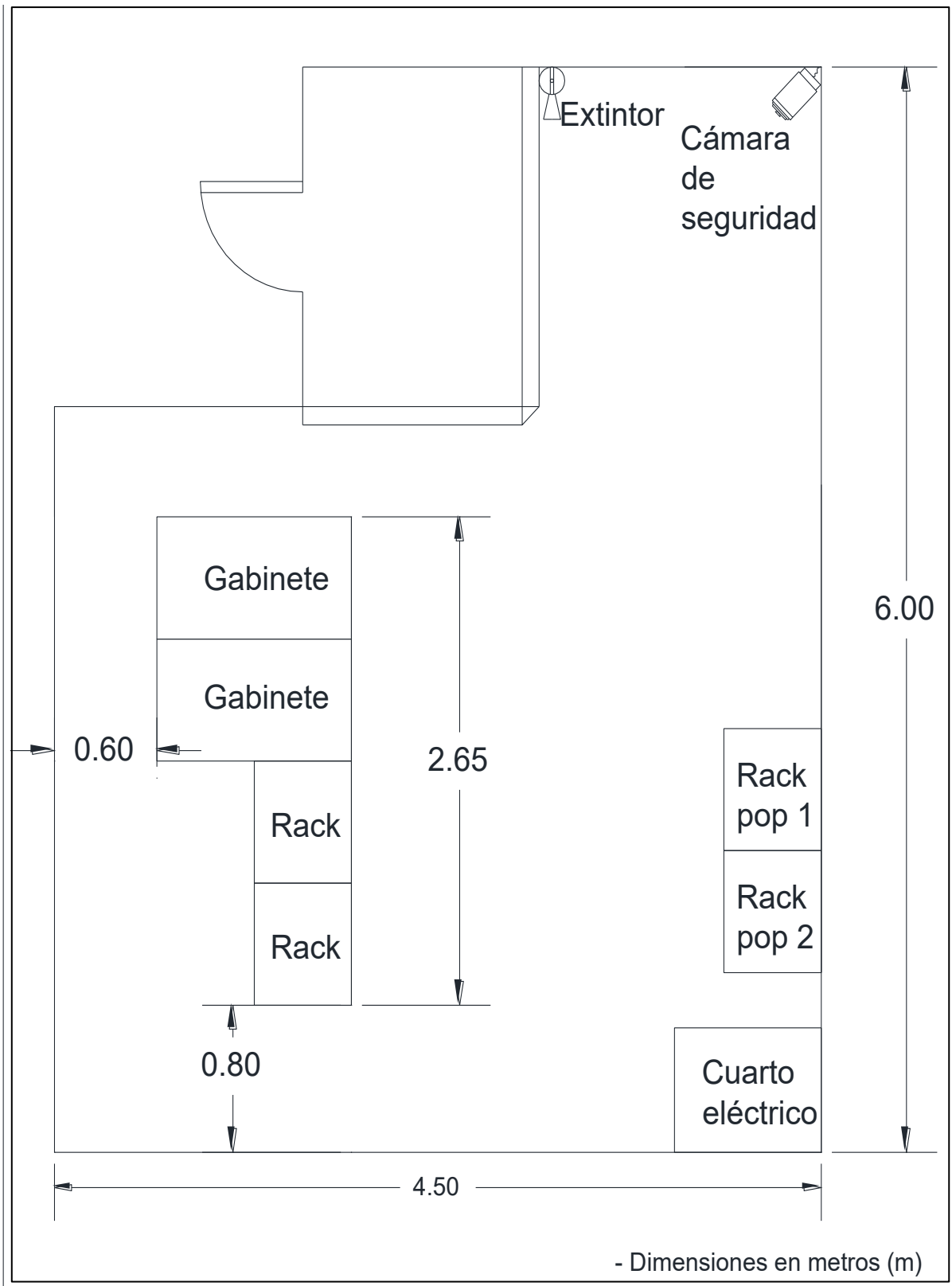
Figura 5.13 Croquis de distribución final del datacenter
