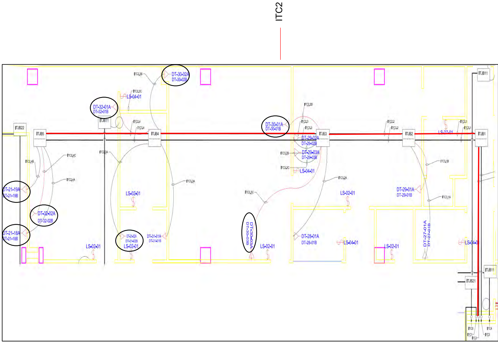
Figura 8.1 Plano parcial de conexiones de tuberías en zona de oficinas
