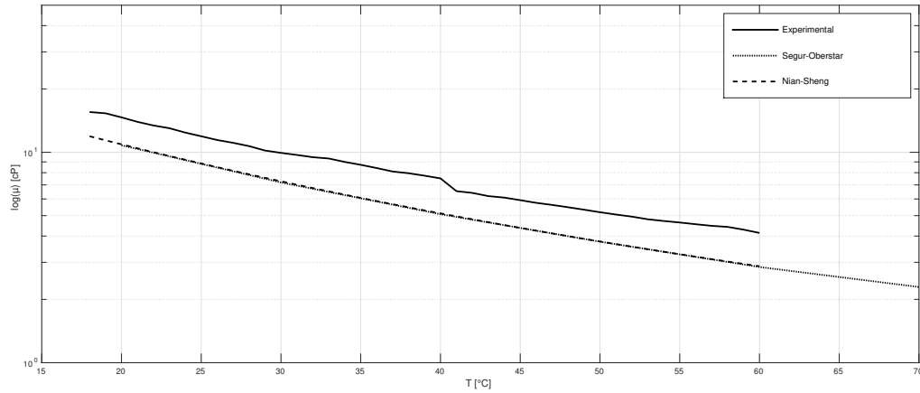
Figura 4.8: Comparación de resultados experimentales para 60%wt de glicerina, con datos calculados con la ecuación de Cheng (2008) y con datos de Segur & Oberstar (1951).
