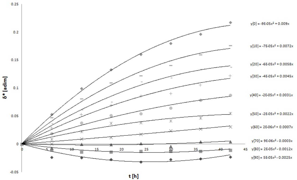
Figura 8. Desplazamiento adimensional de la interfase, contra tiempo, para distintas concentraciones
