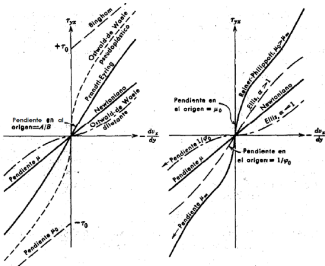
Figura 2.3: Comportamiento de fluidos newtonianos y no newtonianos (Imagen tomada a partir de Bird et al. (2004))
