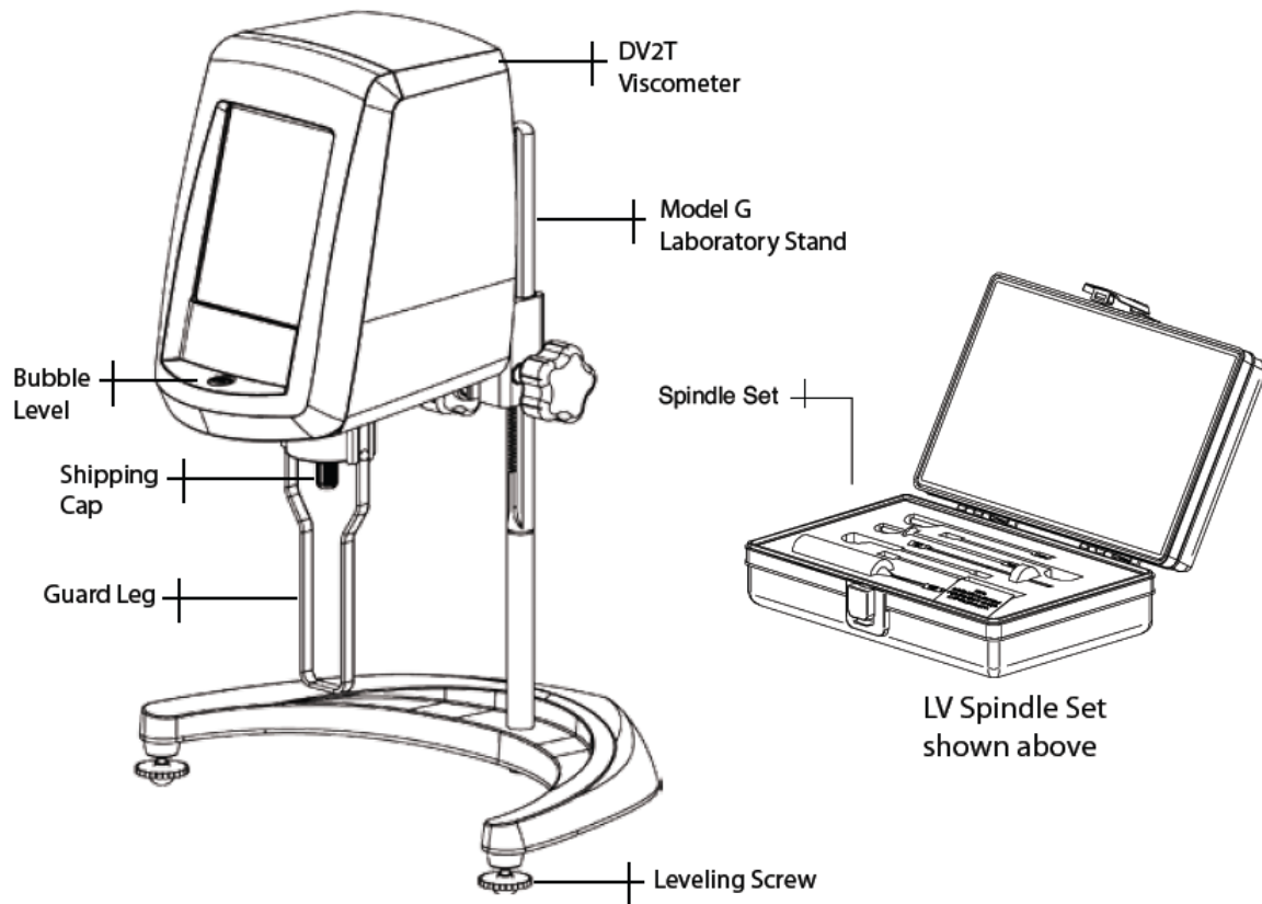
Figura 3.1: Componentes Brookfield Viscosimeter DV2T: Viscosímetro Brookfield DV2T, kit de agujas de medición (Imagen tomada a partir de Brookfield DV2T Manual No. M13-167-B0614 BRO (n.d. a))
