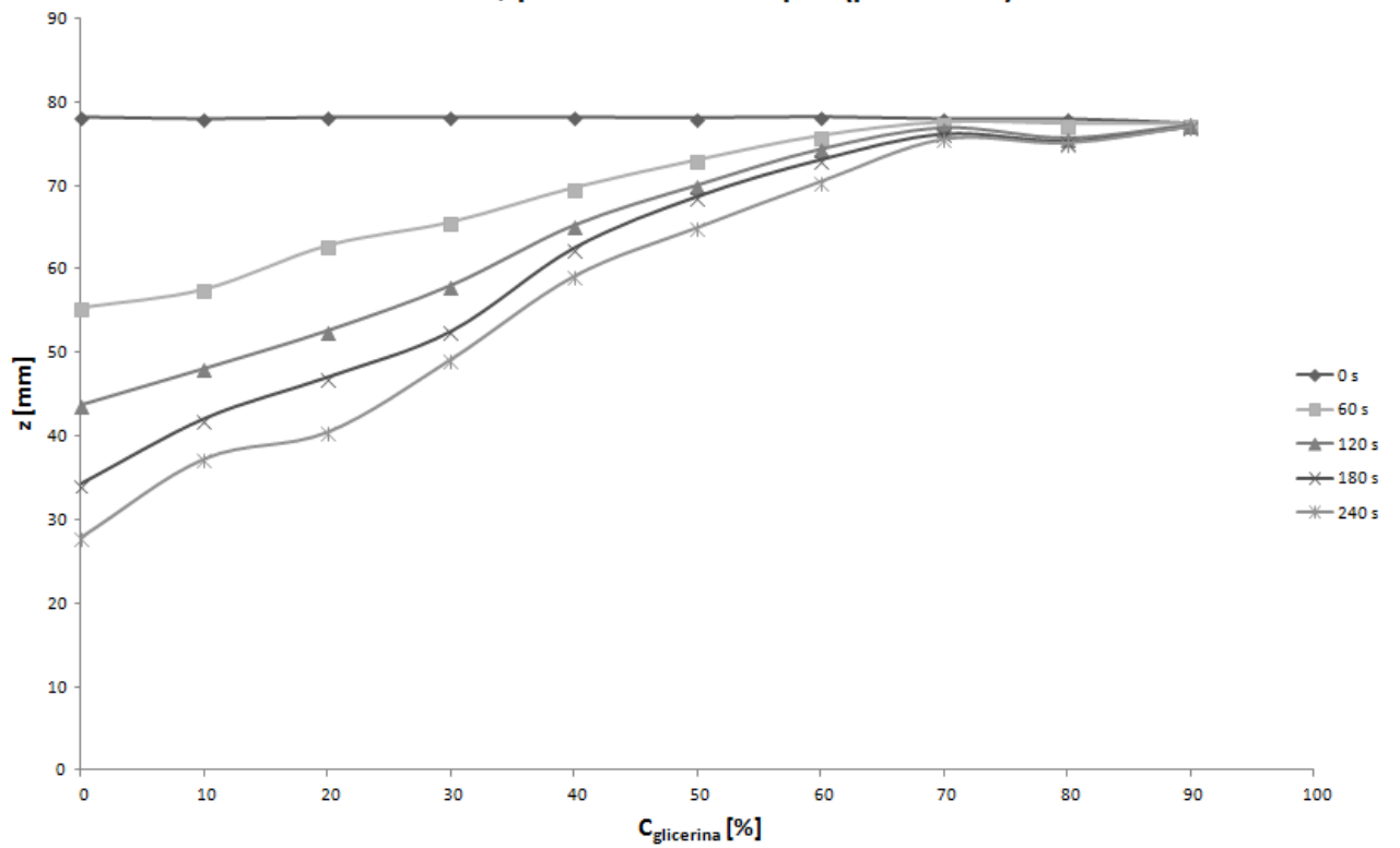
Figura 12. Nivel de la interfase contra concentración, en condiciones dinámicas bruscas, para distintos tiempos
