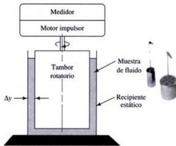
Figura 2.7: Esquema de los componentes de un viscosímetro rotatorio de cilindros concéntricos (Imagen tomada a partir de Mott & Brito (2006))
