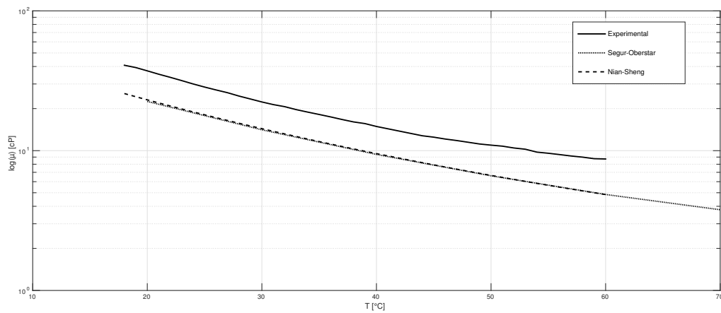
Figura 4.9: Comparación de resultados experimentales para 70%wt de glicerina, con datos calculados con la ecuación de Cheng (2008) y con datos de Segur & Oberstar (1951).
