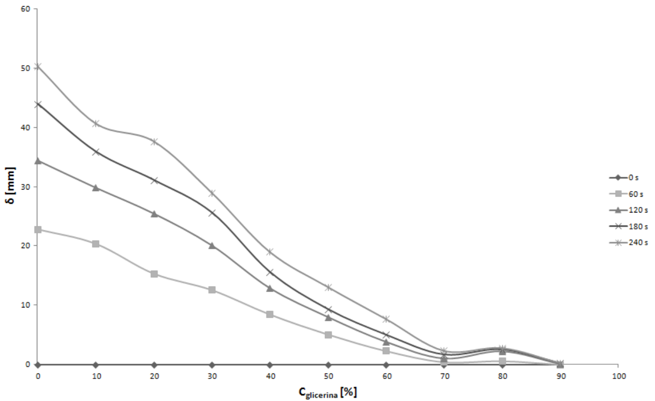
Figura 14. Desplazamiento de la interfase contra concentración, en condiciones dinámicas bruscas, para distintos tiempos
