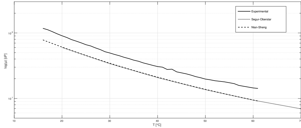
Figura 4.10: Comparación de resultados experimentales para 80 %wt de glicerina, con datos calculados con la ecuación de Cheng (2008) y con datos de Segur & Oberstar (1951).
