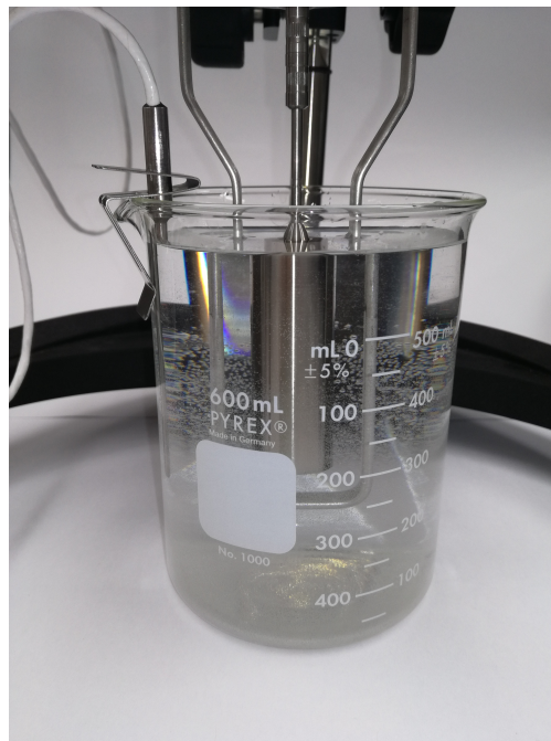
Figura 3.9: Acecamiento de fotografía de prueba con aguja# 61 para glicerina pura en viscosímetro Brookfield DV2T
