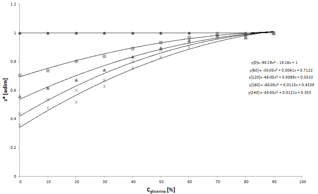
Figura 16. Nivel adimensional de la interfase contra concentración, en condiciones dinámicas bruscas, para distintos tiempos
