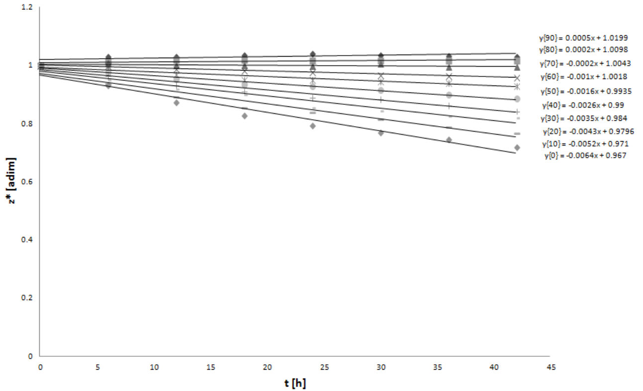
Figura 6. Nivel adimensional de la interfase contra tiempo, en condiciones estáticas, para distintas concentraciones
