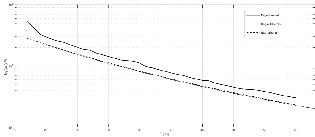
Figura 4.11: Comparación de resultados experimentales para 90 %wt de glicerina, con datos calculados con la ecuación de Cheng (2008) y con datos de Segur & Oberstar (1951).
