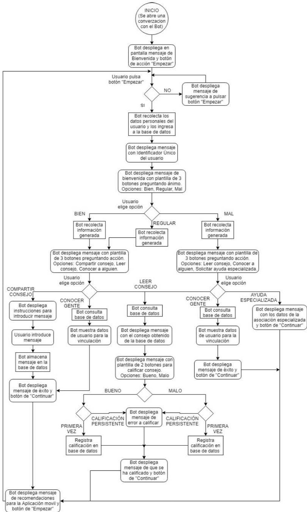
Figura 5.2 Diagrama de flujo para funcionamiento del Bot.
