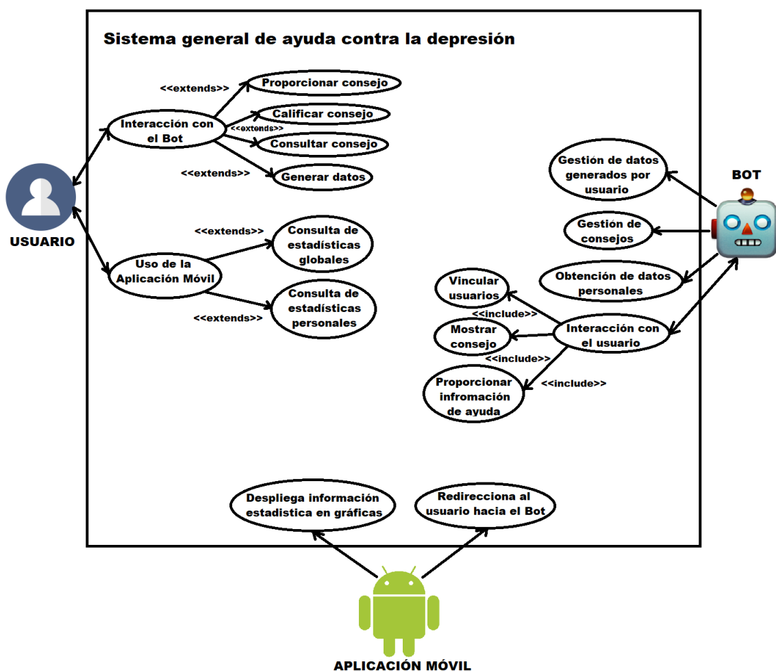
Figura 5.1 Diagrama general de casos de uso.
