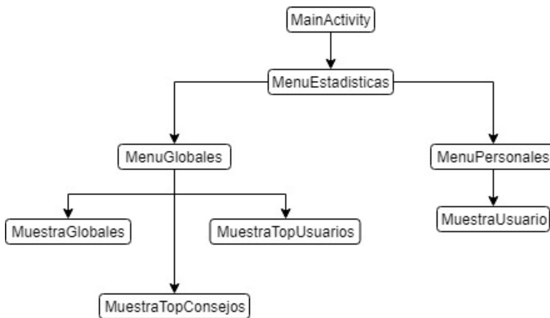
Figura 5.7 Diagrama de flujo para actividades Android
