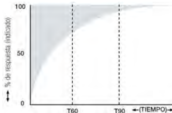
Ilustración 27. Tiempo de respuesta para un sensor catalítico.
