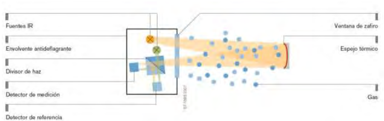
Ilustración 29. Arreglo de sensores infrarrojos. Drager.
