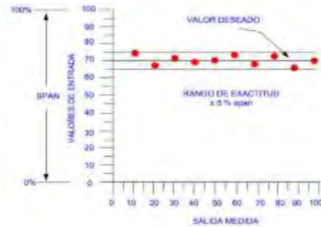
Ilustración 19. Exactitud en un instrumento de medición.
