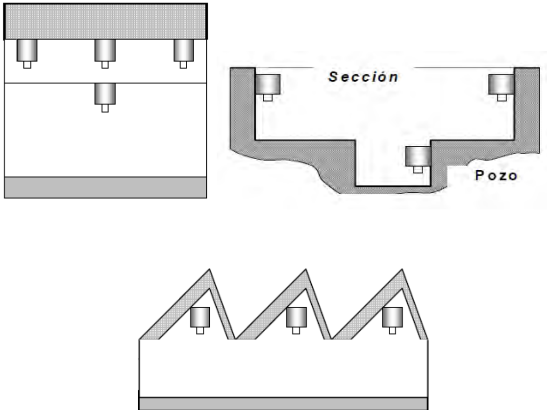
Ilustración 37.Ubicación de sensores de acuerdo al lugar.
