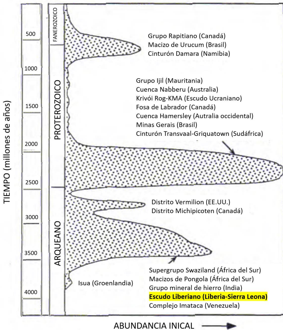
Figura 2. Abundancia estimada de formación de hierro depositado a lo largo del tiempo geológico. Escala horizontal es esquemática-no lineal, aproximadamente logarítmica; rango de 0 – 10^{15} toneladas (tomada y modificada de James, 1983).
