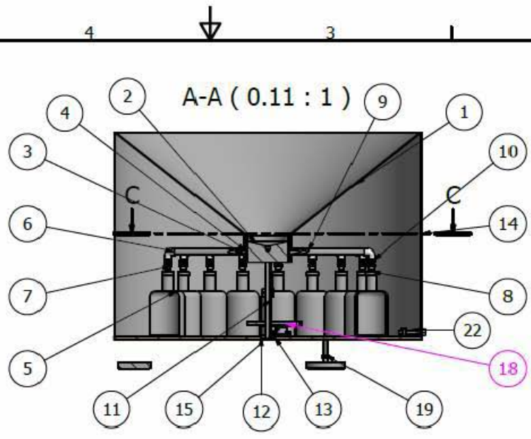
A-A ( 0.11 : 1 )
