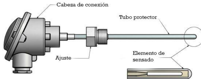
Ilustración 4.4-13 Esquema de un sensor de temperatura por resistencia. Recuperado en http://www.ingmecafenix.com/automatizacion/sensor-temperatura-rtd/
