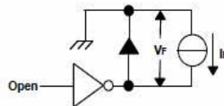
Fig.8 Vf Test Circuit
