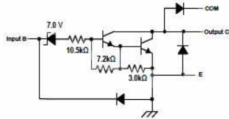
ULN2002A
