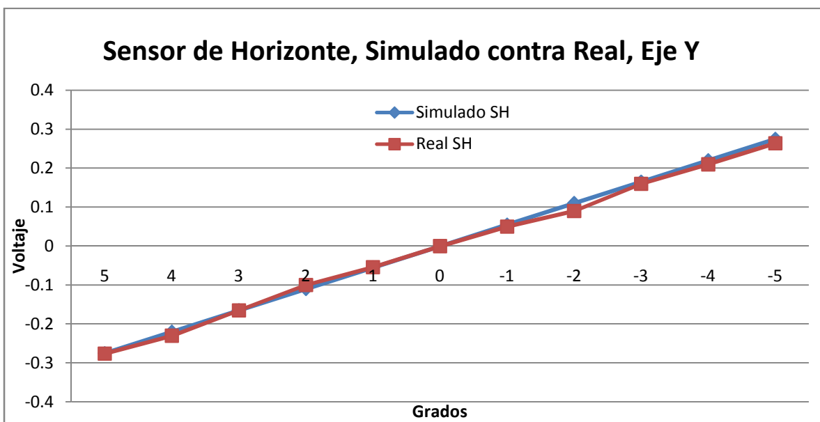
Gráfica 6.15b Respuesta simulada contra real, esto en el eje Y.
