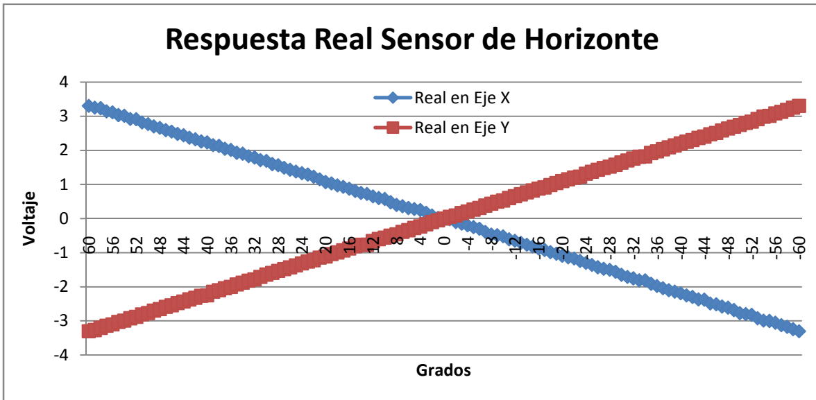
Gráfica 6.13 Respuesta real del sensor de Horizonte.
