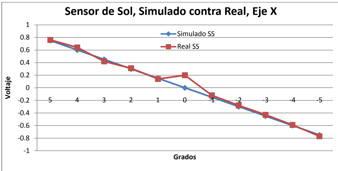
Gráfica 6.14a Respuesta simulada contra real, esto en el eje X.
