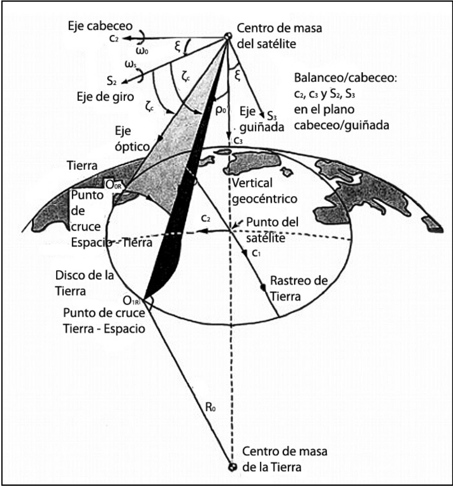
Figura 4.8 Configuración del sensor de Horizonte del tipo de escaneo [51].
