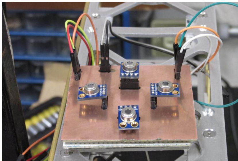
Figura 6.16 Sensor de Horizonte sobre la estructura del nanosatélite.
