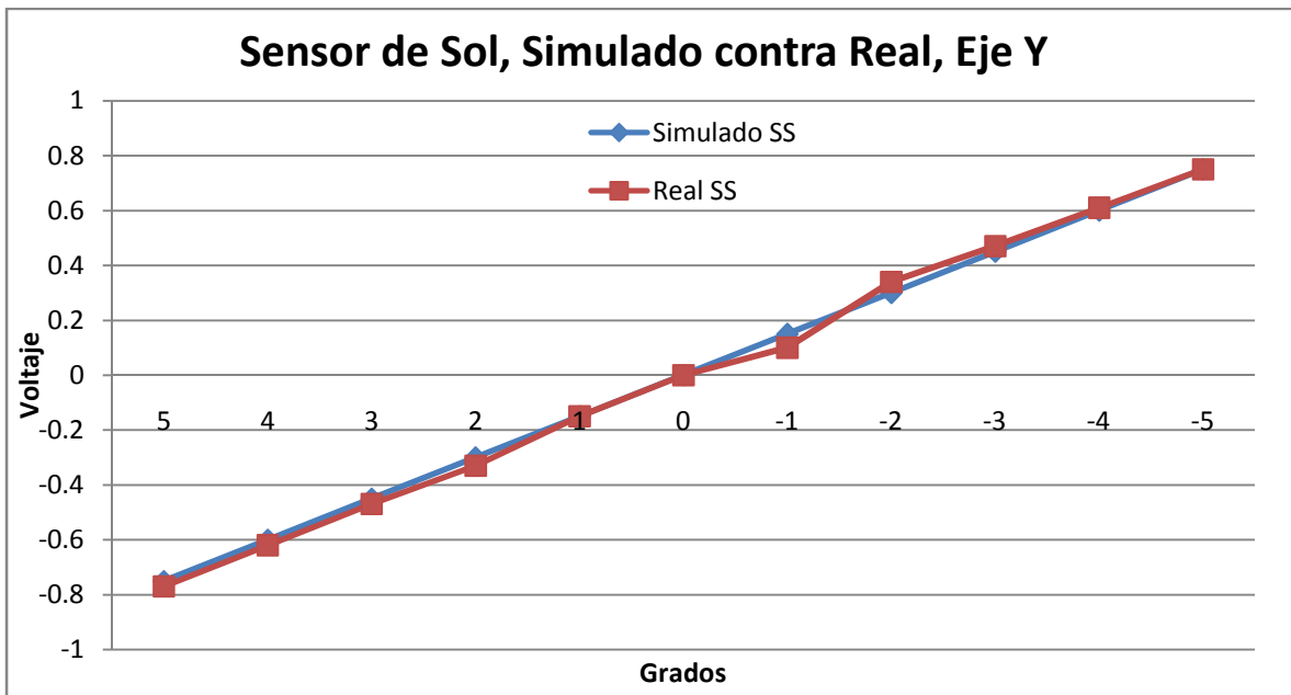
Gráfica 6.14b Respuesta simulada contra real, obtenida en el eje Y.
