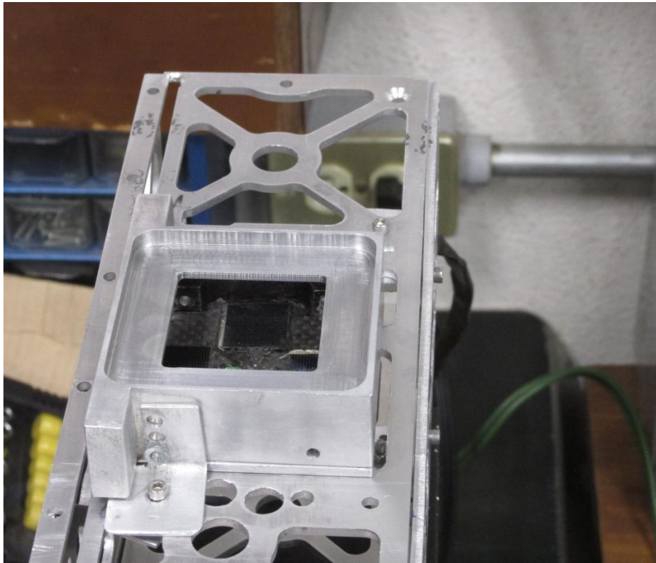
Figura 6.15 Sensor Solar montado sobre la estructura de un nanosatélite tipo Cubesat 3U.
