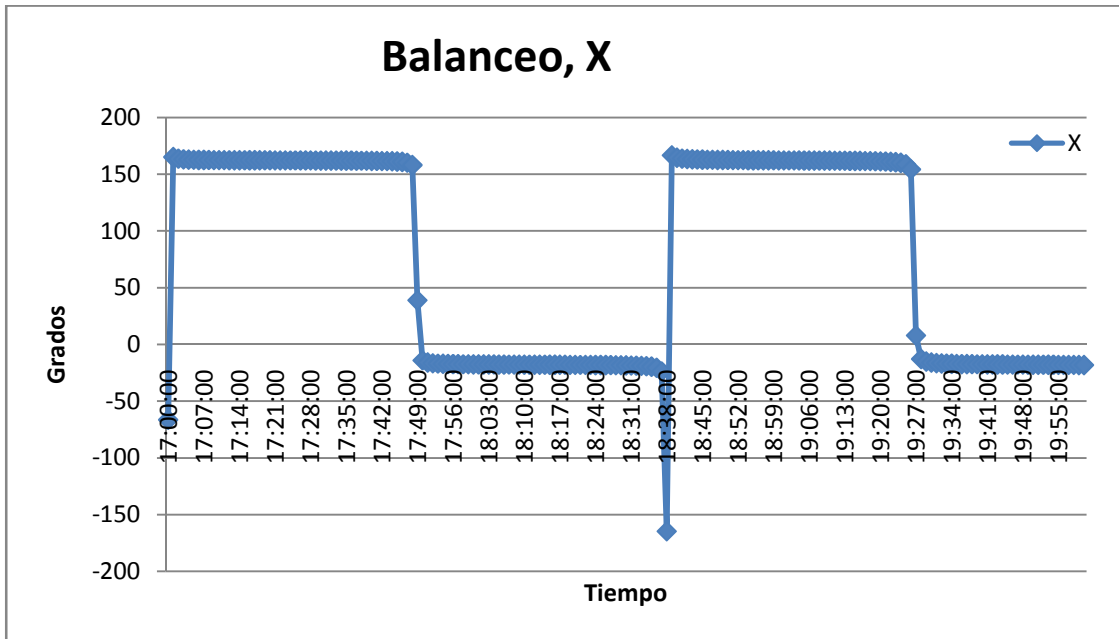
Gráfica 6.2 Datos del comportamiento del eje balanceo, X, en grados.
