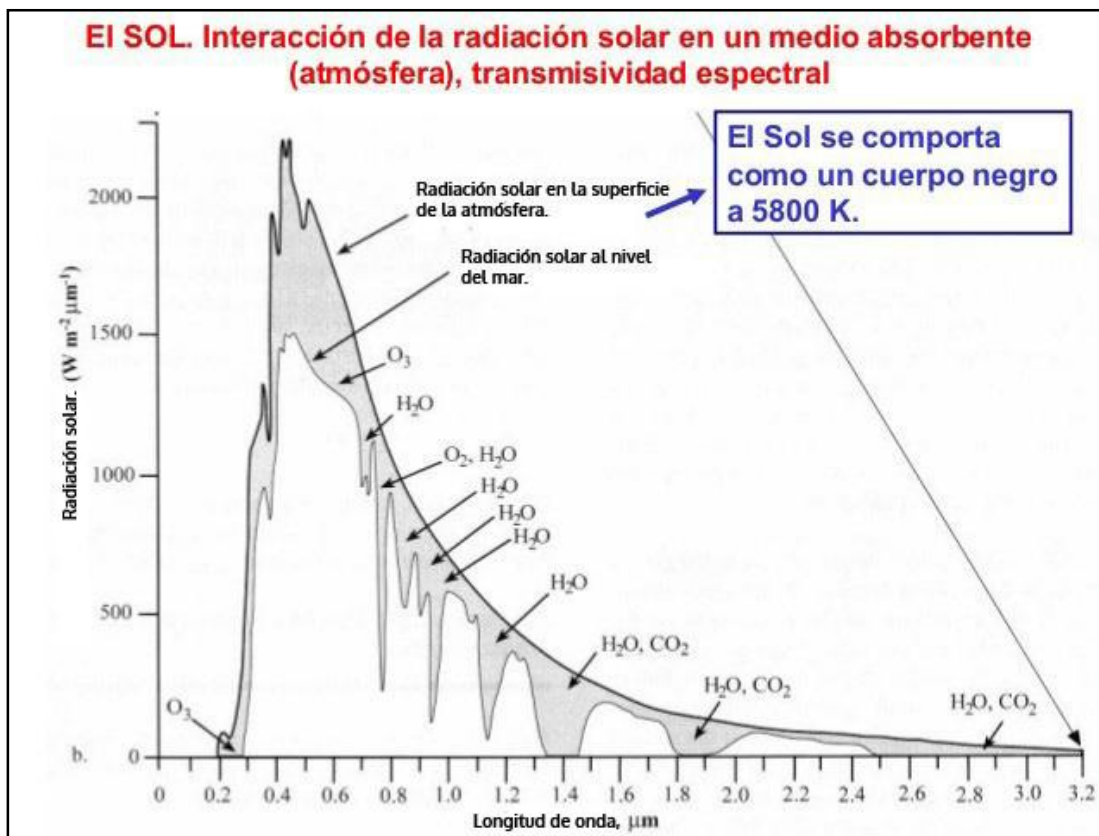
Figura 4.6 Capas de absorción de radiación solar de la atmósfera Terrestre [50].
