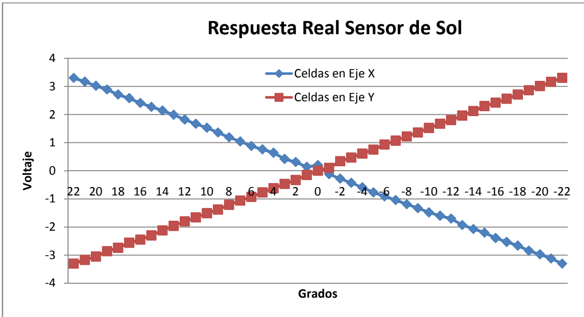
Gráfica 6.12 Respuesta real del sensor de Sol.
