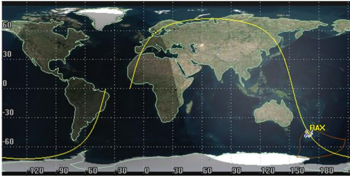
Figura 6.8 Traza de la órbita del satélite sobre el mapa en 2D.
