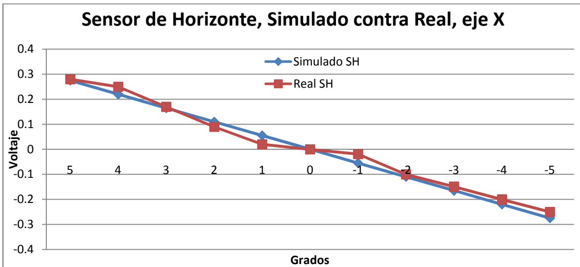
Gráfica 6.15a Respuesta simulada contra real, esto en el eje X.
