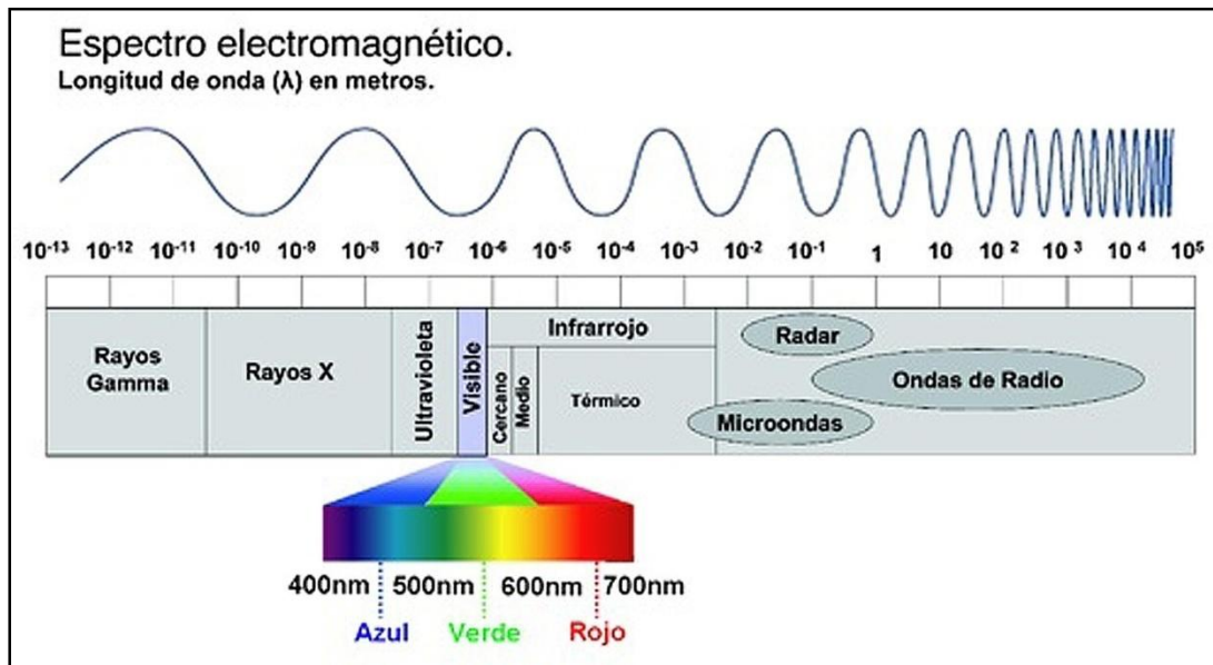
Figura 2.3 Longitudes de onda emitidas por el sol [40].
