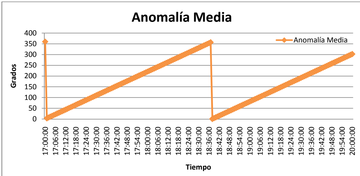
Gráfica 6.8 Anomalía media (en grados). De forma similar a la anomalía verdadera, la anomalía media vuelve a su punto inicial en cada órbita.
