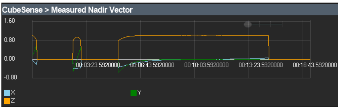
Figura 6.12 Vector de nadir obtenido en una órbita. En estas figuras podemos ver como va cambiando el vector con el movimiento del satélite.
