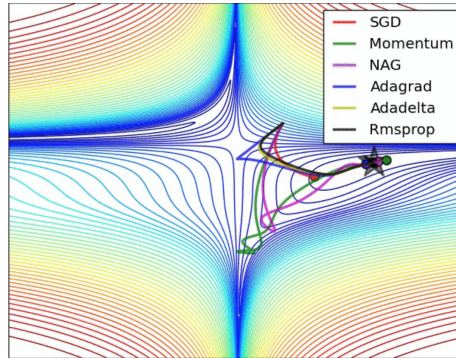
Figura 2.7: La optimización realizada por el algoritmo SGD con mini-lotes. Se muestra el comportamiento de distintos optimizadores. (Tomado de [16].)
