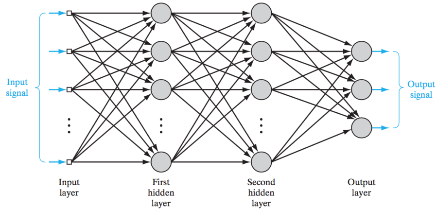
Figura 2.6: Arquitectura de un MLP con dos capas ocultas. (Tomado de [10].)
