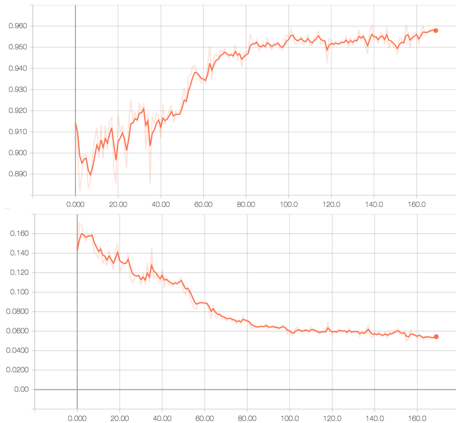
Figura 4.8: Dos funciones de evaluación para la afinación de Inception V3 . El gráfico de la parte superior muestra la precisión con la que el modelo realiza sus clasificaciones, mientras que el gráfico de la parte inferior muestra el error medio absoluto entre las clasificaciones hechas por el modelo contra las verdaderas. Ambos gráficos se generaron a partir de un muestreo del 10% de los datos disponibles. (Fuente: elaboración propia.)
