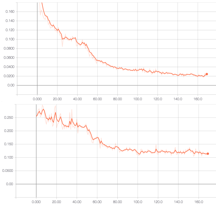
Figura 4.7: Funciones de error de entrenamiento y validación (gráfico de arriba y de abajo, respectivamente) para la afinación de Inception V3 . Esto es, entrenar un clasificador entre lo que es un meme y lo que no es. Se quita la última capa y se añade un MLP con dos dimensiones de salida. (Fuente: elaboración propia.)
