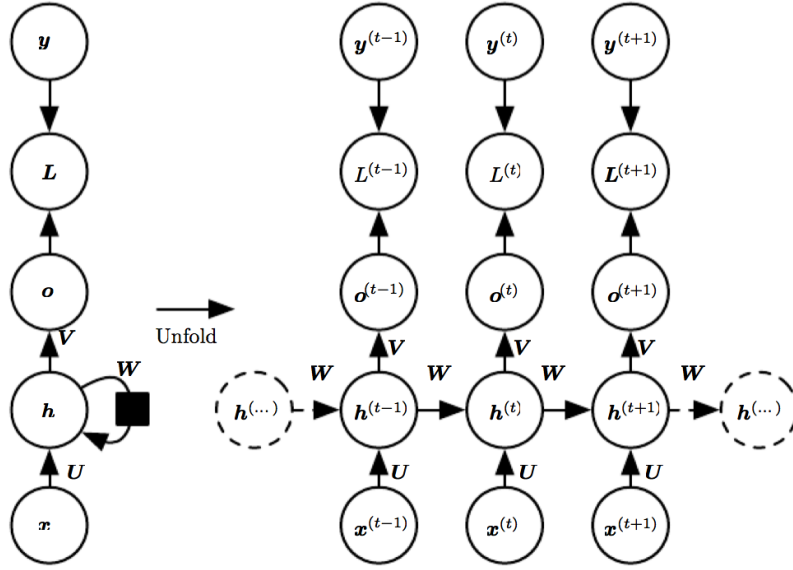
Figura 2.13: Arquitectura gráfica de una red neuronal recurrente. (Tomado de [9])
