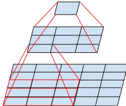
Figura 3.1: Una convolución de 5 \times 5 es un perceptrón multicapa, per se . (Tomado de https://arxiv.org/pdf/1512.00567.pdf .)
