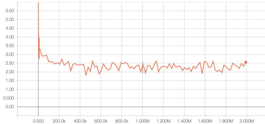
Figura 4.13: Función de error para el entrenamiento de la LSTM, usando 5 leyendas por personaje, un vocabulario reducido y códigos convolucionales generados a partir de una CNN superficial. (Fuente: elaboración propia.)
