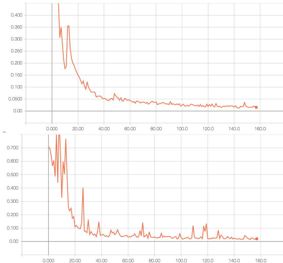
Figura 4.11: Funciones de error de entrenamiento y validación (gráfico de arriba y de abajo, respectivamente) de la CNN superficial. Obsérvese que solo se requirieron alrededor de 150 épocas de entrenamiento para llegar a un valor óptimo; esto dado el tamaño del conjunto de datos ( memes y no memes ) que es bastantes órdenes de magnitud más pequeño el conjunto de datos de entrenamiento presentado en la Sección 4.1. (Fuente: elaboración propia.)
