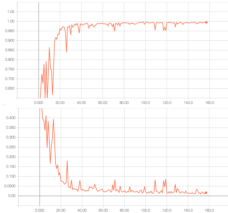
Figura 4.12: Dos funciones de evaluación para el modelo convolucional superficial. El gráfico de la parte superior muestra la precisión con la que el modelo realiza sus clasificaciones, mientras que el gráfico de la parte inferior muestra la error medio absoluto entre las clasificaciones hechas modelo contra las verdaderas. Ambos gráficos se generaron a partir de un muestreo del 10% de los datos disponibles. (Fuente: elaboración propia.)
