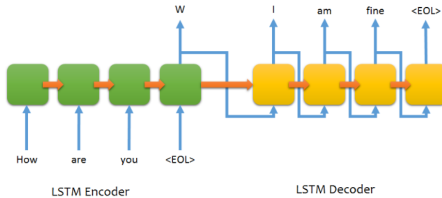
Figura 5.2: Arquitectura Seq2Seq aplicada al aprendizaje de modelos de lenguaje para un agente conversacional. Típicamente, se utilizan conjuntos de datos que enseñen al agente a responder preguntas que haría un usuario. (Tomado de https://github.com/farizrahman4u/seq2seq.git ).
