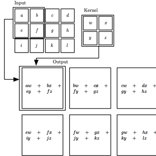
Figura 2.11: Ilustración del proceso de convolución. El filtro se desliza por la imagen de entrada y se efectúa un producto pixel por pixel.) (Tomado de [9].)
