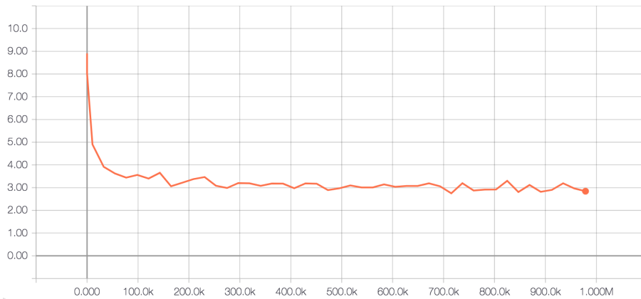
Figura 4.10: Función de error para el experimento que involucra la red Inception V3 afinada y 5 leyendas por personaje en el entrenamiento. (Fuente: elaboración propia.)
