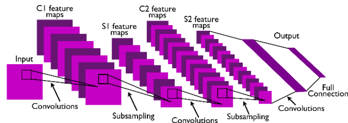
Figura 2.12: Estructura básica de una red neuronal convolucional, con dos fases de extracción de características. (Tomado de [13])
