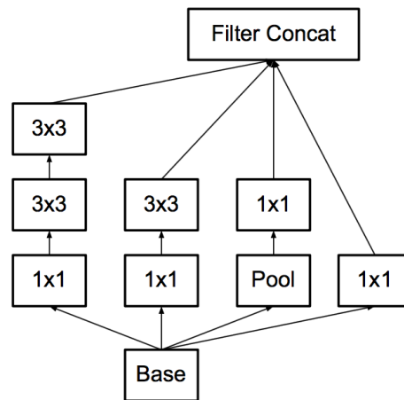
Figura 3.2: Otra manera de factorizar una convolución consiste en paralelizar el cómputo del filtro. Cabe destacar que los parámetros de cada nuevo filtro son compartidos entre sí, por cada nueva capa. Aquí reemplazamos un filtro de 5 \times 5 con dos filtros de 3 \times 3 y una capa de pooling. (Tomado de https://arxiv.org/pdf/1512.00567.pdf .)
