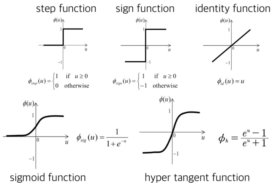
Figura 2.5: Las funciones de activación más comunes. (Tomado de https://www.slideshare.net/SungJuKim2/multi-layer-perceptron-back-propagation )
