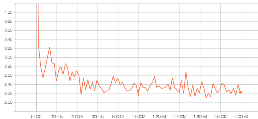
Figura 4.14: Función de error para el entrenamiento de la LSTM, con códigos convolucionales dados por una CNN superficial y 20 leyendas por imagen. Como se observa, existe una ligera disminución en el error resultante al final del entrenamiento, con respecto al obtenido en experimentos anteriores. (Fuente: elaboración propia.)
