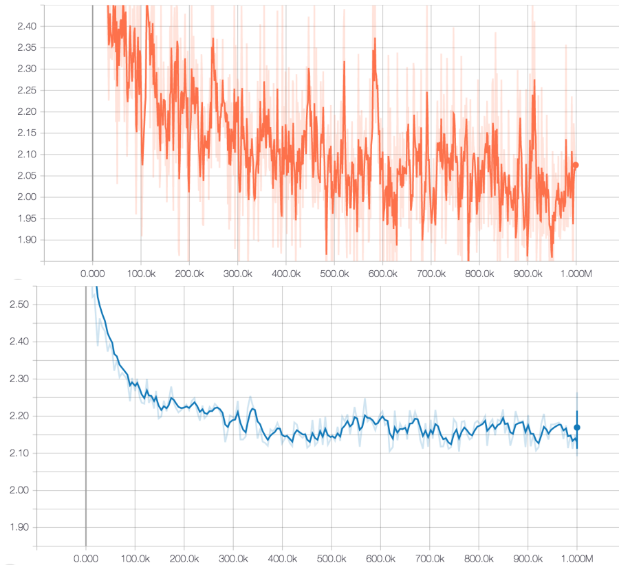
Figura 4.5: Función de error de entropía cruzada para el primer experimento exploratorio. En el gráfico de la parte superior se muestra el error a través de cada época del entrenamiento, mientras que el de la parte inferior se calculó por medio de un conjunto de datos de validación (de menor tamaño que el de entrenamiento). Ambos gráficos indican el valor de la entropía cruzada (eje de las ordenadas) a través del tiempo (eje de las abscisa). (Fuente: elaboración propia.)
