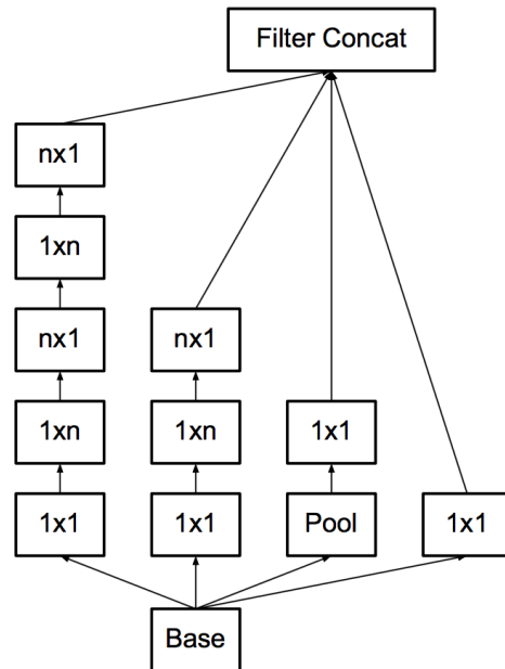
Figura 3.3: Factorización de una convolución de n \times n , donde n = 7 . (Tomado de https://arxiv.org/pdf/1512.00567.pdf .)
