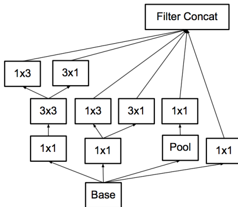
Figura 3.4: Factorización de una convolución de 8 \times 8 . (Tomado de https://arxiv.org/pdf/1512.00567.pdf .)
