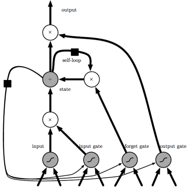
Figura 2.14: Estructura de la compuerta cerrada de una LSTM. (Tomado de [9])
