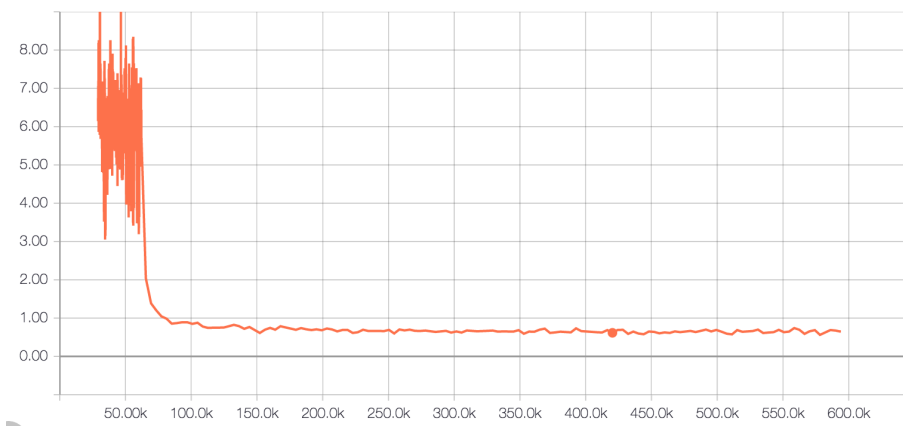
Figura 4.9: Función de error para el entrenamiento de la LSTM, dándole como estado inicial un tensor generado a partir de la red Inception V3 afinada. (Fuente: elaboración propia.)
