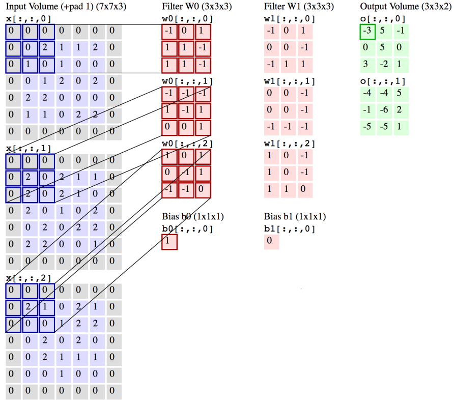
Figura 2.9: Ilustración de una pequeña capa convolucional. Cada imagen de entrada contiene tres niveles de profundidad, con los cuales trabaja el filtro (un tensor de pesos). Cabe destacar que cada valor de x está relleno por ceros. Dado que la profundidad del volumen de la salida es sólo 2, hay igual número de filtros en total. (Tomado de http://cs231n.github.io/convolutional-networks/ .)
