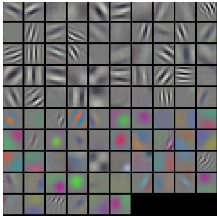
Figura 3.6: Así se ven los filtros entrenados de la primera capa de una CNN profunda. En este caso se trata de una AlexNet. La literatura suele conocer a los resultados de estos filtros como “ características generales ”. (Tomado de http://cs231n.github.io/understanding-cnn/ .)
