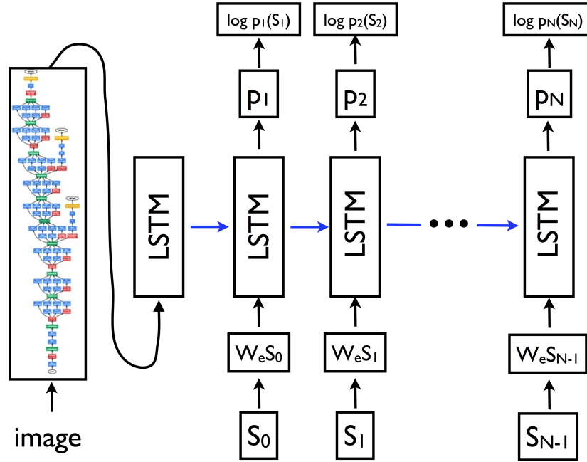
Figura 3.5: La arquitectura Show and Tell , propuesta por Vinyals, et al. , [23] en la cual se conecta una CNN Inception con una LSTM. (Tomado de https://arxiv.org/pdf/1411.4555.pdf .)
