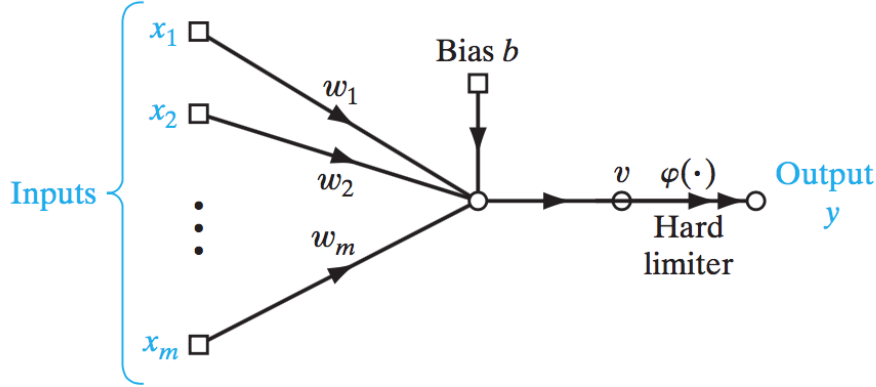
Figura 2.3: El perceptrón de Rosenblatt es un modelo gráfico cuya salida depende de las contribuciones lineales de cada una de las entradas, de un sesgo y de una función no lineal de activación. (Tomado de [10])
