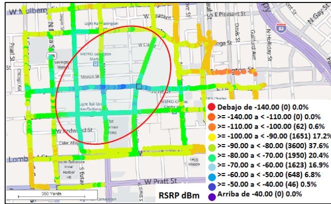
Figura 3.5 Ejemplo de mapa de RSRP con scanner PCTEL.
