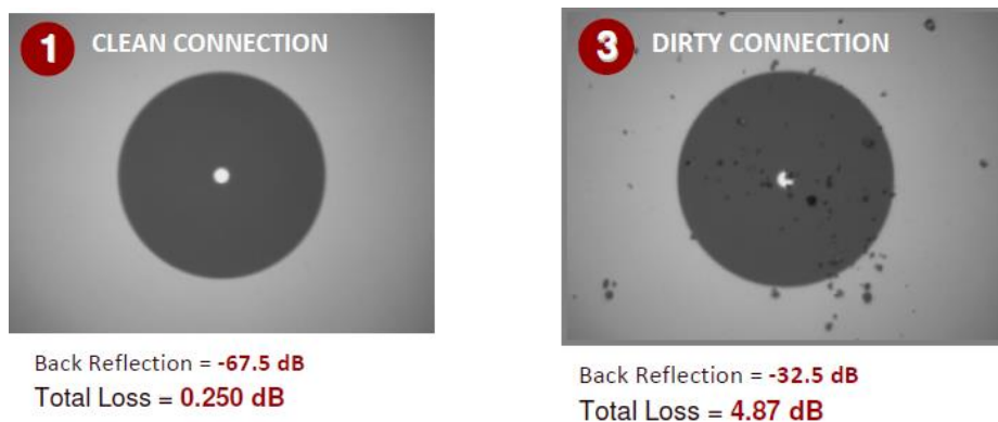
Figura 3.13 Fibra óptica limpia y contaminada.
