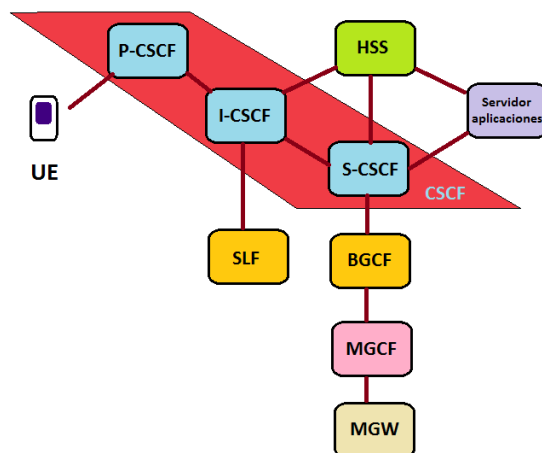
Figura B.4 Arquitectura IMS.
