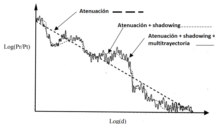
Figura A.13 Comportamiento del canal inalámbrico.
