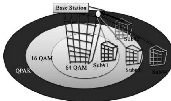
Figura B.16 Utilización de modulación adaptativa por LTE.
