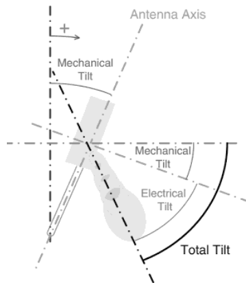
Figura 3.20 Tilt total de una antena.
