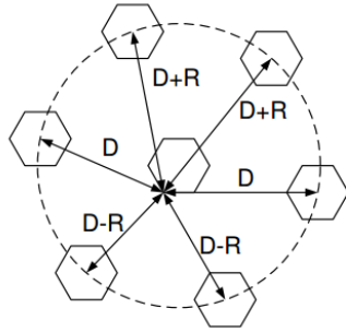
Figura A.9 Segunda fórmula de Lee de interferencia co-canal.
