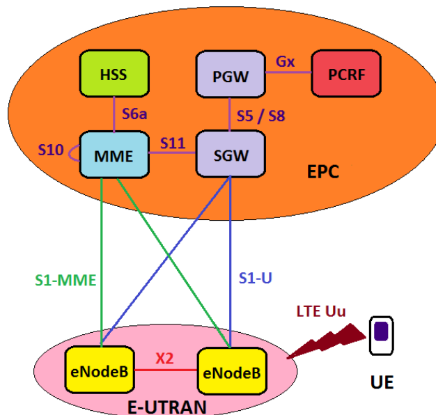
Figura B.1 Arquitectura de la tecnología LTE.
