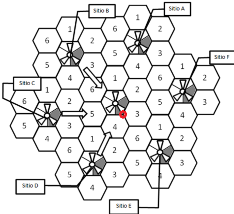
Figura A.12 Método de sectorización para un clúster de factor de reúso 7.
