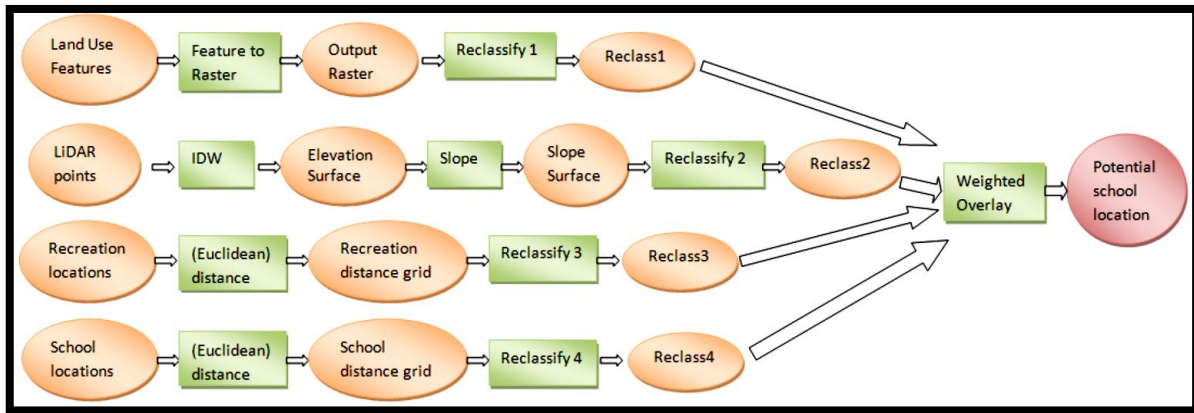
Figura 5. Modelo de geoprocésamiento complejo para el análisis de localización de una escuela (Zhiwei Cao, 2016).
