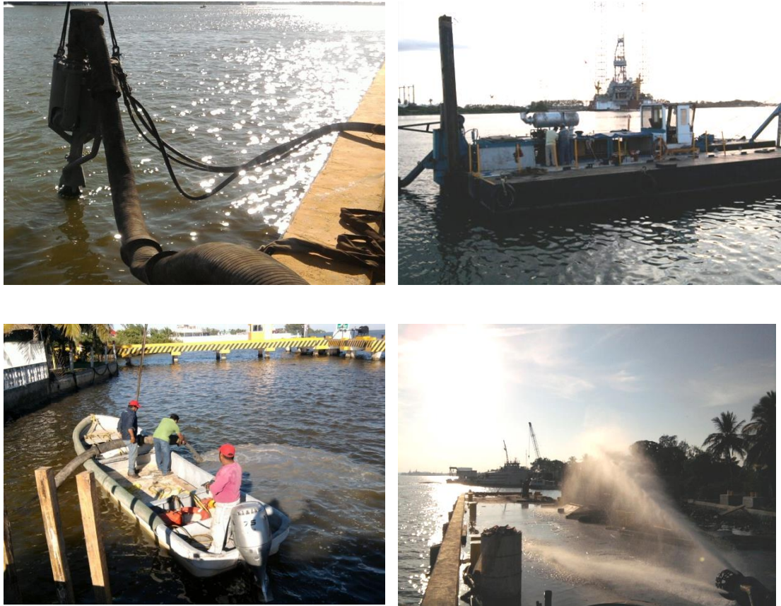
Imagen No.160.-Draga hidráulica de succión, probando el sistema de inyección de agua a presión (bomba tipo JET) y descarga del material producto del dragado, realizadas en las áreas de la dársena y maniobras para el buque oceanográfico, en el río Tuxpan.
