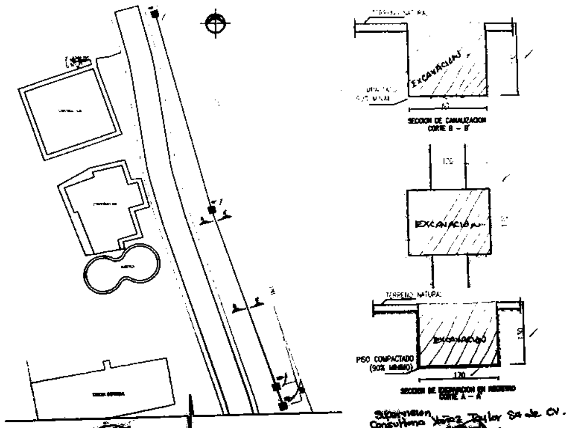
Imagen No.187.- Planta y secciones de la trayectoria de las canalizaciones para la acometida de la subestación eléctrica al muelle.
