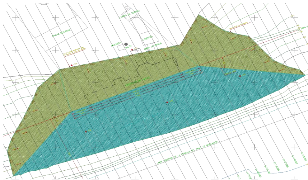
Imagen No.155.- Planta general del dragado en la dársena y áreas de maniobras del buque.
