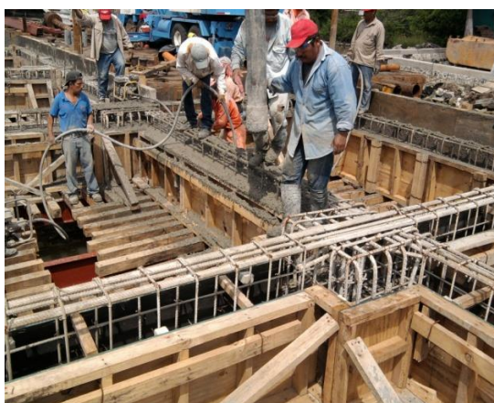
Imagen No.116.- Colocación de concreto (colado) en pilotes, cabezales y traveses entre los ejes del 6 al 1 y del D a G, del muelle.
