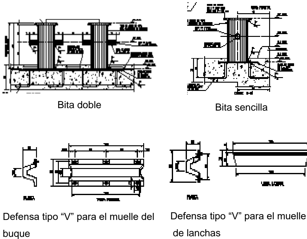
Imagen No.16.- Equipamiento para el atraque y amarre del buque "Justo Sierra".
