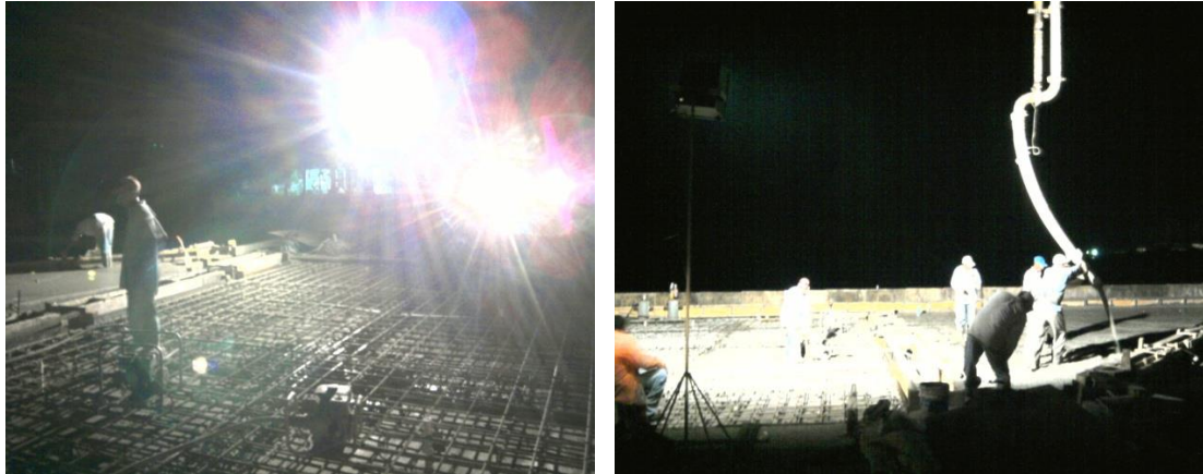
Imagen No.130.- Continuando con el colado de la trabe T-4, guarniciones y losa del muelle, con alumbrado provisional.
