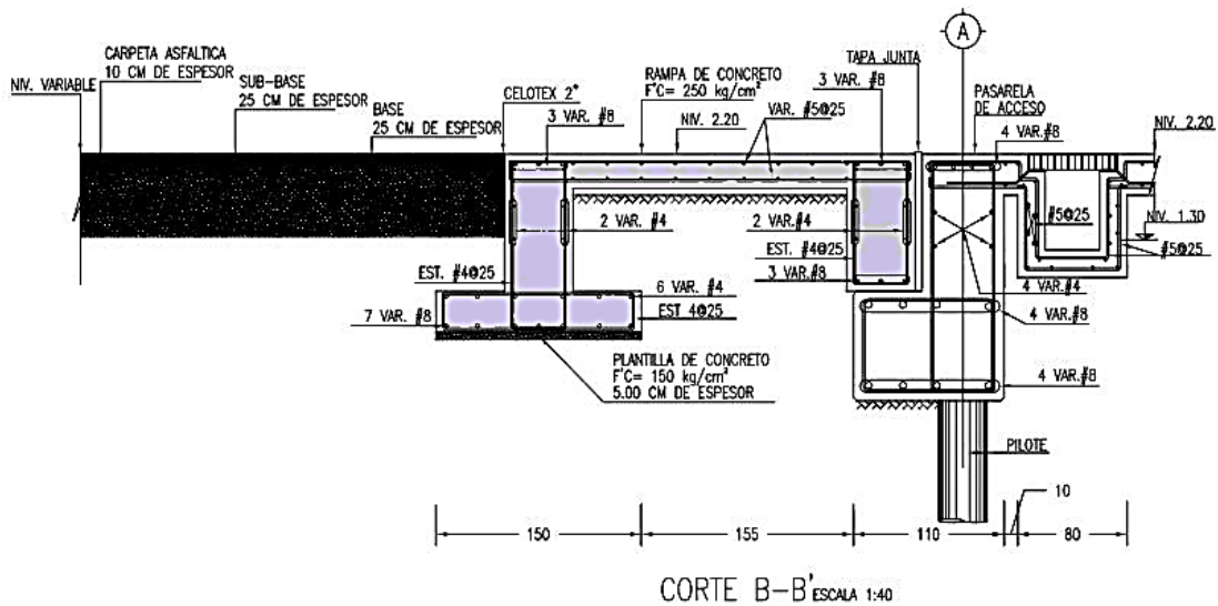
Imagen No.59.- Zapata, traves de la rampa de concreto acceso al muelle.
