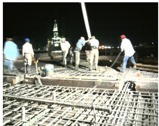
Imagen No.129.- Continuando con el colado siendo las 18:30 hrs., en la trabe T-4, guarniciones y losa del muelle, en el eje 4 al 7 entre G a D.
