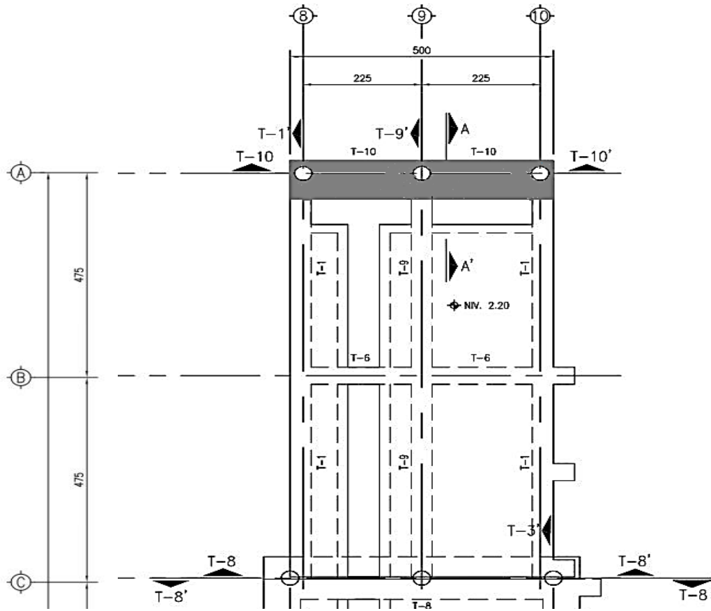
Imagen No.50.- Planta de la cimentación para la Trabe T-10 en eje-A.
