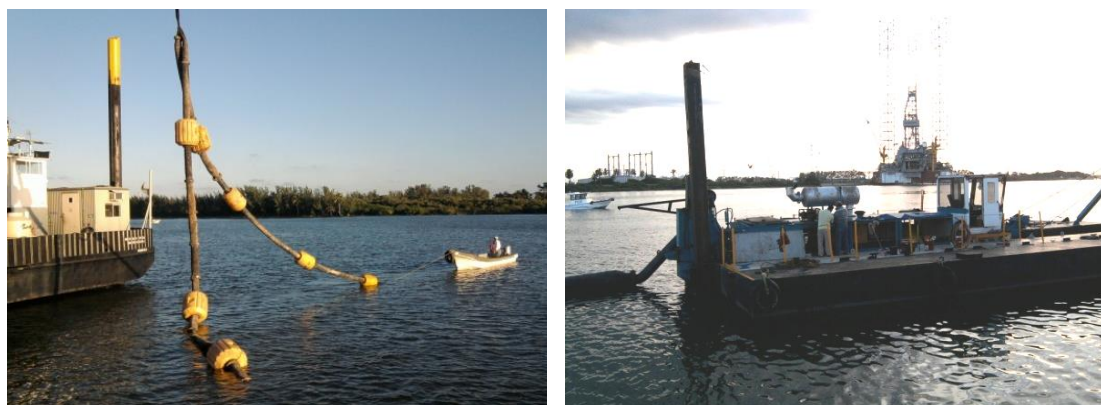
Imagen No.158.- Acoplamiento de la tubería a la draga con apoyo de la grúa y plataforma flotante, en el embalse del rio Tuxpan.
