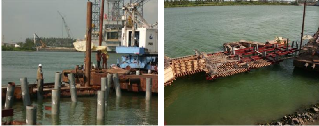
Imagen No.113.- Últimos hincados de pilotes y colocación de la obra falsa, arrastre de polines para la cimbra, habilitados y armados de los pilotes, cabezales y traveses en los ejes 3, 2, y 1 entre los ejes D a G.
