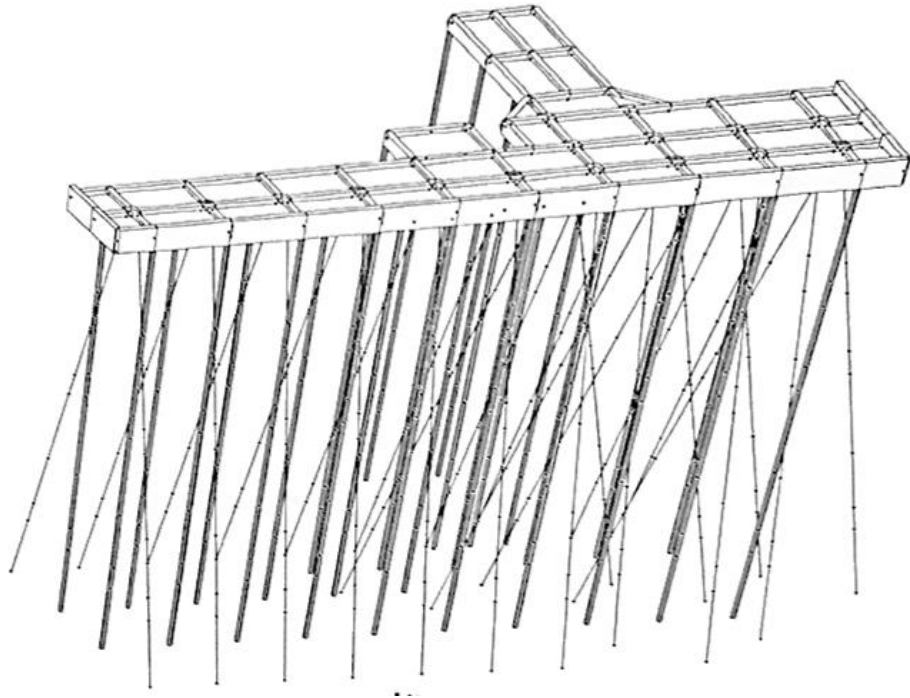
Imagen No.8.- Subestructuras del muelle a base de losa, pantallas, traveses y cabezales de concreto reforzado f'c=250 \text{ Kg/cm}^2 .
