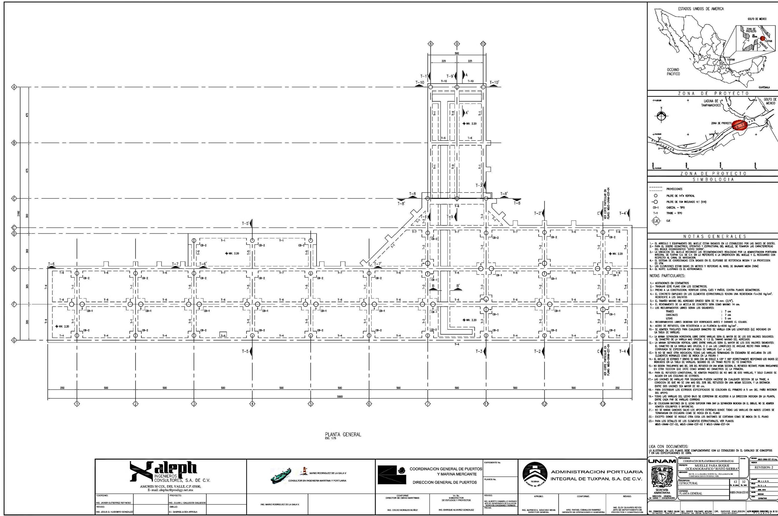
Imagen No.102.- Plano de la planta general de las estructuras (cabezales y traves) de las superestructuras del muelle.
