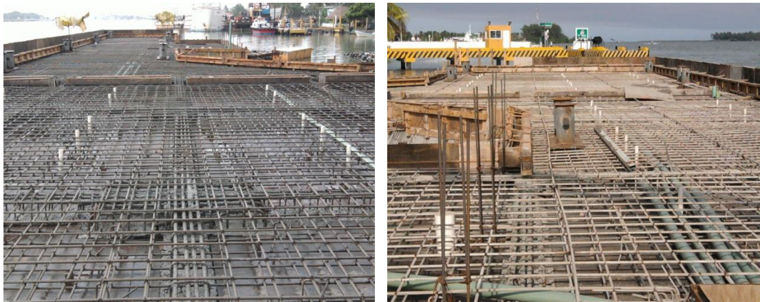
Imagen No.124.- Colocación de drenes pluviales a base de tubería de PVC de 2" de diámetro en la losa del muelle.
