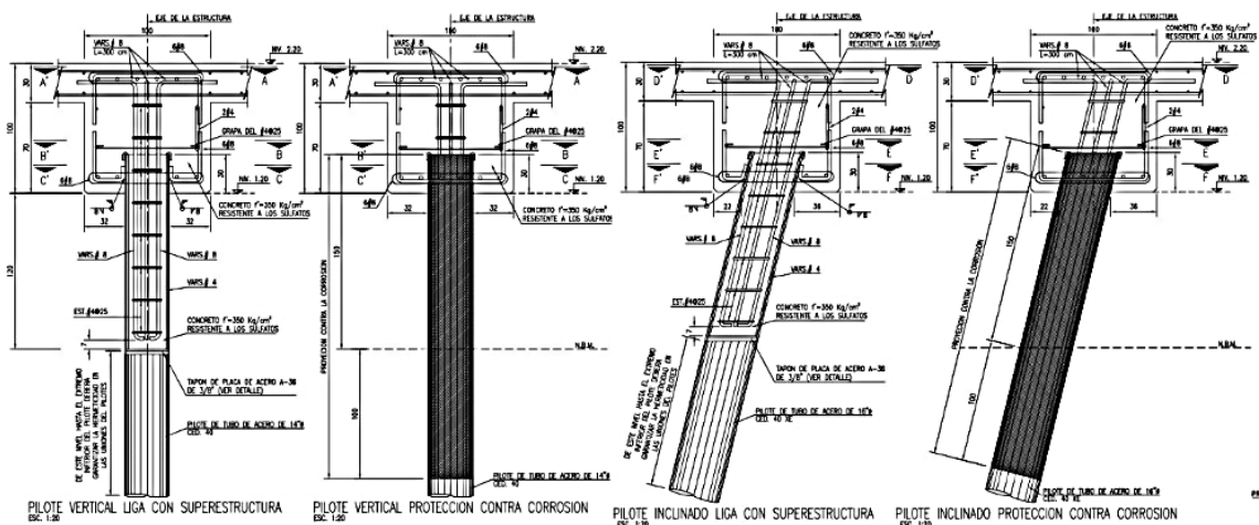
Imagen No.7.- Subestructuras del muelle a base de pilotes verticales(PV) y pilotes inclinados (PI) de tubos de acero de 16" de diámetro de acero A-36.
