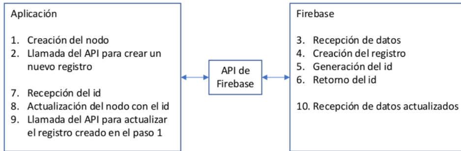
Figura 3.51 Comunicación de la Aplicación con Firebase en la Creación de un Reigstro
