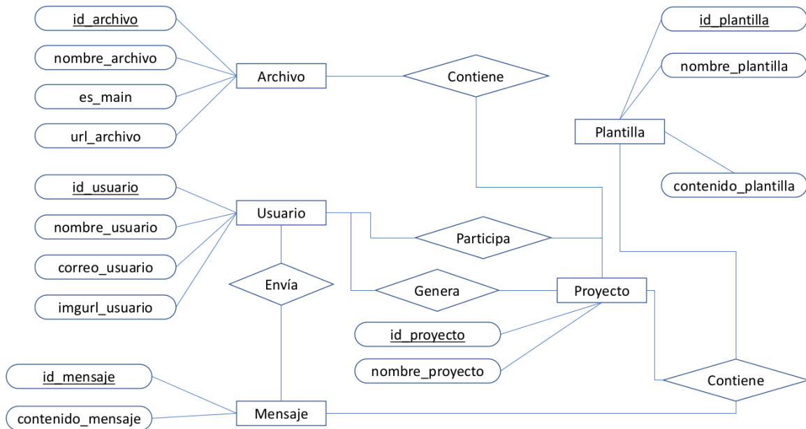
Figura 2.1 Diagrama Entidad-Relación y sus Atributos
