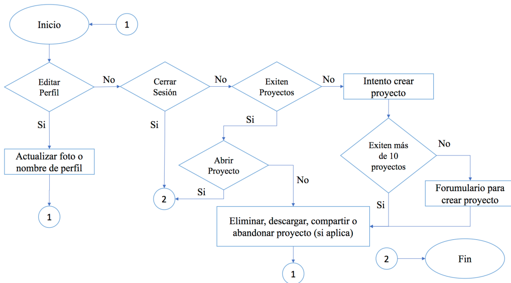
Figura 2.6 Diseño Procedimental Consola de Proyectos
