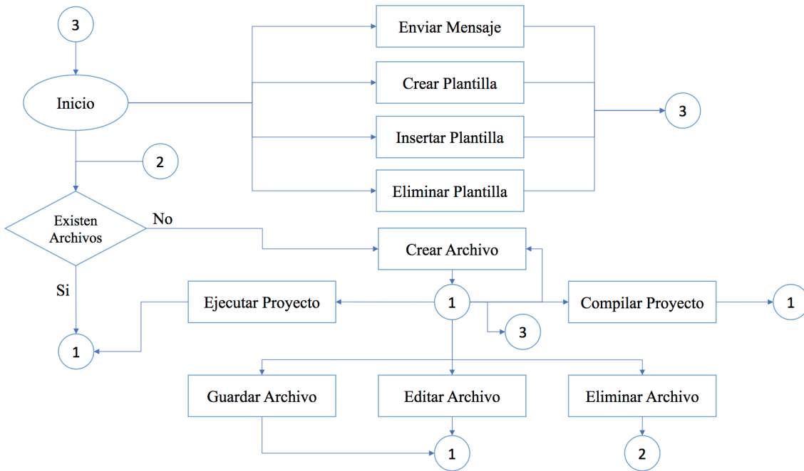
Figura 2.7 Diseño Procedimental Área de Trabajo
