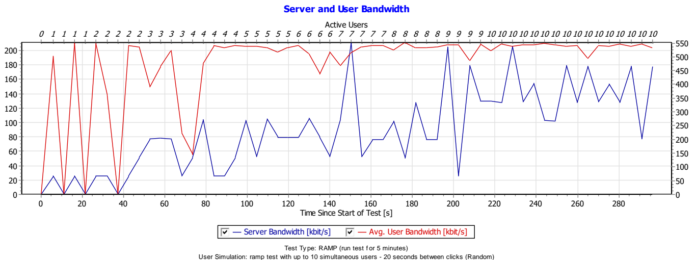
Figura 6.5 Ancho de banda del servidor y el cliente.
