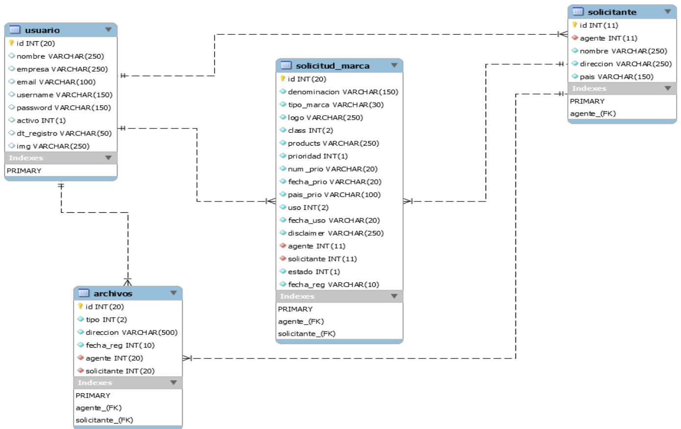
Fig. 4.6 Modelado de datos, modelo relacional de la base de datos de tres tablas del prototipo de “ABLEIP”.
