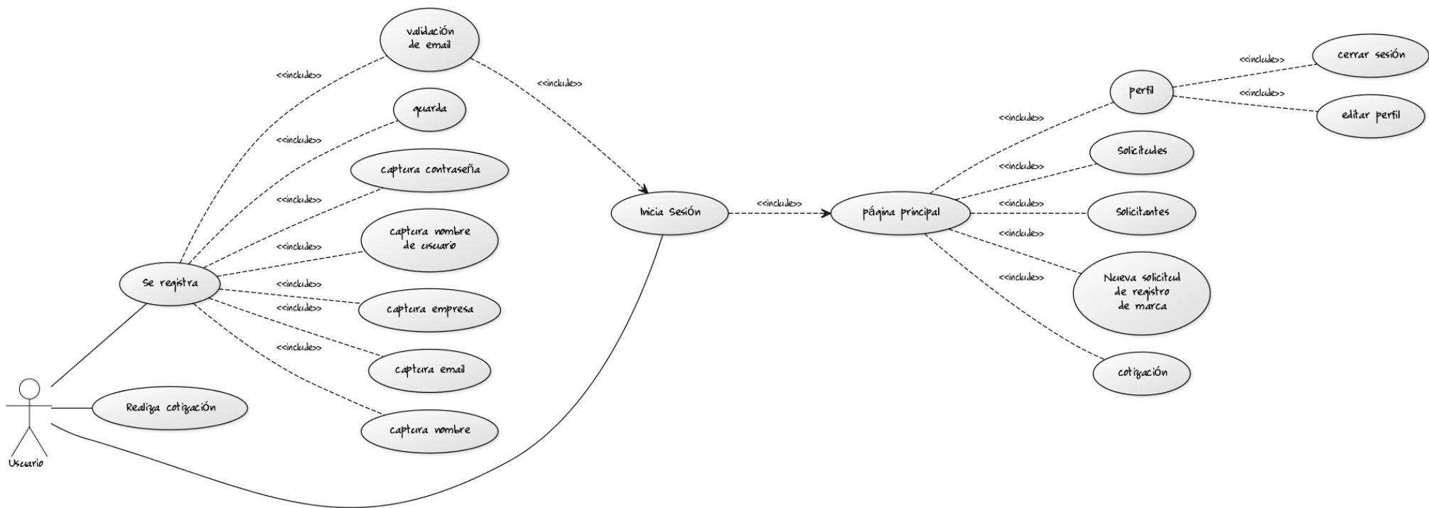
Fig 4.5 Caso de uso de las posibles formas de la primera interacción con el sistema.
