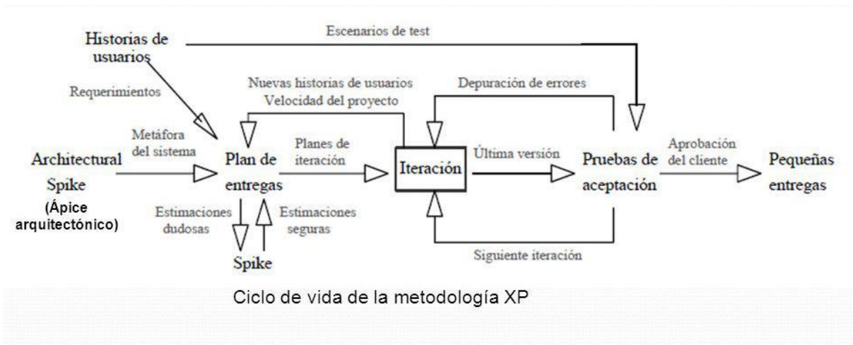
Fig. 3.8 Representación de la metodología de XP.
