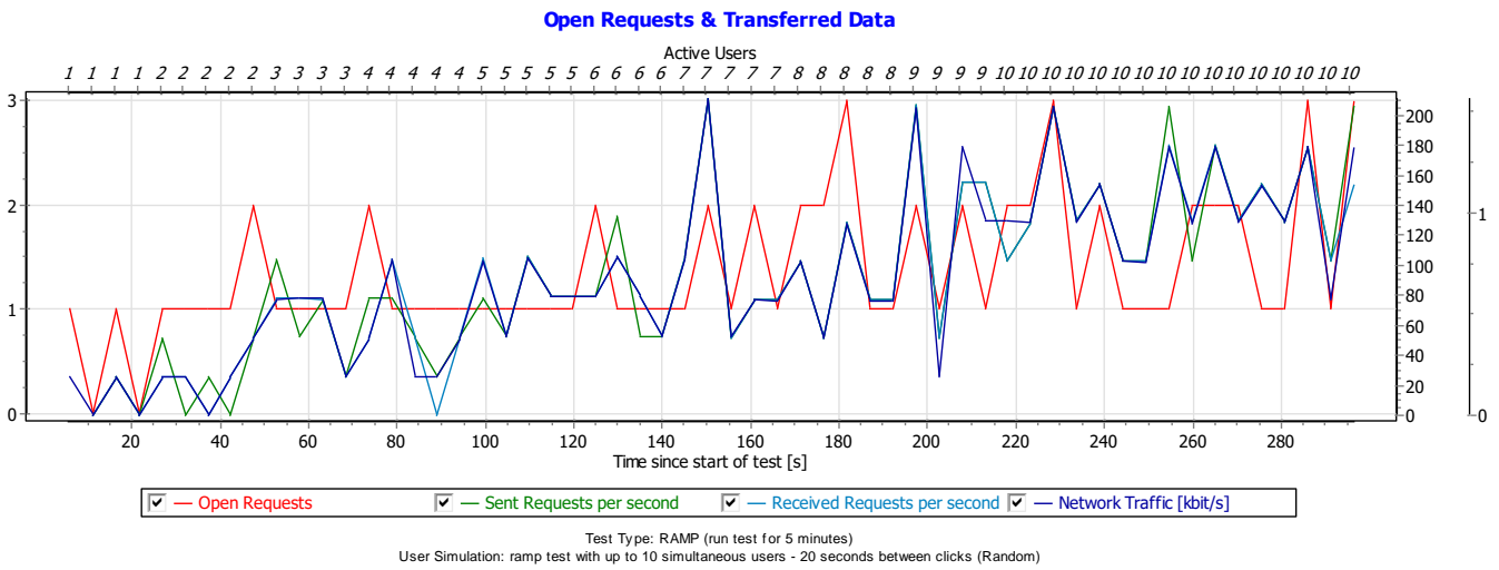
Figura 6.7 Datos transferidos y solicitudes (POST, GET).
