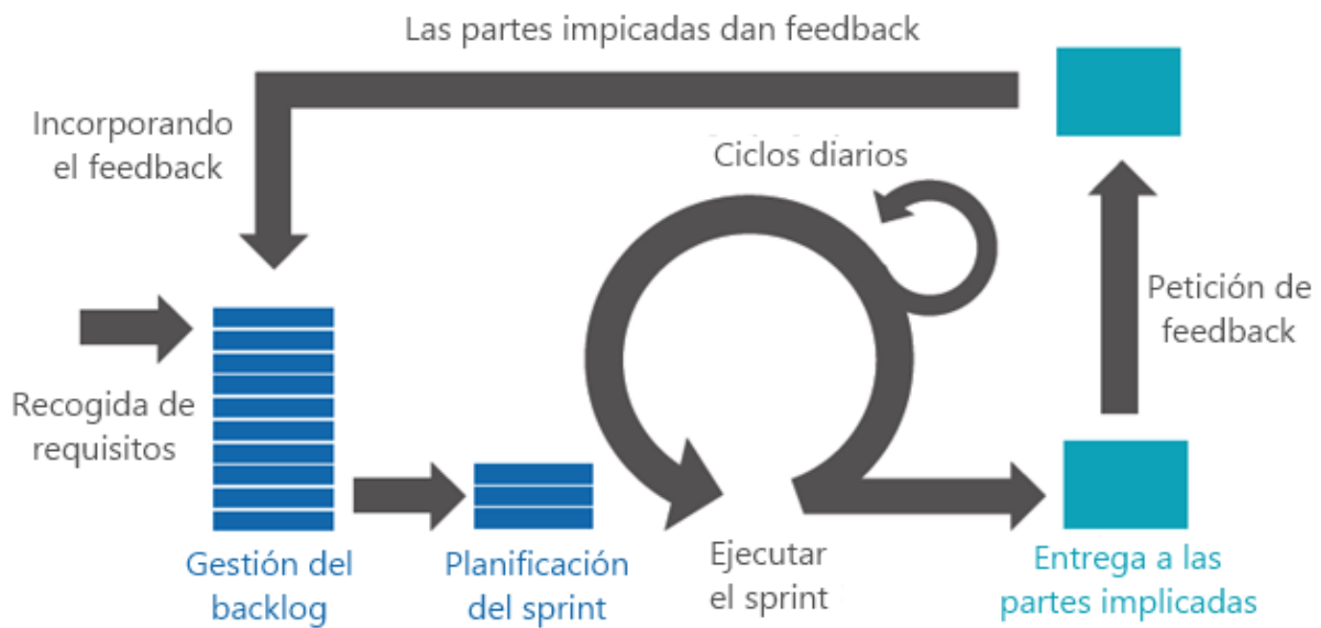
Fig. 3.6 Representación de la metodología de Scrum.
