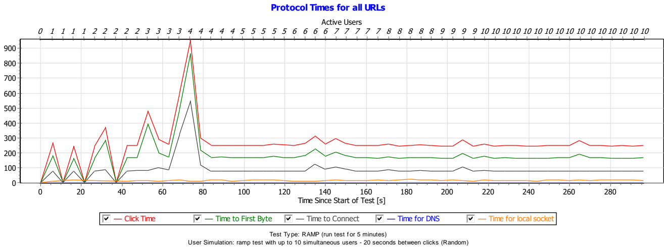
Figura 6.4 Gráfica de tiempos de conexión y respuesta.
