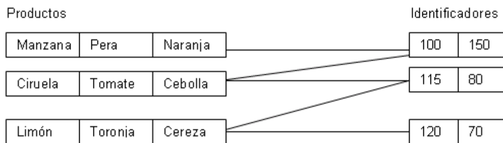
Fig. 3.13 Representación de la base de datos en red.
