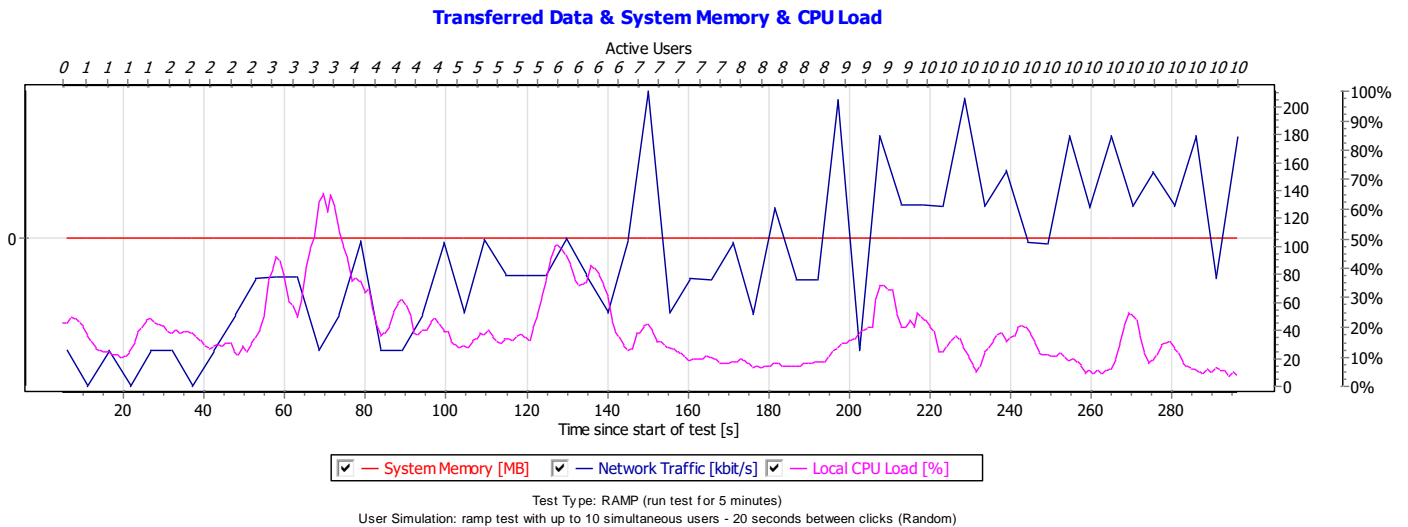
Figura 6.6 Datos transferidos, carga del CPU y de la memoria.
