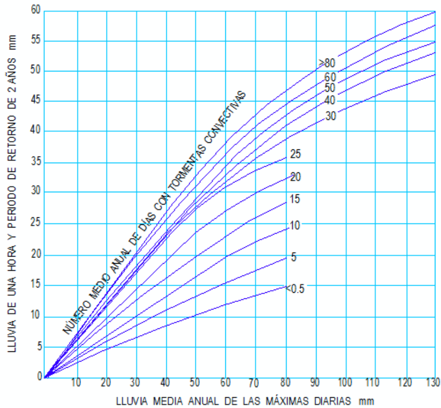
Figura 1-1 Obtención de la lluvia Hp_{T=2\text{años}}^{1\text{hora}} (SARH, 1982)
