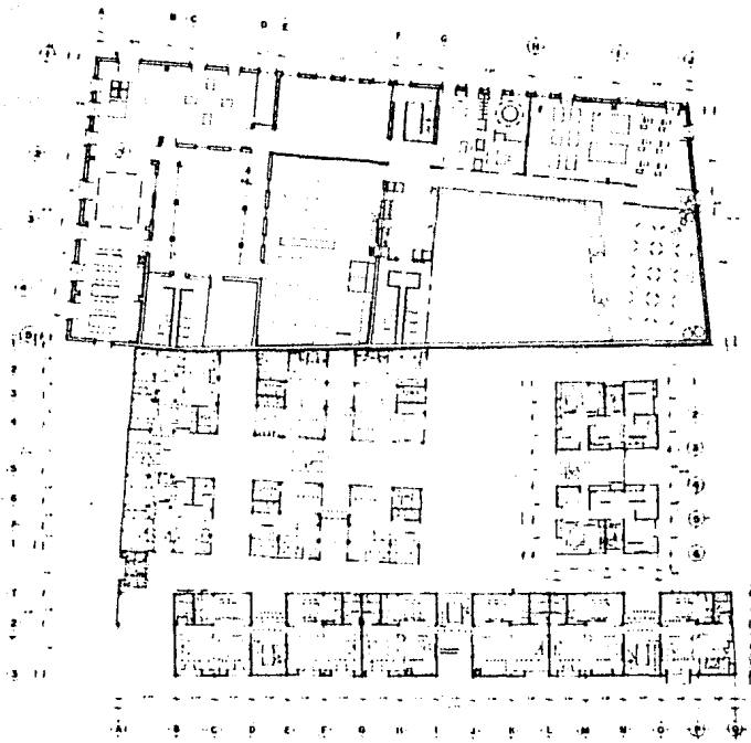
PLANTA ALTA ARQUITECTONICA
