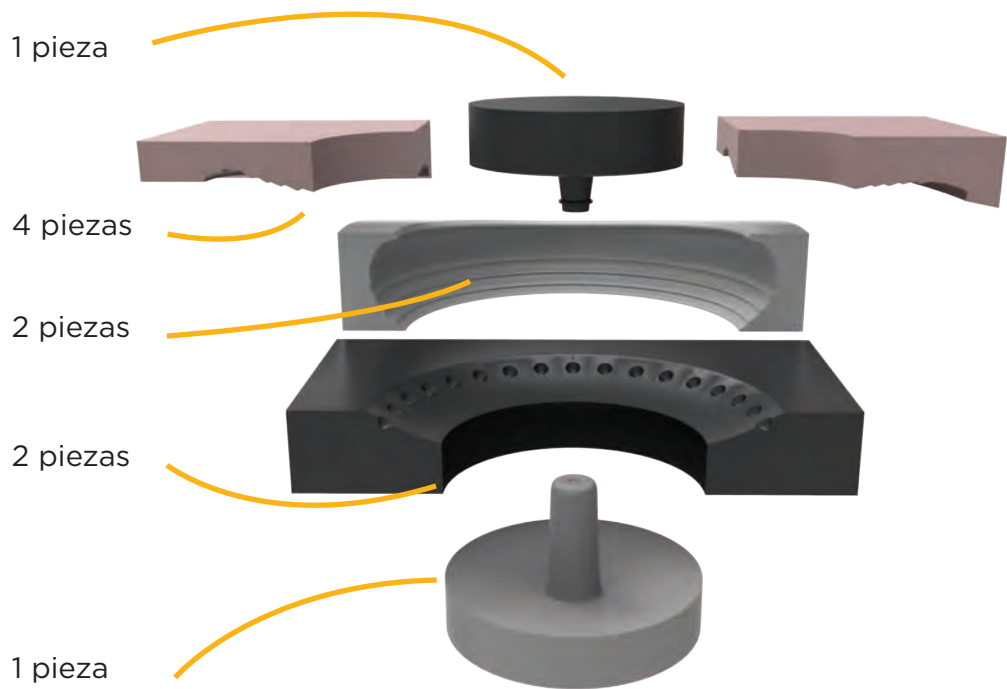
Esquema 25 Adevedo TM (2017) Molde de diez piezas en fundición de aluminio.
