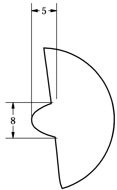
DETALLE J ESCALA 2 : 1
