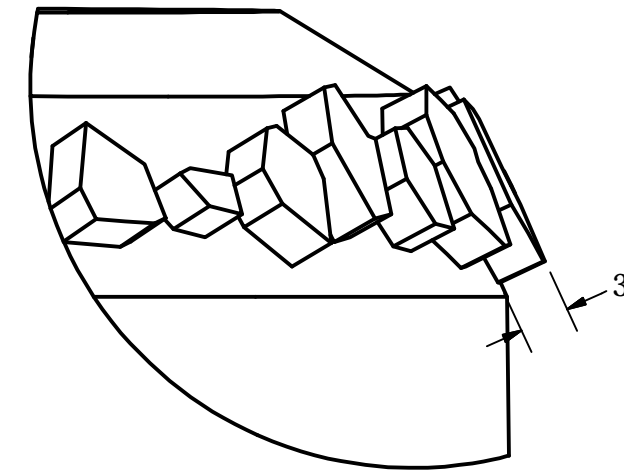
DETALLE M ESCALA 2 : 1
