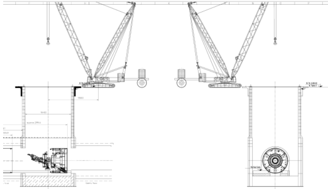
Fig. 3.20. Se ensambla en su sitio el transportador helicoidal o mejor conocido como tornillo sinfín, este ya se encontraba en el fondo de la lumbrera pero por cuestiones de logística y de espacio, se deja a un lado mientras los pasos 2 al 8 transcurren. De esta forma queda armado el escudo de la TBM. 103
