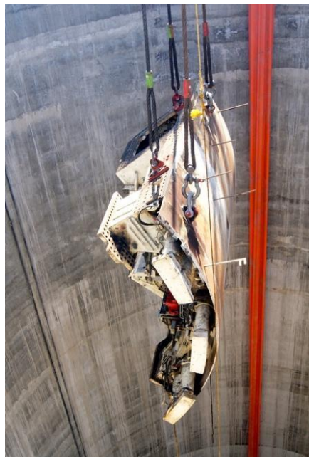
Fig. 2.7. Introducción de las partes de una TBM a una galería de montaje. 63
