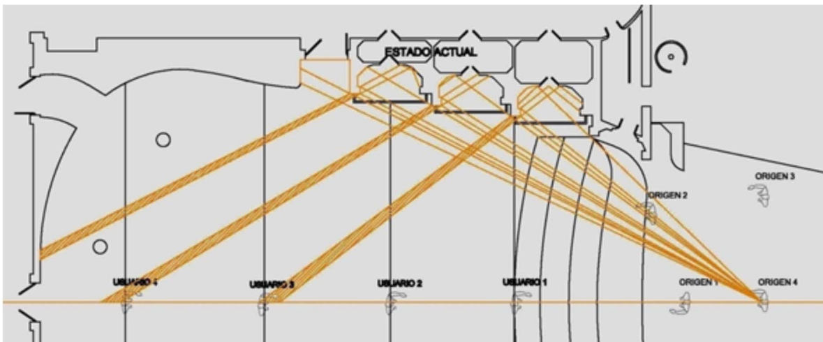
Fig. 5. Reflecto-grama teatro estado actual.
