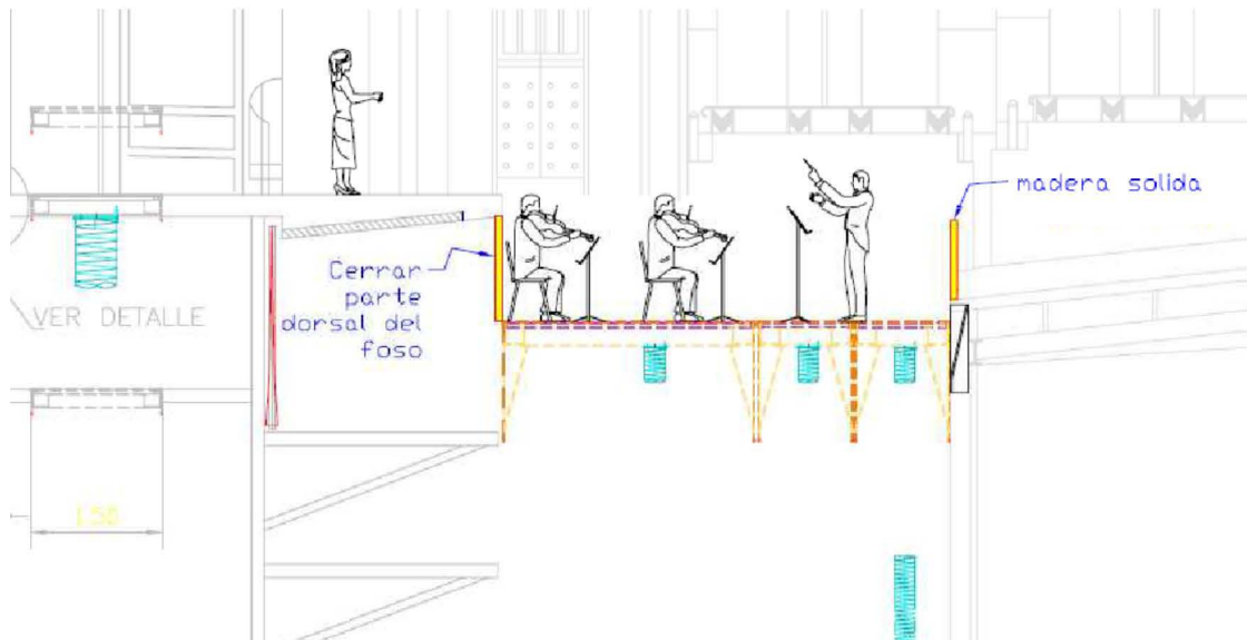
Figura 47. Corte usando solo las plataformas móviles cubriendo la parte frontal y trasera con madera sólida.
