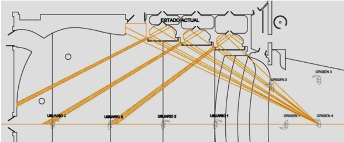
Fig. 14. Reflecto-grama teatro estado actual.
