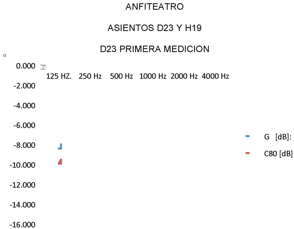
Figura 74. G, C80 asiento D23
