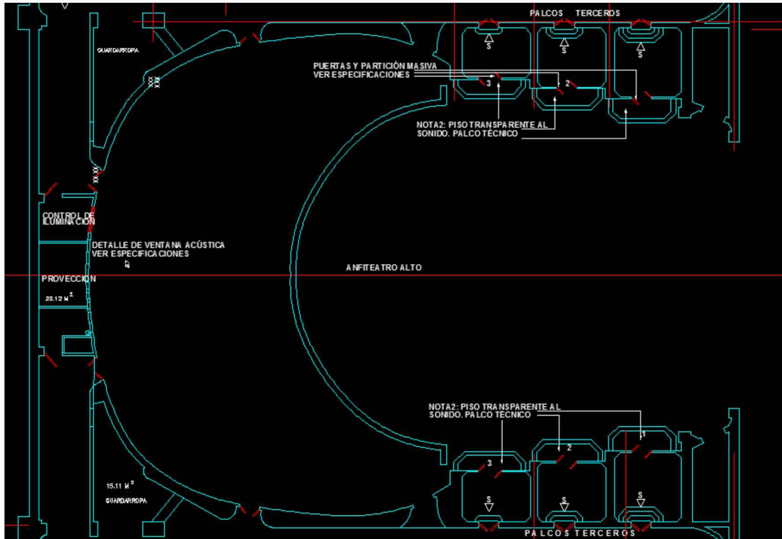
Figura 50. Palco 2º. Balcón Cambios sugeridos.
