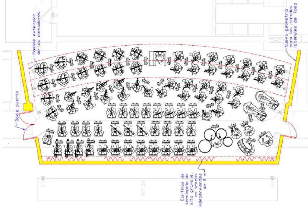
Figura 45. Configuración Foso de Orquesta para orquesta de 89 elementos
