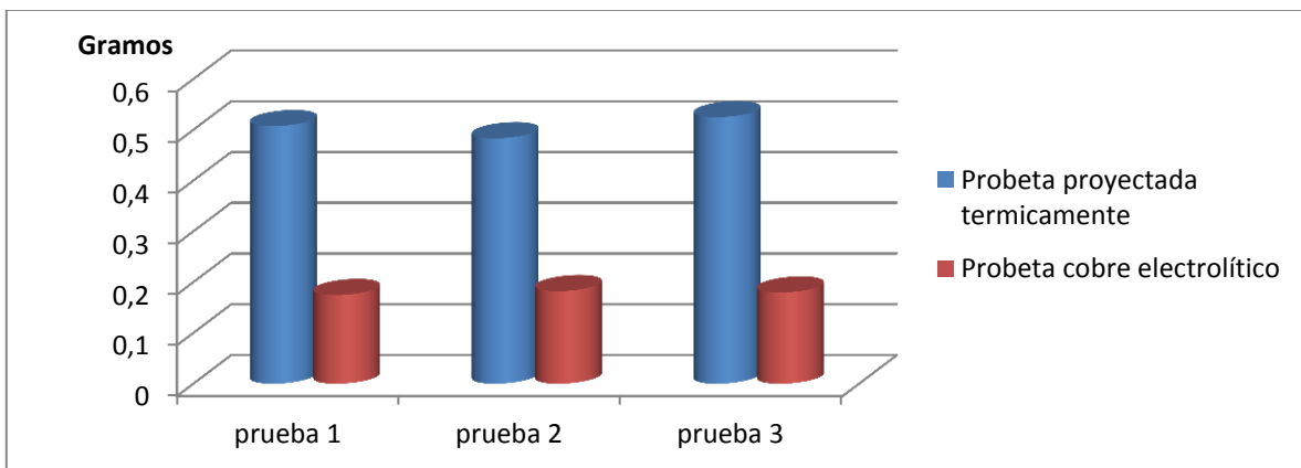
Gráfica 3.2. Comparativa pérdida de masa después de electroerosión en gramos.
