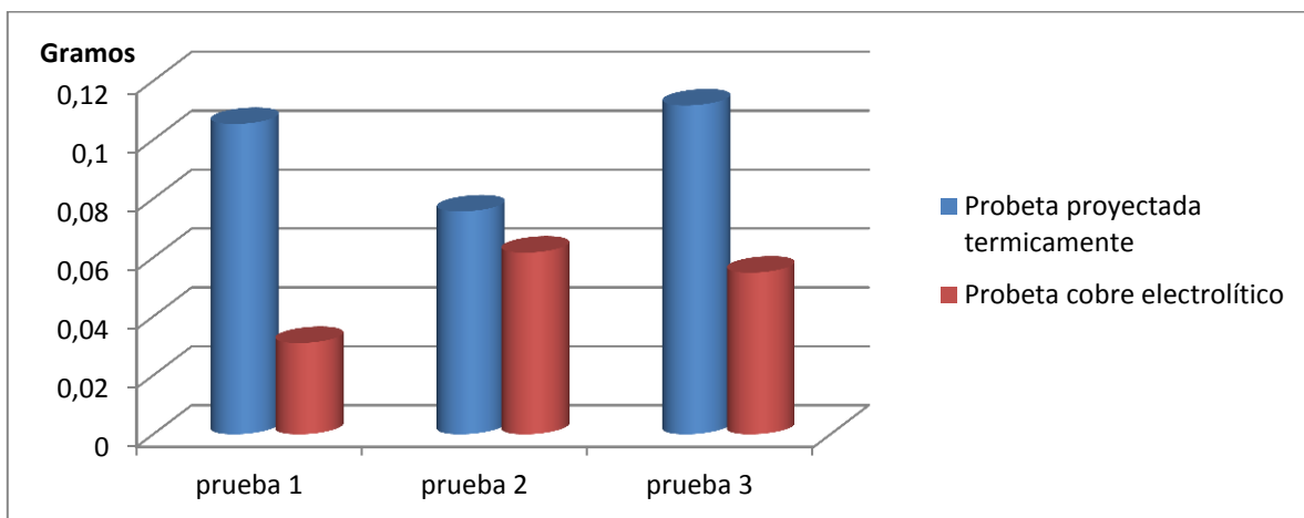
Gráfica 3.6. Comparativa pérdida de masa después de electroerosión en gramos.
