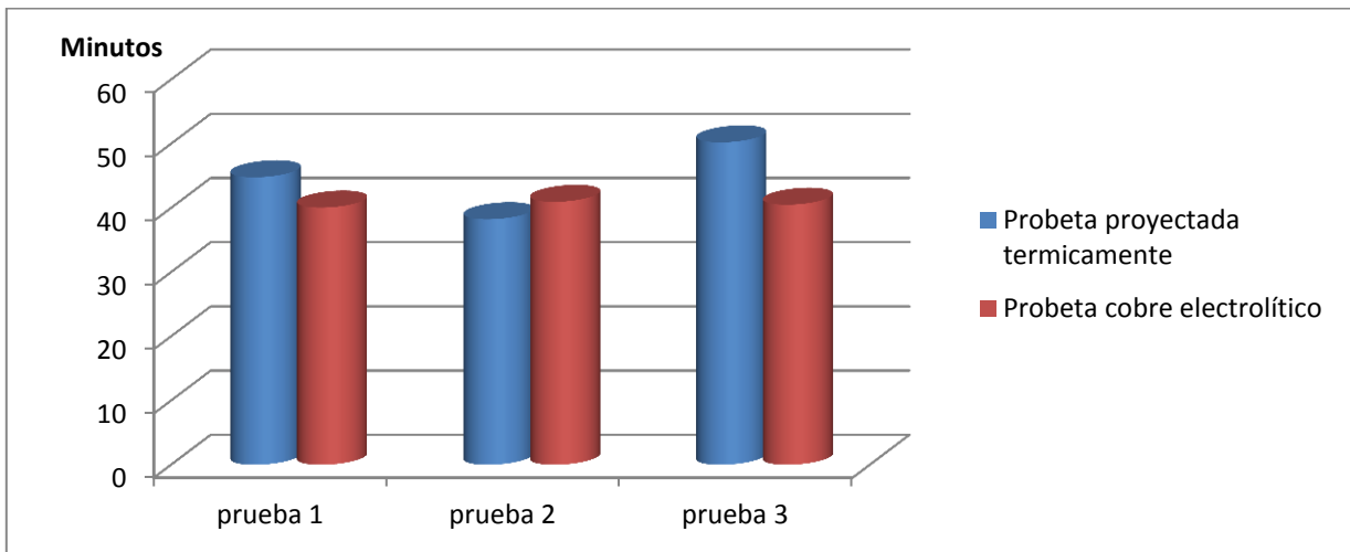
Gráfica 3.1. Comparativa Tiempo de electroerosión en minutos.
