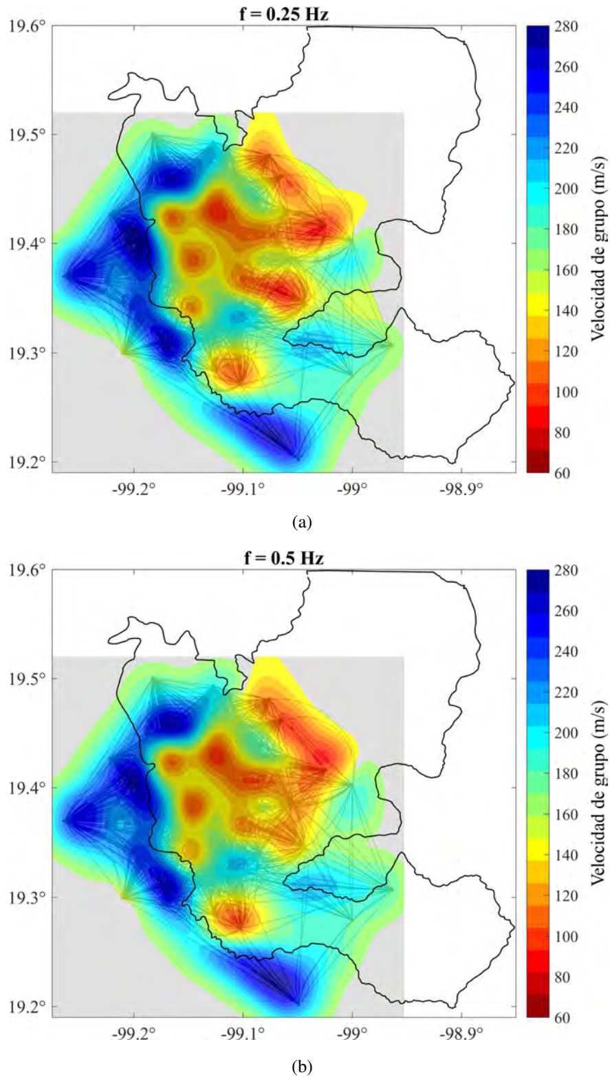
Figura 5.12: Tomografías sísmicas de las velocidades de grupo de las ondas de Rayleigh en el Valle de México, para las frecuencias: (a) 0.25 Hz, y (b) 0.50 Hz. La distribución de las estaciones se observa en el fondo con puntos negros, al igual que los trayectos entre pares de estaciones con líneas. La línea negra delinea el límite de los depósitos lacustres, propuesto por Marsal y Mazari (1959).
