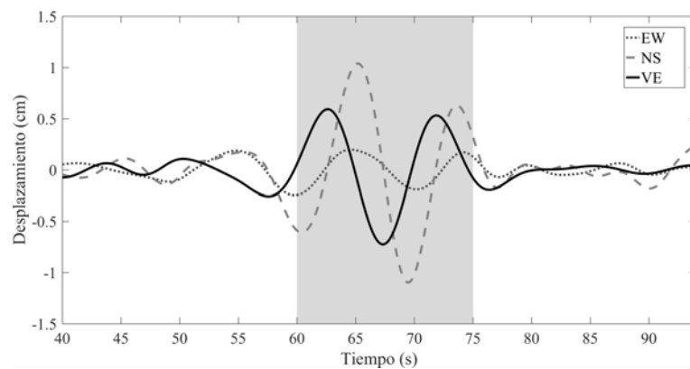
Figura 1.4: Desplazamientos promedio de los registros de la RACM (55 trazas) del sismo del 25 de abril de 1989, filtrados entre 0.05 y 0.15 Hz. Las líneas punteada gris, discontinua gris y continua negra, corresponden a las dirección Este-Oeste (EW), Norte-Sur (NS) y Vertical (VE), respectivamente. El área sombreada indica la ventana de tiempo que contiene la onda de Rayleigh de 10 s de período.
