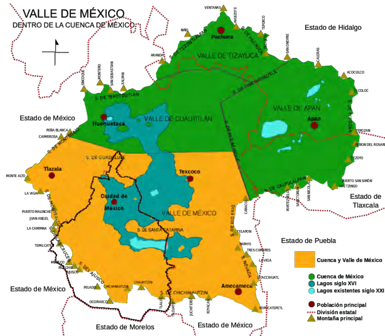
Figura 1: Cuenca de México dividida por los Valles de México, de Cuautitlán, de Apan y de Tiza-yuca. Se muestra el gran lago existente en el siglo XVI conformado por los lagos de Zumpango, Xaltocan, Texcoco, Xochimilco, y Chalco. La línea negra dentro del Valle de México enmarca la Ciudad de México.
