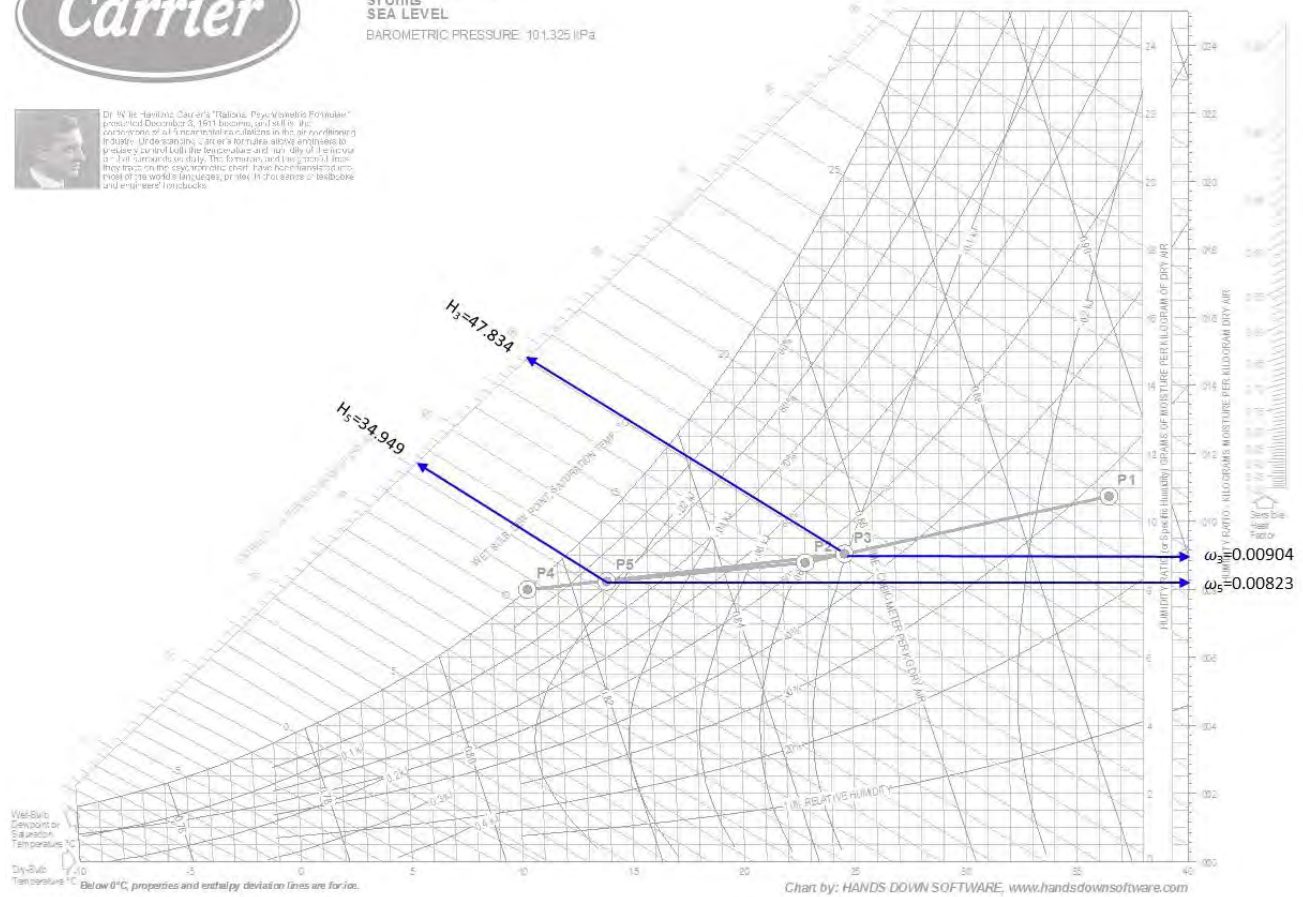
Ilustración 24. Forma gráfica de obtener la humedad y la entalpía de los estados (3) y (5)
