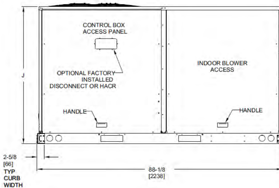
Ilustración 29. Vista frontal del equipo. Fuente: Ficha técnica Unidad tipo Paquete de Carrier
