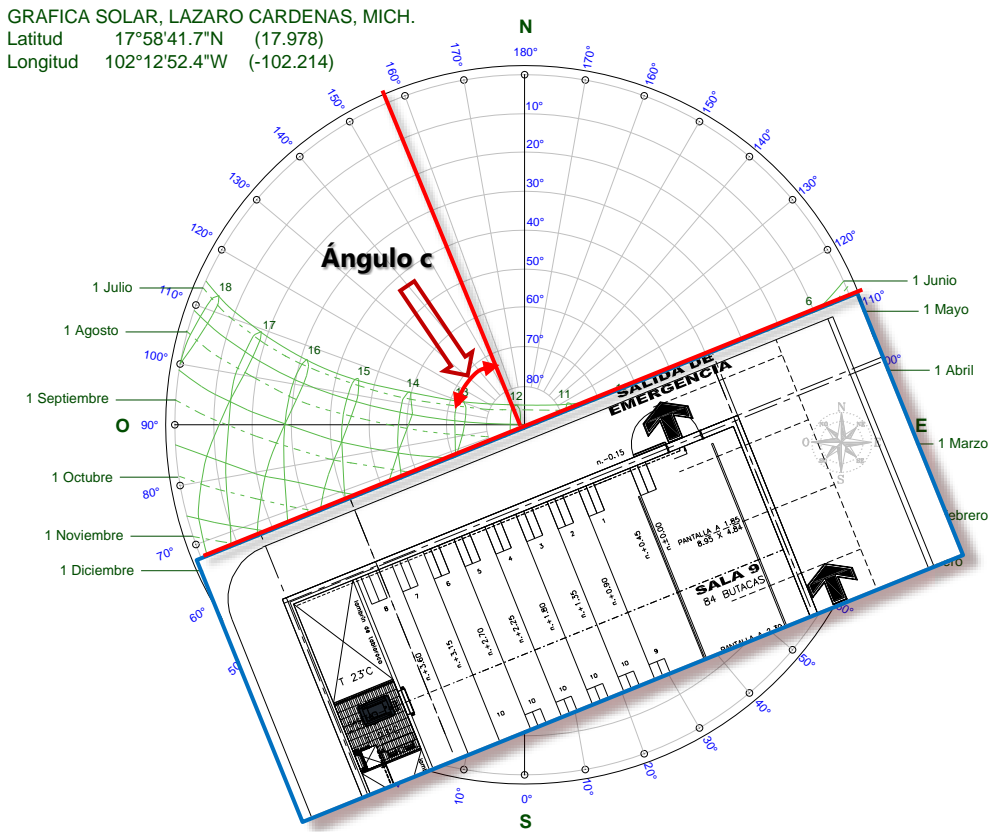
Ilustración 19. Ángulo c en la fachada NO Fuente: Elaboración propia empleando AutoCAD 2016
