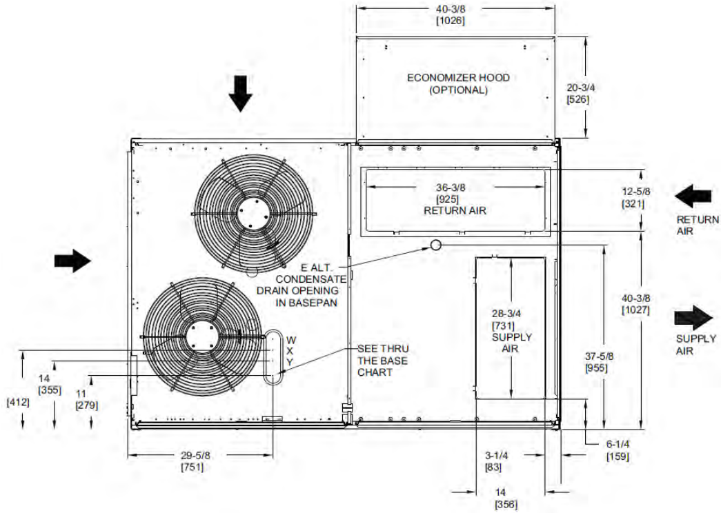
Ilustración 26. Vista superior del equipo.
