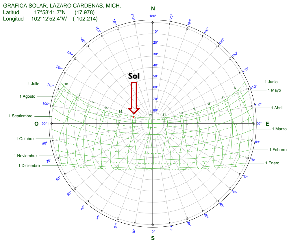
Ilustración 16. Gráfica solar con la ubicación del sol el 21 de julio a las 13:00 h.
