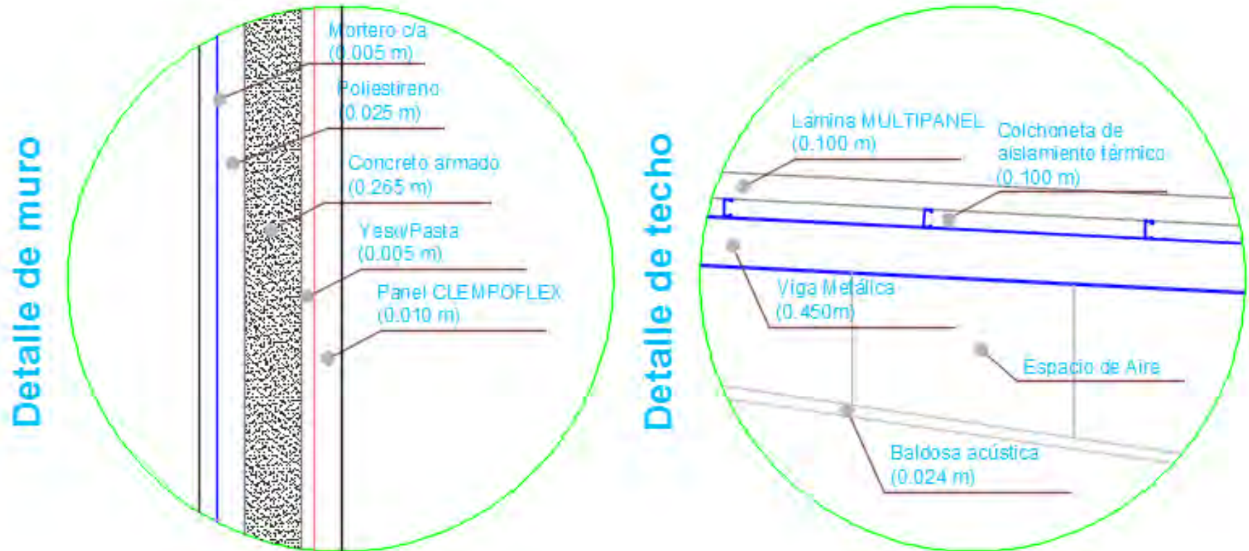
Ilustración 11. Detalle de la composición del muro y del techo.
