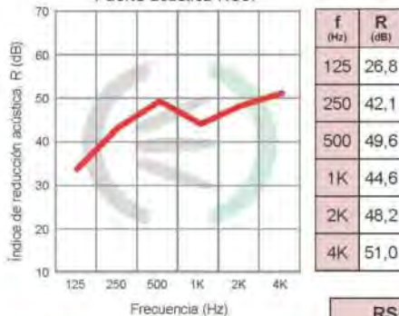
Puerta acústica RS5F
