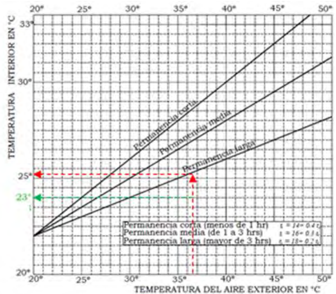
Ilustración 3. Temperaturas interiores recomendables para verano en función de la temperatura de cálculo exterior.
