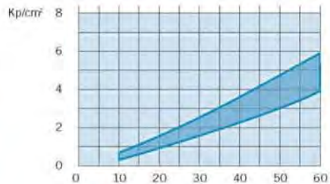
Resistencia a la compresión de la espuma rígida de Poliestireno con un 10% de deformación (campo de dispersión).
