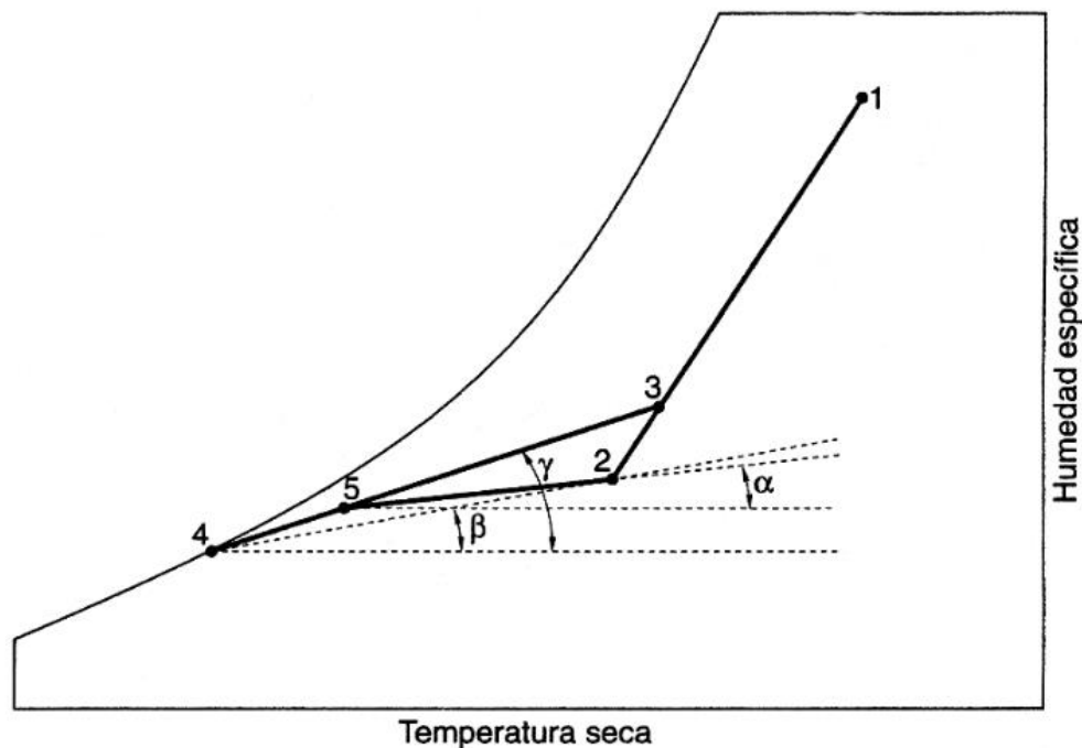
Ilustración 21. Representación gráfica del proceso típico de acondicionamiento en verano.
