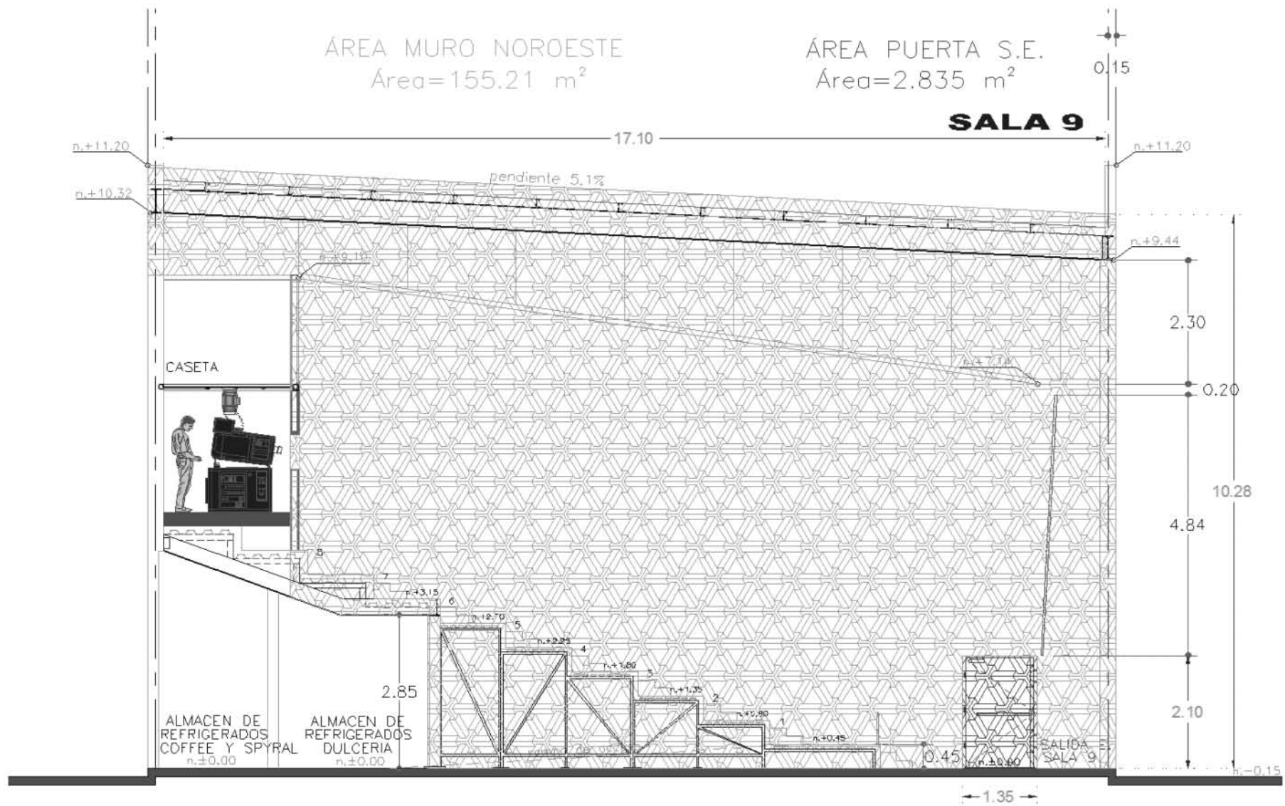
Ilustración 9. Detalle del Área del muro Noroeste Fuente: Elaboración propia empleando AutoCAD 2016
