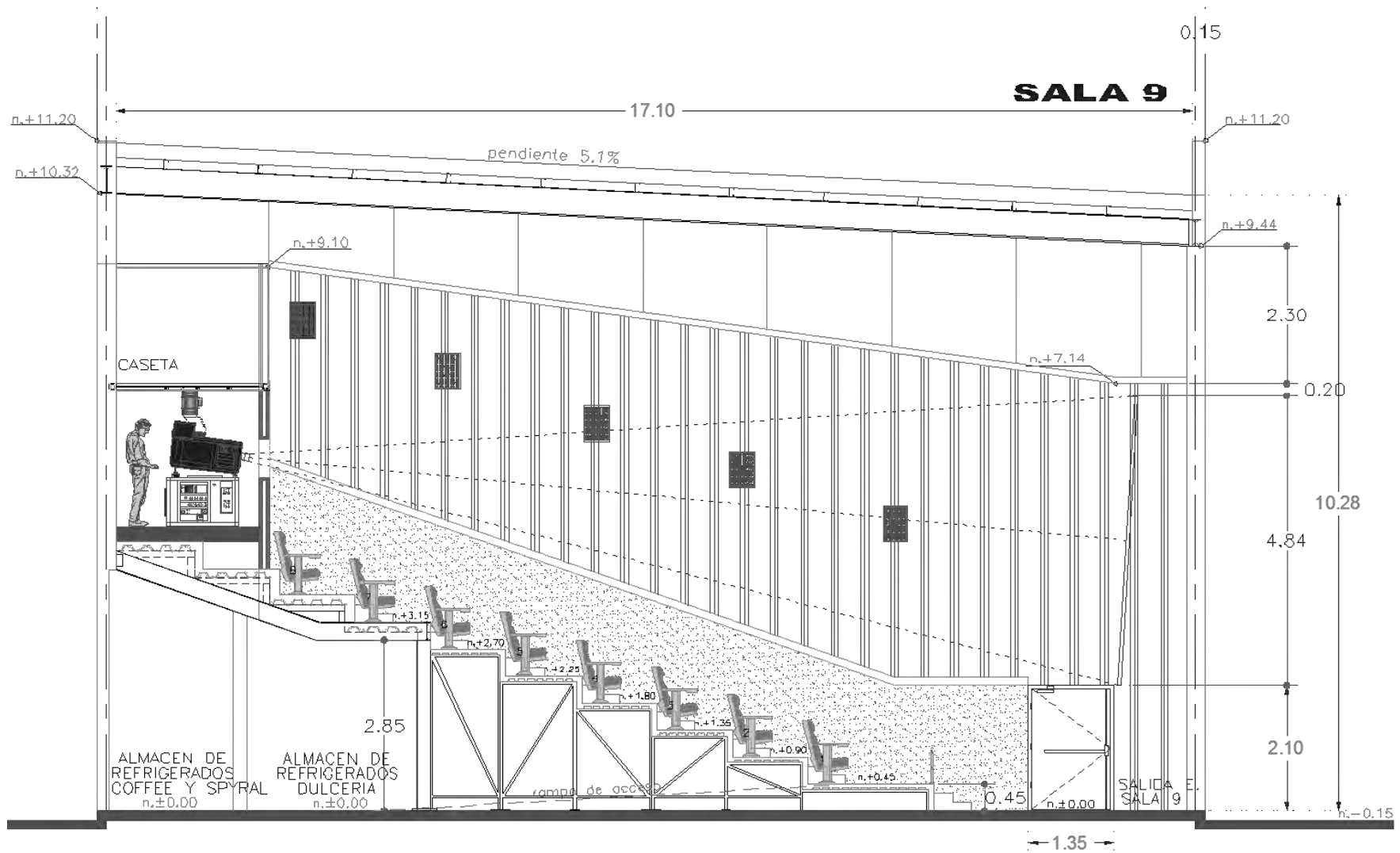
Ilustración 7. Corte longitudinal C-C; Sala 9 Fuente: Elaboración propia empleando AutoCAD 2016
