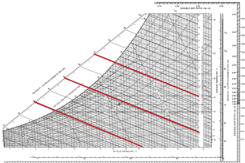
Ilustración 38. Líneas que representan la entalpía en la carta psicrométrica.
