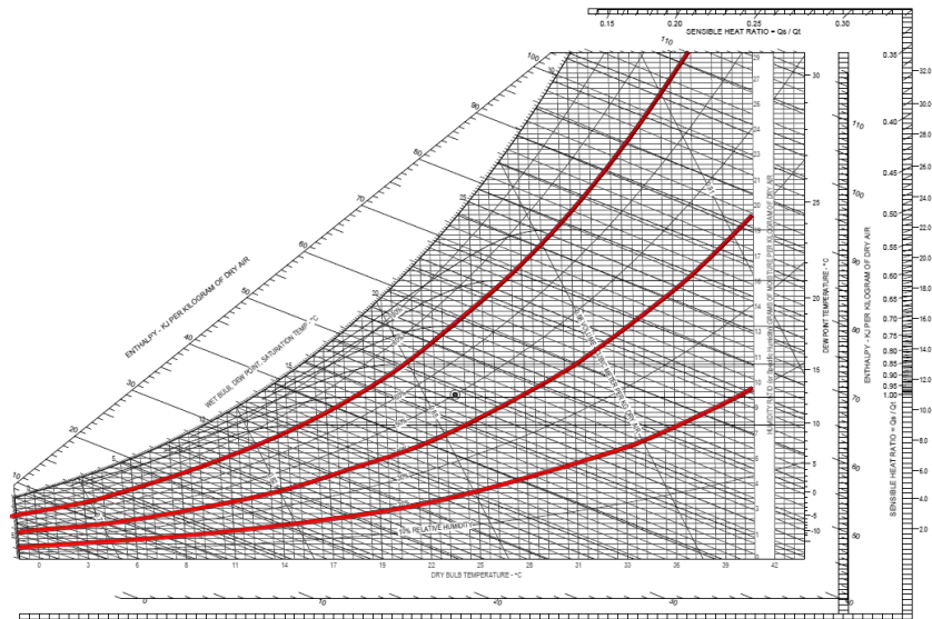
Ilustración 36. Líneas que representan la humedad relativa en la carta psicrométrica
