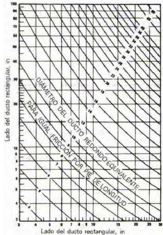
Ilustración 31. Diámetros de ductos redondos equivalentes
