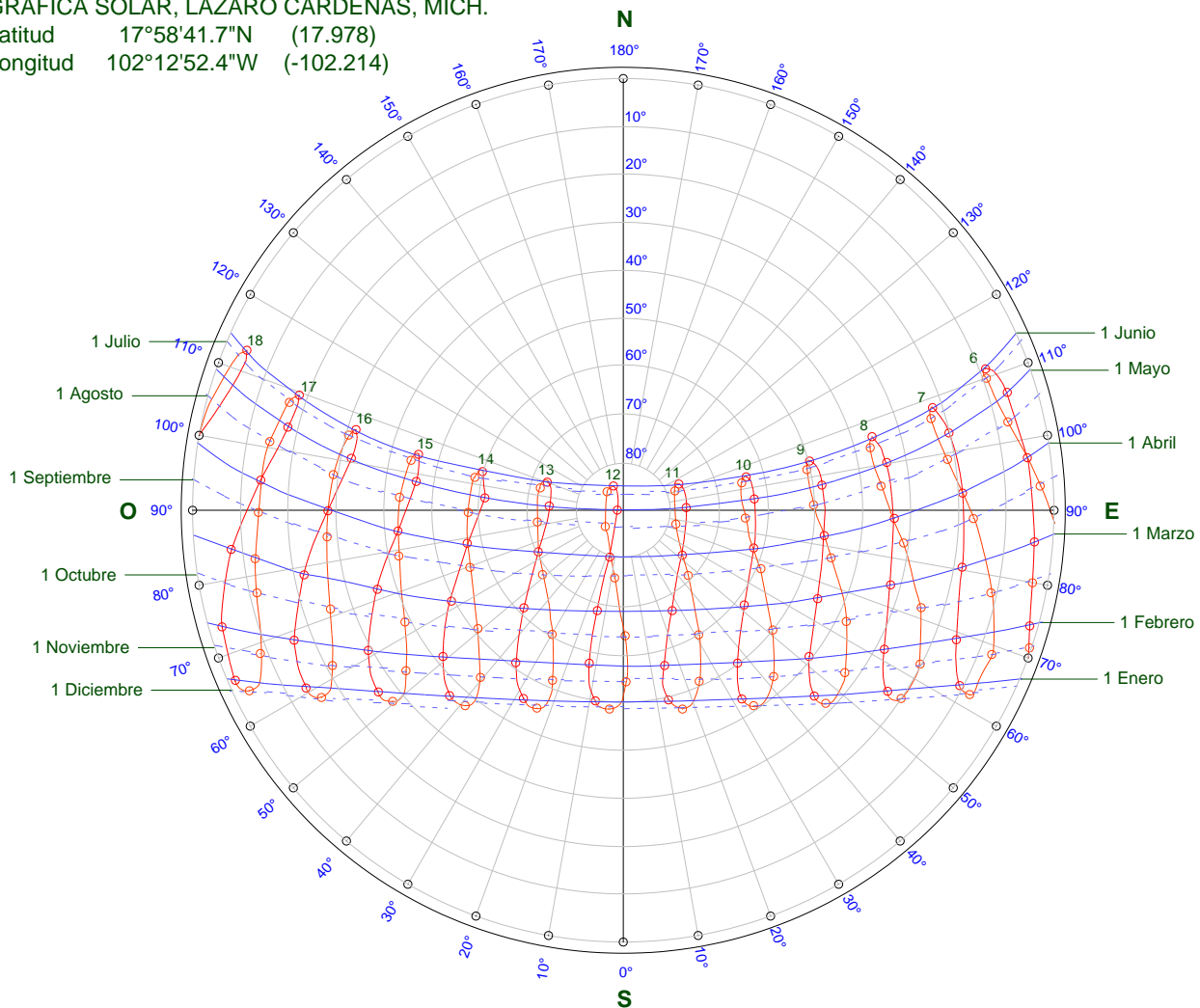
Ilustración 13. Gráfica solar equidistante de la ubicación del Cine.
