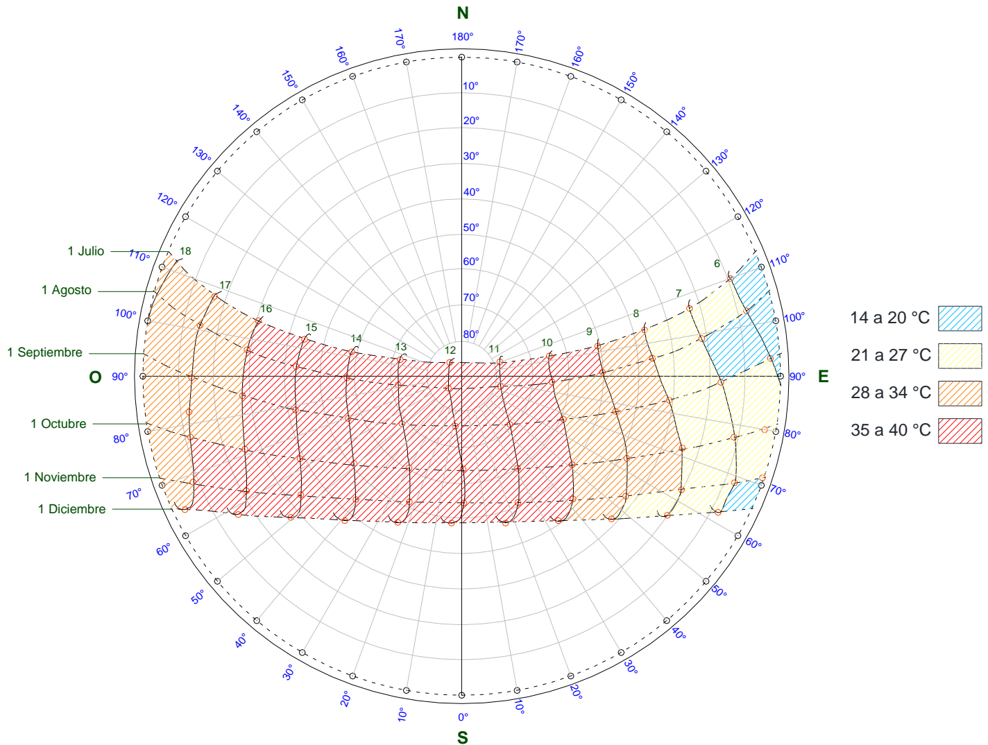
Ilustración 15. Gráfica solar equidistante con sombreado respecto a la temperatura promedio por hora y época del año. (Julio a Diciembre)
