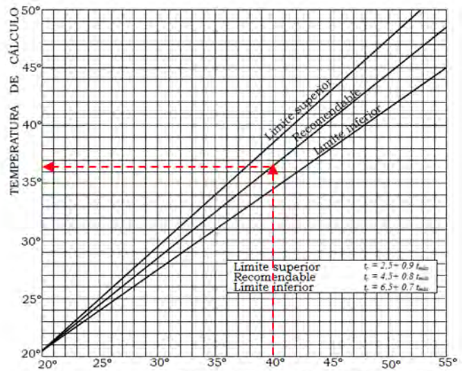
Ilustración 2. Temperaturas de cálculo exterior para refrigeración en función de la temperatura máxima extrema del lugar.
