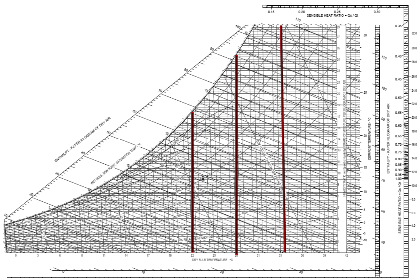
Ilustración 35. Líneas que representan la temperatura de bulbo seco en la carta psicrométrica
