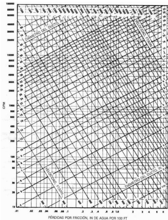
Ilustración 32. Pérdidas por fricción de flujo de aire a través de ductos redondos de lámina galvanizada
