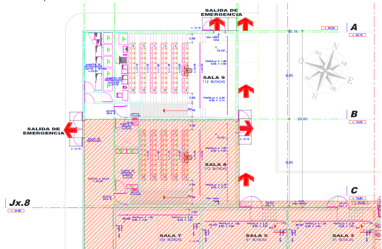
Ilustración 5. Planta general, sala 9; vista de planta.
