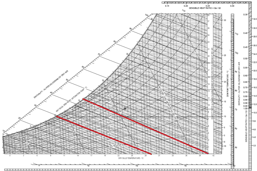
Ilustración 34. Líneas que representan la temperatura de bulbo húmedo en la carta psicrométrica
