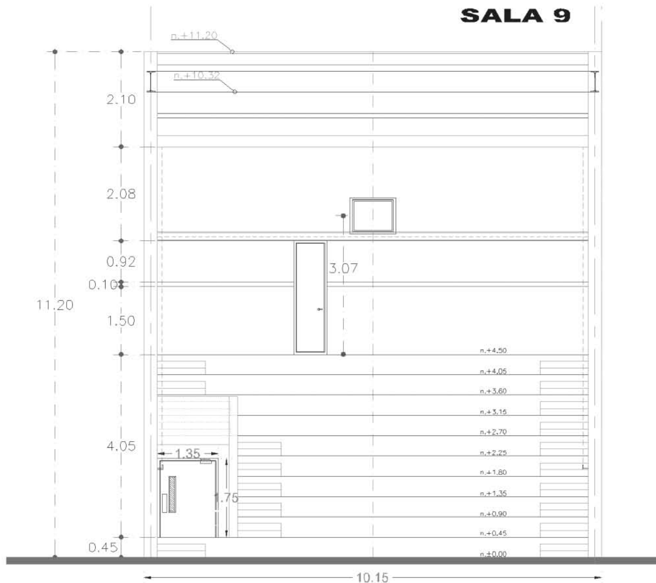
Ilustración 8. Vista posterior, Sala 9
