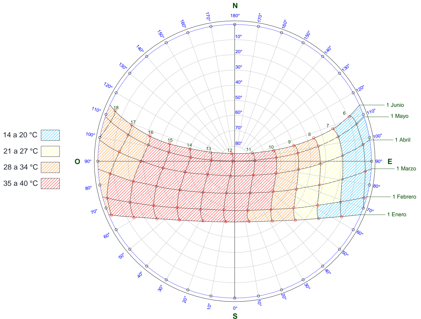
Ilustración 14. Gráfica solar equidistante con sombreado respecto a la temperatura promedio por hora y época del año. (Enero a Junio)
