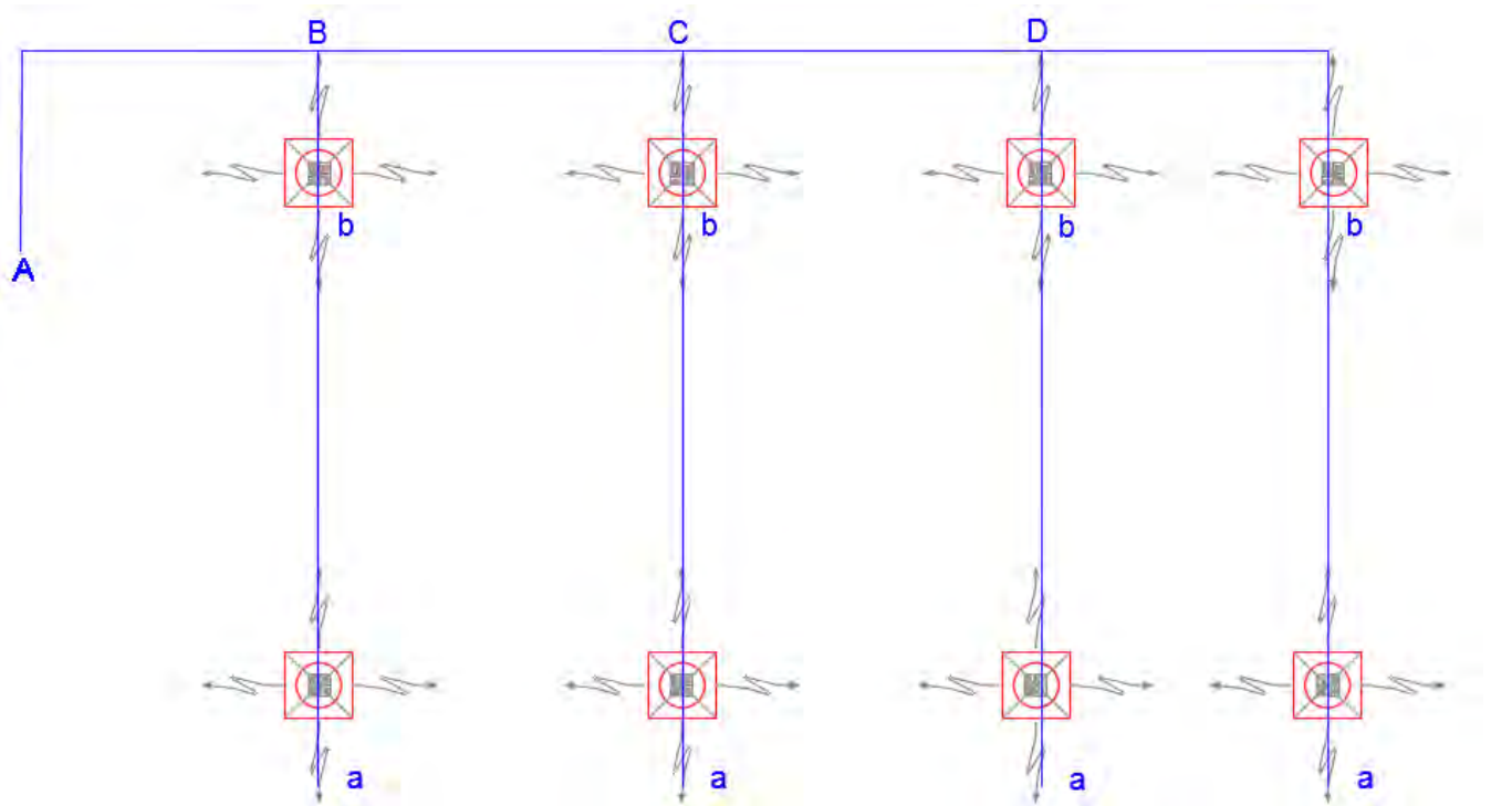
Ilustración 30. Esquema de la distribución de los ductos de inyección
