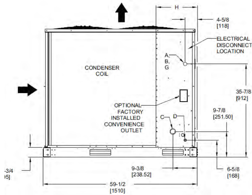
Ilustración 27. Vista lateral izquierda del equipo.
