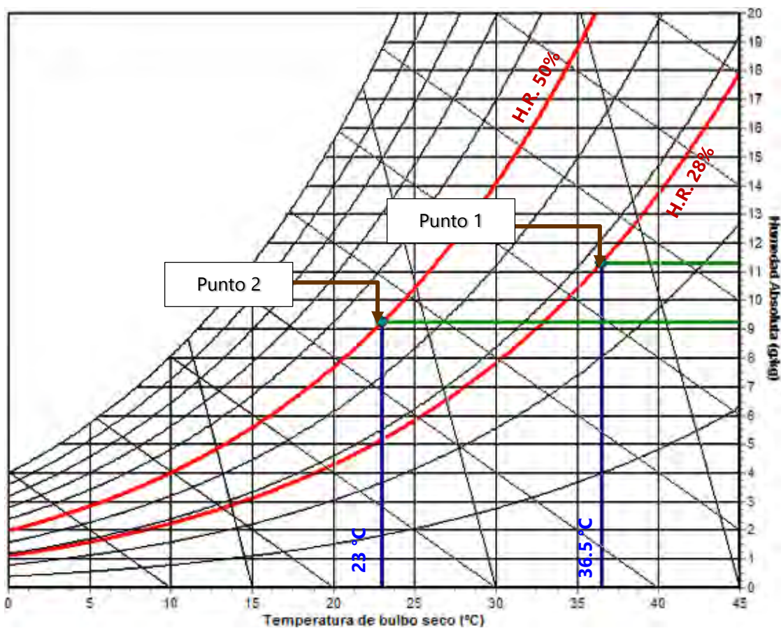
Ilustración 4. Carta Psicrométrica a 11 m.s.n.m, condiciones exterior e interior.
