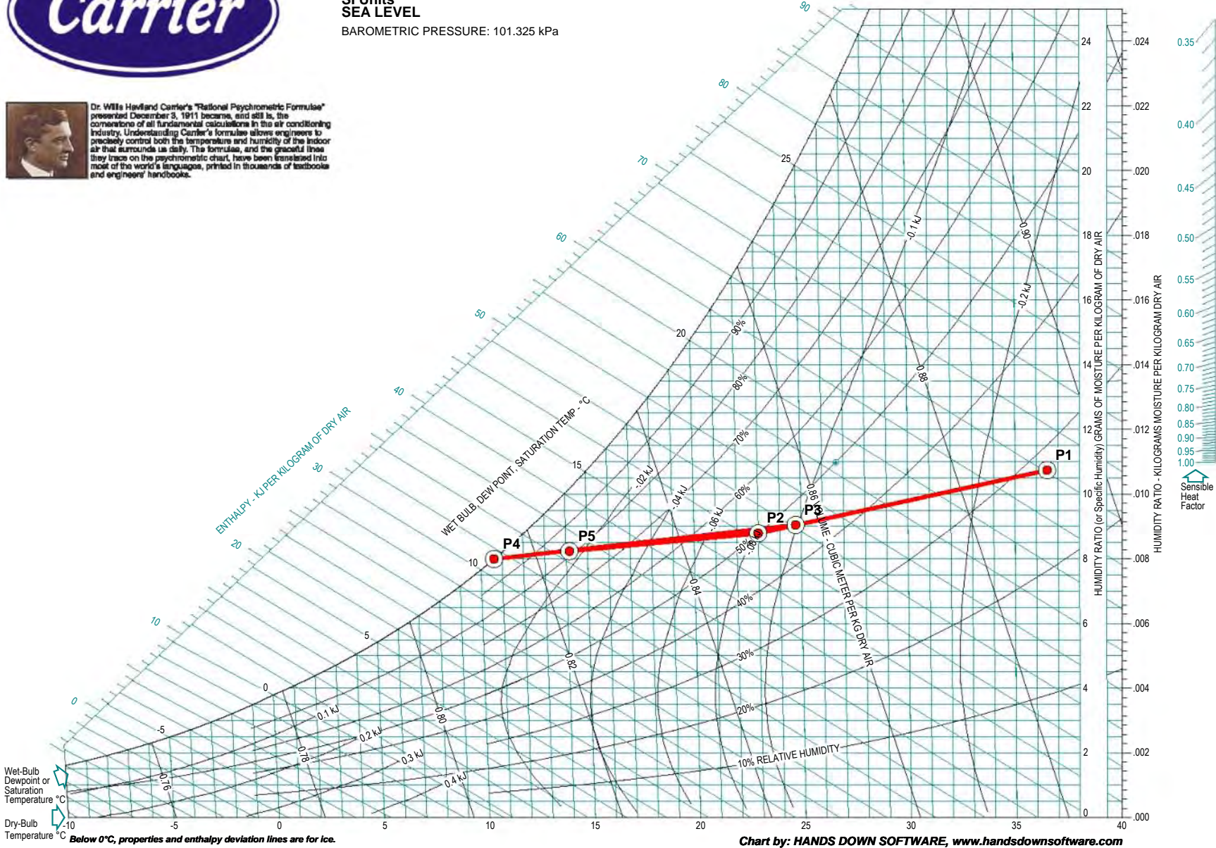
Ilustración 23. Proceso de climatización con los 5 estados indicados.
