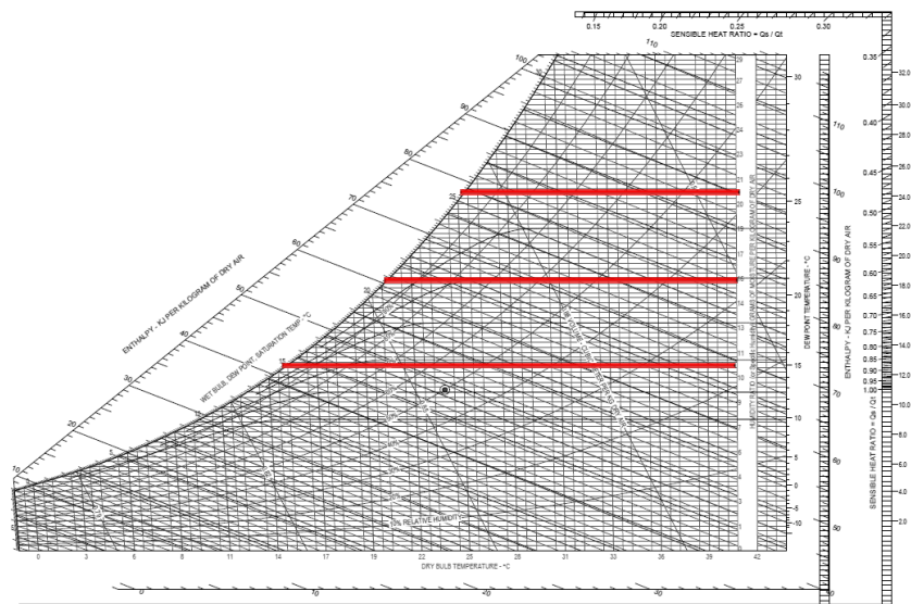
Ilustración 37. Líneas que representan la humedad absoluta o específica en la carta psicrométrica
