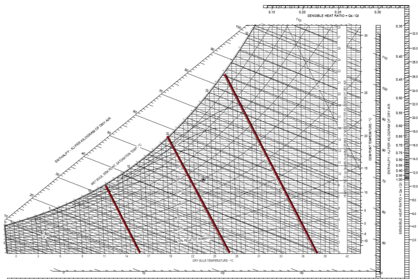
Ilustración 39. Líneas que representan el volumen específico en la carta psicrométrica.
