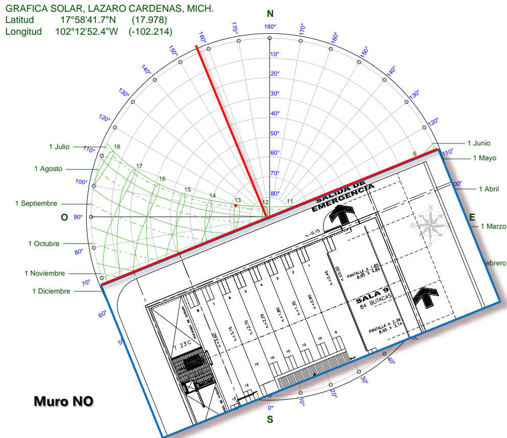
Ilustración 17. Gráfica solar con la ubicación del sol y la superficie del proyecto.
