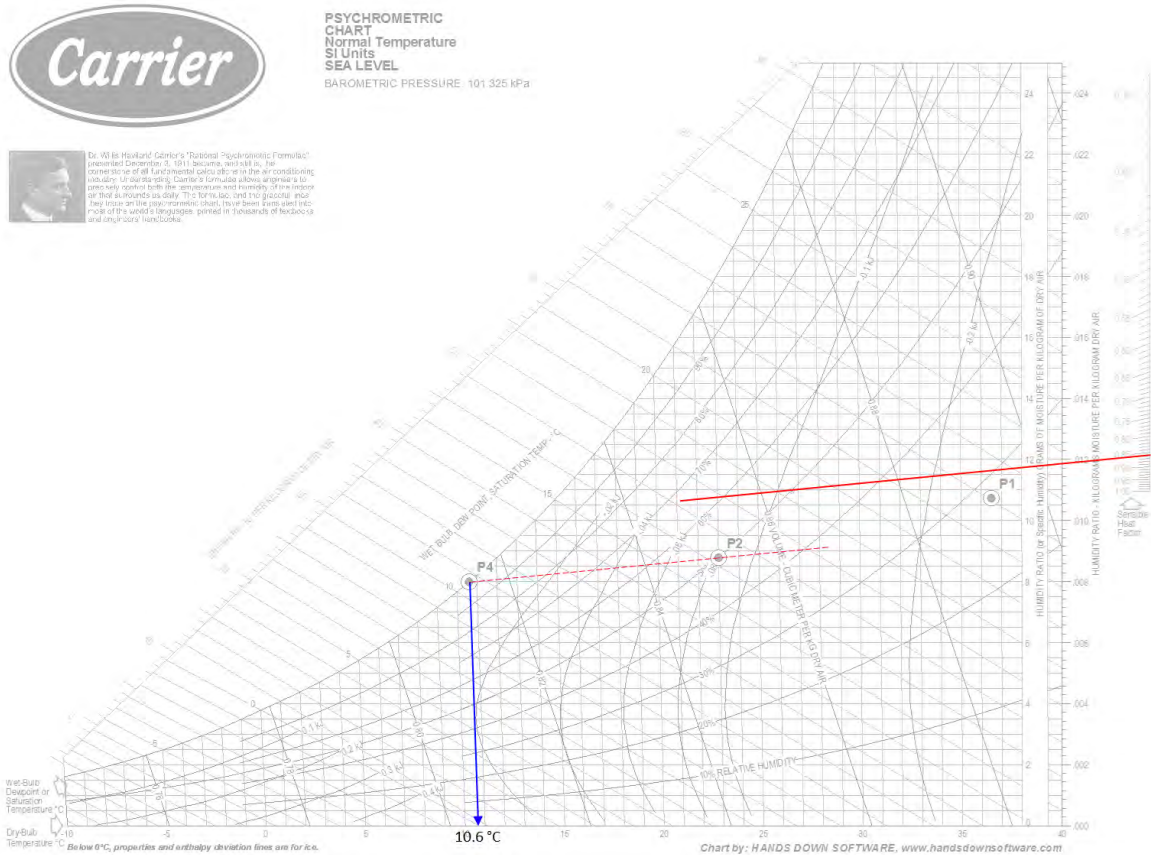
Ilustración 22. Forma gráfica de obtener el punto (4) en el diagrama psicrométrico. Fuente: Elaboración propia
