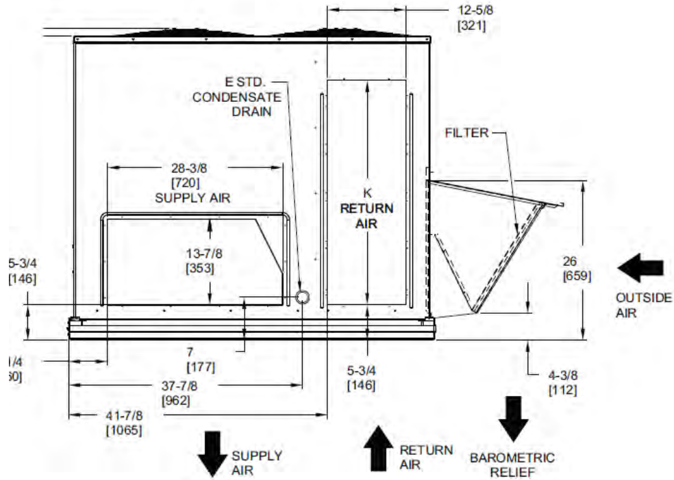
Ilustración 28. Vista lateral derecha del equipo. Fuente: Ficha técnica Unidad tipo Paquete de Carrier
