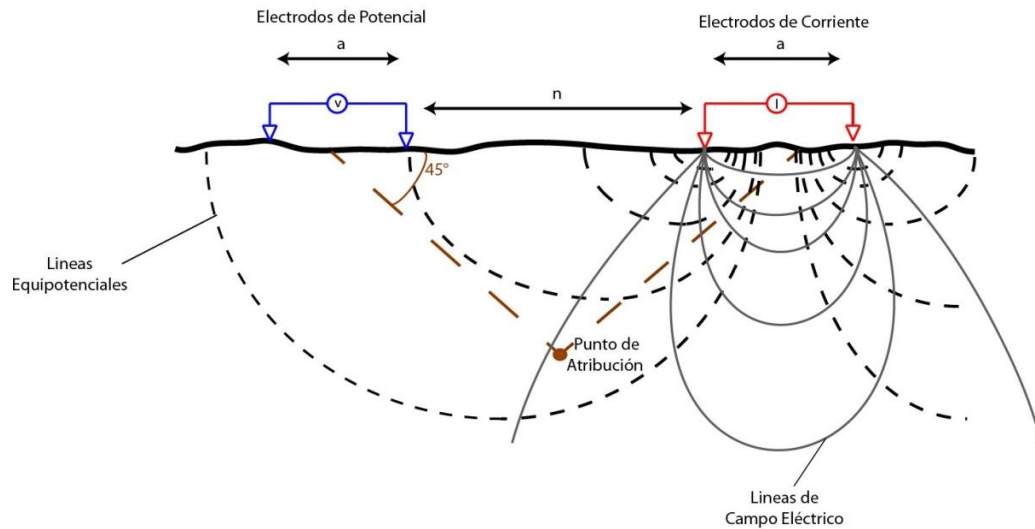
Figura 6. Electrodos de corriente y de potencial, que se van separando conforme se requiera la profundidad de investigación. Imagen modificada de http://geotech.mex.tl/986328_geofisica.html .
