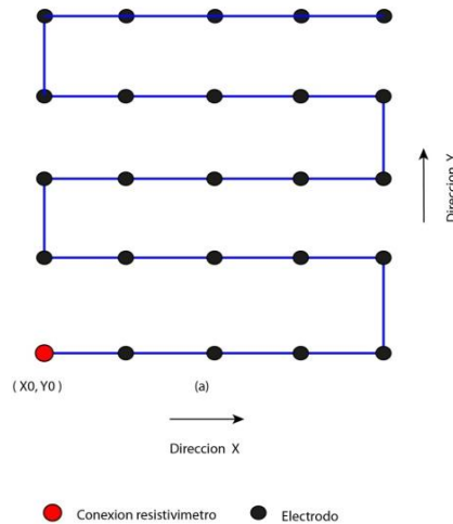
Figura 7 Ubicación de los electrodos a lo largo de un cable multi-electrónico para un levantamiento 3D de resistividad (imagen tomada y modificada Loke (1996a)).
