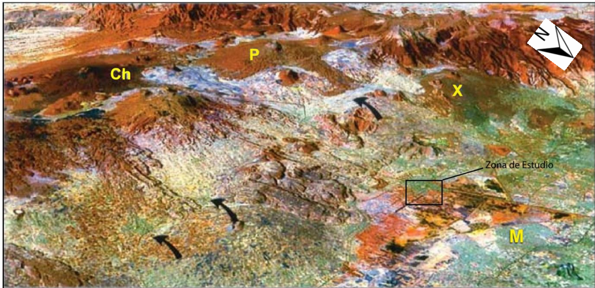
Figura 12. Imagen de Satélite LANDSAT con perspectiva hacia el SW se puede ubicar el volcán Xitle (X) y la extensión del pedregal así como parte de la SCN. M=ciudad de México, Ch= Volcán Chichinautzin, P= Volcán El Pelado, las flechas indican la traza de una falla normal con dirección E-W (Imagen tomada y modificada de Siebe, 2009).
