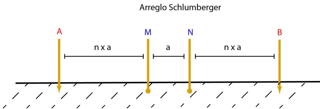
Figura 4. Esquema de la Configuración Electrónica Schlumberger.
